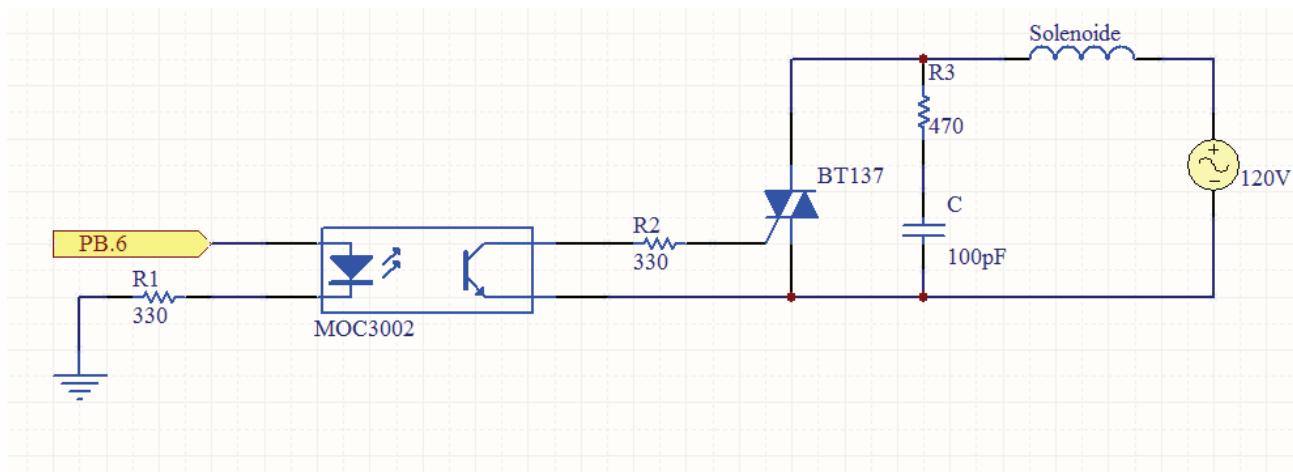
Figura 90 Etapa de potencia para el solenoide, basado en un optoacoplador y un triac.
