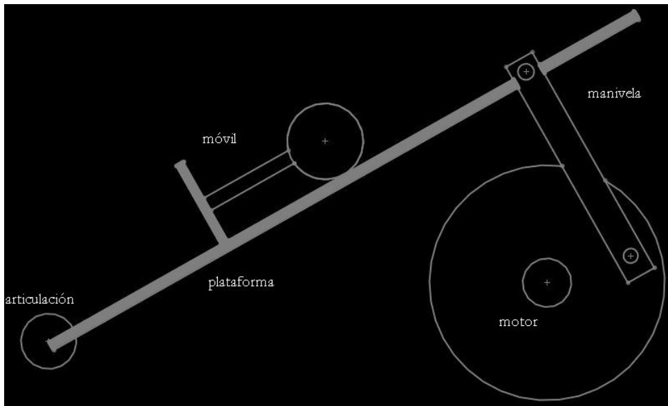
Figura 2 Esquema del subsistema manivela.
