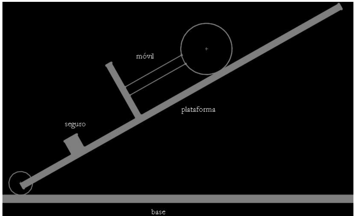
Figura 14 Esquema del subsistema seguro.
