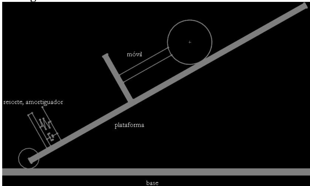
Figura 18 Esquema del subsistema resorte-amortiguador.
