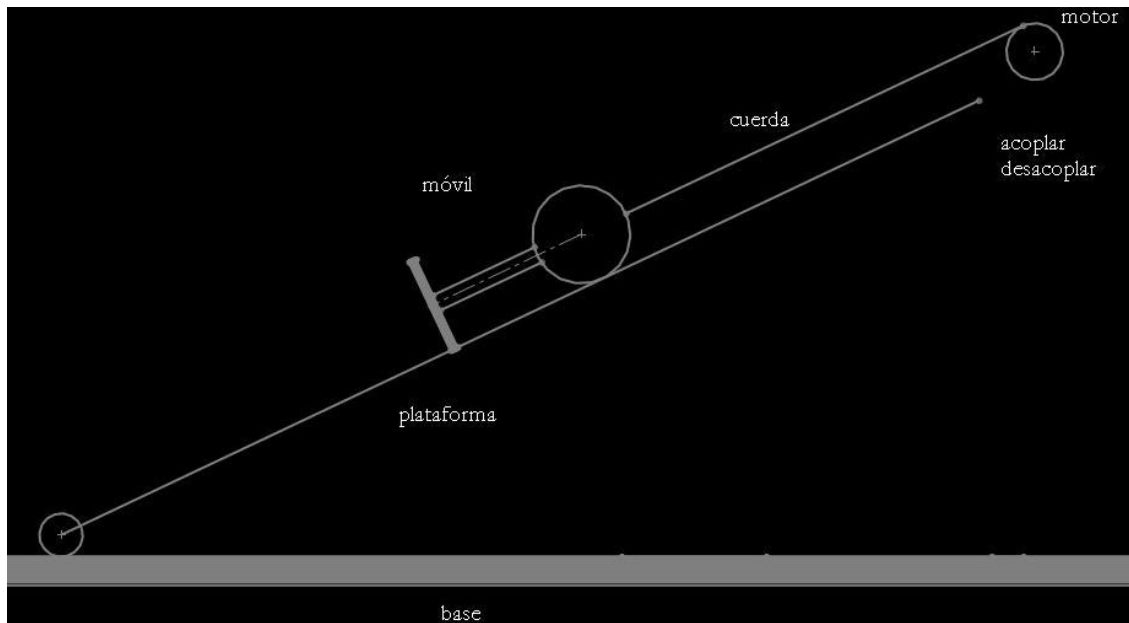
Figura 11 Esquema del subsistema acoplamiento.
