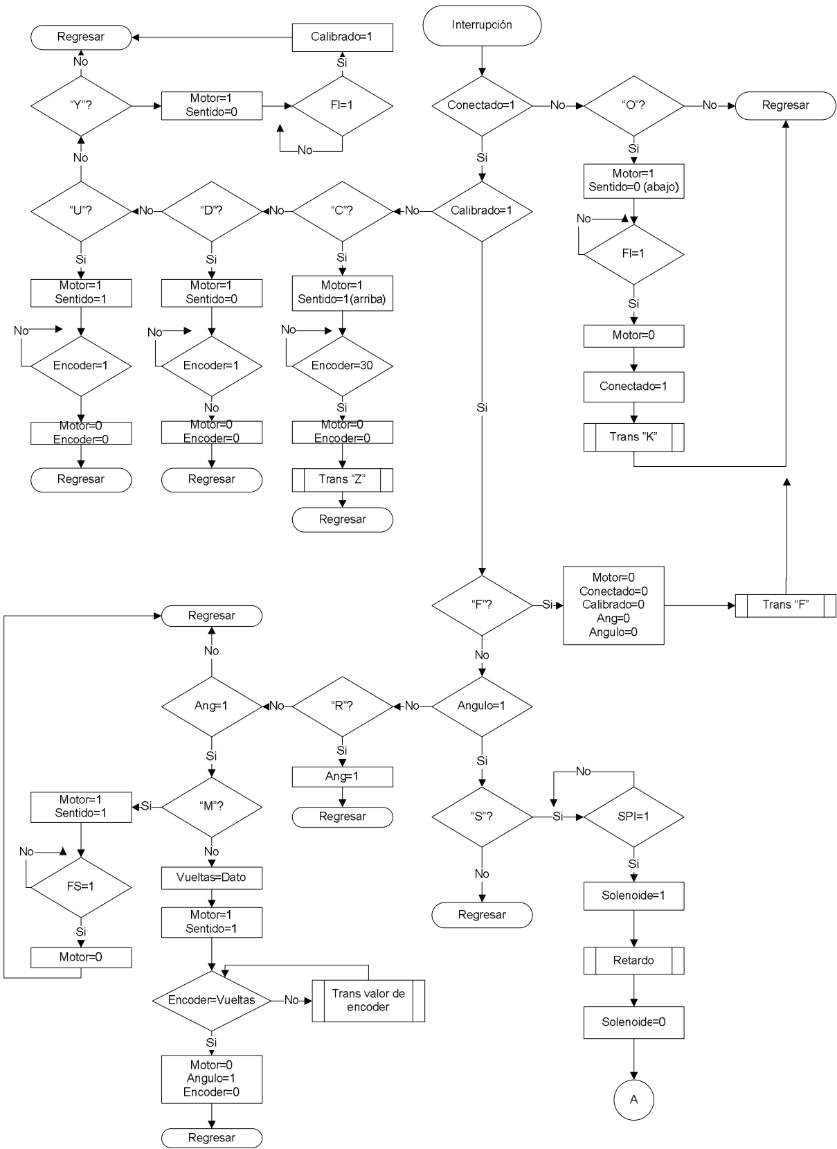
Figura 96 Diagrama de flujo de la interrupción del programa del microcontrolador.
