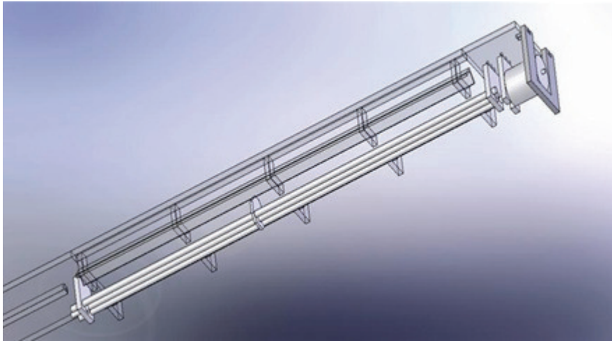
Figura 53 Subsistema completo del esparrago acoplado a la plataforma.
