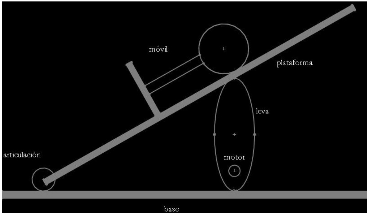
Figura 6 Esquema del subsistema leva.
