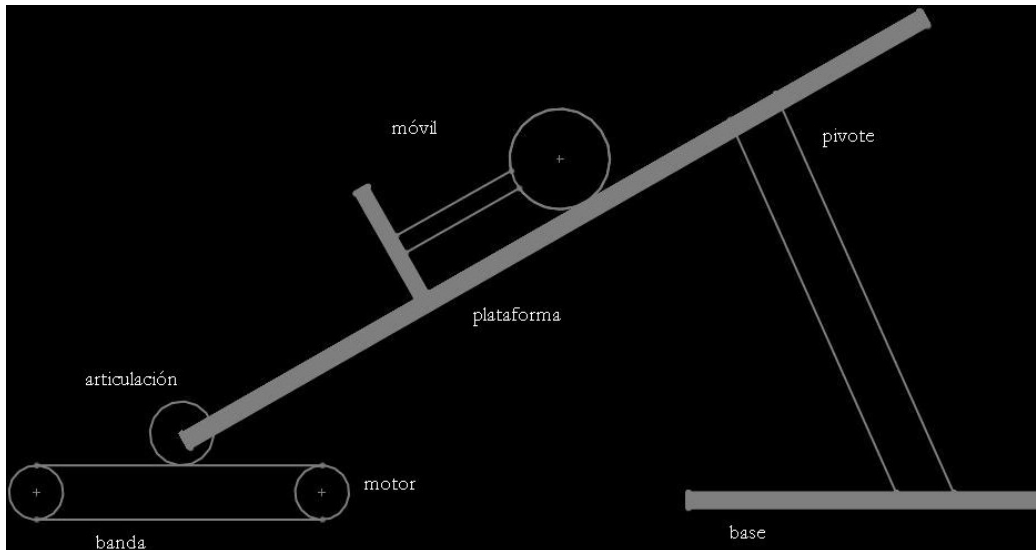
Figura 3 Esquema del subsistema banda-pivote.
