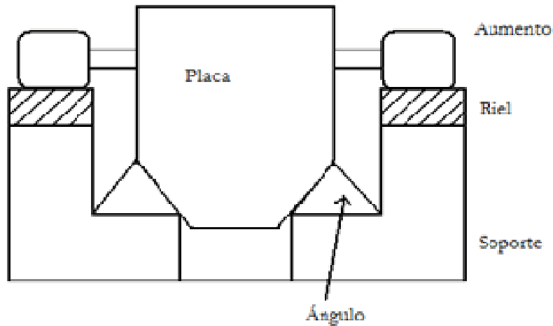
Figura 36 Esquema de la configuración final de la plataforma.
