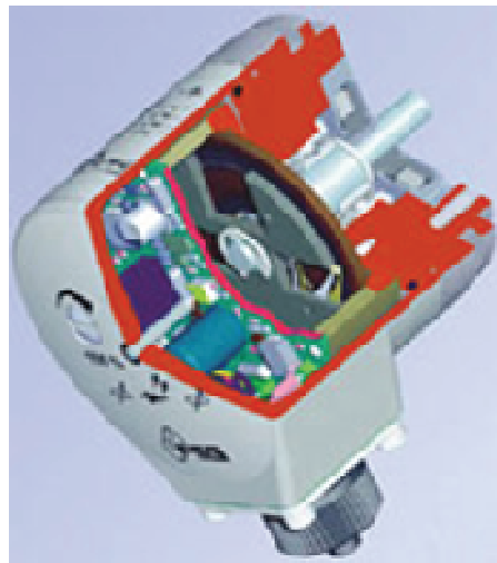
Figura 26 Potenciómetro rotativo.
