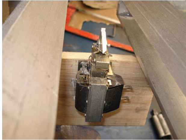
Figura 79 Solenoide-trinquete.
