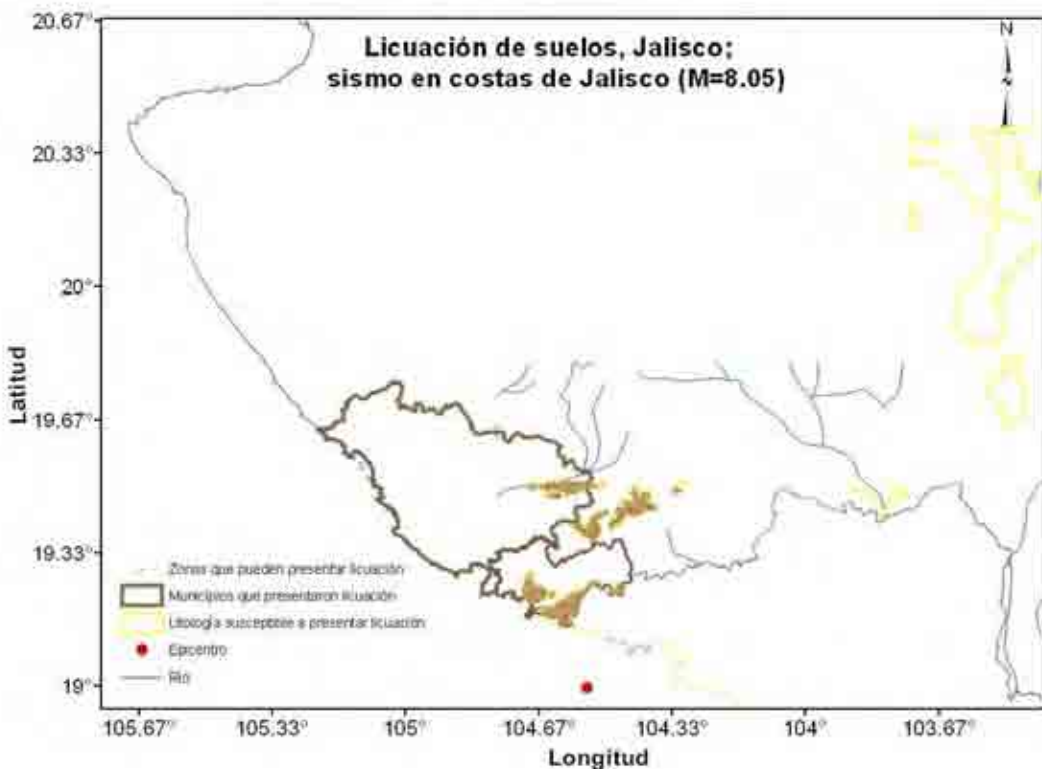
Figura 4.6 a) Mapa de datos bibliográficos, litología y pendientes de la zona sur de Jalisco .b) Mapa de datos bibliográficos, litología, pendientes y aceleraciones mayores a 0.15 de g para un evento de M= 8.05. c) Zonas susceptibles a licuación obtenidos de la intersección de litologías, aceleraciones mayores a 0.15 de g (por un evento de M=8.05) y pendientes.
