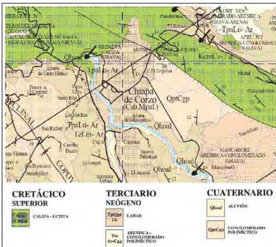
Figura 2.21. Geología del área de Chiapa de Corzo. SGM (2009)
