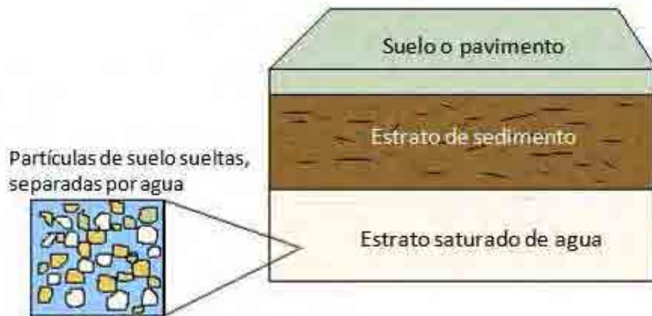
Figura 1.1. Estado de esfuerzos entre partículas antes de la aplicación de carga cíclica
