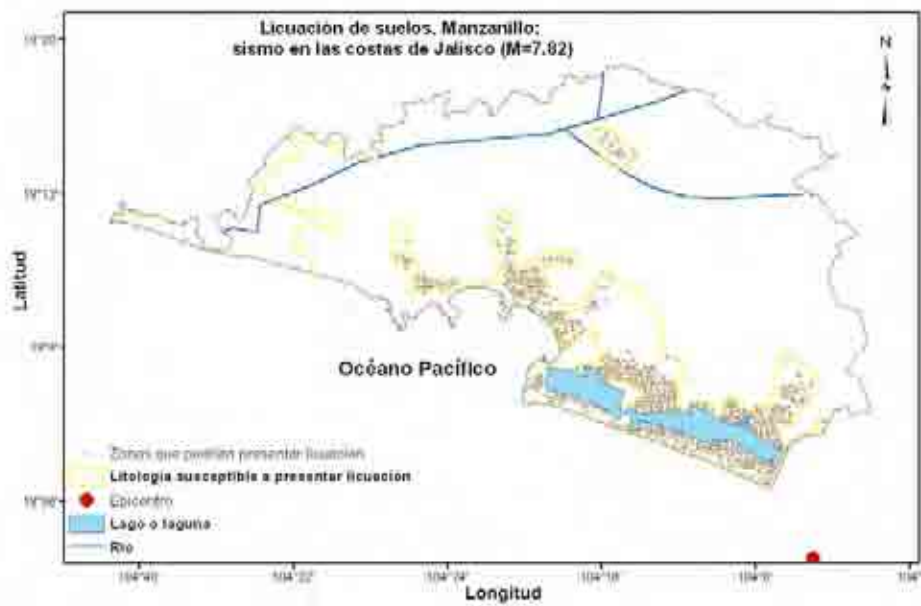
Figura 5.6 a) Mapa de pendientes y litología susceptible a licuación en el área de la Bahía de Manzanillo. Se observan sitios en color verde claro en donde si se relaciona ésta figura con la 5.5 se observan zonas planas de depósitos aluviales. b) Mapa de datos bibliográficos, litología, pendientes y aceleraciones mayores a 0.15 de g para un evento de M=7.82 . c) Zonas susceptibles a licuación, datos obtenidos de la intersección de litologías, aceleraciones mayores a 0.15 de g (por un evento de M=7.82 ) y pendientes.
