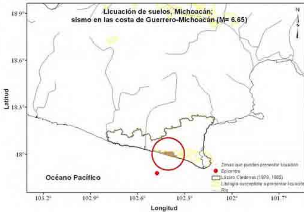
Figura 4.8 a) Mapa de datos bibliográficos, litología y pendientes de la zona de Michoacán. b) Mapa de datos bibliográficos, litología, pendientes y aceleraciones mayores a 0.15 de g para un evento de M= 6.65 , estas últimas se presentan en el área delimitada por el círculo rojo. c) Zonas susceptibles a licuación (enmarcadas por círculo rojo), datos obtenidos de la intersección de litologías, aceleraciones mayores a 0.15 de g (por un evento de M=6.65 ) y pendientes.
