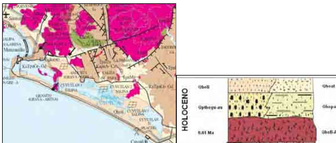
Figura 2.13. Geología de la zona de Manzanillo, Colima. (SGM, 2008)
