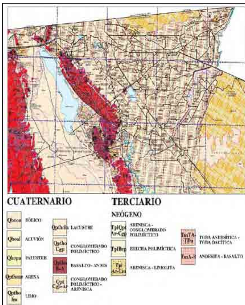
Figura 2.22. Geología del Valle de Mexicali. SGM (2008).
