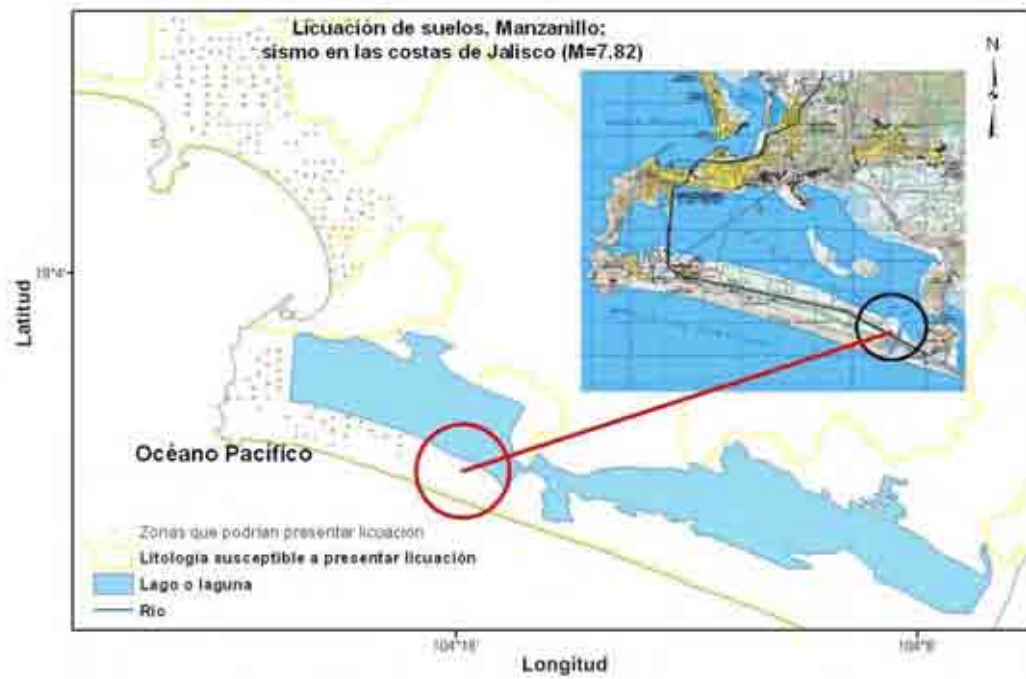
Figura 5.8 a) Localización de la zona de estudio mencionada en reporte de ERN (2009). Tomada de ERN (2009). b) Comparación con los resultados obtenidos en la figura 5.7b.
