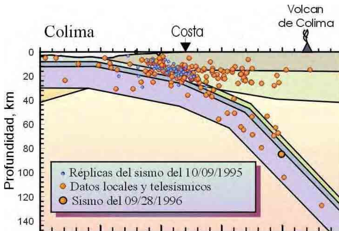
Figura 5.3 Se observa un modelo de la placa de Cocos subduciendo bajo la Norteamericana frente a las costas del estado de Colima, creado a partir de datos sísmicos de diferentes eventos. SSN (2003)
