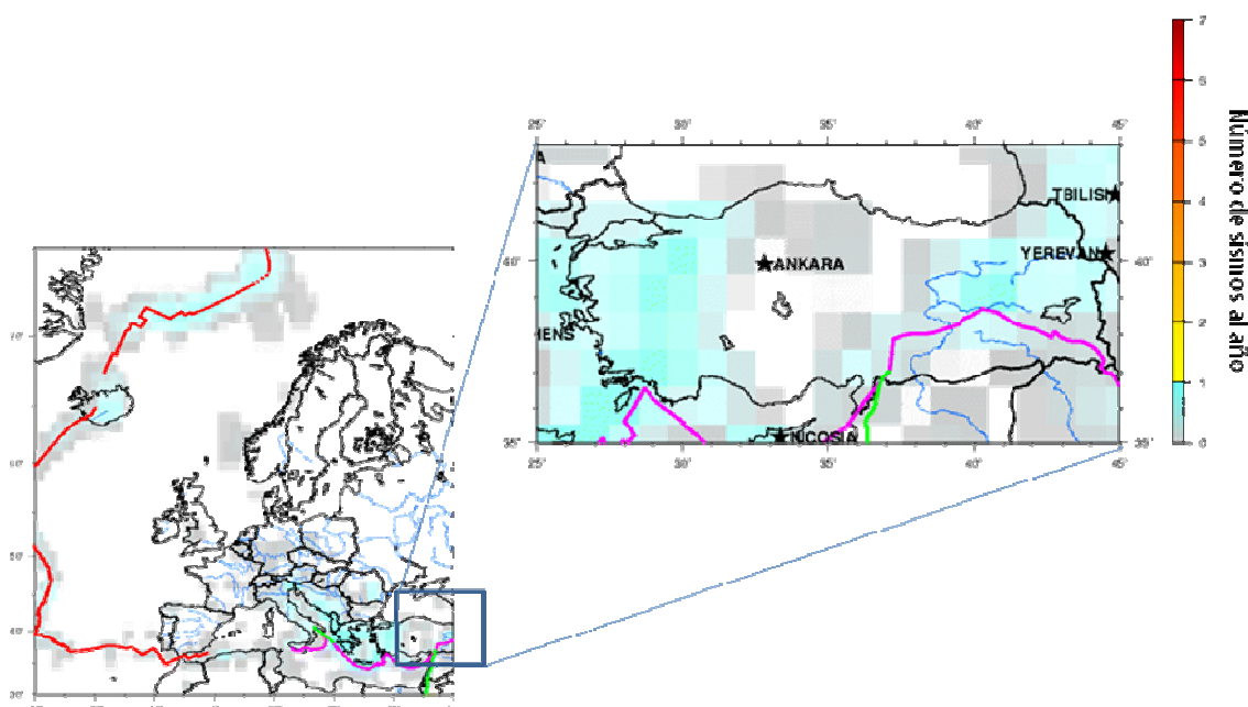
Figura 2.7 Densidad sísmica de la zona del Mar Mediterráneo y de Turquía, para su realización se tomaron eventos con magnitud 5 o más. Tomada y modificada del USGS ( www.usgs.gov )
