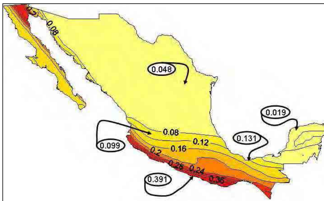
Figura 2.11. Mapa de regionalización sísmica, tomando en cuenta valores de aceleración máxima del suelo. (Pérez, et al., 2008 )
