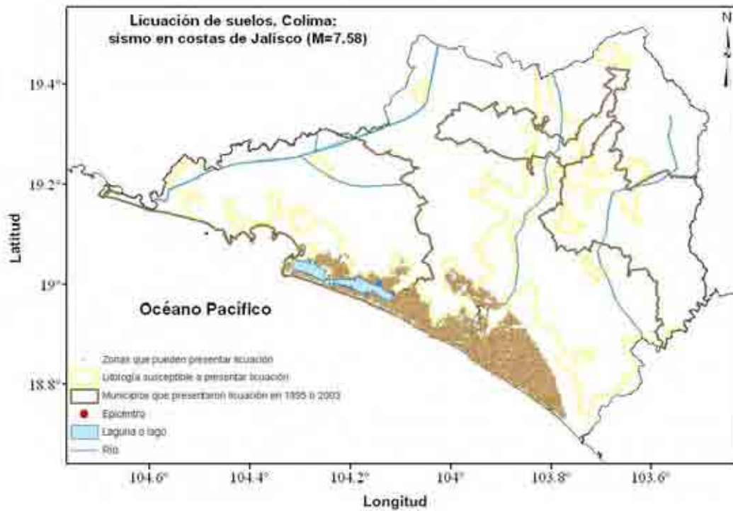
Figura 4.7 a) Mapa de datos bibliográficos, litología y pendientes de la zona de Colima. b) Mapa de datos bibliográficos, litología, pendientes y aceleraciones mayores a 0.15 de g para un evento de M=7.58 . c) Zonas susceptibles a licuación obtenidos de la intersección de litologías, aceleraciones mayores a 0.15 de g (por un evento de M=7.58 ) y pendientes.
