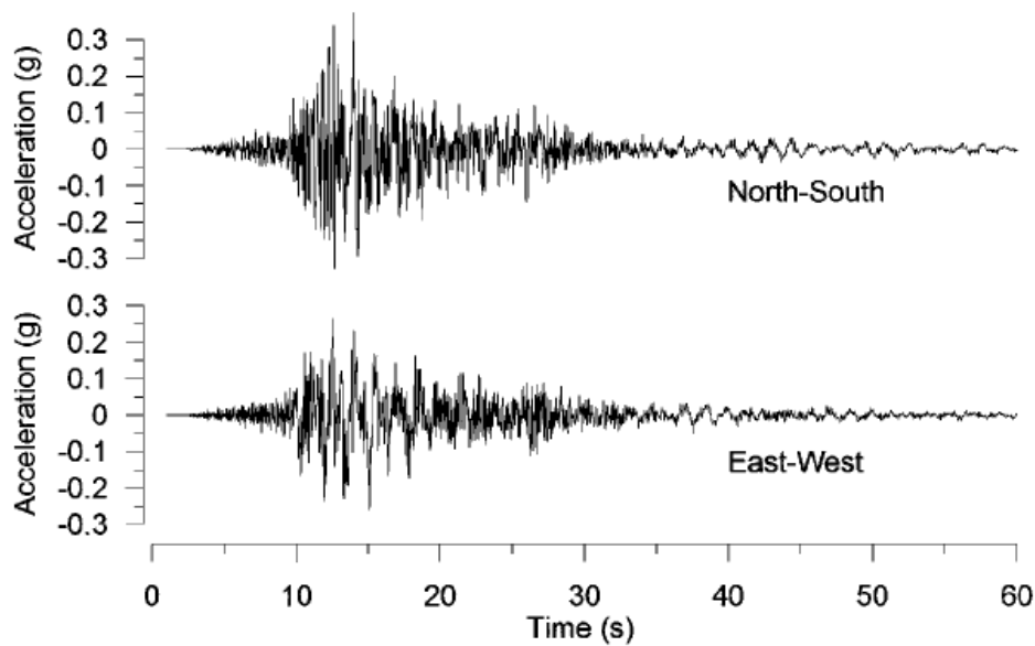
Figura 1.3. Acelerograma del sismo de Tecomán, Colima. Tomada de Wartman et al, 2003.
