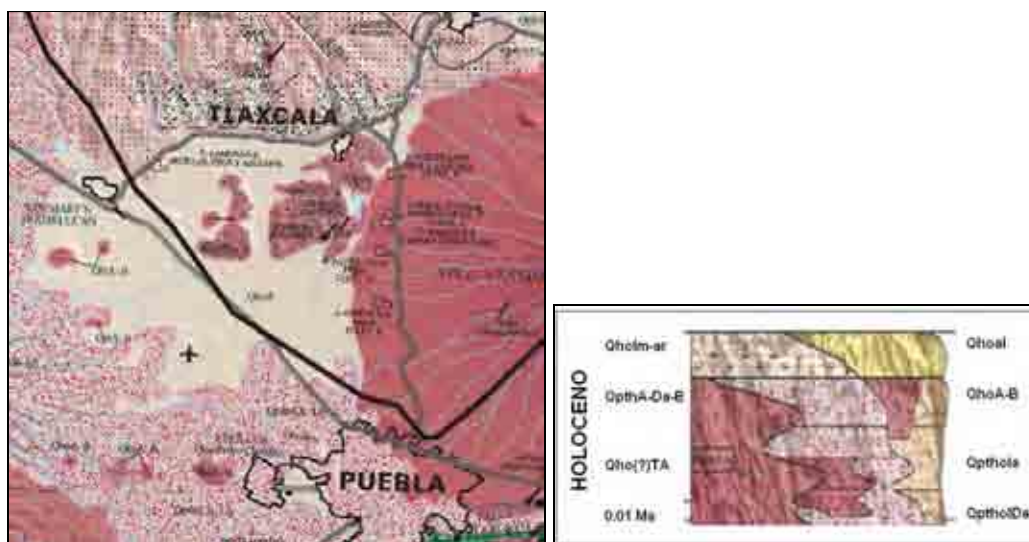
Figura 2.18. Geología de la región del Altiplano de Tlaxcala.(SGM, 2008)
