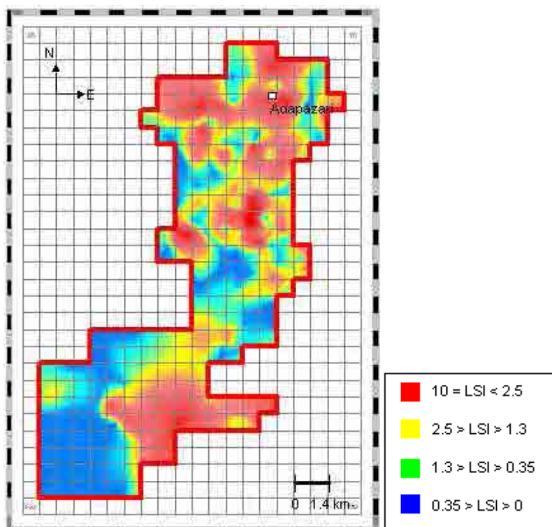
Figura 2.8 LSI calculado en un SIG para la ciudad de Sakarya. Tomada de Yilmaz y Celtin (2004).
