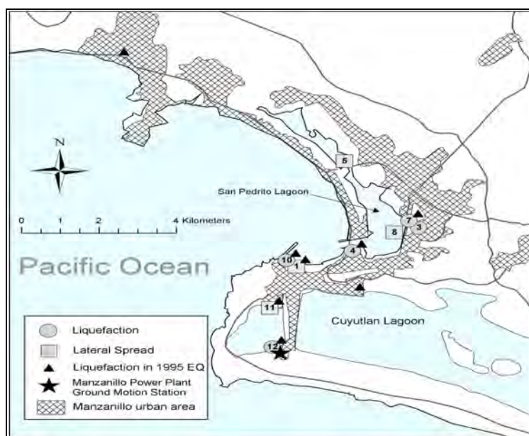
Figura 2.14. Mapa comparativo de zonas que presentaron licuación de arenas durante los sismos de Manzanillo (1995) y Tecomán (2003). ( Wartman, et al., 2003 )
