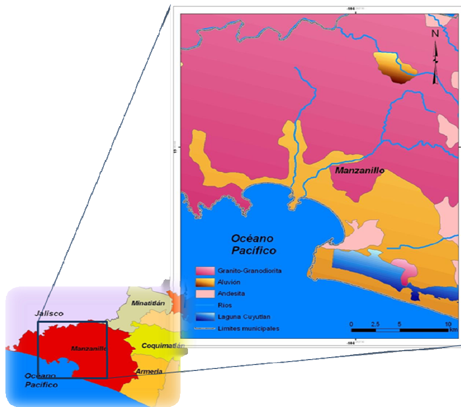
Figura 5.5 Litología del área de la Bahía de Manzanillo. En la parte sur-este predominan los depósitos aluviales.
