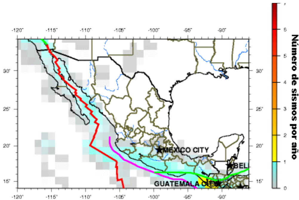
Figura 4.1. Sismos con magnitud 5.0 o más en México. En color morado las zonas de subducción, en rojo las de dorsales y en verde las de fallas transformantes. Modificado del SUGS.
