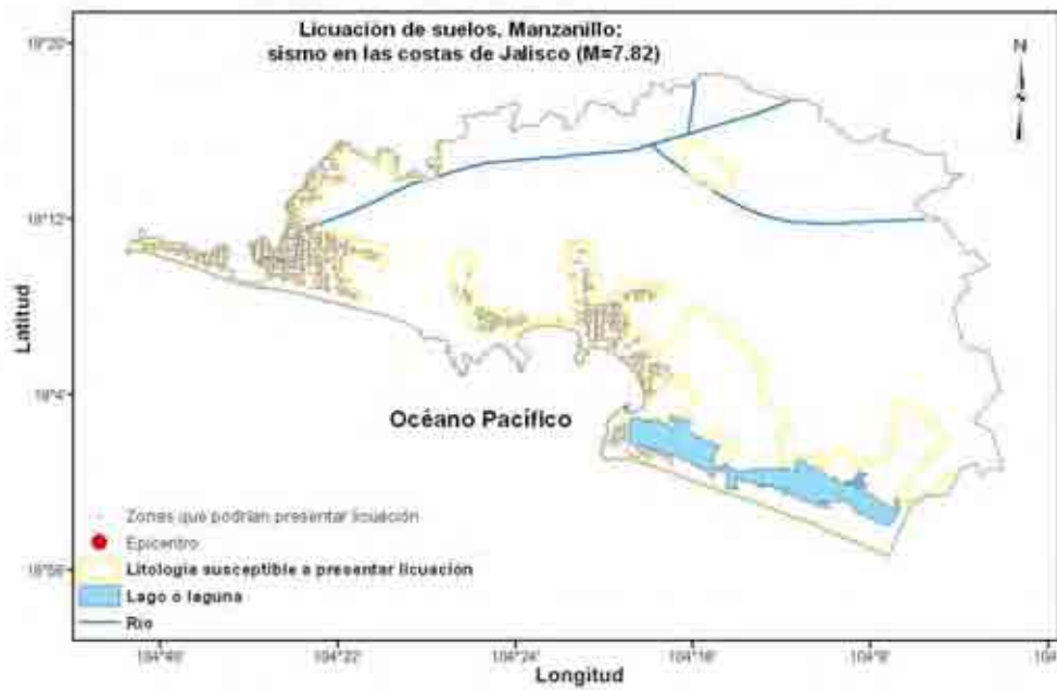
Figura 5.7 a) Mapa de datos bibliográficos, litología, pendientes y aceleraciones mayores a 0.15 de g para un evento de M= 7.82. b) Zonas susceptibles a licuación, datos obtenidos de la intersección de litologías, aceleraciones mayores a 0.15 de g (por un evento de M=7.82) y pendientes.
