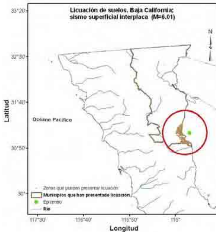
Figura 4.5 a) Mapa de datos bibliográficos, litología, pendientes y aceleraciones mayores a 0.15 de g para un evento de M=6.01 , estas últimas se presentan en el área delimitada por el círculo rojo. b) Zonas susceptibles a licuación en el estado de Baja California, datos obtenidos de la intersección de litologías, aceleraciones mayores a 0.15 de g (por un evento de M=6.01 ) y pendientes.
