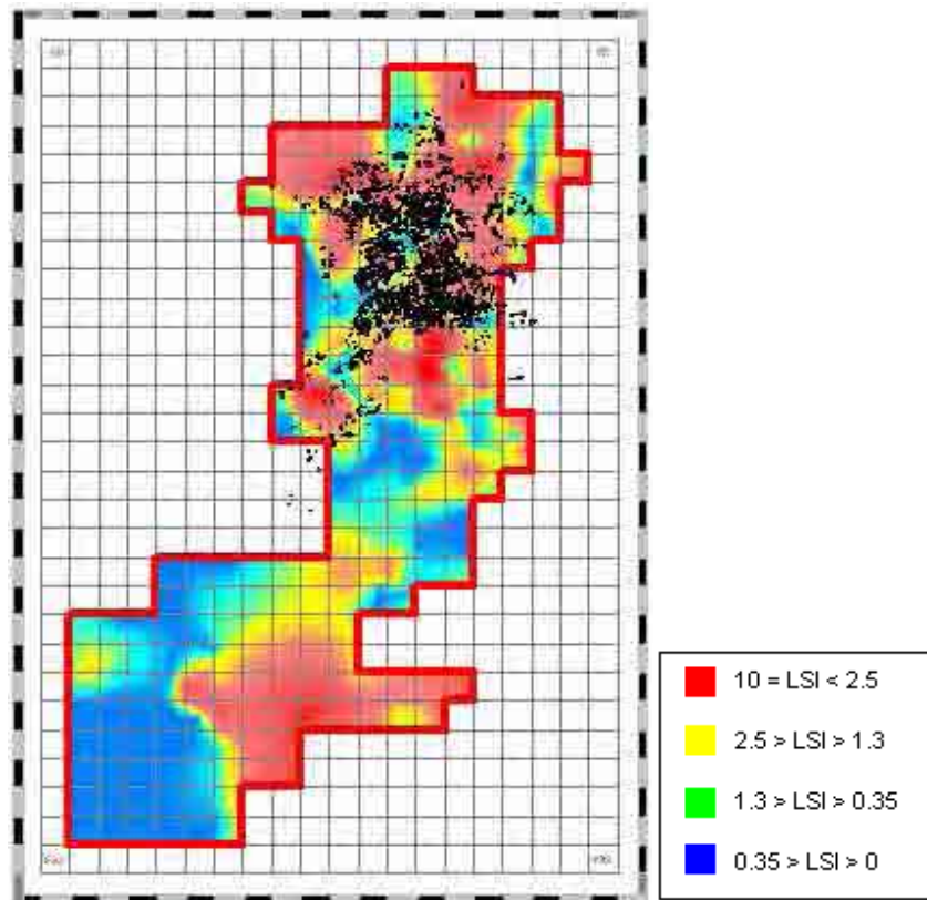
Figura 2.9 Comparación de los datos obtenidos del LSI calculado en un SIG y la distribución de daños después del sismo de Kocaeli para la ciudad de Sakarya. Tomada de Yilmaz y Celtin (2004).
