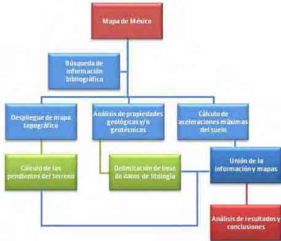
Figura 4.2. Fases para la obtención de mapas de peligro por licuación del suelo debido a un sismo
