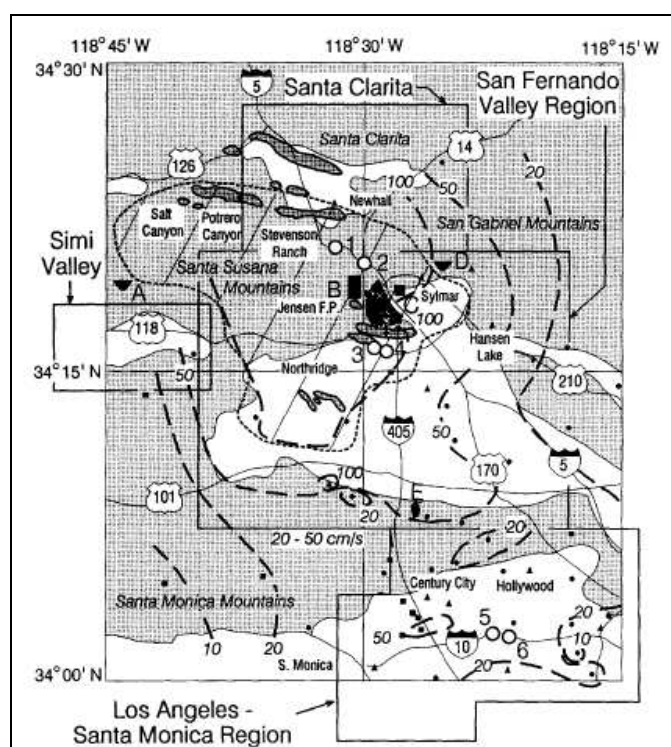
Figura 2.4 Mapa de velocidades pico del suelo (cm/s) durante el sismo de Northridge, 1994. Área de Los Ángeles y Valle de Santa Mónica. (Tomada de Trifunac, et al., 1998 )
