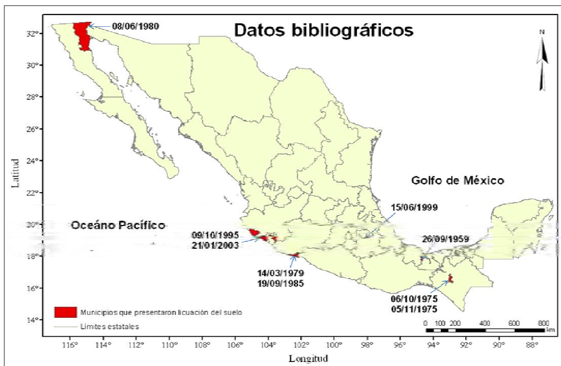
Figura 2.20 Representación gráfica de los lugares en donde se ha registrado licuación de suelo, de acuerdo a la bibliografía.
