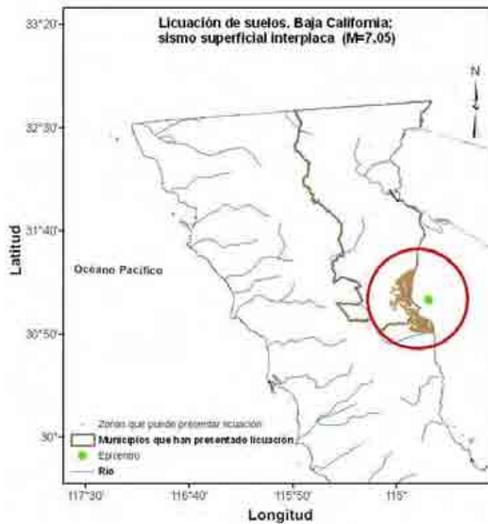
Figura 4.4 a) Mapa de datos bibliográficos, litología y pendientes del municipio de Mexicali .b) Mapa de datos bibliográficos, litología, pendientes y aceleraciones mayores a 0.15 de g para un evento de M= 7.05, estas últimas se presentan en el área delimitada por el círculo rojo. c) Zonas susceptibles a licuación en el estado de Baja California, datos obtenidos de la intersección de litologías, aceleraciones mayores a 0.15 de g (por un evento de M=7.05) y pendientes.
