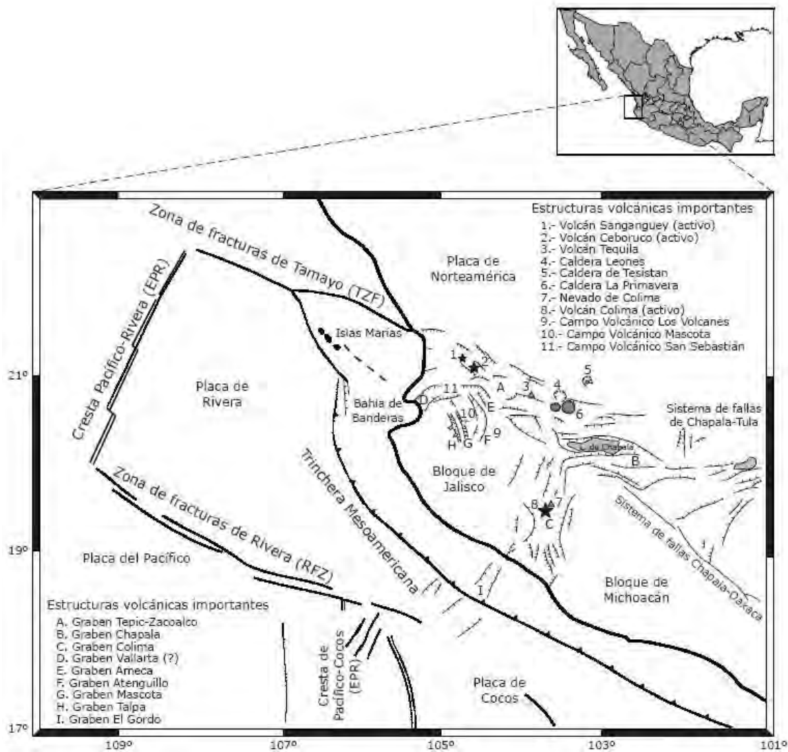
Figura 5.4 Límites del bloque de Jalisco donde se observan el graben de Colima y el graben El Gordo. Se aprecian también las principales estructuras volcánicas de la zona. (Rutz et al, 2004)
