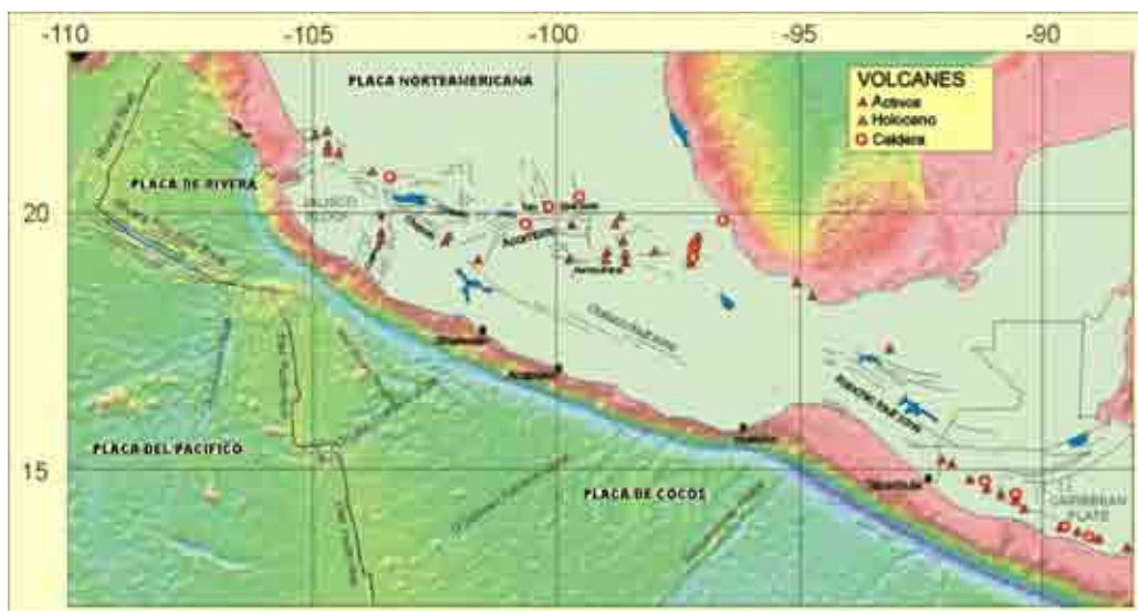
Figura 5.2 Se muestran los límites de la placa de Cocos obtenidos a partir de batimetría. Modificada de lacaeelel.igeofcu.unam.mx/.../mextec.html
