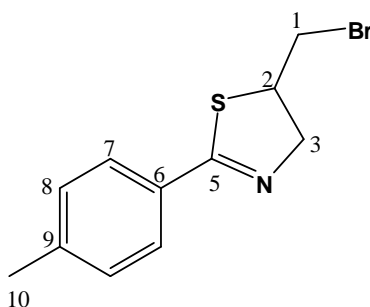
5-(bromometil)-2-(4-metilfenil)tiazolina (4d)
