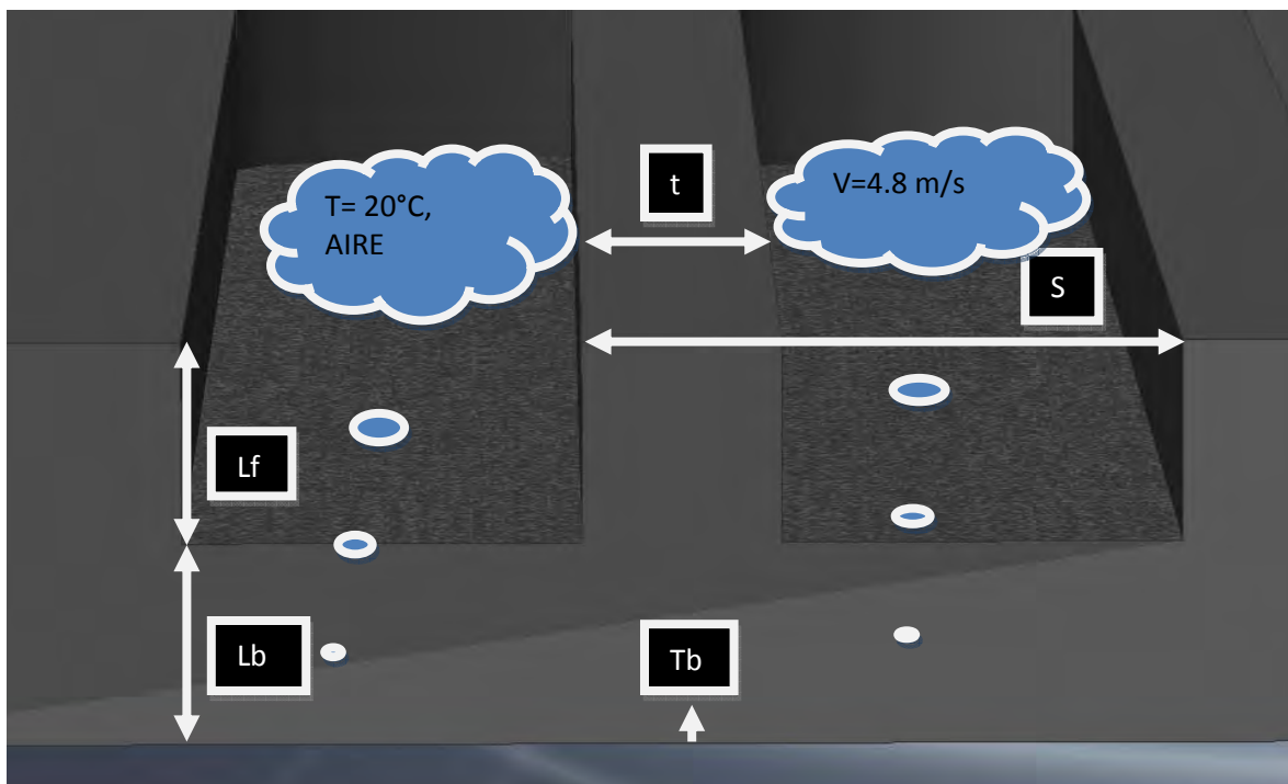
Esquema para el planteamiento del problema y obtención de datos geométricos y de operación.
