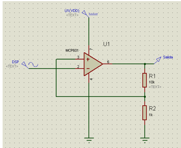
Figura 4.12, Comparador implementado.
