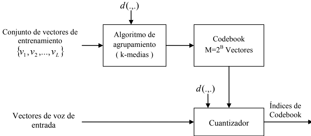
Figura 2.8, Diagrama de bloques de un VQ básico, entrenamiento y estructura de clasificación
