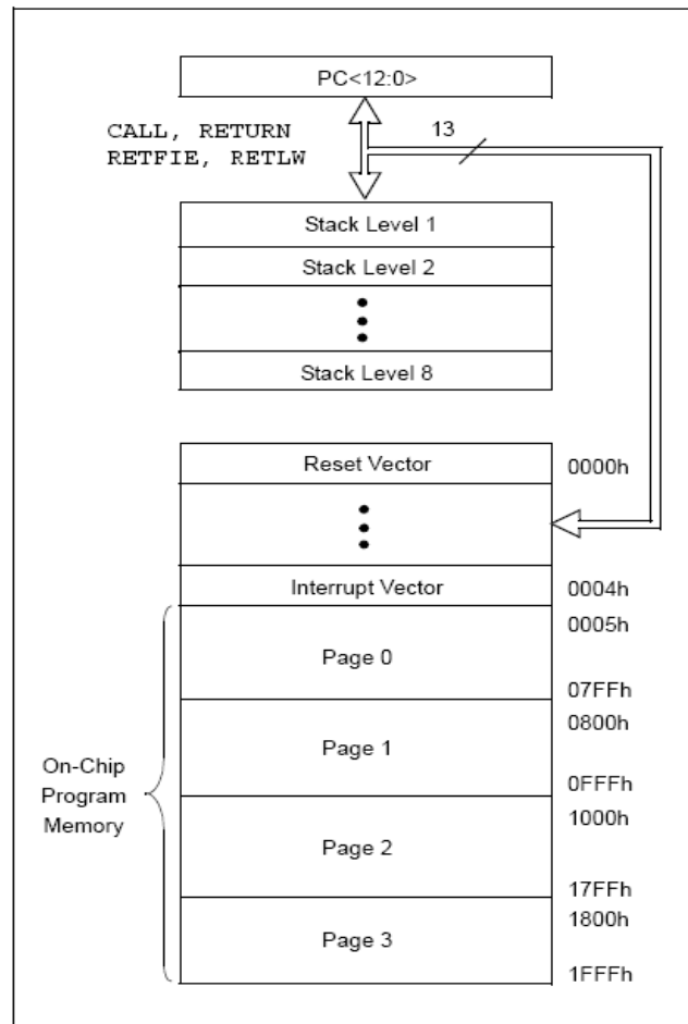
Figura 3.11 , Mapa de memoria de programa y pila del PIC 16F877A.
