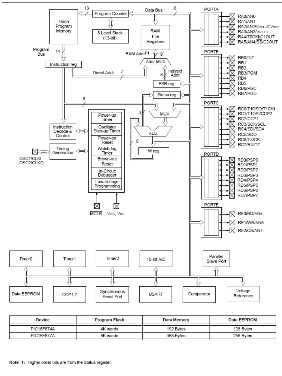
Figura 3.10, Diagrama de bloques del PIC 16F877A.
