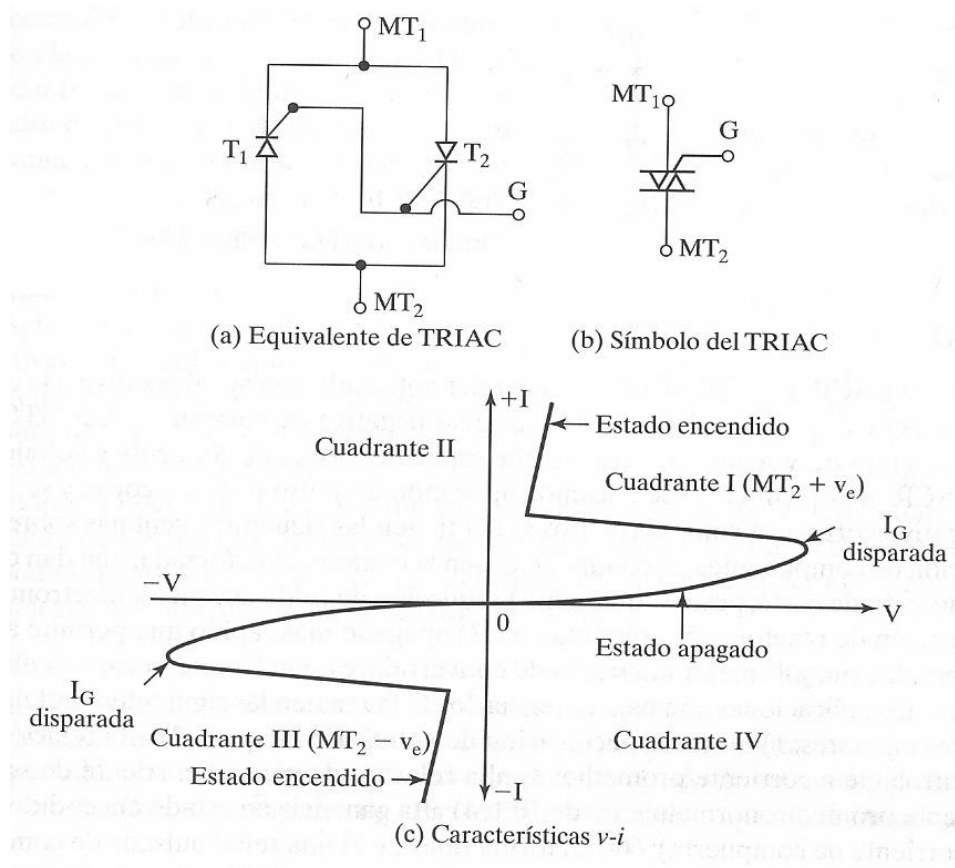
Figura 4.16, Comportamiento del triac en los diferentes cuadrantes.
