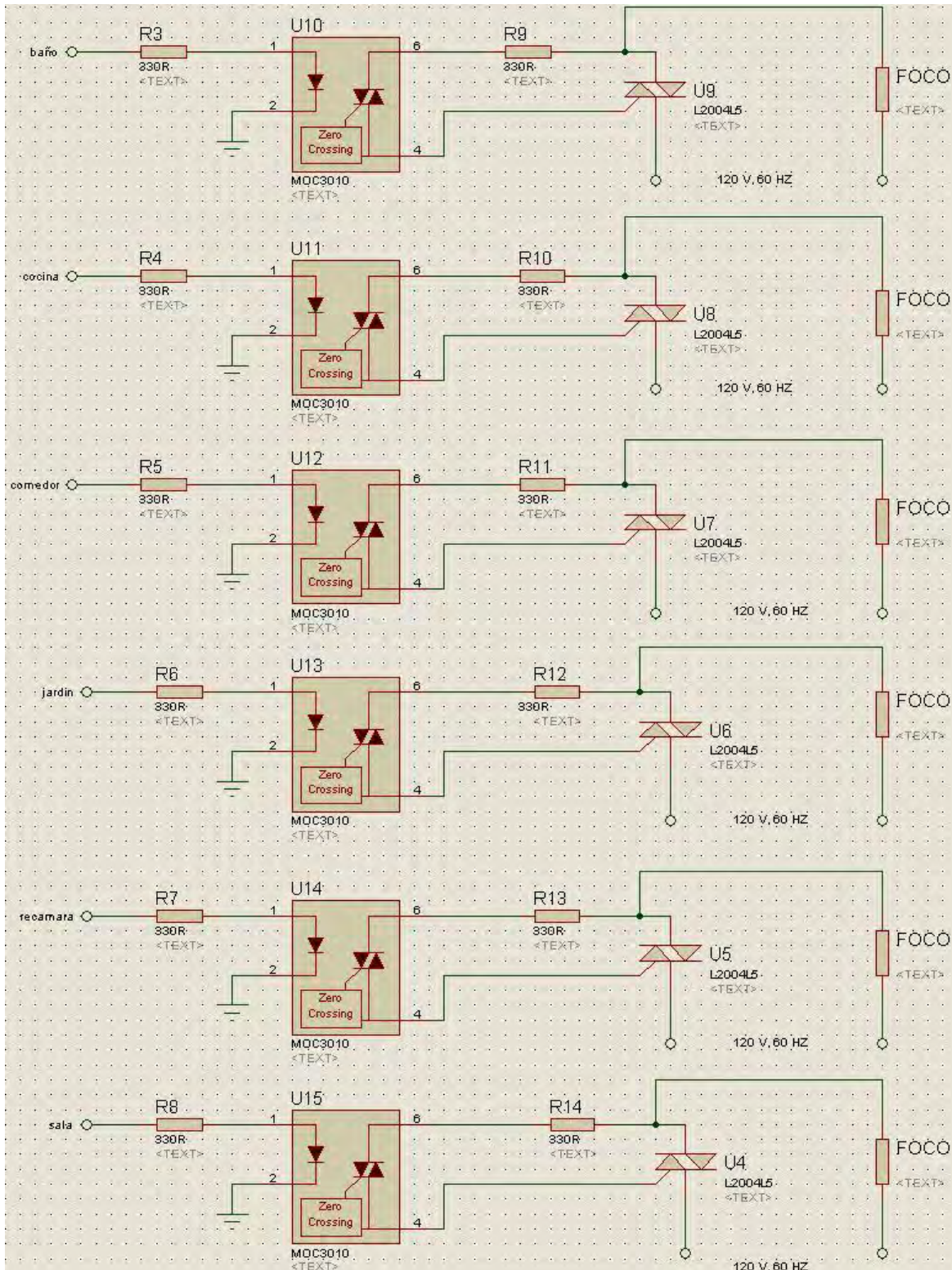
Figura 4.21, Esquemático del circuito electrónico de potencia.
