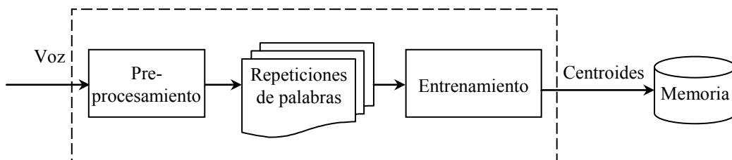
Figura 2.1, Etapa de Entrenamiento
