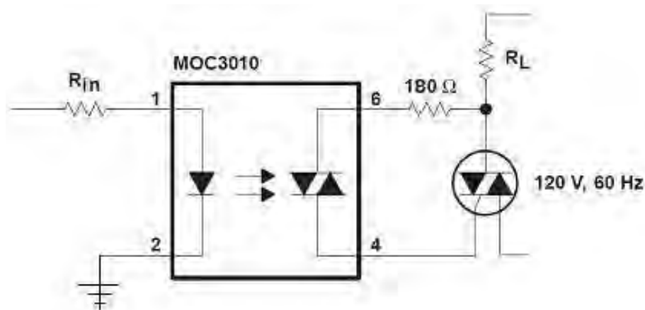
Figura 4.18, Diagrama de conexiones utilizado para el optoacoplador.
