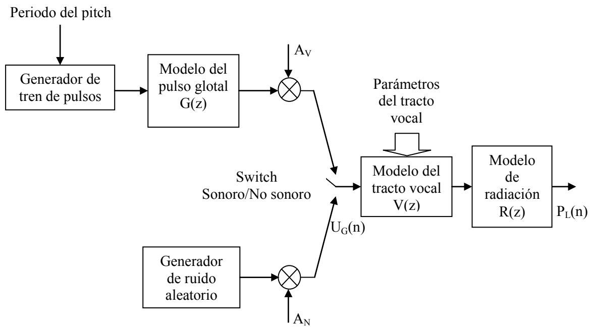
Figura 1.3, Modelo digital para la voz
