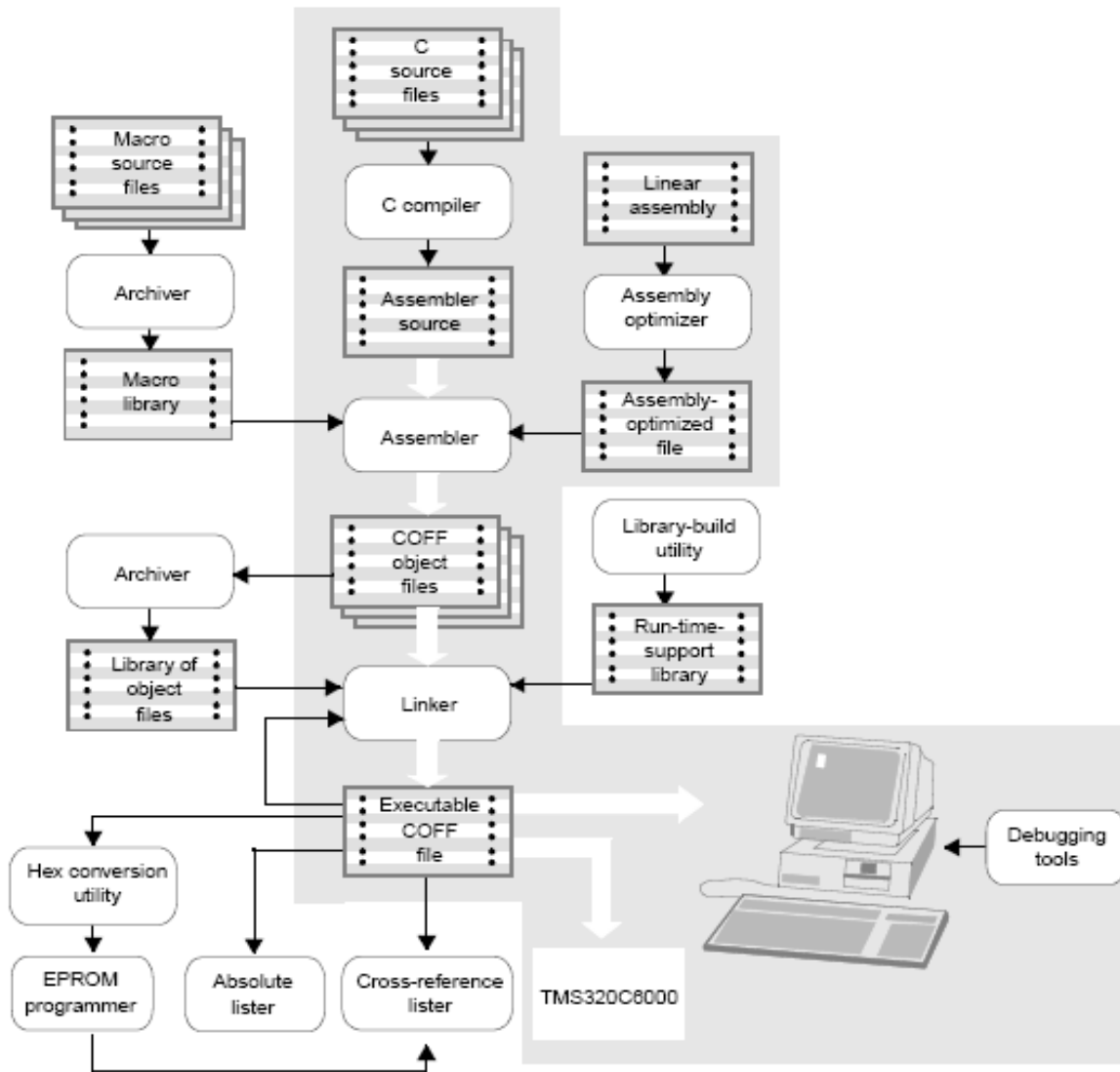
Figura 3.6, Flujo para el desarrollo de aplicaciones con los DSP C6000
