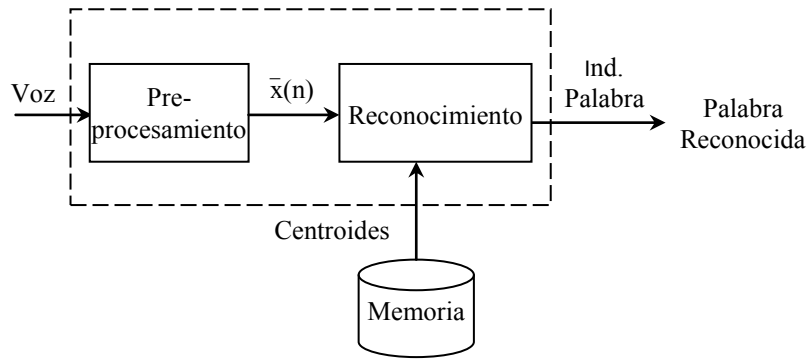
Figura 4.1 b), Etapa de reconocimiento.
