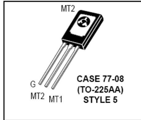
Figura 4.17, Terminales del triac.
