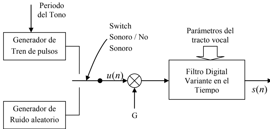
Figura 2.6 , Modelo sintetizador de voz basado en el modelo de LPC
