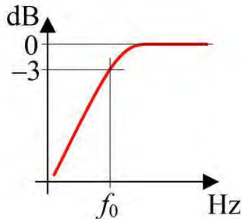
Figura 4.10, Respuesta en frecuencia del filtro para eliminar el offset.
