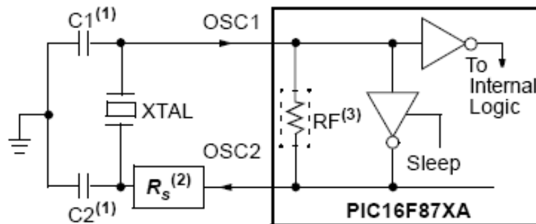
Figura 3.13 , El PIC operado en el modo XT, utilizando un cristal de Cuarzo.
