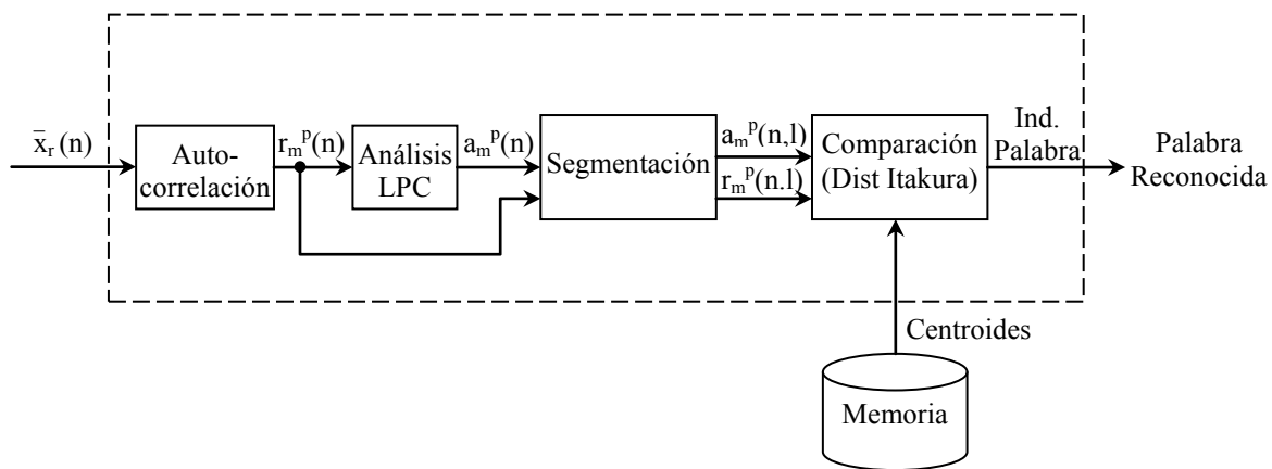
Figura 4.5 , procesos requeridos para reconocer los comandos.
