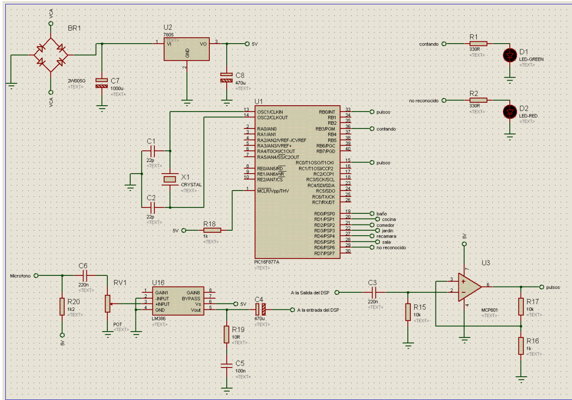
Figura 4.20, Esquemático del circuito electrónico de decodificación y control.
