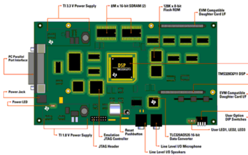
Figura 3.1, Tarjeta de desarrollo DSK.
