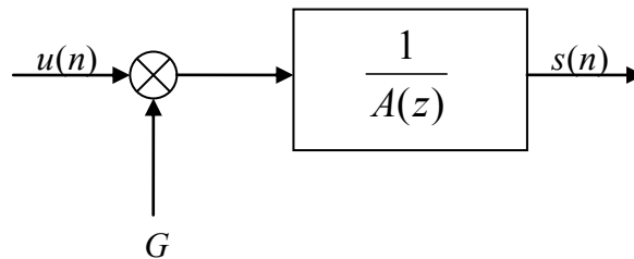
Figura 2.5 , Modelo de predicción lineal
