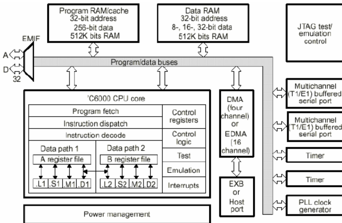
Figura 3.2, Diagrama de bloques del TMS320C62x/C67x
