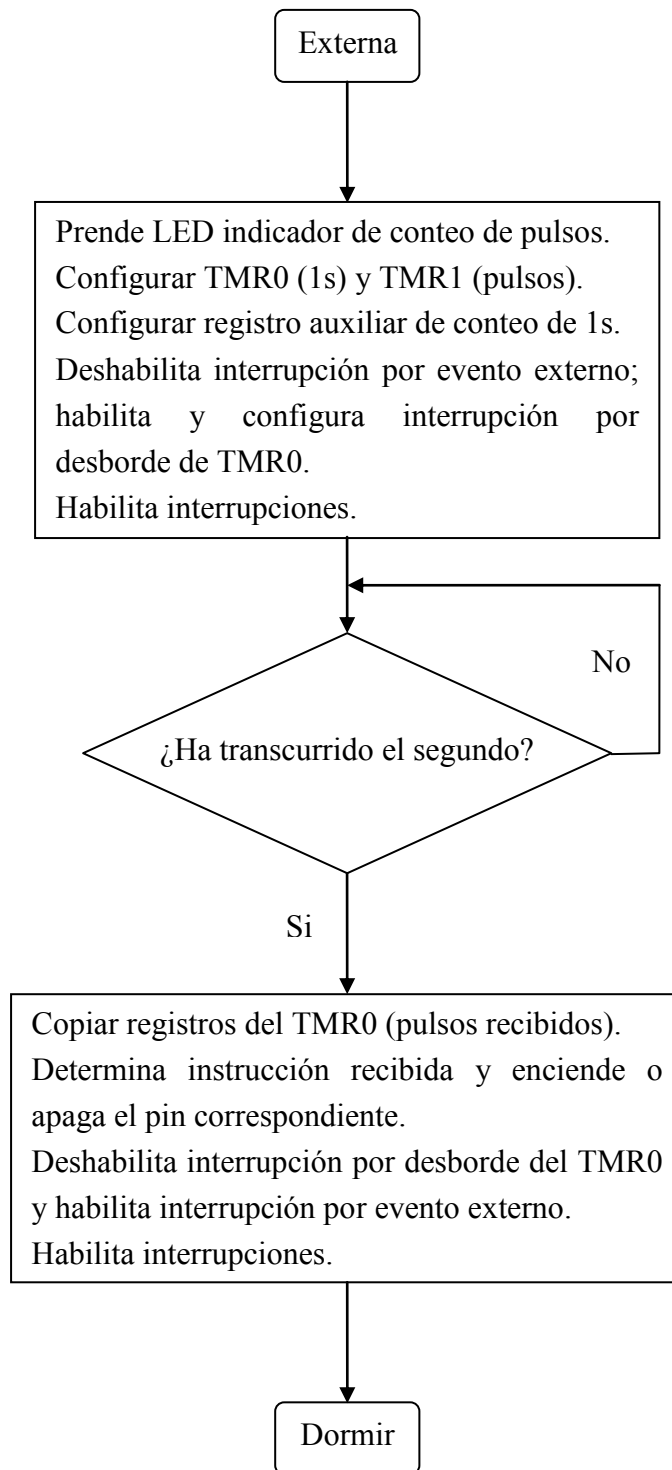
Figura 4.14 b), Continuación del diagrama de flujo del programa del PIC.
