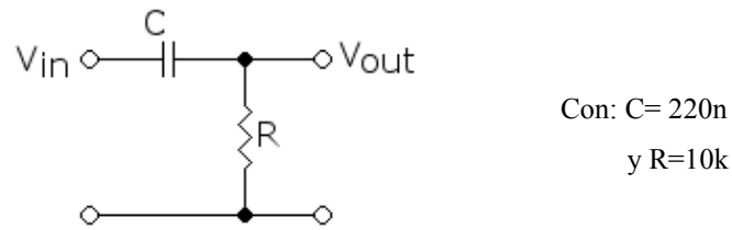
Figura 4.9, Filtro implementado para eliminar el offset de la señal.
