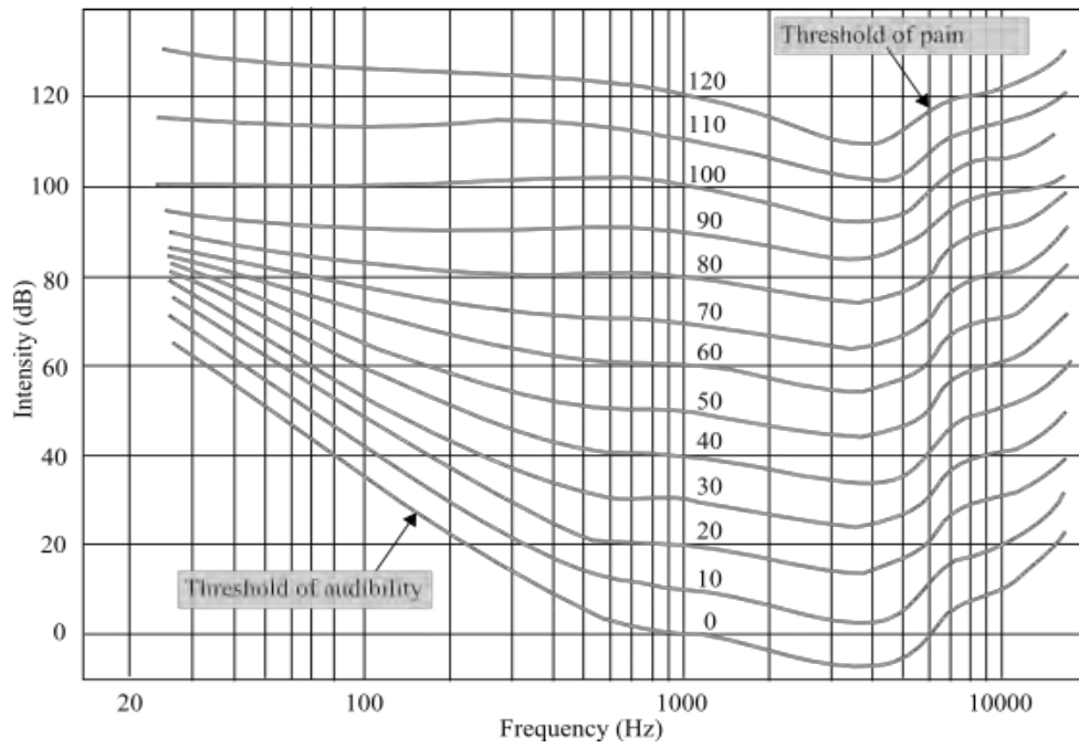
Figura 1.1, sonoridad.
