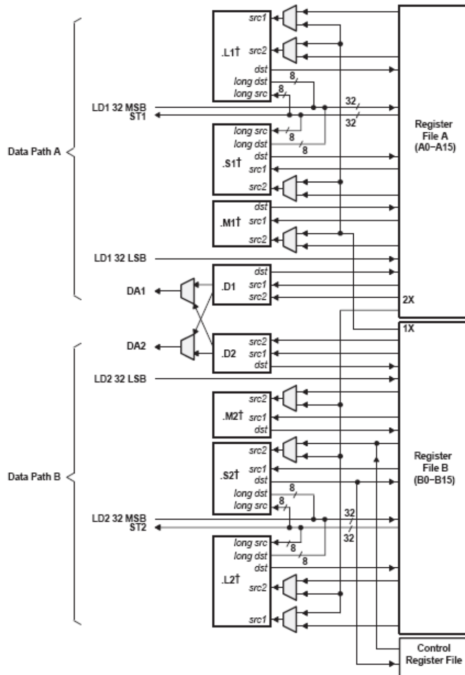
Figura 3.3, Trayectorias de los datos en el CPU TMS320C67x (núcleo del DSP)
