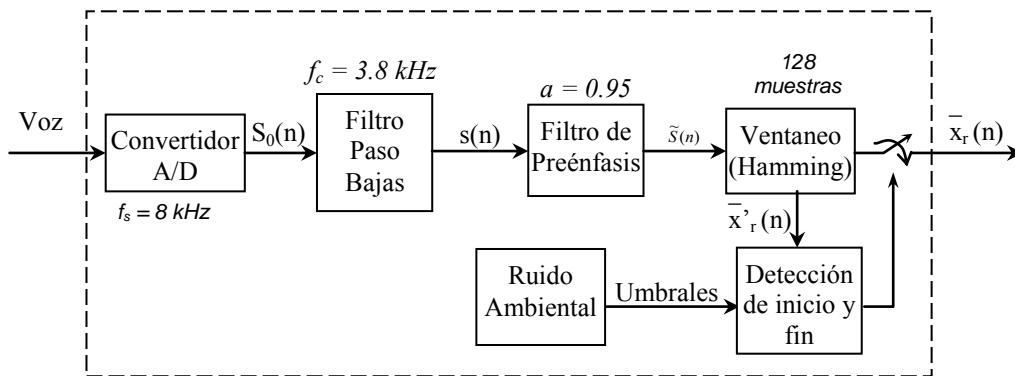
Figura 4.2, Diagrama de bloques para el módulo de preprocesamiento.
