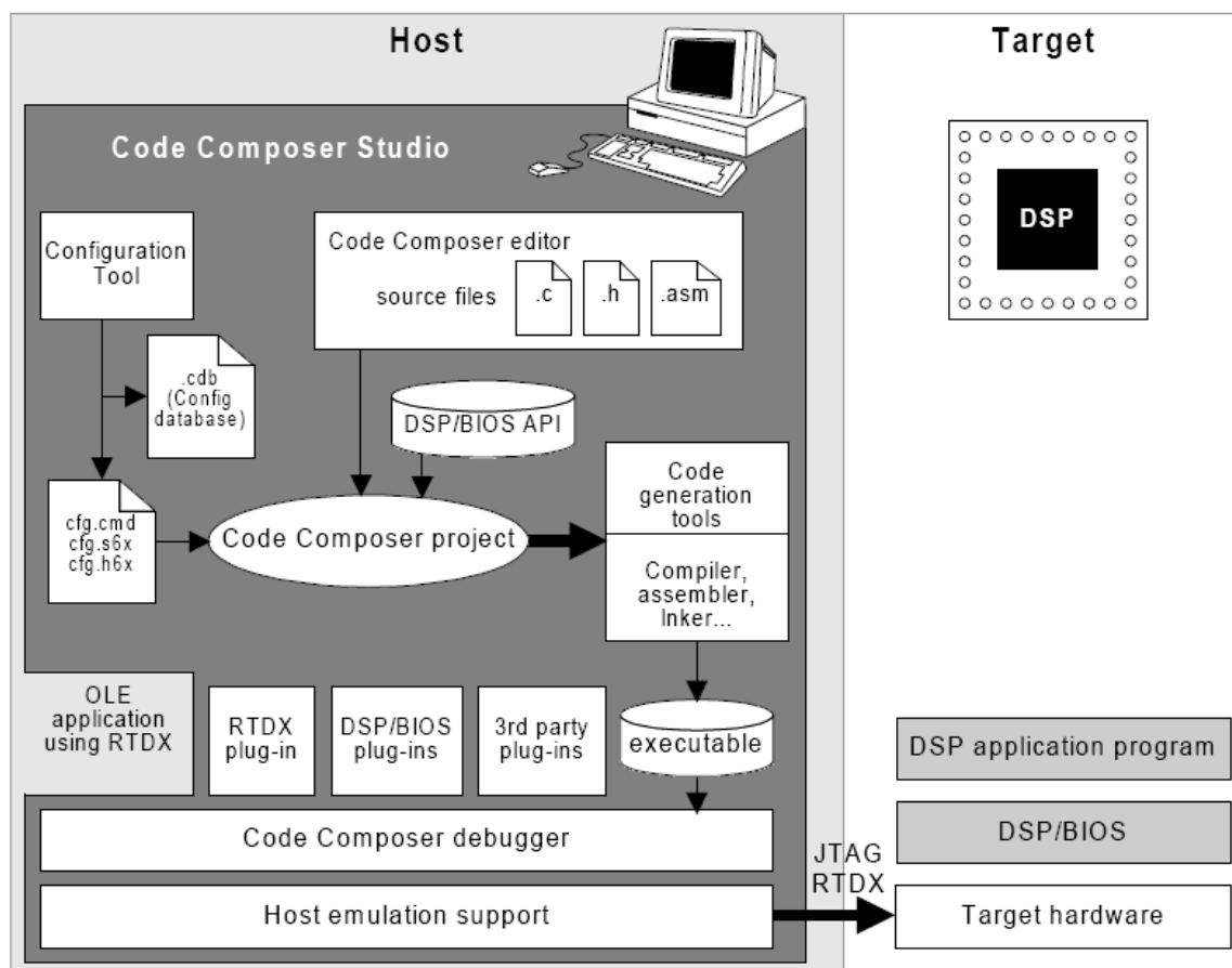
Figura 3.5, Componentes de trabajo del CCS
