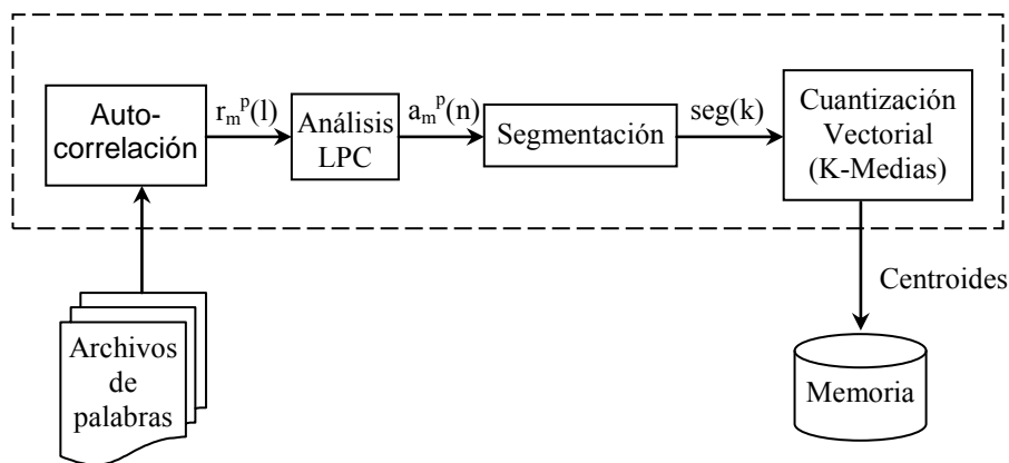
Figura 4.4 , procesos requeridos para entrenar el sistema.
