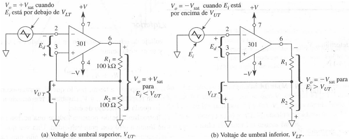
Figura 4.11, Configuraciones para la realimentación positiva.
