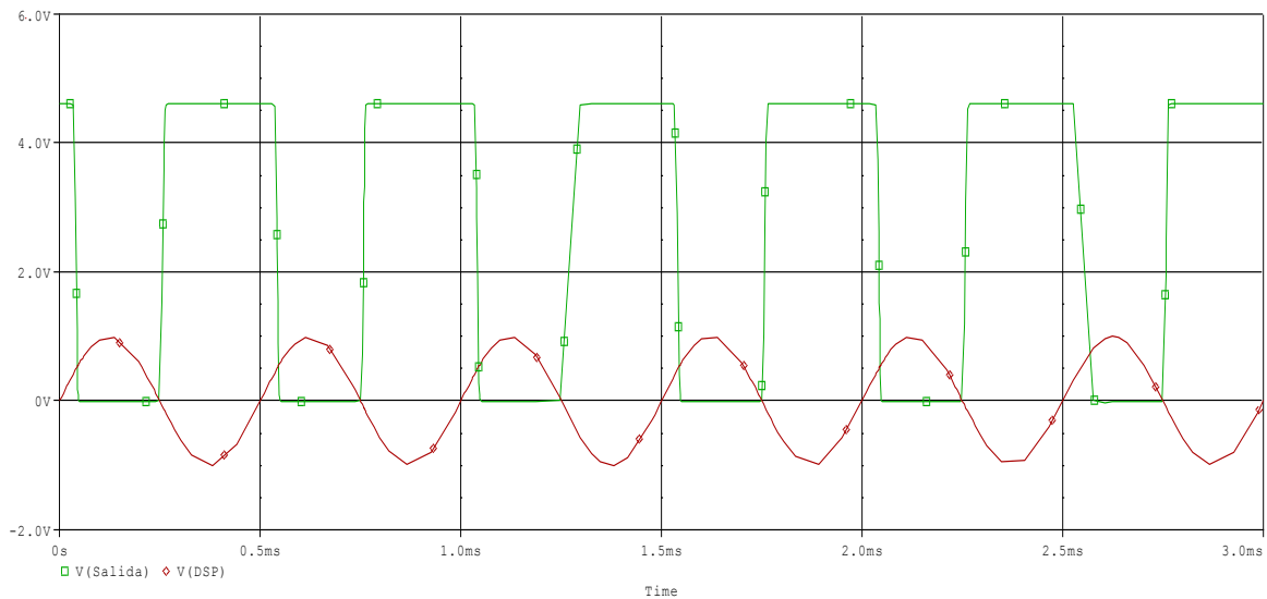
Figura 4.13, Modificación de la forma de onda de la señal.
