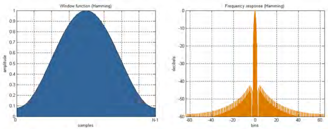
Figura 4.3 , Forma de la ventana de Hamming y Respuesta en Frecuencia.
