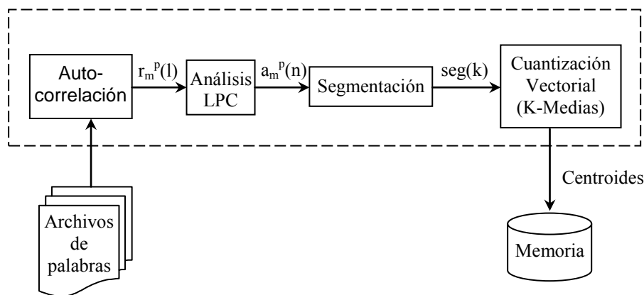
Figura 2.4, Módulo de Entrenamiento
