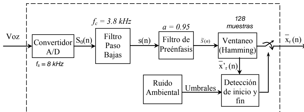
Figura 2.3, Diagrama de bloques para el módulo de preprocesamiento
