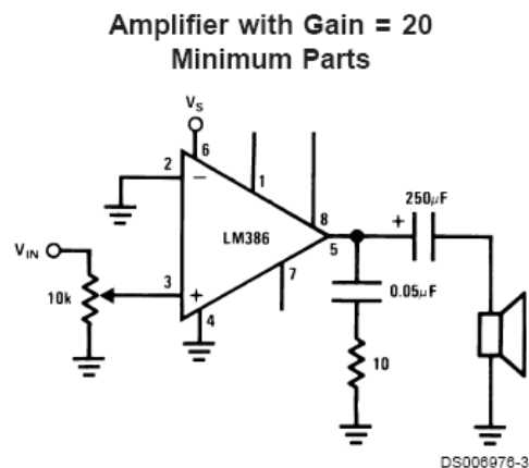
Figura 4.19 , Diseño de un preamplificador para audio.
