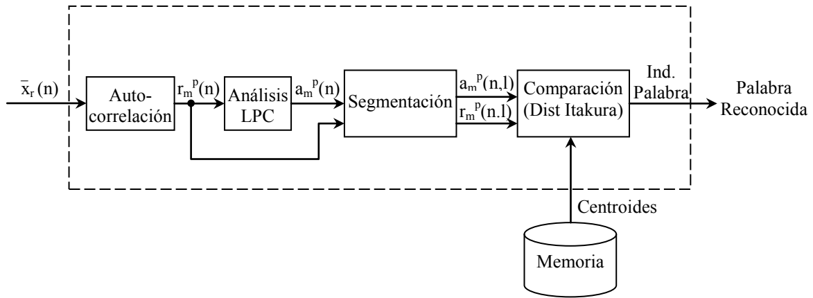
Figura 2.9 Módulo de Reconocimiento
