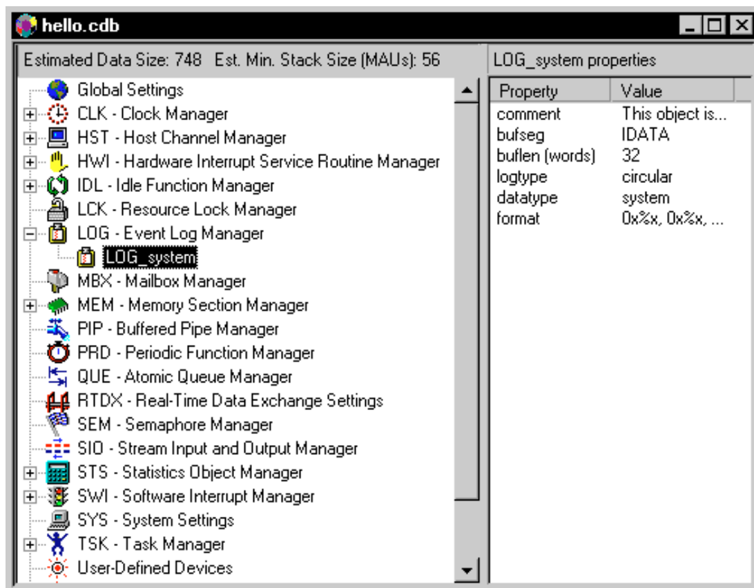
Figura 3.9, Ventana de configuración de los objetos del DSP/BIOS.
