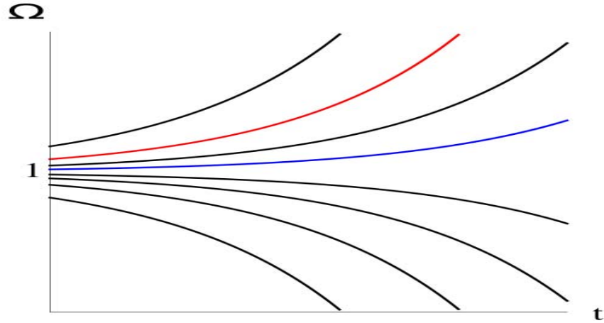
Figura 1.5: El problema de la planitud mostrado en una gráfica de densidad relativa \Omega contra el tiempo cosmológico t (ningún eje está a escala). En esta imagen se muestra como la solución \Omega = 1 es repulsiva. Cada línea muestra un posible universo. Un universo similar al nuestro es la línea azul con |\Omega - 1| \sim 0 . El universo representado por la línea roja es uno que difirió muy de las condiciones iniciales del universo representado por la línea azul. Figura tomada del Wikicommons http://en.wikipedia.org/wiki/File:Flatness_problem_density_graph.svg
