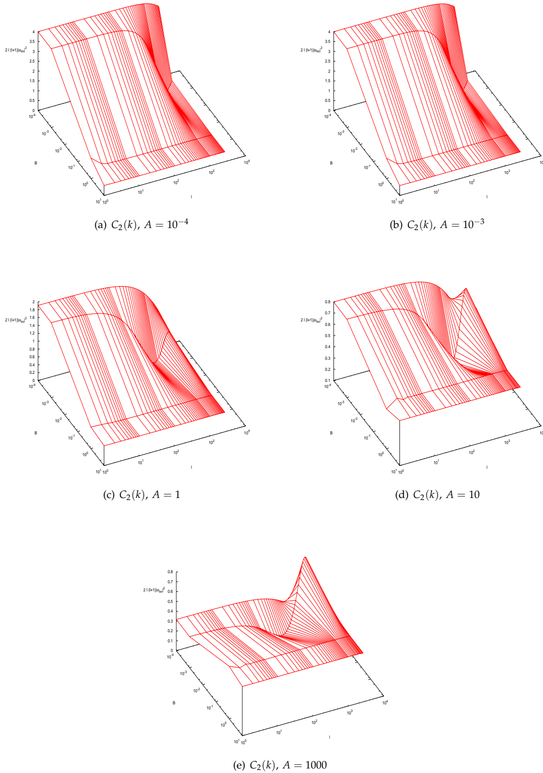
Figura 3.8: Gráfica mostrando como la integral de |\alpha_{1m}|^2(C_2) varía con respecto a cambios en B ( 10^{-4} - 10 ), manteniendo A fija. Ambos ejes B y l están en escala logarítmica. Ver el texto para una explicación más extensa.
