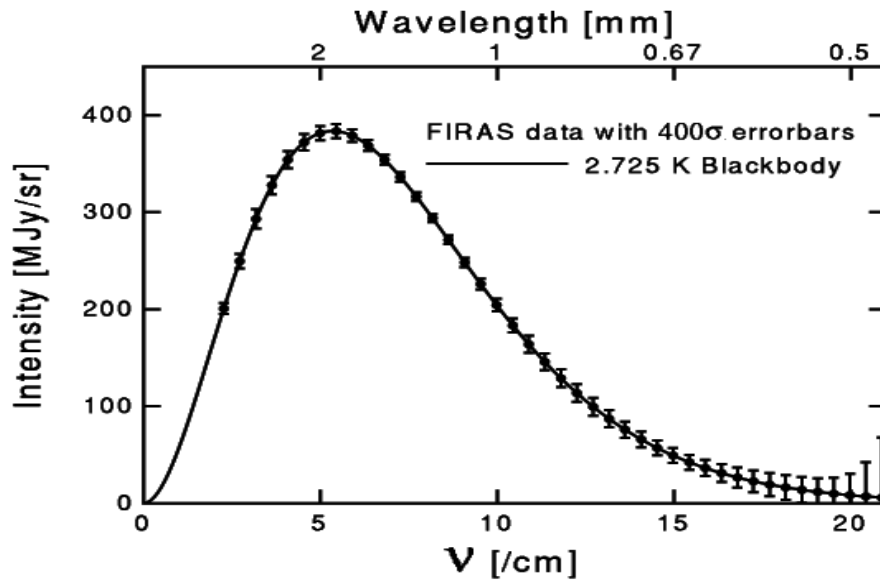
Figura 1.2: Espectro del fondo de radiación cósmica (CBR) correspondiente a la temperatura T_0 = 2.725 \text{ K} obtenido por el instrumento FIRAS del COBE Garcia-Bellido, 2005 [76].
