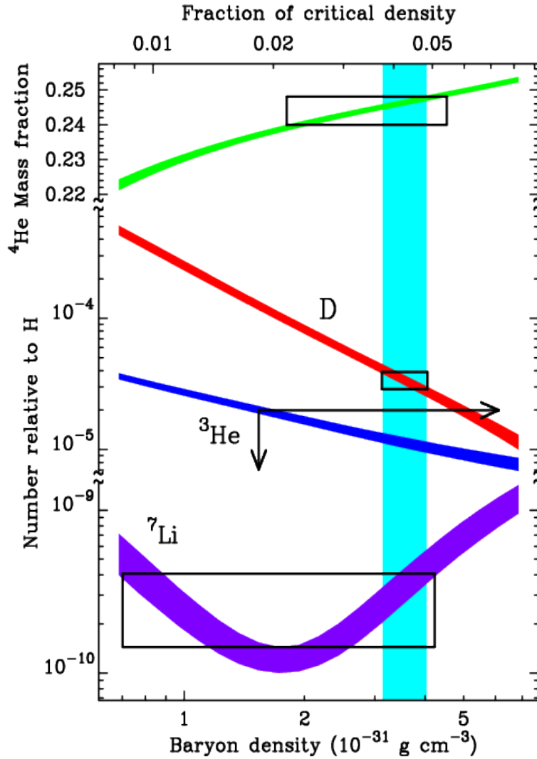
Figura 1.1: Constricciones sobre la densidad bariónica de la Nucleosíntesis. Son mostradas las predicciones de cuatro elementos (de arriba a abajo): ^4\text{He} (verde), D (roja), ^3\text{He} (azul) y ^7\text{Li} (morada). Estas predicciones abarcan 10 ordenes de magnitud (ver texto). La banda sólida son las mediciones de D primordial. Las cajas muestran observaciones sobre las abundancias de elementos, nótese que para el ^3\text{He} sólo se conoce el límite superior. Figura tomada de Burles y otros, 1999 [35].
