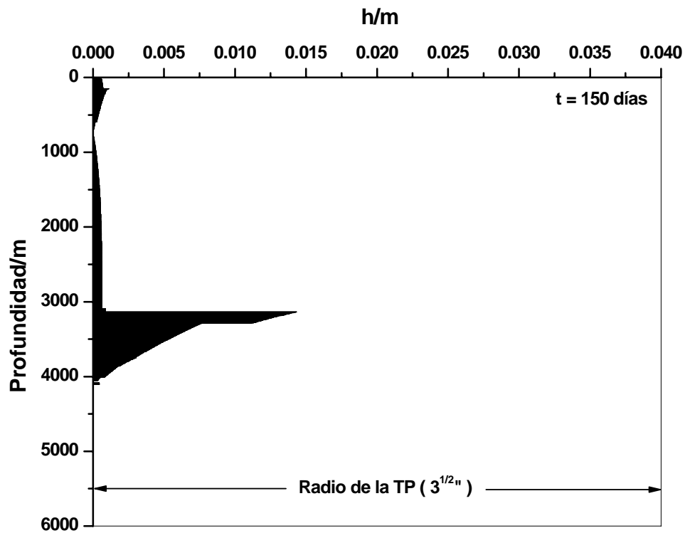
Figura V.7 Profundidad contra radio de la TP.
