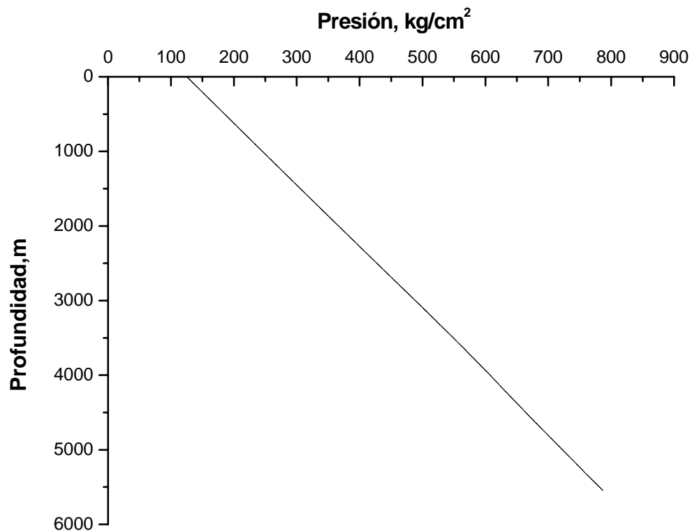
Figura V.2 Gráfica de la presión contra la profundidad.
