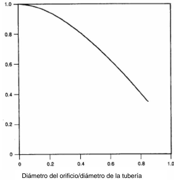
Figura III.1 Perfil de presiones en el estrangulador, Perkins (1993).
