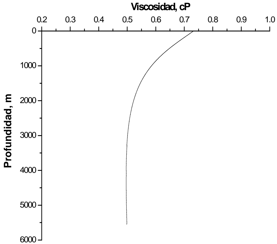
Figura V.6 Gráfica de la Viscosidad contra profundidad.
