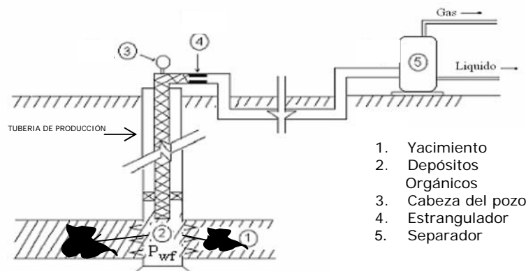
Figura I.3 Pozo productor de petróleo.
