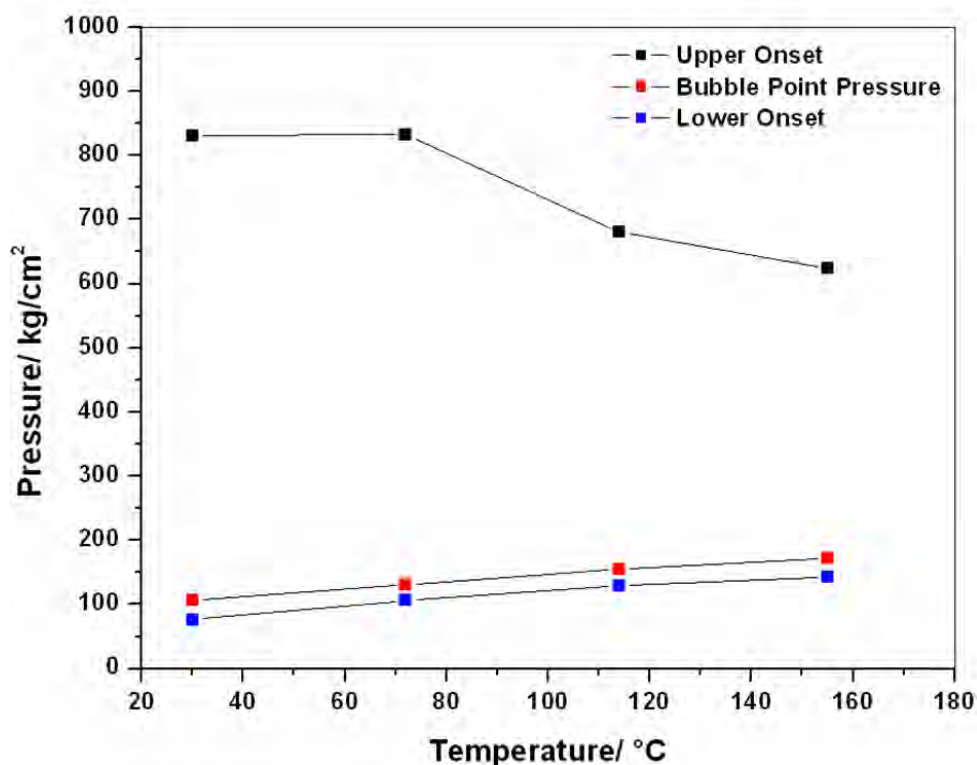
Figura V.1 Predicción de la envolvente de fases.
