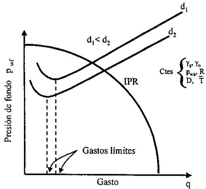
Figura II.3 Curvas típicas de Gasto vs p_{wf} para diferentes diámetros de T.P (Martínez 1999).
