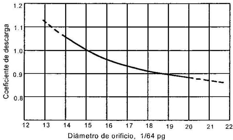
Figura A.8 Coeficiente de descarga para flujo no crítico.
