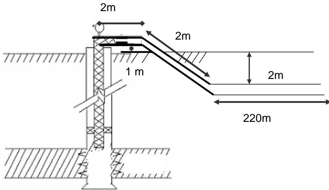
Figura IV.10 Diagrama del pozo A.
