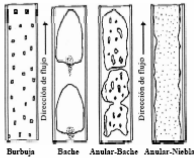
Figura II.1 Patrones de Flujo Típicos en Flujo Vertical.
