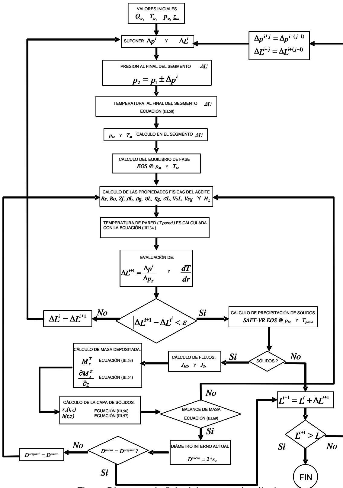
Figura Diagrama de flujo del proceso de cálculo.
