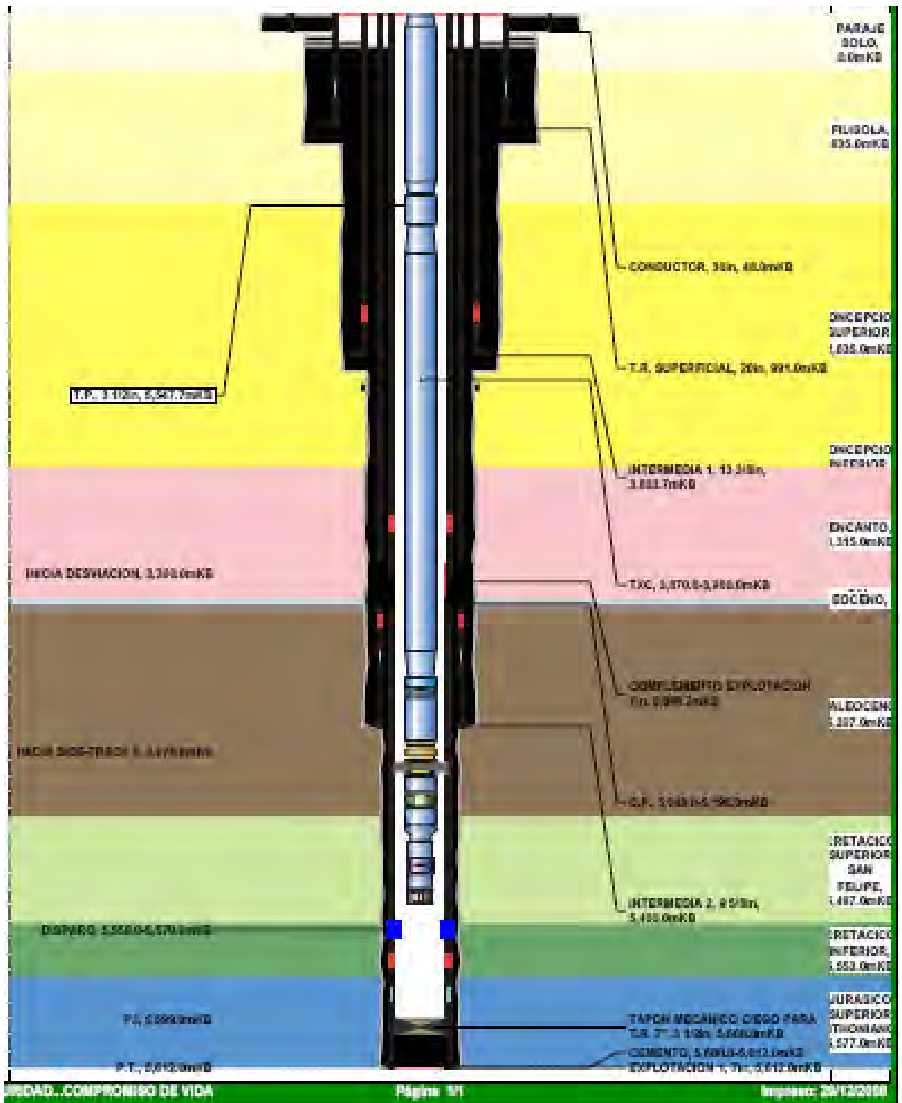
Figura IV.7 Estado Mecánico del Pozo A.
