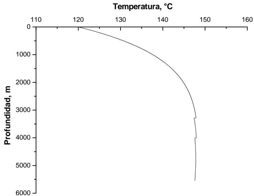
Figura V.3 Gráfica de la temperatura contra la profundidad.
