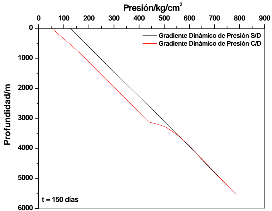
Figura V.8 Profundidad contra presión.
