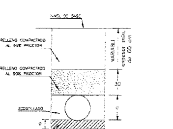
ZANJA TIPO FUENTE: PLANO TIPO SA-OP V.C. 1979
