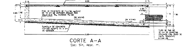
CORTE A-A Esc. Sín. Acot. m.
