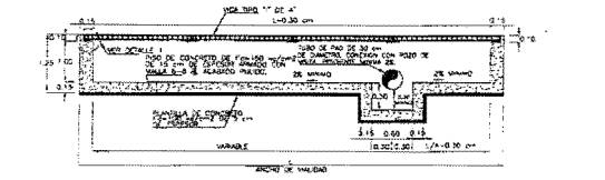
CORTE C-C Esc. Sín. Acot. m.
