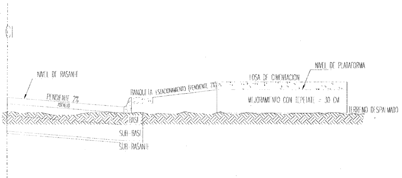
Figura 12. Modelo Conceptual de Rasantes y Plataformas
