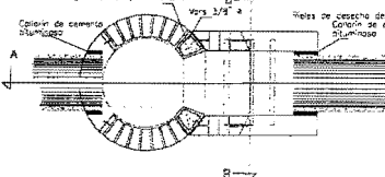
CORTE A-A
