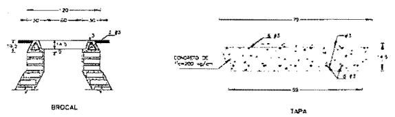
BROCAL Y TAPA DE CONCRETO PARA POZO DE VISITA FUENTE: PLANO TIPO SA-OP V.C. 1983 Esc. Sín. Acot. m.
