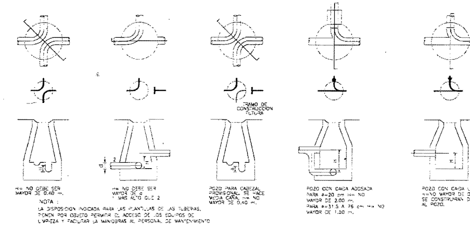
DISPOSICION DE PLANTILLAS EN POZOS DE VISITA FUENTE: PLANO TIPO SA-OP V.C. 1984
