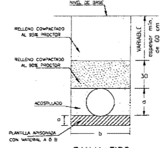
ZANJA TIPO FUENTE: PLANO TIPO SAHOP N.- VC-1979
