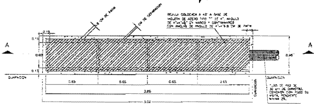
PLANTA Esc. Sín. Acot. m.
