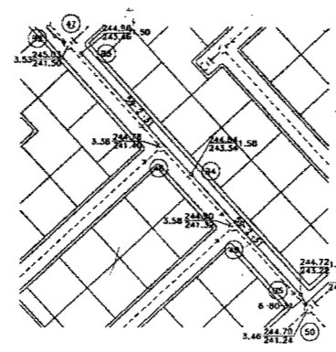
DETALLE 3 Esc. Sin. Acot. cm.
