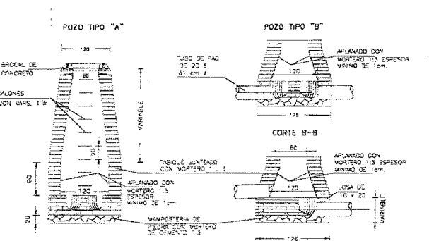
POZO TIPO A and POZO TIPO B
