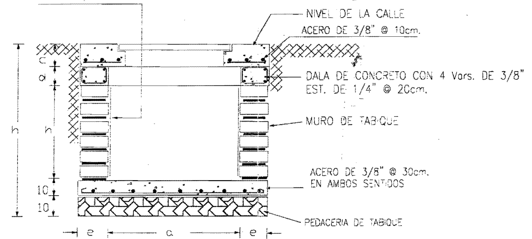
ELEVACION
