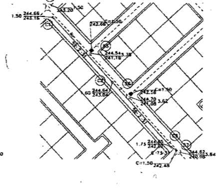
DETALLE 4 Esc. Sin. Acot. cm.
