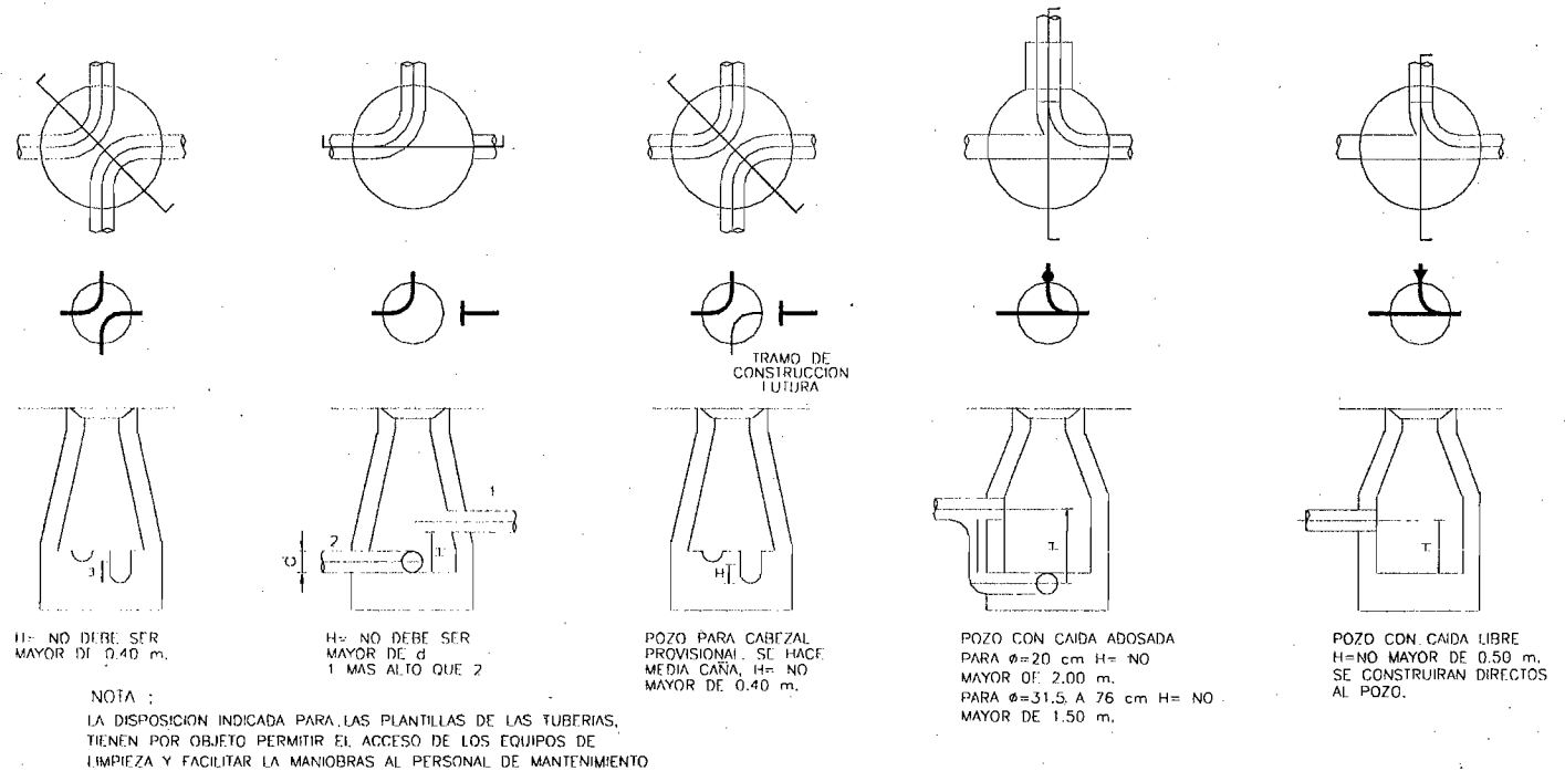
DISPOSICION DE PLANTILLAS EN POZOS DE VISITA
