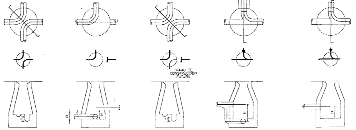
DETALLE DE UNIONES DE TUBERIA CON POZO DE VISITA Y REGISTRO
