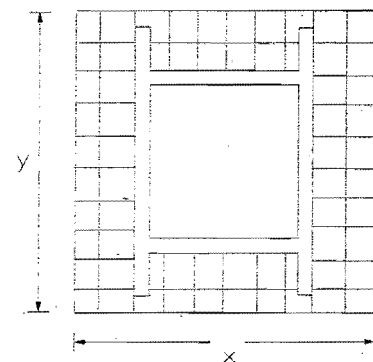
LOSA Y CONTRAMARCO
