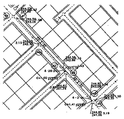
DETALLE 7 Esc. Sin. Acot. cm.
