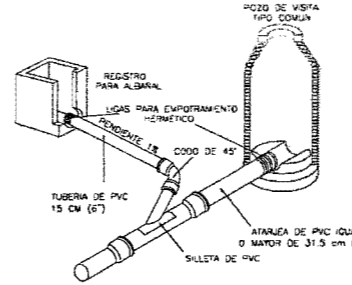
DETALLE DE UNIONES DE TUBERIA CON POZO DE VISITA Y REGISTRO
