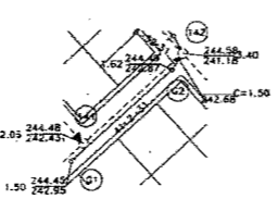
DETALLE 9 Esc. Sin. Acot. cm.
