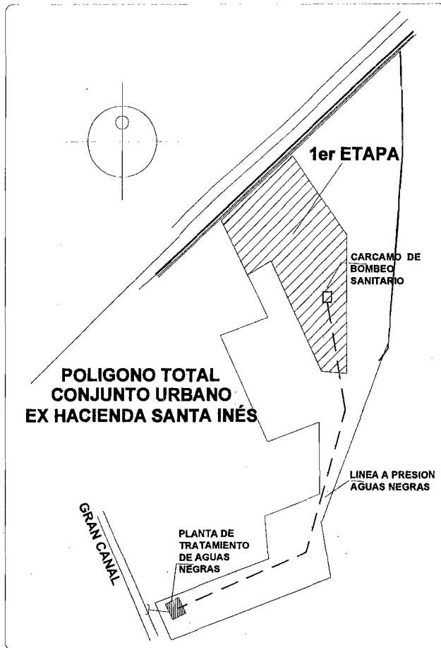
Figura 18. Esquema a plan maestro del drenaje sanitario.
