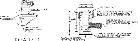
CORTE D-D Esc. Sín. Acot. m.
