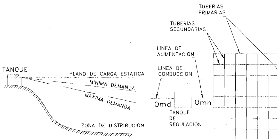
Figura 2. Distribución por gravedad (recomendable).
