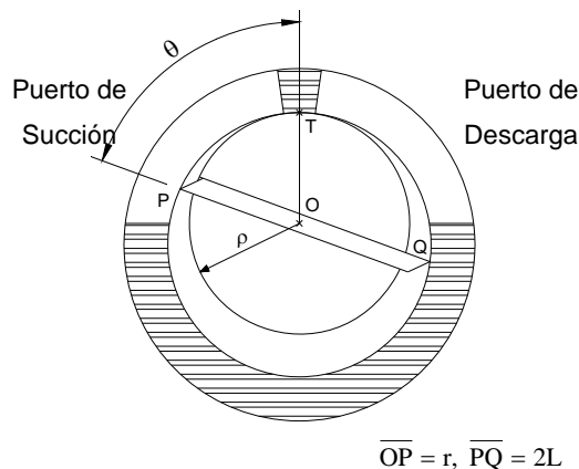
Figura I.4 Bomba Monopaleta
