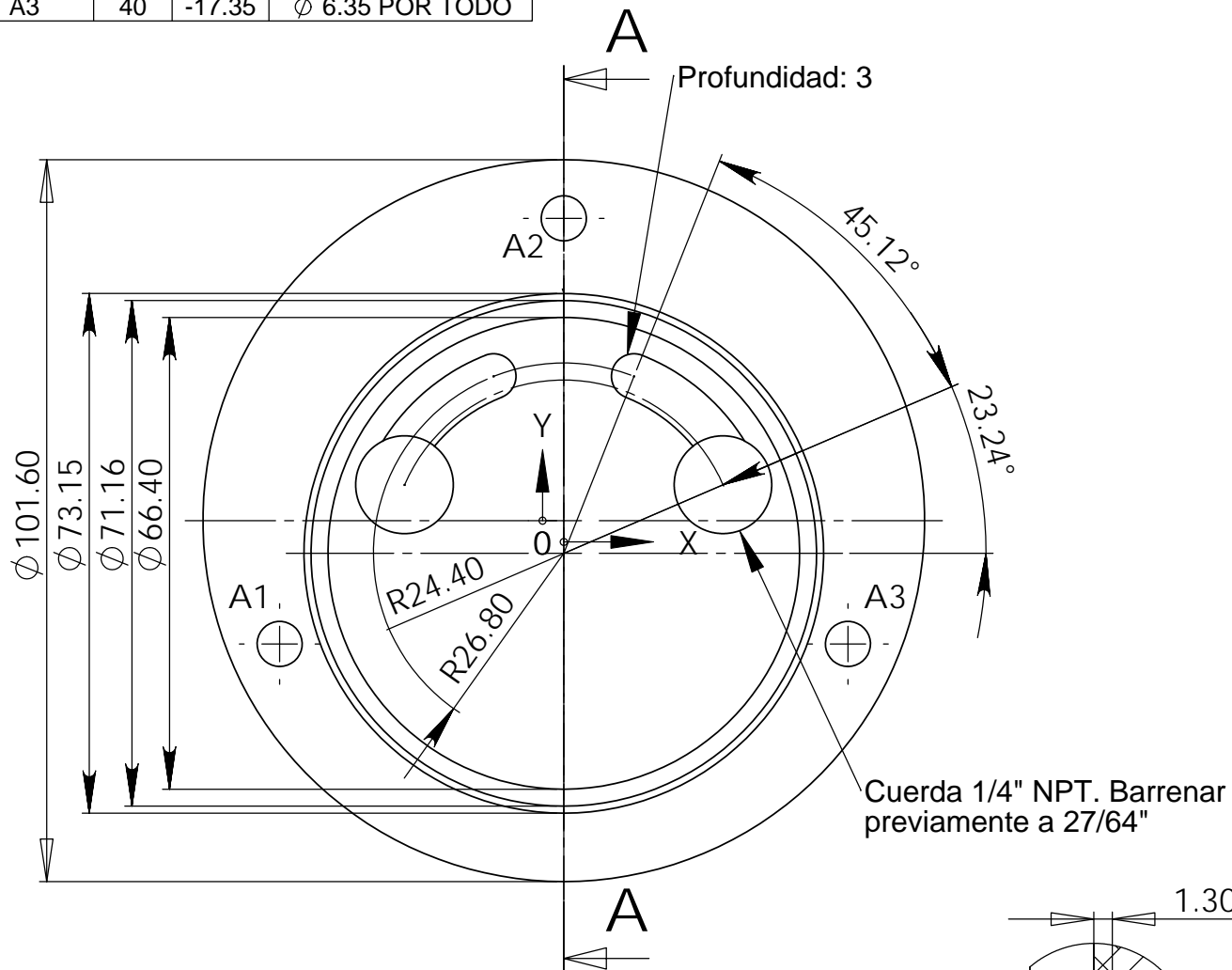
DETALLE a ESCALA 2 : 1
