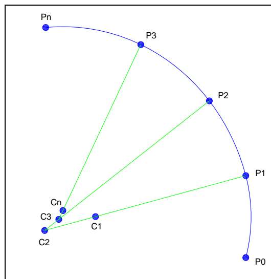
Figura II.14 Proceso secuencial para la obtención del perfil del anillo.
