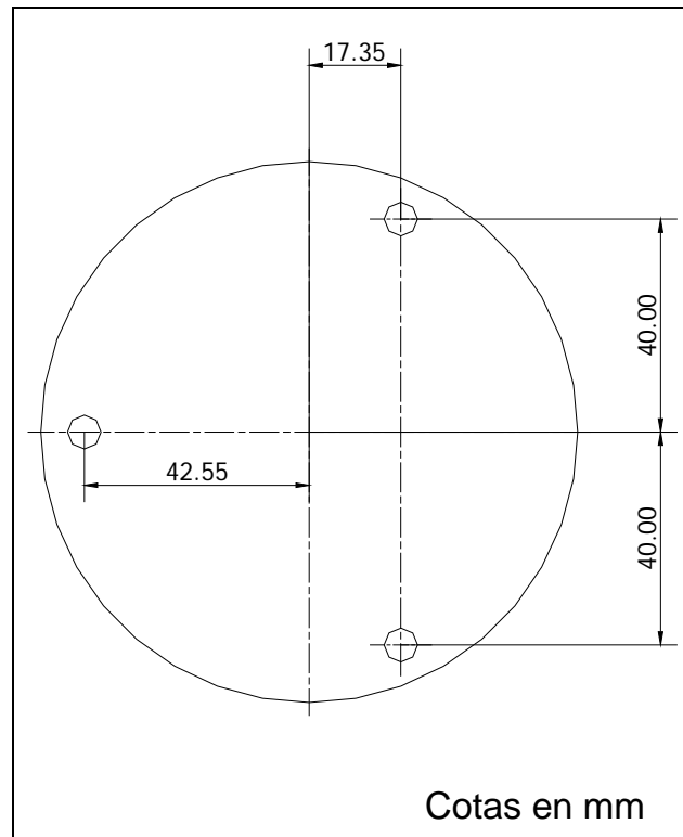
Figura II.20 Ubicación de los barrenos en la tapa y carcasa.
