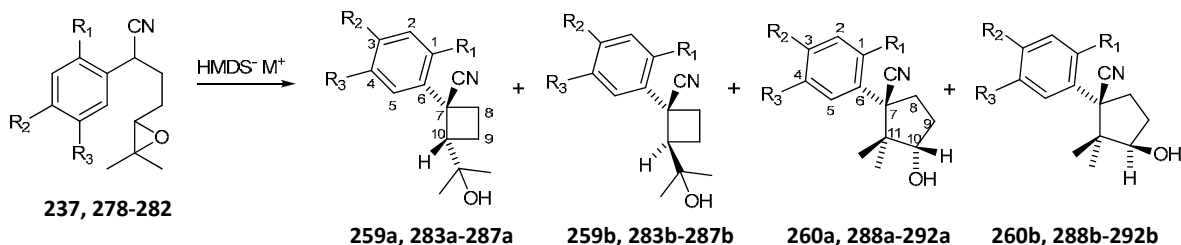
Esquema 46. Posibles productos de ciclaciones aniónicas de \alpha -aril- \delta -epoxinitrilos.
