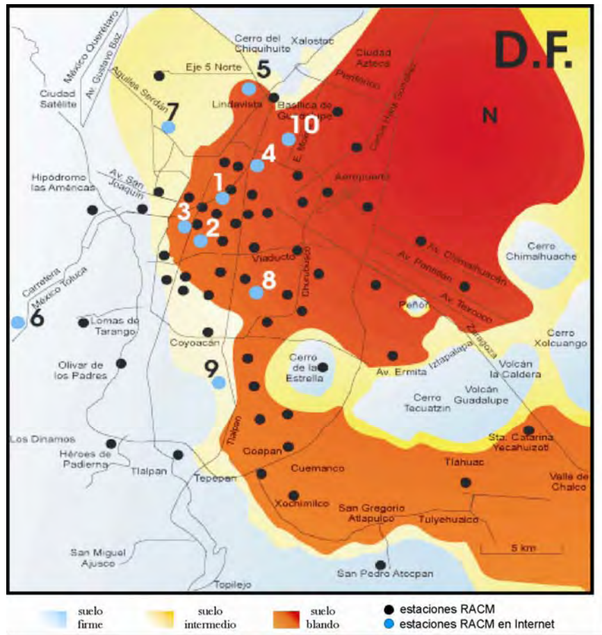
Figura 3.2.- Ubicación de las estaciones de la Red Acelerográfica de la Ciudad de México (RACM). Se observa que existen estaciones de monitoreo en zonas de suelo firme. Imagen tomada de la pág. http://www.cires.org.mx .
