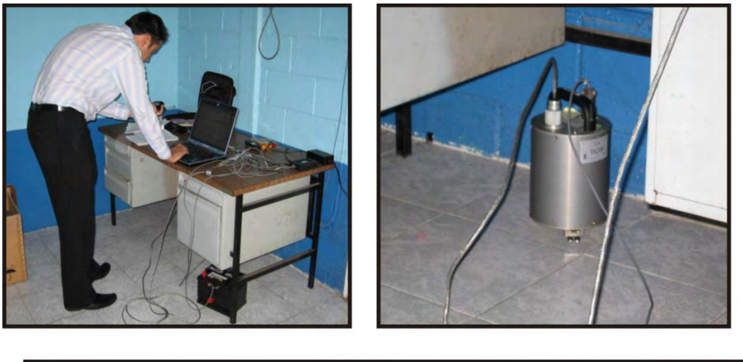
Figura 4.4: En estas fotos se muestra la instalación de la estación COCH para el arreglo 2, el equipo utilizado es un CMG-6TD, en la parte izquierda se aprecia la puesta en funcionamiento mediante una computadora portátil, también se muestra la batería de 12 V que proporciona la alimentación de corriente. En la parte derecha se muestra el sensor el cual ya está formado por un registrador y un arreglo de tres sensores que registran simultáneamente, el dispositivo GPS que proporciona el tiempo absoluto se coloca en lo alto de la construcción.
