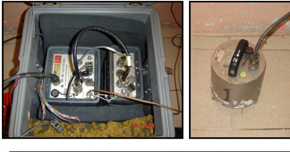
Figura 4.2: Tipo de sismógrafos instalados en las estaciones, registrador (izq.) sensor (der.)
