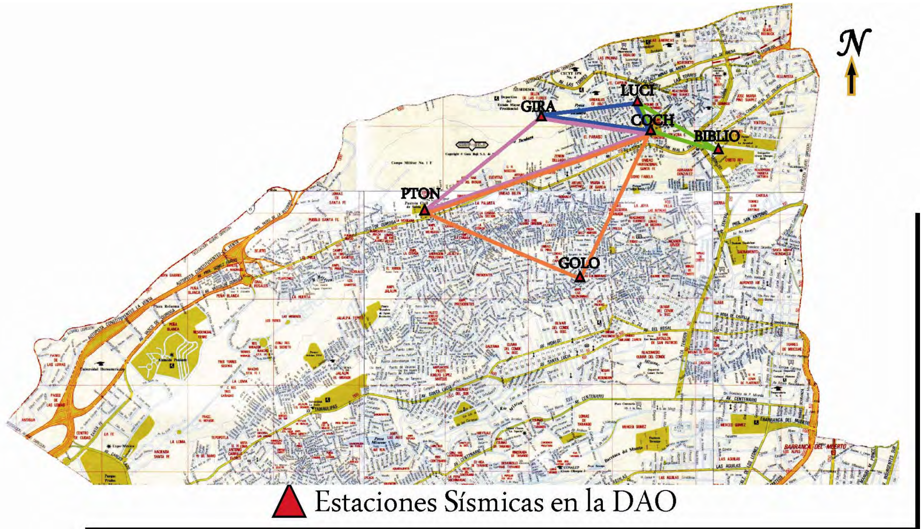
Figura 4.1: Ubicación de estaciones sísmicas, y de los arreglos que formaron en las diferentes campañas. La triangulación verde muestra a las estaciones que forman el arreglo 1; la triangulación azul muestra a las estaciones que conforman el arreglo 2; la triangulación rosa muestra a las estaciones involucradas en el arreglo 3; la triangulación naranja muestra a las estaciones que forman parte del arreglo 4. Los nombres de las estaciones están referidos a las colonias cercanas a ellas.
