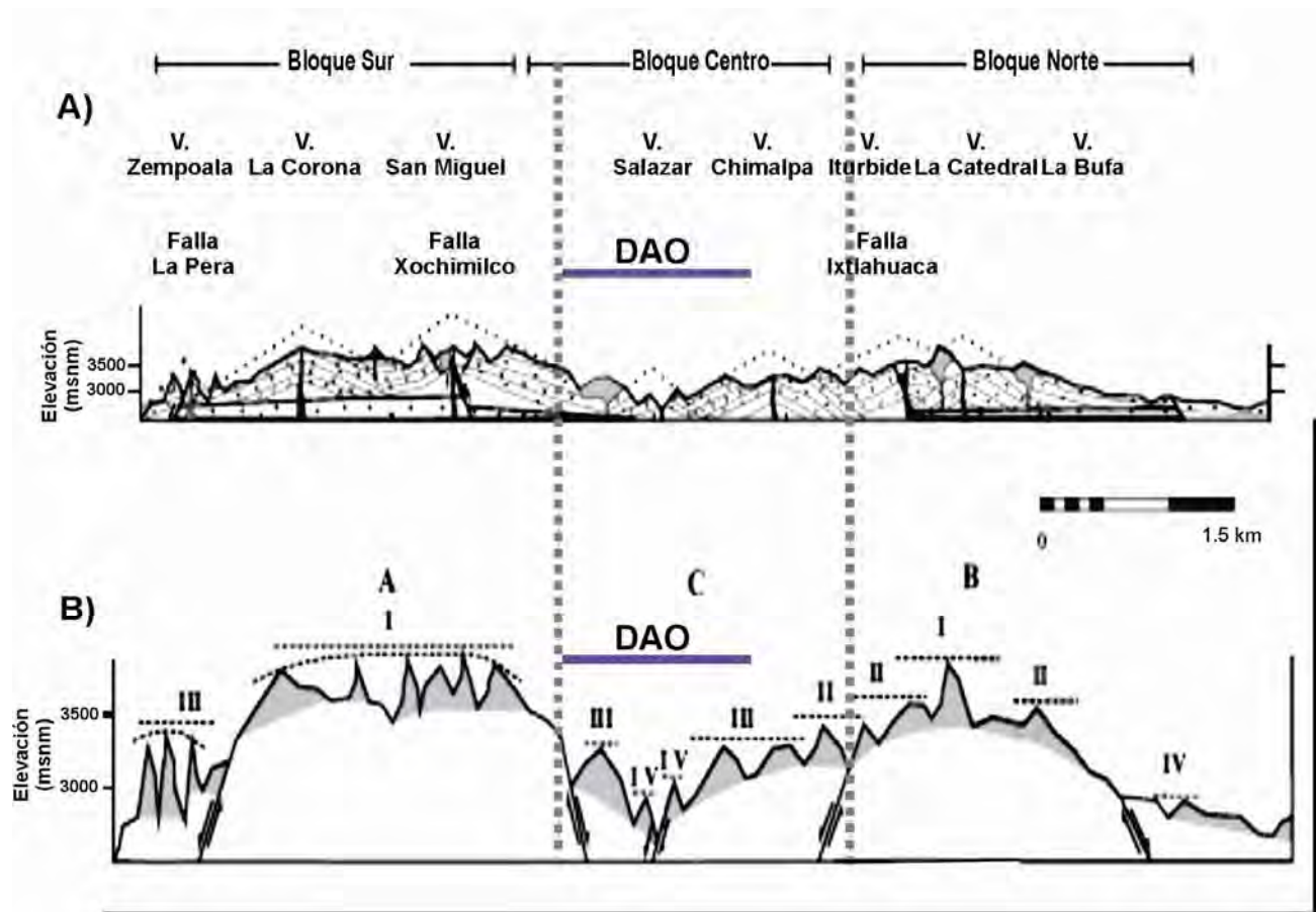
Figura 2.7.- Perfil de la SC, A) ubicación de los cuerpos volcánicos y las fallas que diferencian los tres bloques de la sierra. B) representación de las estructuras de la sierra, las letras A y B representan pilares, la letra C indica una fosa. En línea sólida se muestra la ubicación de la DAO. (García-Palomo, et al., 2008)
