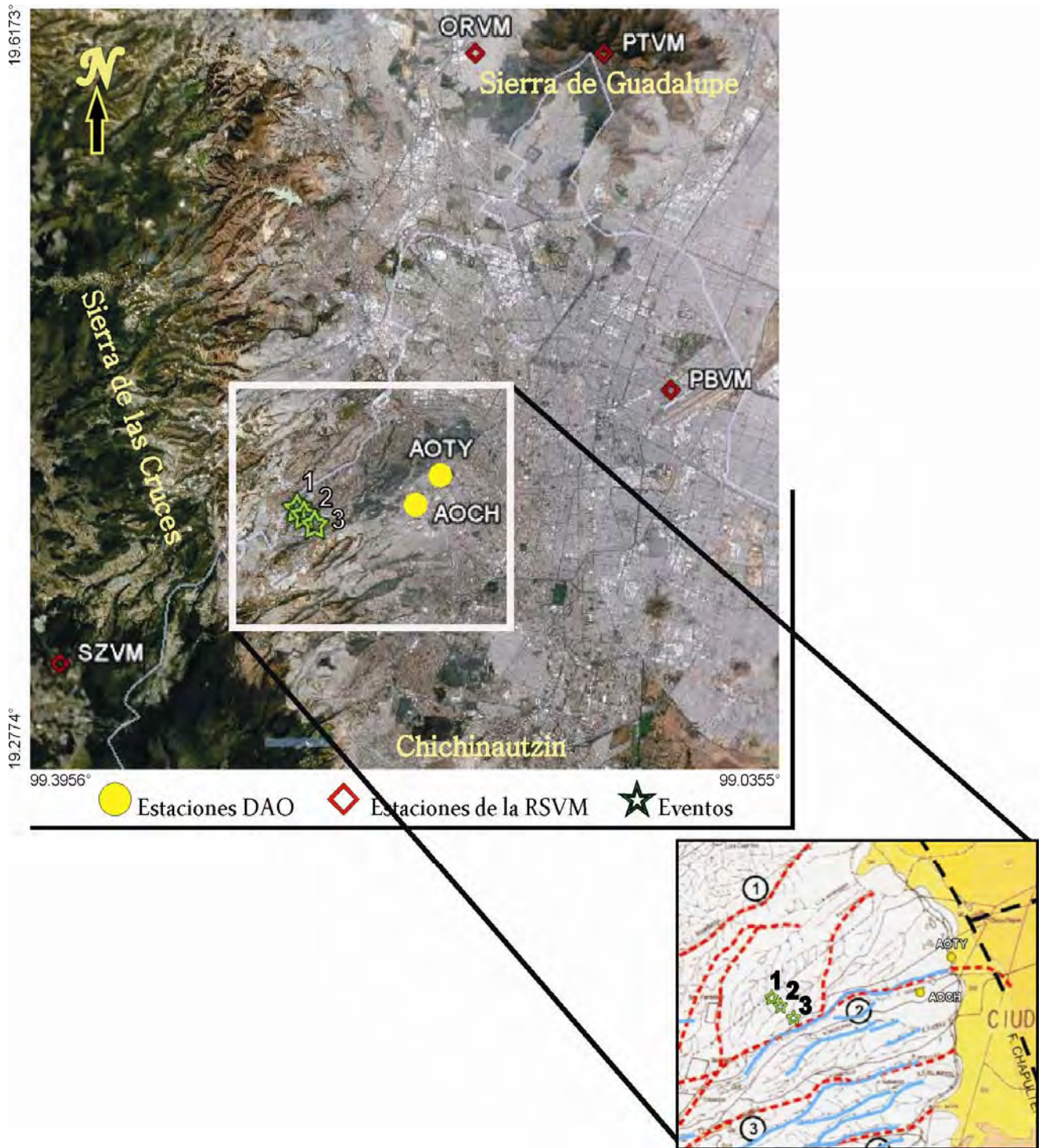
Figura 5.5: Ubicación epicentral de los tres eventos del 23 de Nov. 2008. En círculos amarillos se marcan las estaciones de la DAO, en rombos rojos las estaciones de la RSVM, en estrellas verdes los epicentros de los tres eventos. En el recuadro se muestra la ubicación de las fallas (azul) y colapsos (rojo) y su posible relación con la ubicación epicentral.
