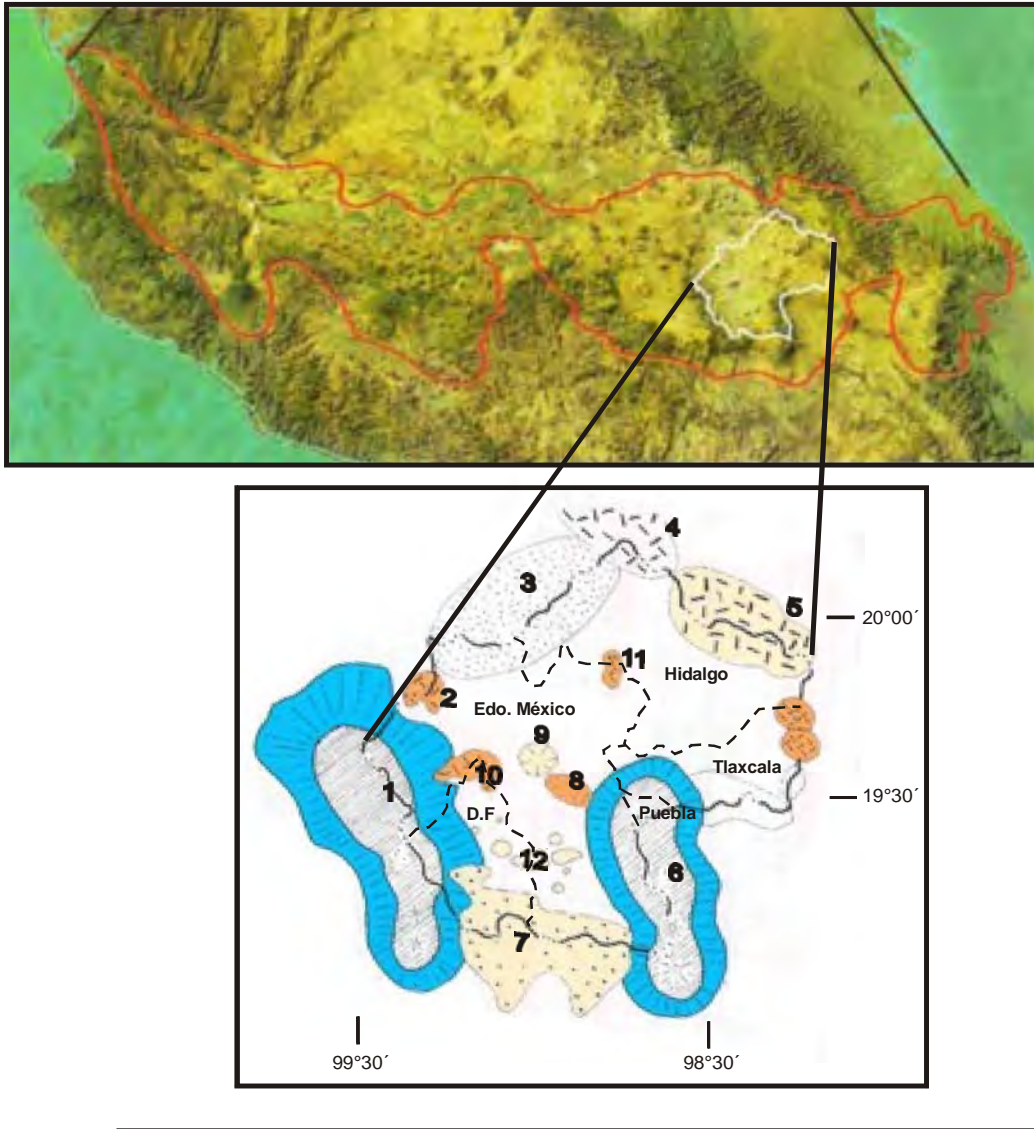
Figura 2.1.- Bosquejo de los elementos morfológicos mas importantes de la cuenca de México dentro de la FVTM (Figura superior). 1.- Sierra de las Cruces-Monte Alto. 2.- Sierra de Tepozotlan, 3.- Sierra de Tezontlapan, 4.- Sierra de Pachuca, 5.- Sierra de Singuilucan, 6.- Sierra Nevada- Rio Frio, 7.- Sierra Chichinautzin, 8.- Sierra Patlachique, 9.- Cerro Chiconautla, 10.- Sierra Guadalupe, 11.- Sierra de las Pitayas, 12.-Sierra de Santa Catarina, 13.- Sierra Calpulalpan. Modificada de (Santoyo-Villa et al. (2005) ).
