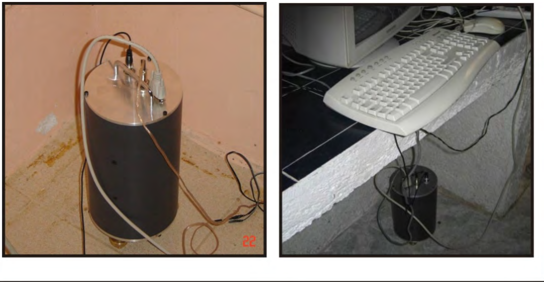
Figura 4.5: Instalación del sismómetro fabricado por el Instituto de Ingeniería de la UNAM, en la parte izquierda se muestra al sensor para su funcionamiento es necesario proporcionar alimentación eléctrica por medio de un adaptador de corriente, debe estar conectado a una computadora para el almacenamiento de los datos, cuenta con una antena GPS para el registro de tiempo absoluto. En la parte derecha se muestra al equipo instalado en la estación LUCI.
