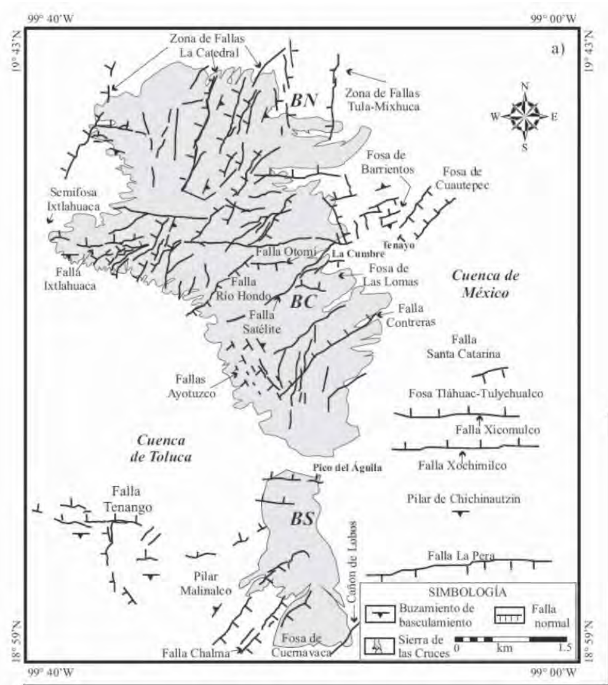
Figura 2.8.- Mapa de las principales fallas en la Sierra de las Cruces. Tomada de (García-Palomo, et al., 2008)
