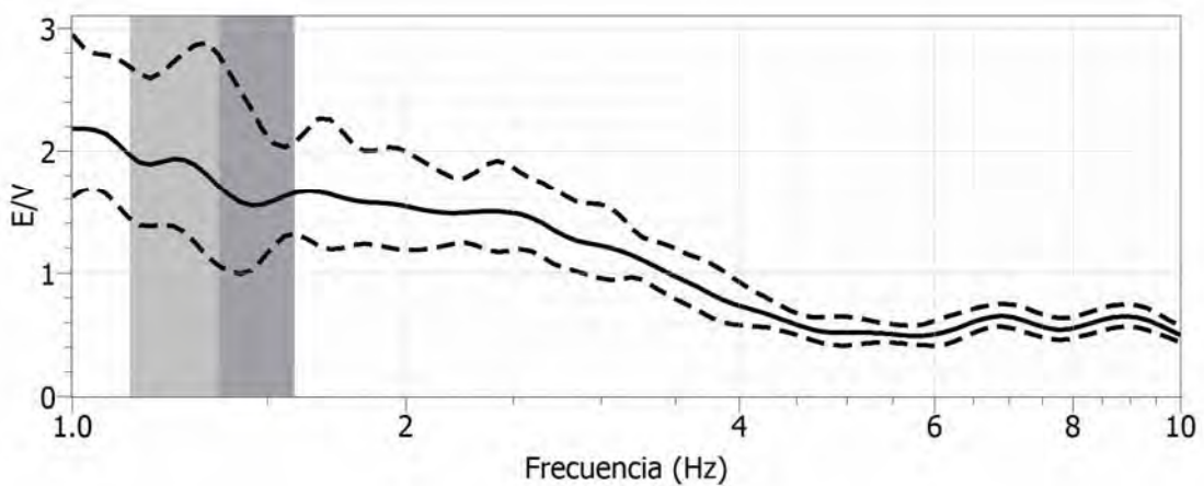
Figura A5.- Cocientes espectrales para la estación BIBLIO.
