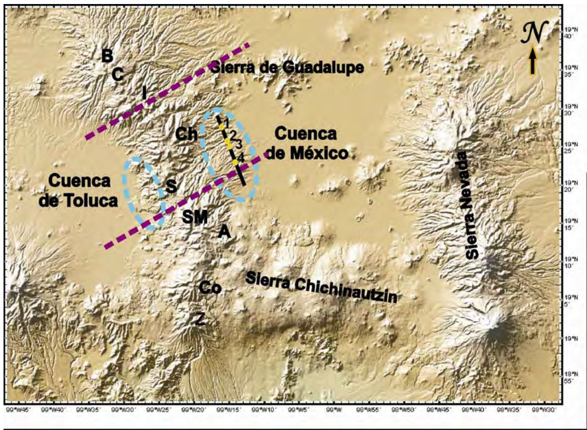
Figura 2.5.- Relieve de la Sierra de las Cruces. En los círculos de color azul se marcan las zonas de piedemonte en ambas cuencas, se puede observar que la orientación de los flujos de drenaje para la Cuenca de México están dirigidos al NE-SW. Las letras corresponden a los nombres de los estratovolcanes mencionados arriba y que le dan estructura a la SC. Las
