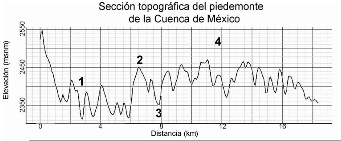
Figura 2.6.- Sección topográfica del piedemonte de la Cuenca de México, la ubicación de los altos y bajos topográficos marcados con números, están señalados en la figura 2.5 como una línea negra continua.
