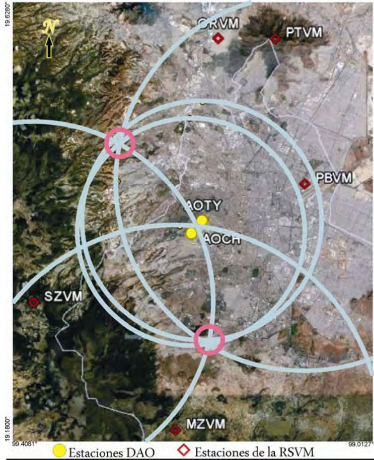
Figura 5.4: Epicentro para el evento 1 con una velocidad obtenida del modelo para la CVM (Huesca-Perez, 2008), valor de V_{p4} en la tabla 5.4.
