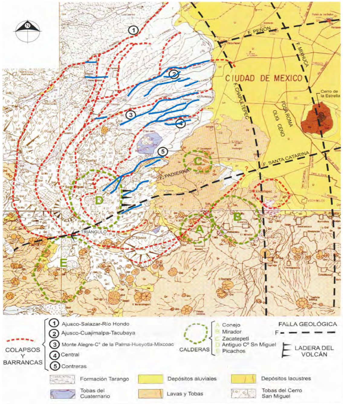
Figura 2.9.- Mapa de los colapsos del cerro de San Miguel, las líneas en azul son algunas de las fallas de la zona de piedemonte, imagen modificada de (Santoyo-Villa E., et al. 2005).
