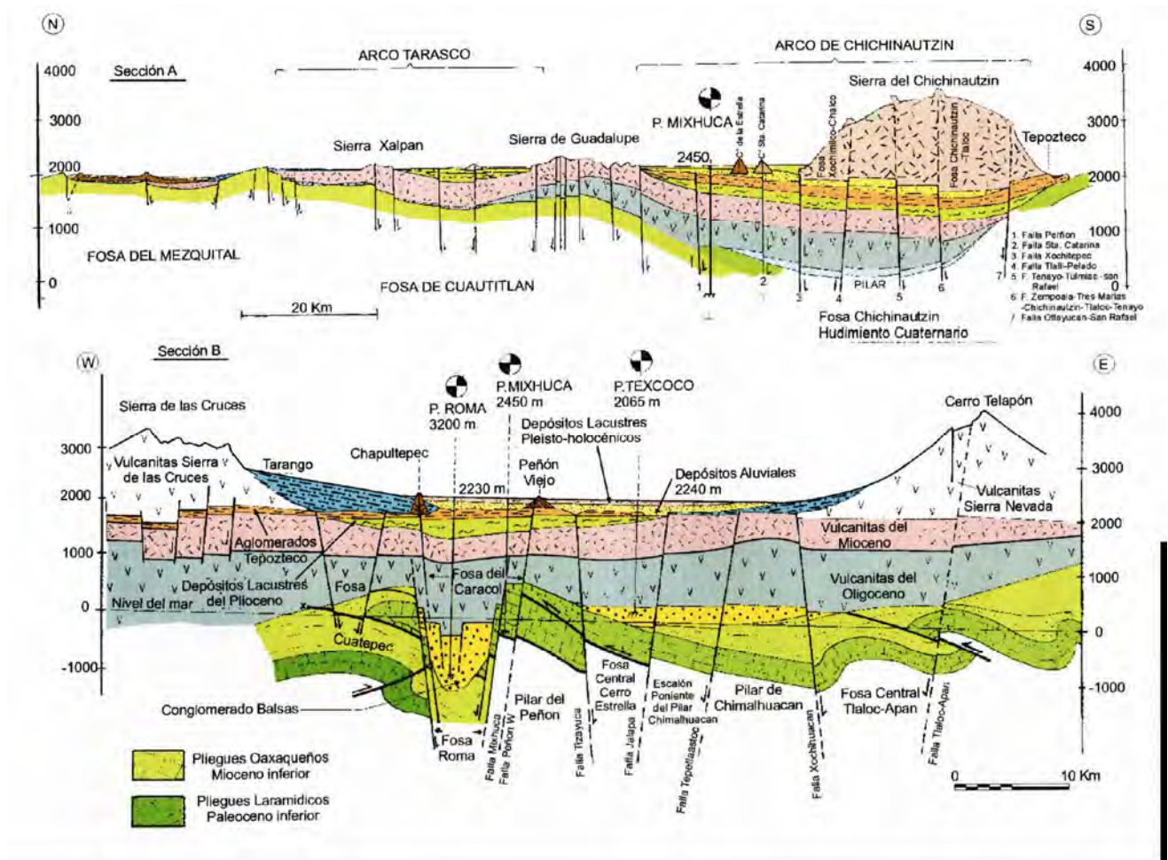
Figura 2.2.- Secciones de la Cuenca de México, la sección superior esta en dirección N-S, la inferior en dirección E-W. Imagen tomada de (Santoyo-Villa, E., et al., 2005). La información detallada de cada una de las formaciones mostradas, se encuentran en el texto.
