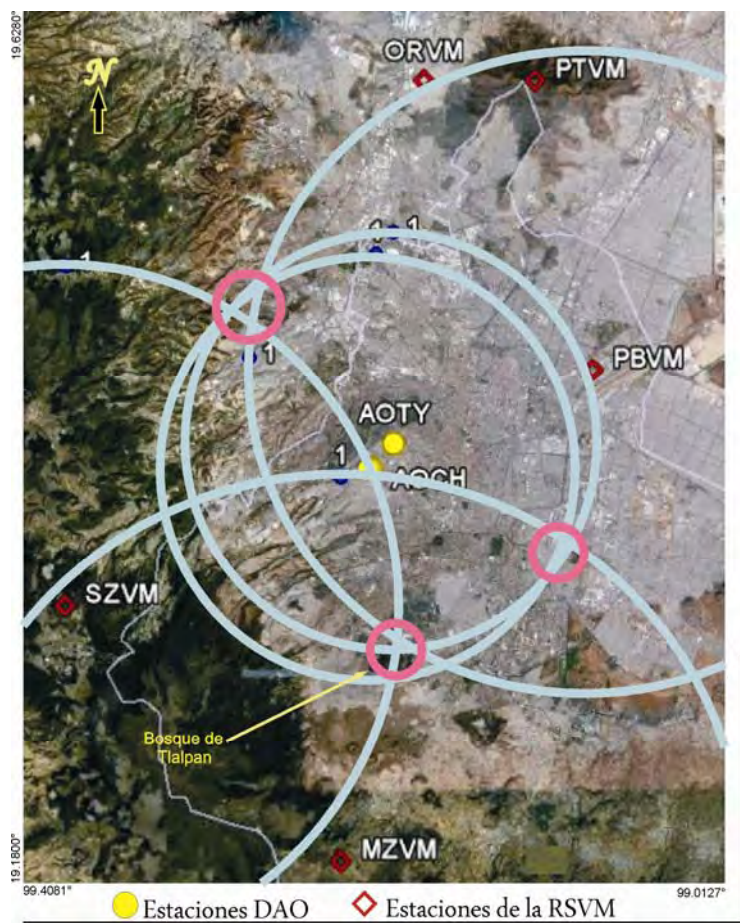
Figura 5.3: Epicentro del evento 1 para una velocidad de Basalto (Valor de V_{p3} en la tabla 5.4).
