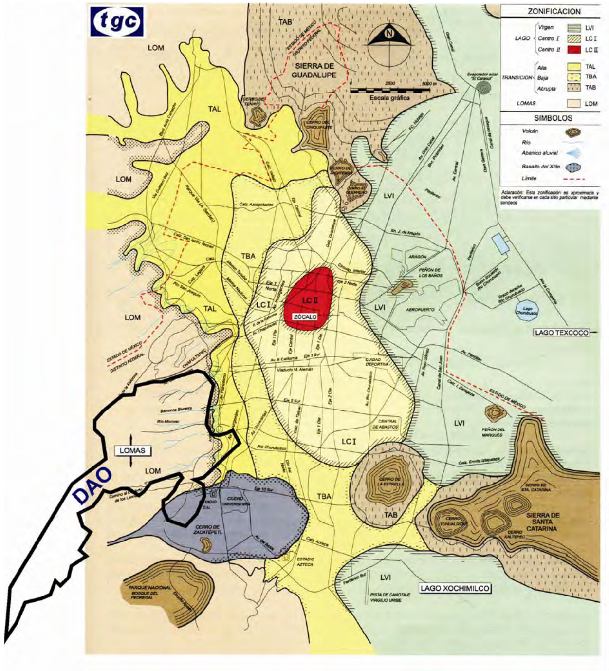
Figura 2.4.- Zonificación de la Cuenca de México, en la imagen se muestra la ubicación de la DAO en forma de bosquejo. Mapa modificado de (Santoyo-Villa, E., et al., 2005)
