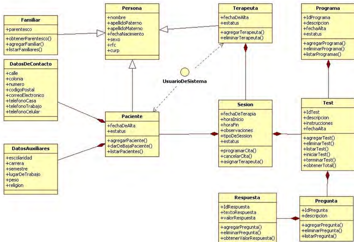
Figura 4.3 Diagrama de clases
