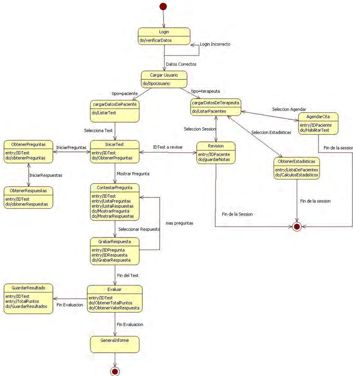
Figura 3.4 Diagrama de Estados
