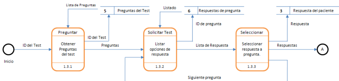
Diagrama de flujo de datos nivel 2.
