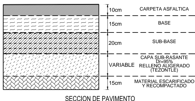
Fig. 15 Sección del pavimento
