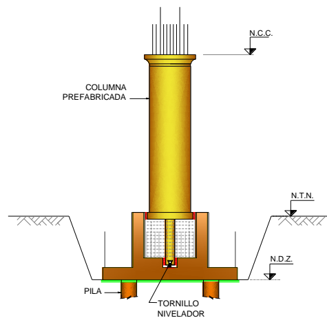
Detalle de montaje de columna
