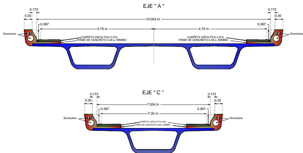
Distancias principales con respecto al parapeto de concreto
