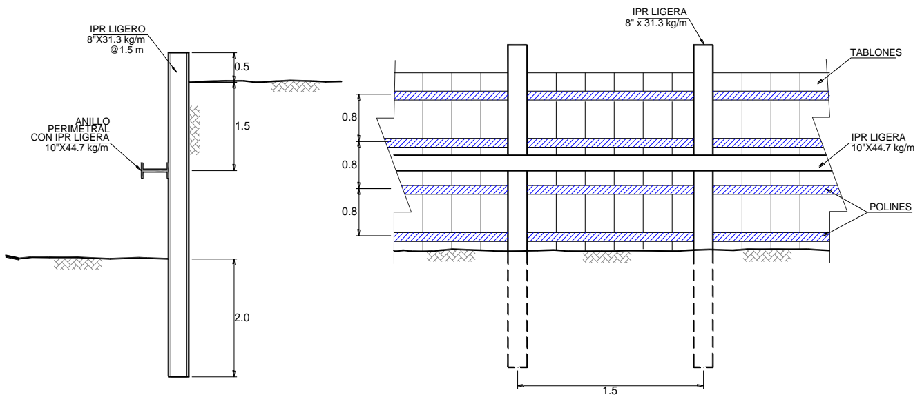
Sistema de Tablaestacado
