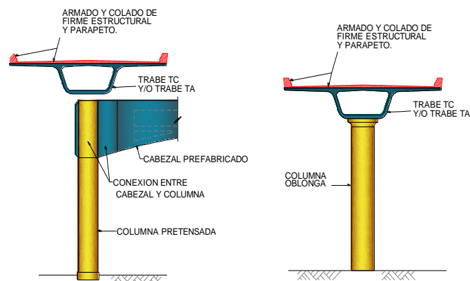
Detalle de Firme de compresión
