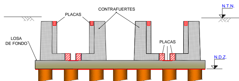
Ubicación de placas en contrafuertes
