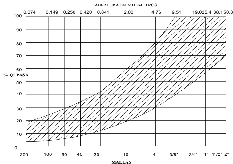
Fig. 17 Granulometría en relleno aligerado
