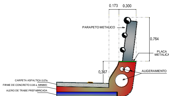
Detalle de parapeto metálico.
