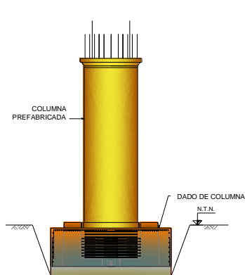
Armado y colado de segunda etapa
