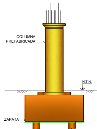
Relleno de zapata
