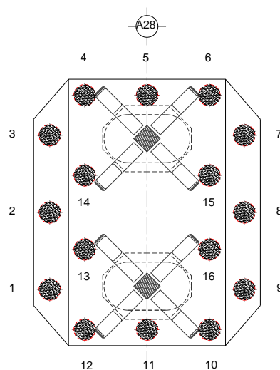
Planta de la zapata en el eje A-28, con la numeración de las pilas
