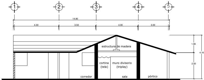
CORTE LONGITUDINAL X-X'
