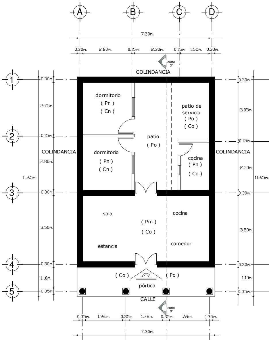
PLANTA ARQUITECTONICA
