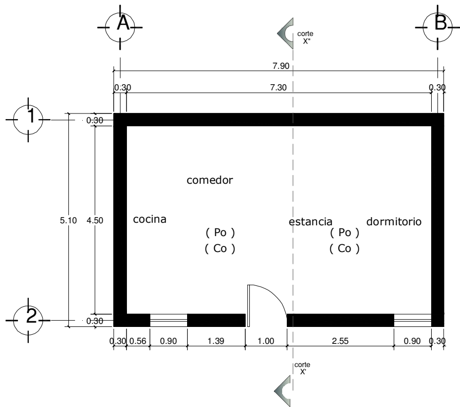
PLANTA ARQUITECTONICA
