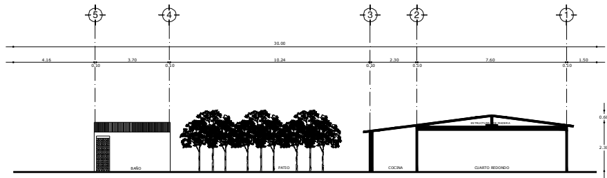
CORTE LONGITUDINAL X-X'
