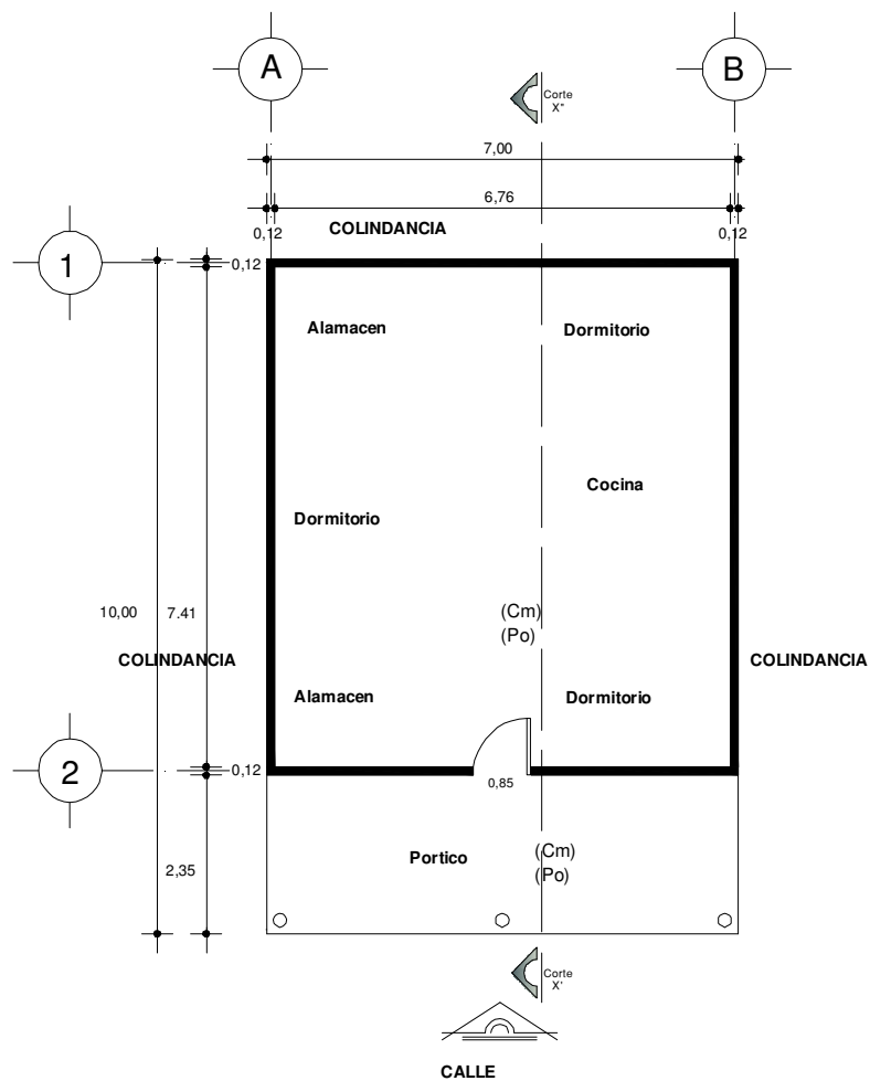
PLANTA ARQUITECTONICA
