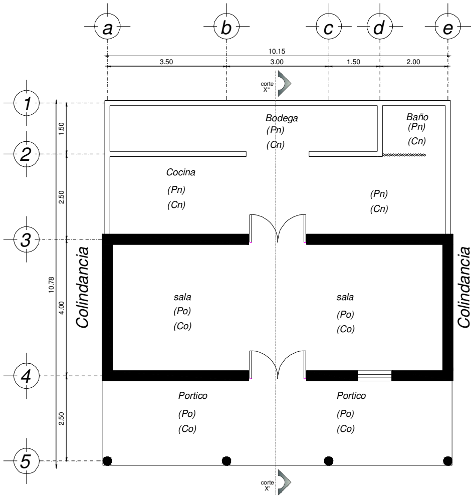
PLANTA ARQUITECTONICA
