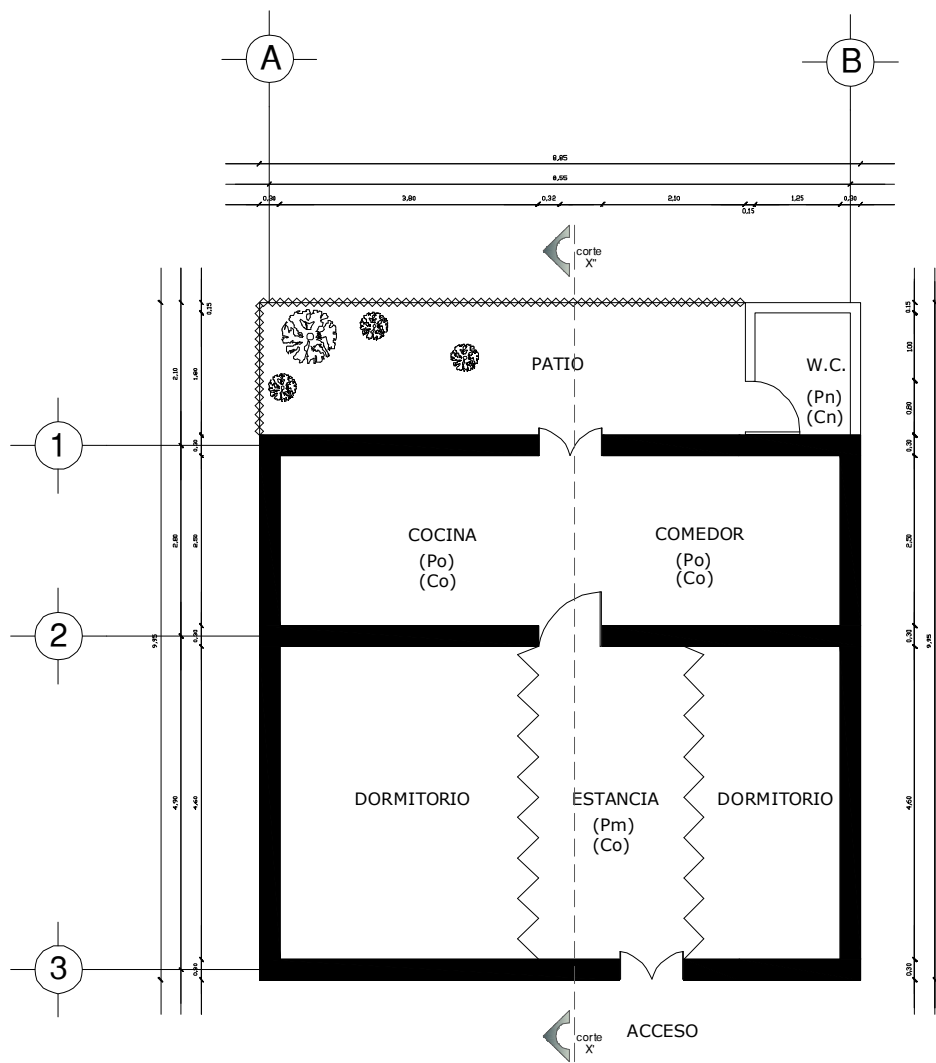
PLANTA ARQUITECTONICA
