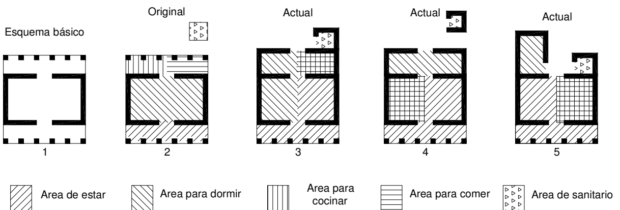
Figura V.5 Esquemas generales de la evolución de la vivienda tradicional
