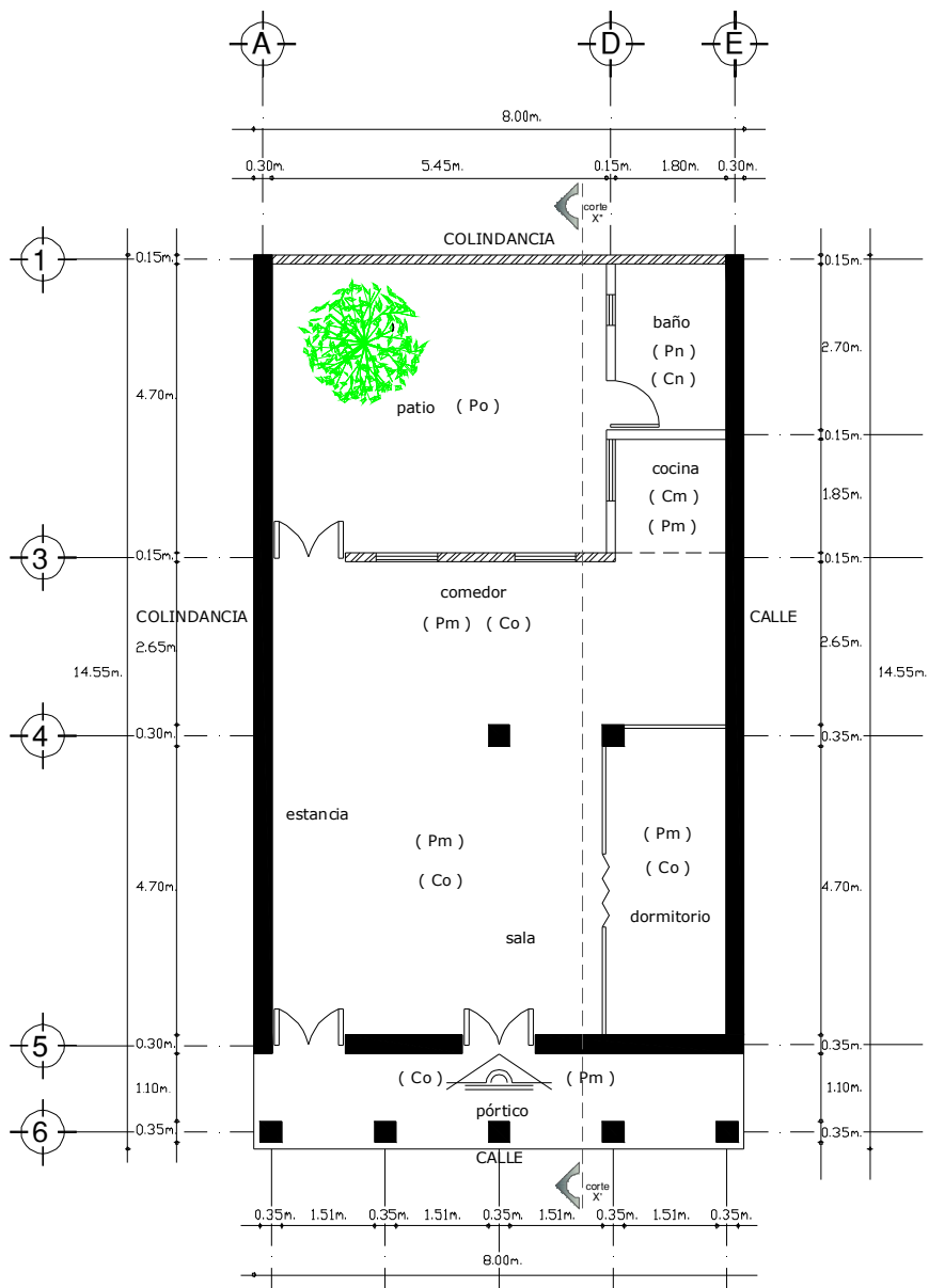
PLANTA ARQUITECTONICA
