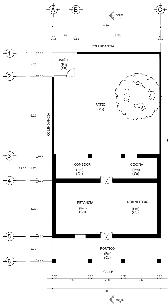
PLANTA ARQUITECTONICA
