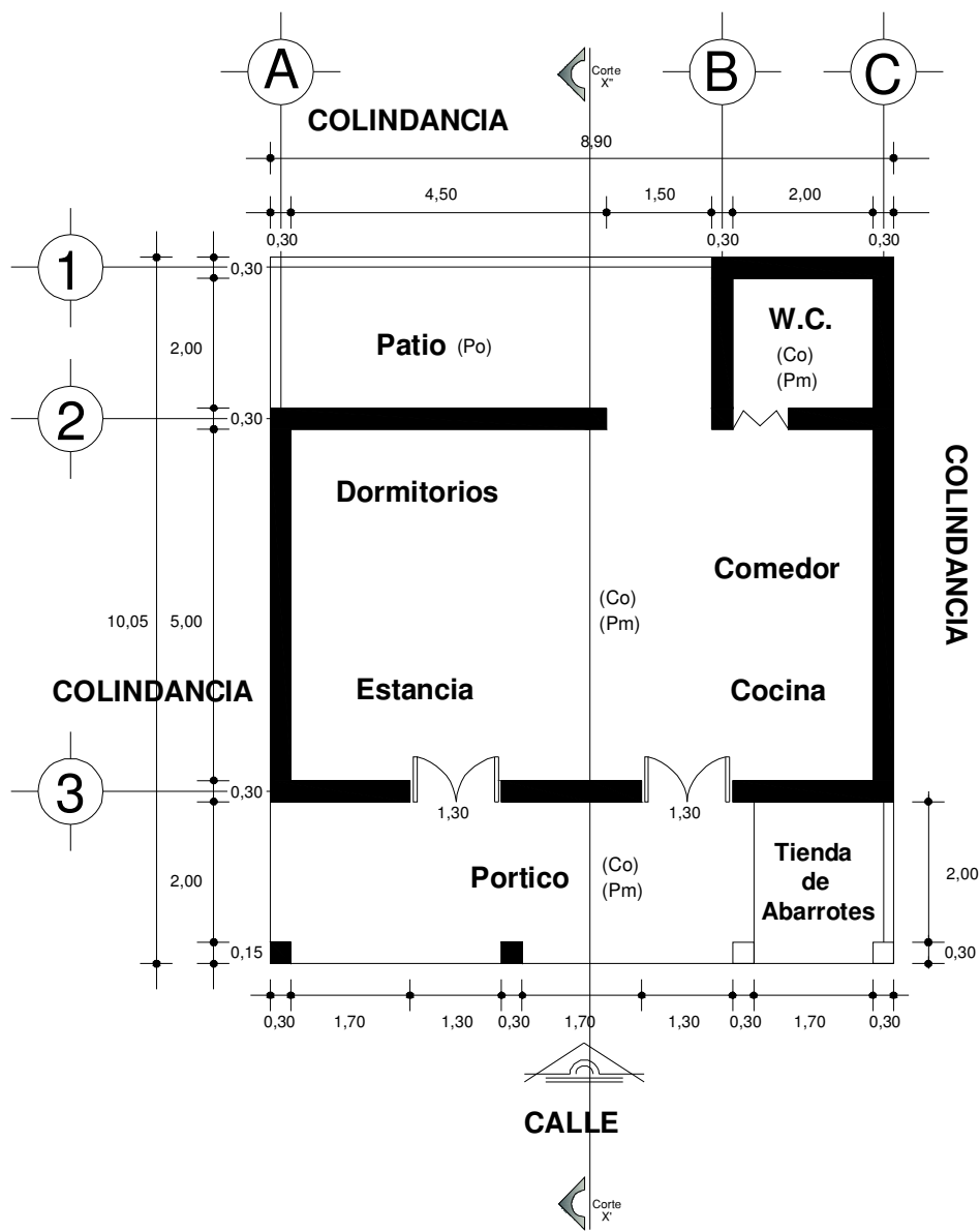
PLANTA ARQUITECTONICA
