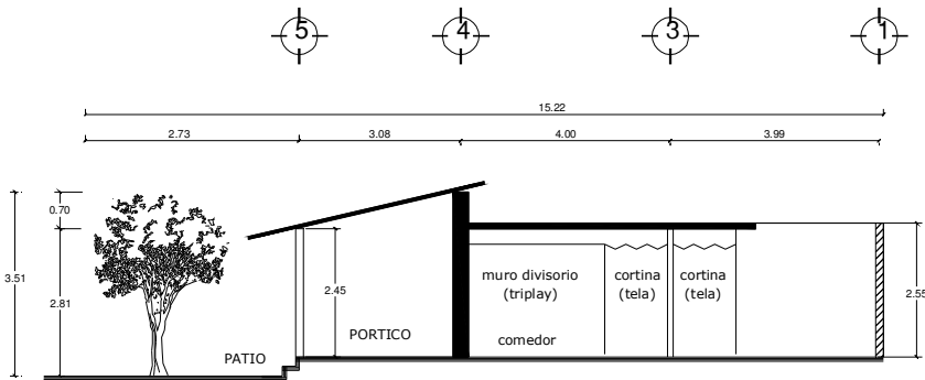
CORTE LONGITUDINAL X-X'
