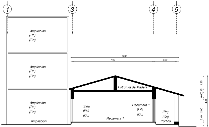
CORTE LONGITUDINAL X-X'
