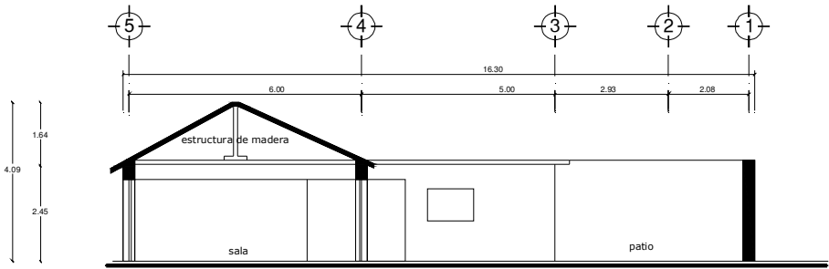
CORTE LONGITUDINAL X-X'
