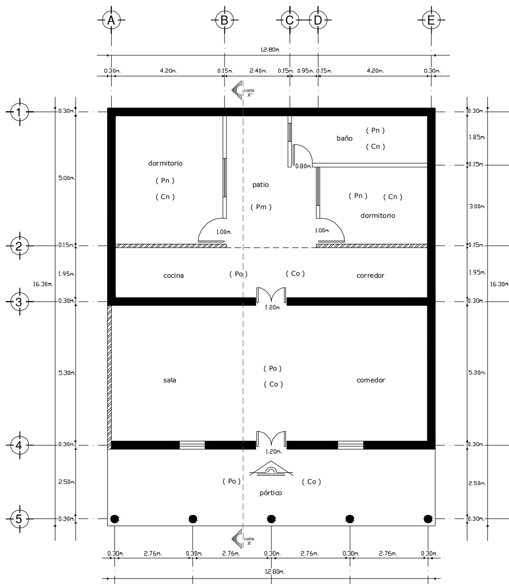
PLANTA ARQUITECTONICA
