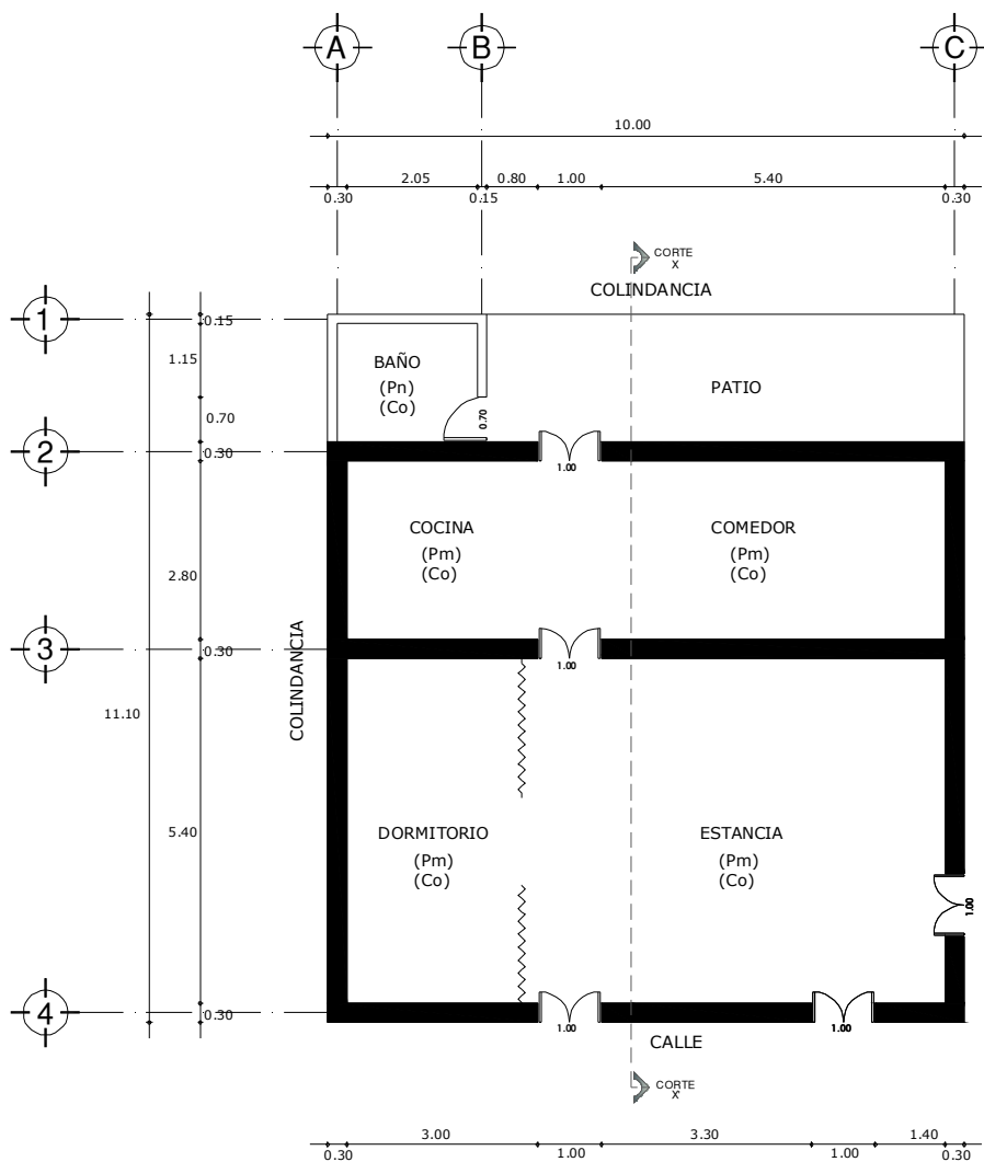
PLANTA ARQUITECTONICA
