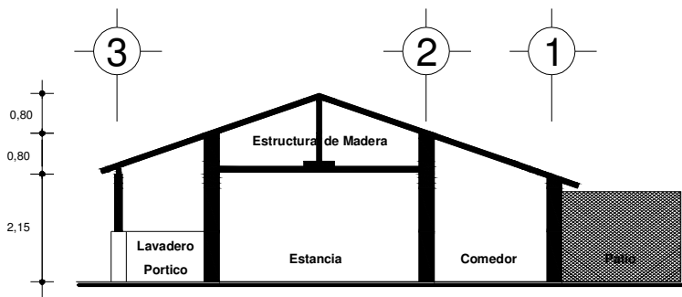
CORTE LONGITUDINAL X-X'
