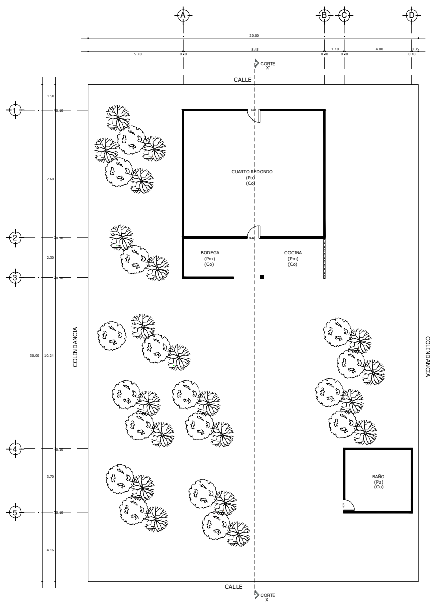
PLANTA ARQUITECTONICA
