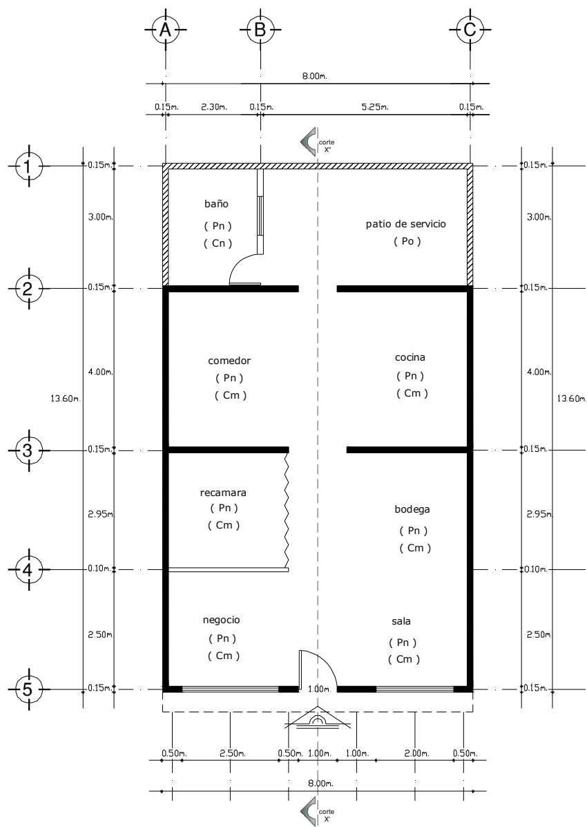
PLANTA ARQUITECTONICA
