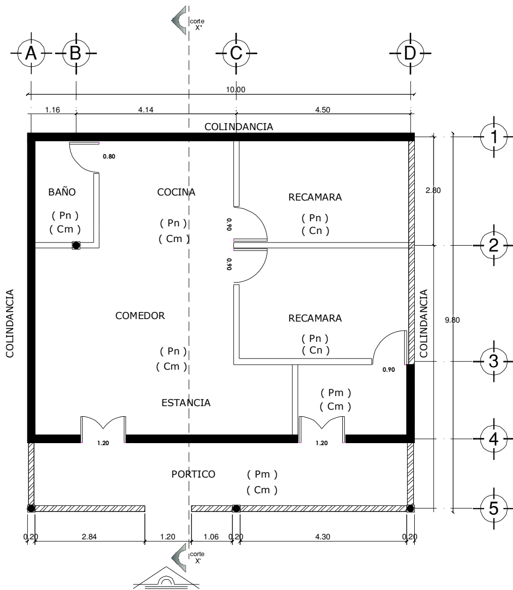
PLANTA ARQUITECTONICA
