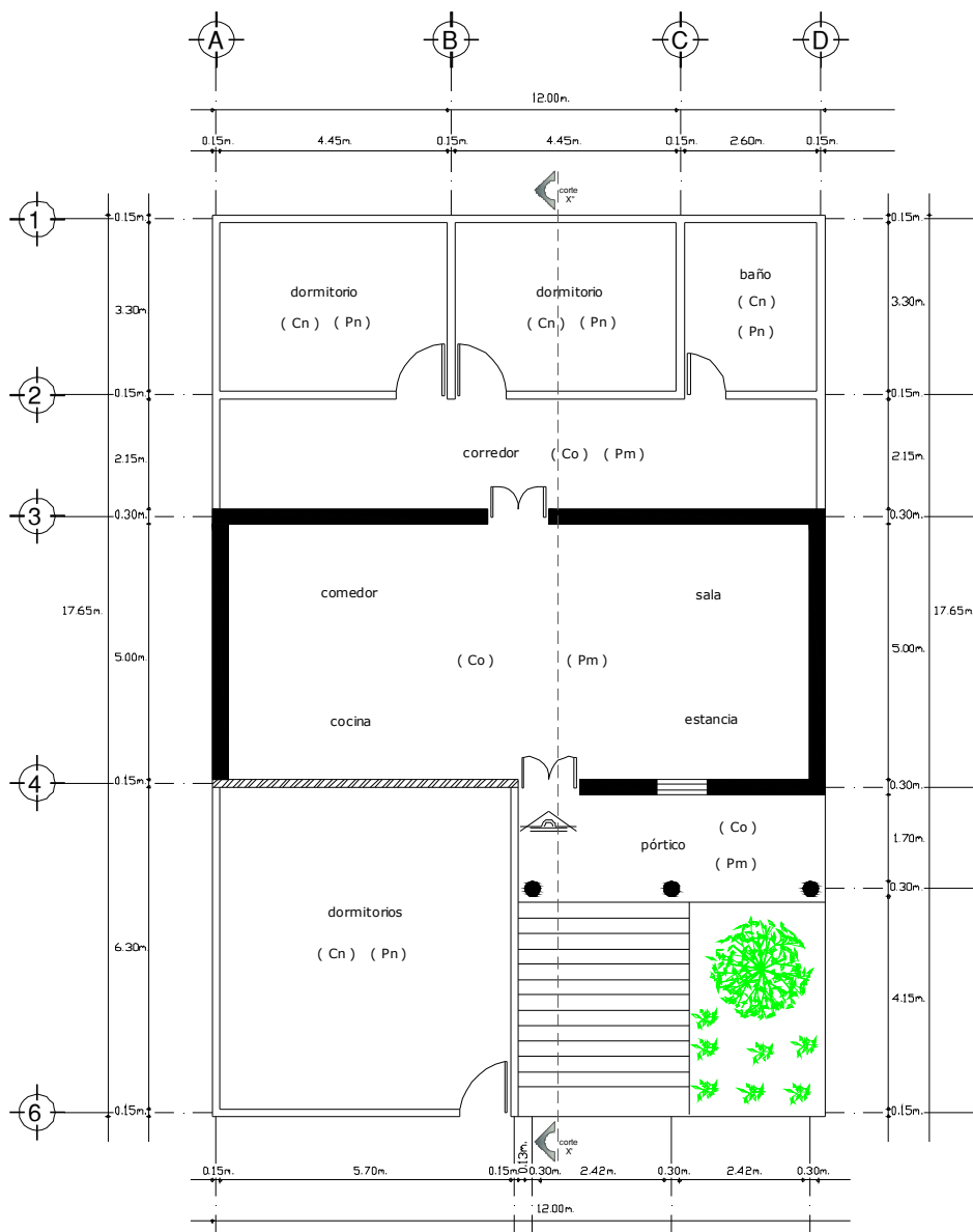
PLANTA ARQUITECTONICA
