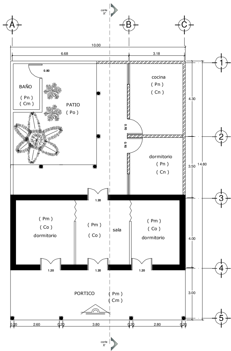
PLANTA ARQUITECTONICA
