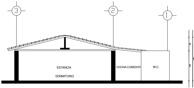
CORTE LONGITUDINAL X-X'
