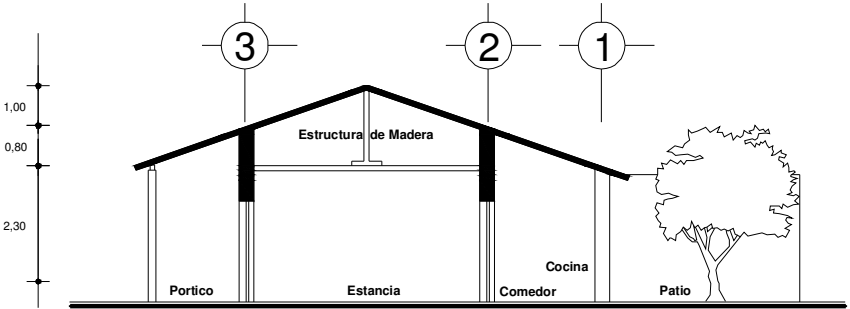
CORTE LONGITUDINAL X-X'
