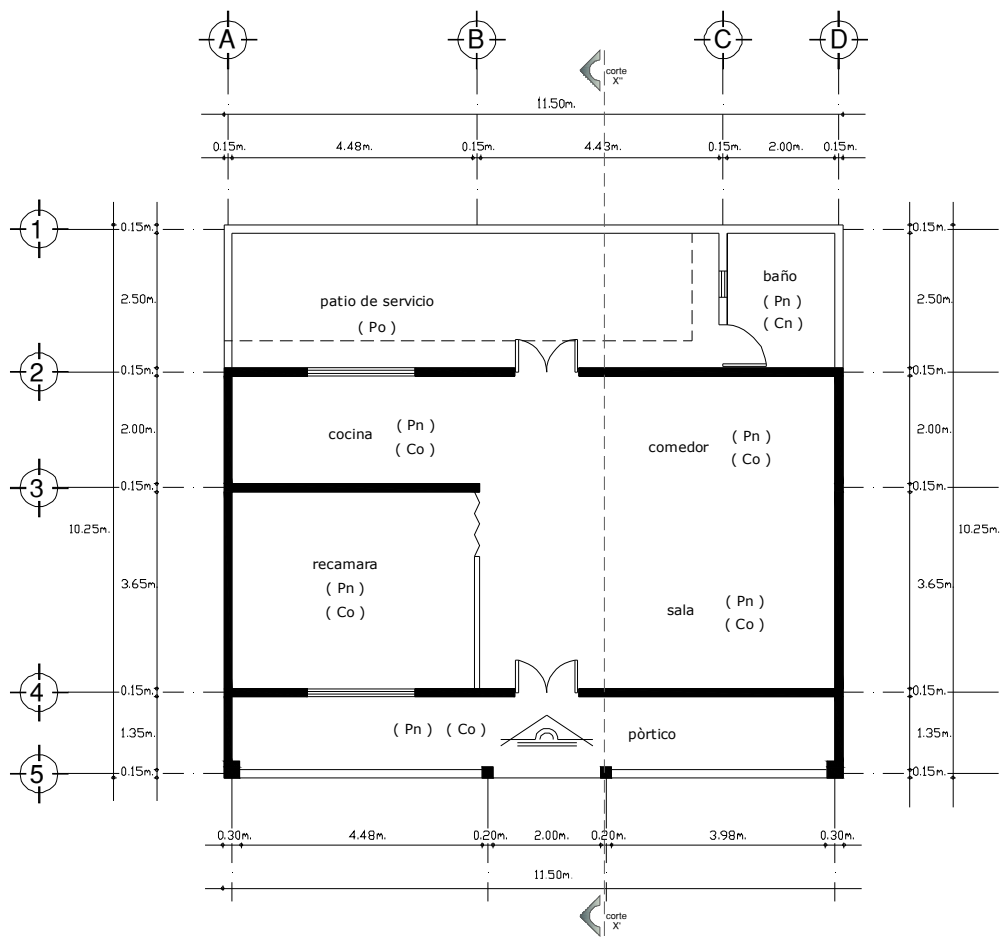
PLANTA ARQUITECTONICA
