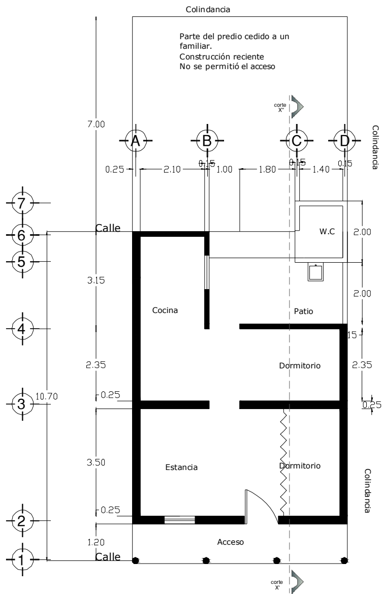
PLANTA ARQUITECTONICA
