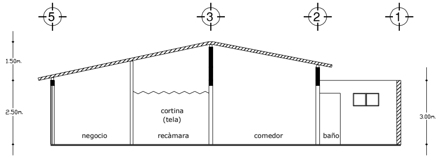
CORTE LONGITUDINAL X-X'
