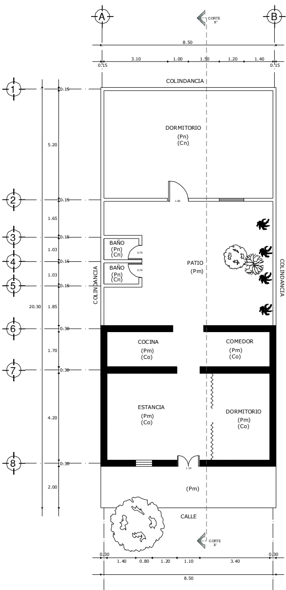
PLANTA ARQUITECTONICA
