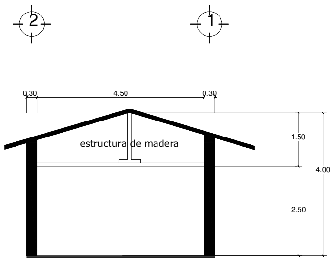
CORTE LONGITUDINAL X-X'
