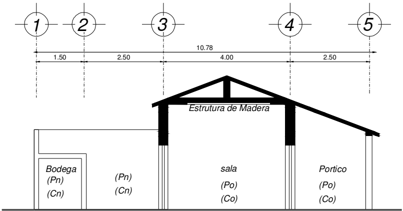
CORTE LONGITUDINAL X-X'
