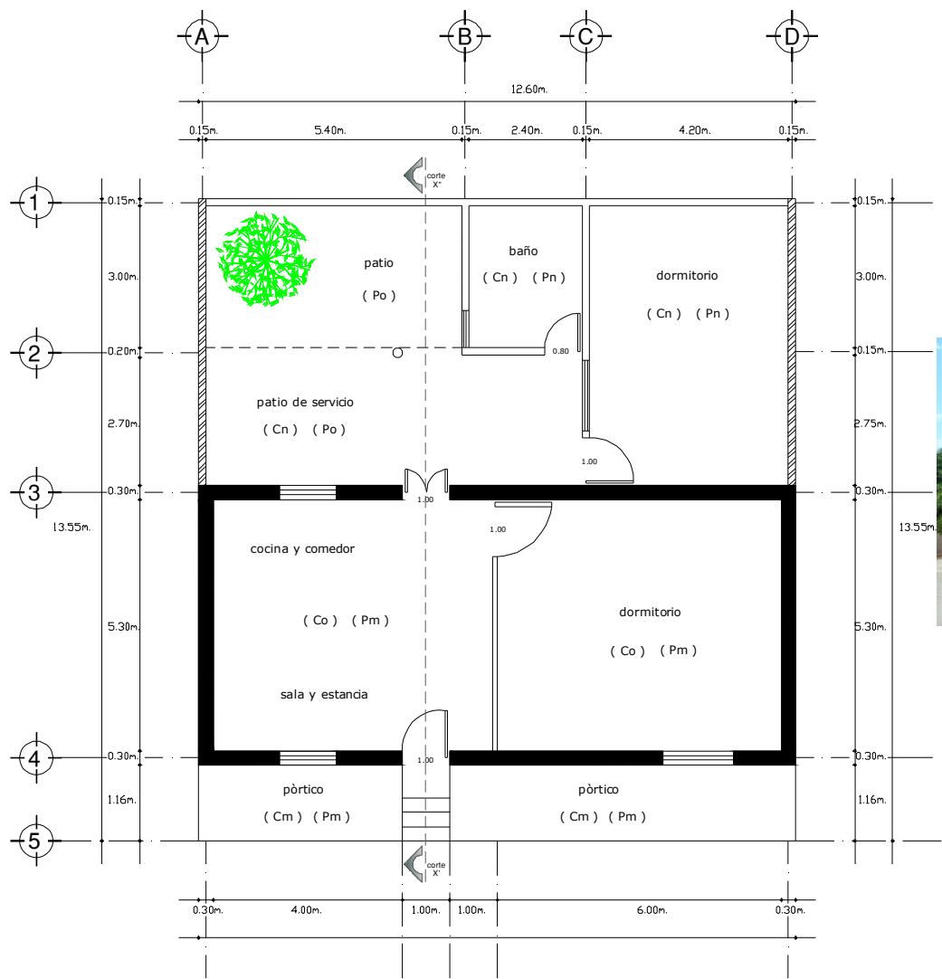
PLANTA ARQUITECTONICA
