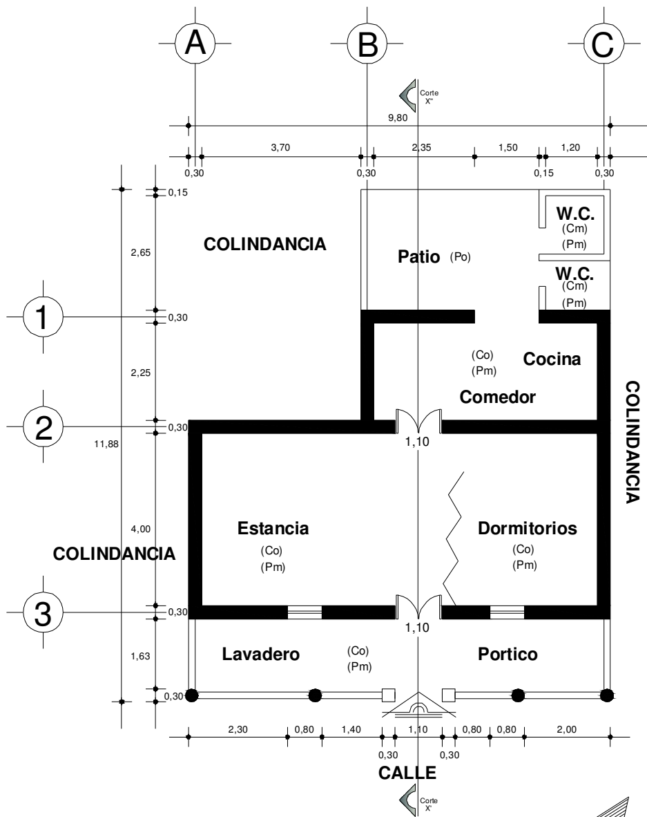
PLANTA ARQUITECTONICA
