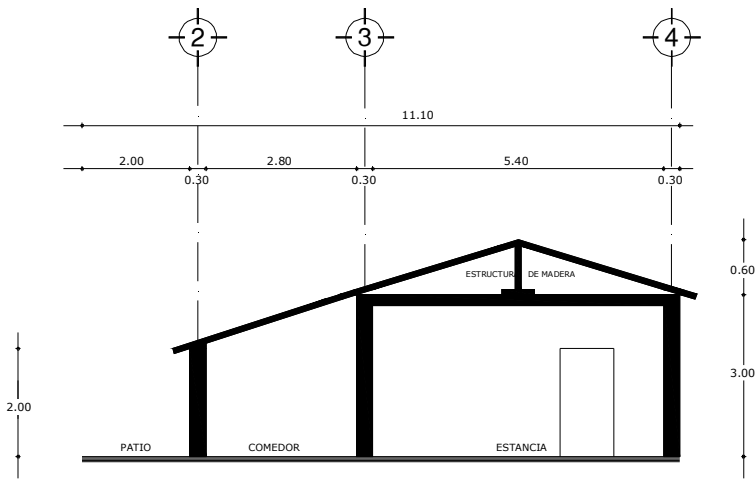
CORTE LONGITUDINAL X-X'
