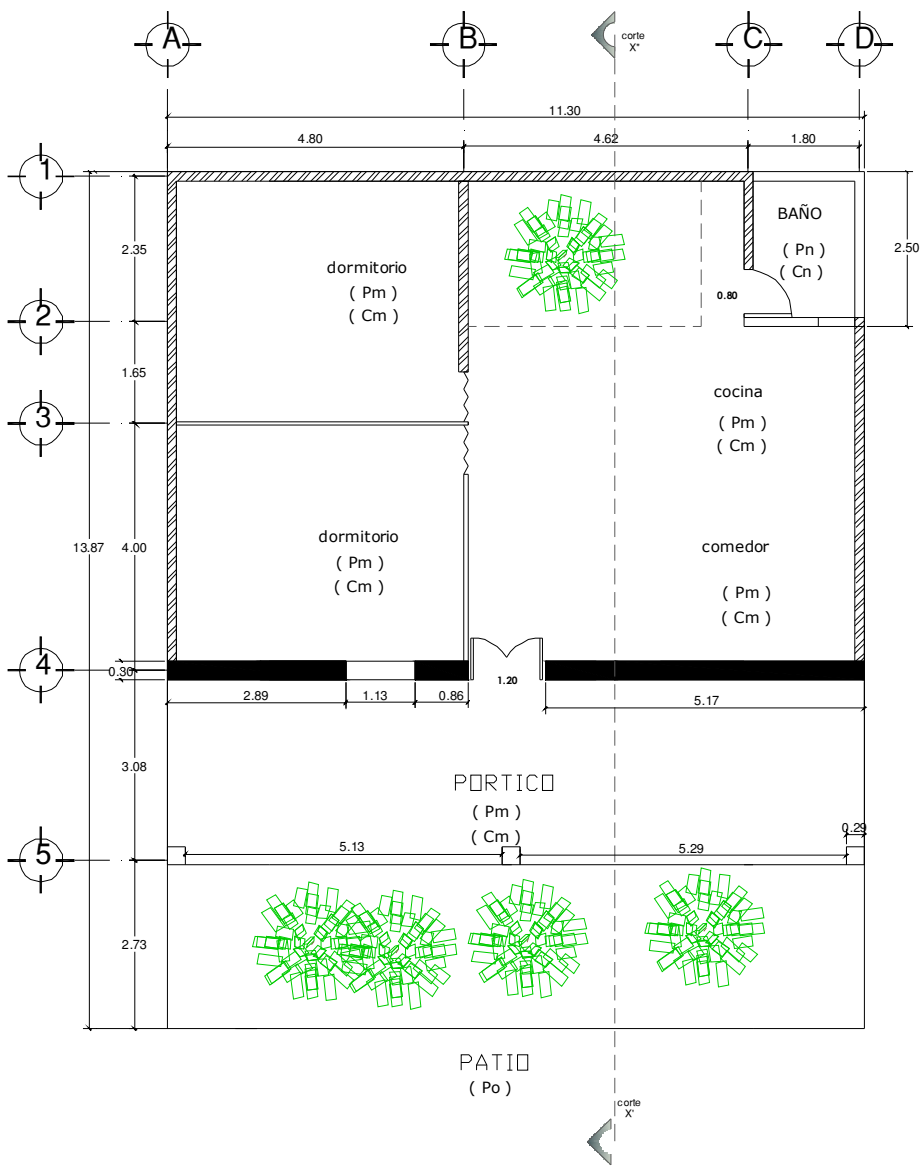
PLANTA ARQUITECTONICA
