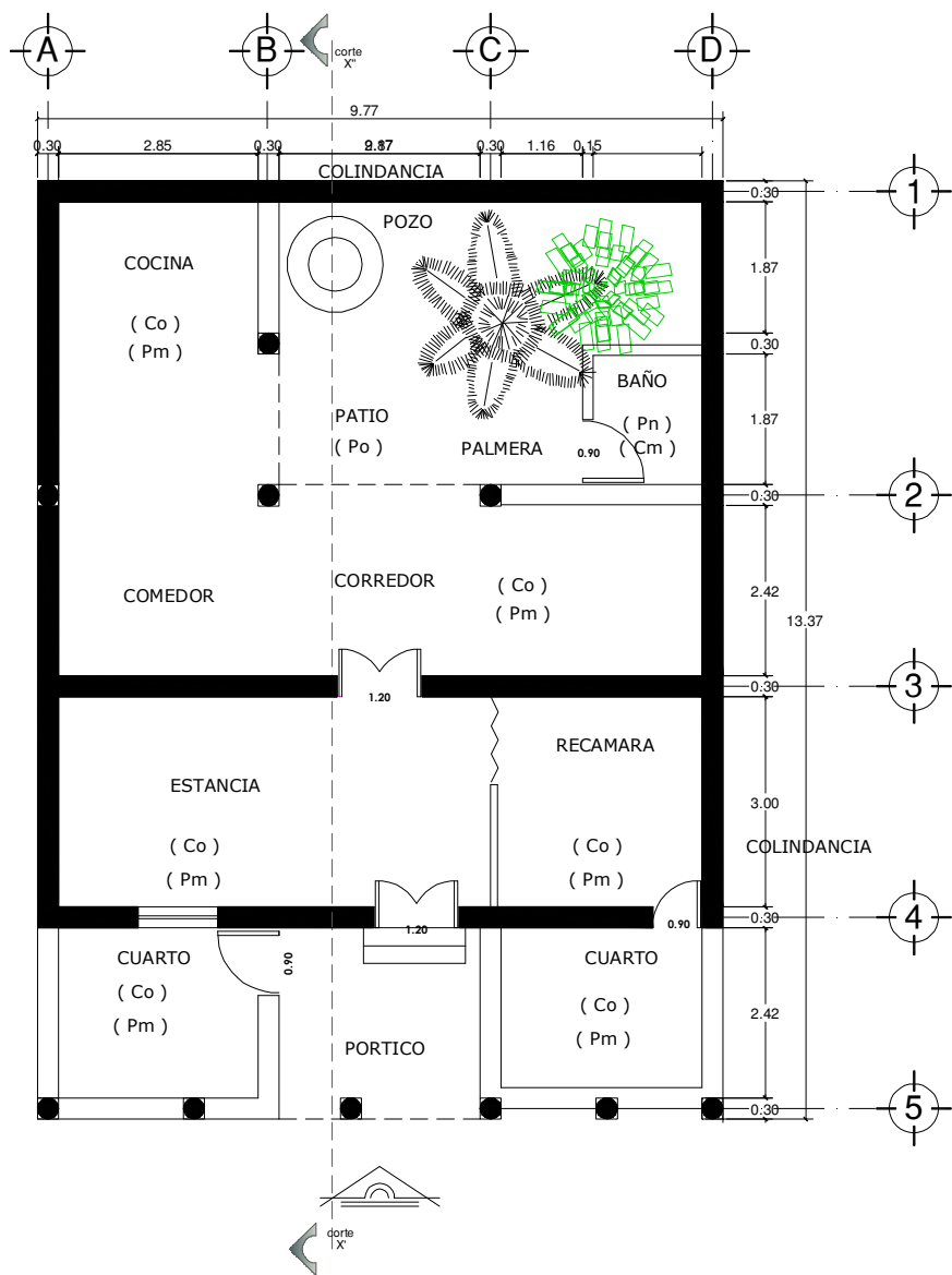
PLANTA ARQUITECTONICA
