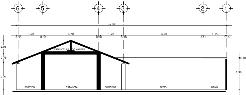
CORTE LONGITUDINAL X-X'
