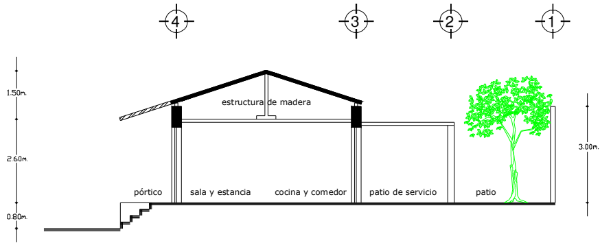
CORTE LONGITUDINAL X-X'
