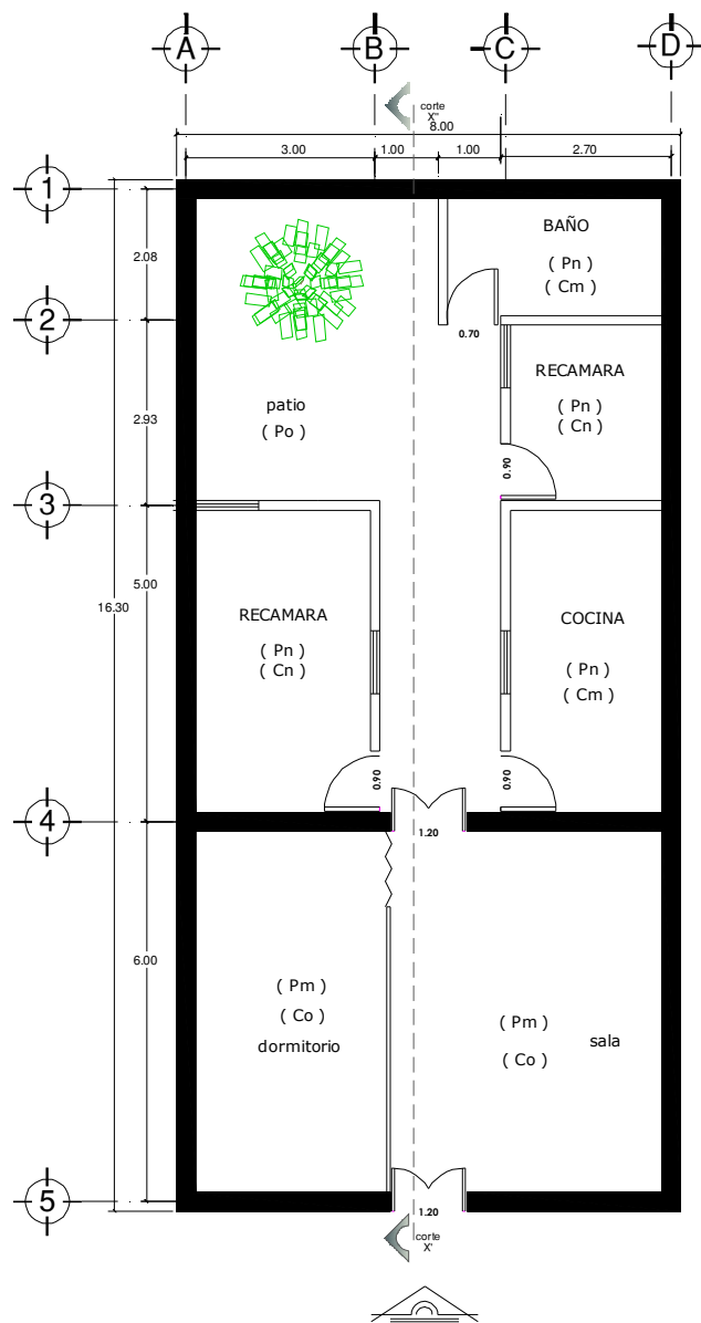
PLANTA ARQUITECTONICA
