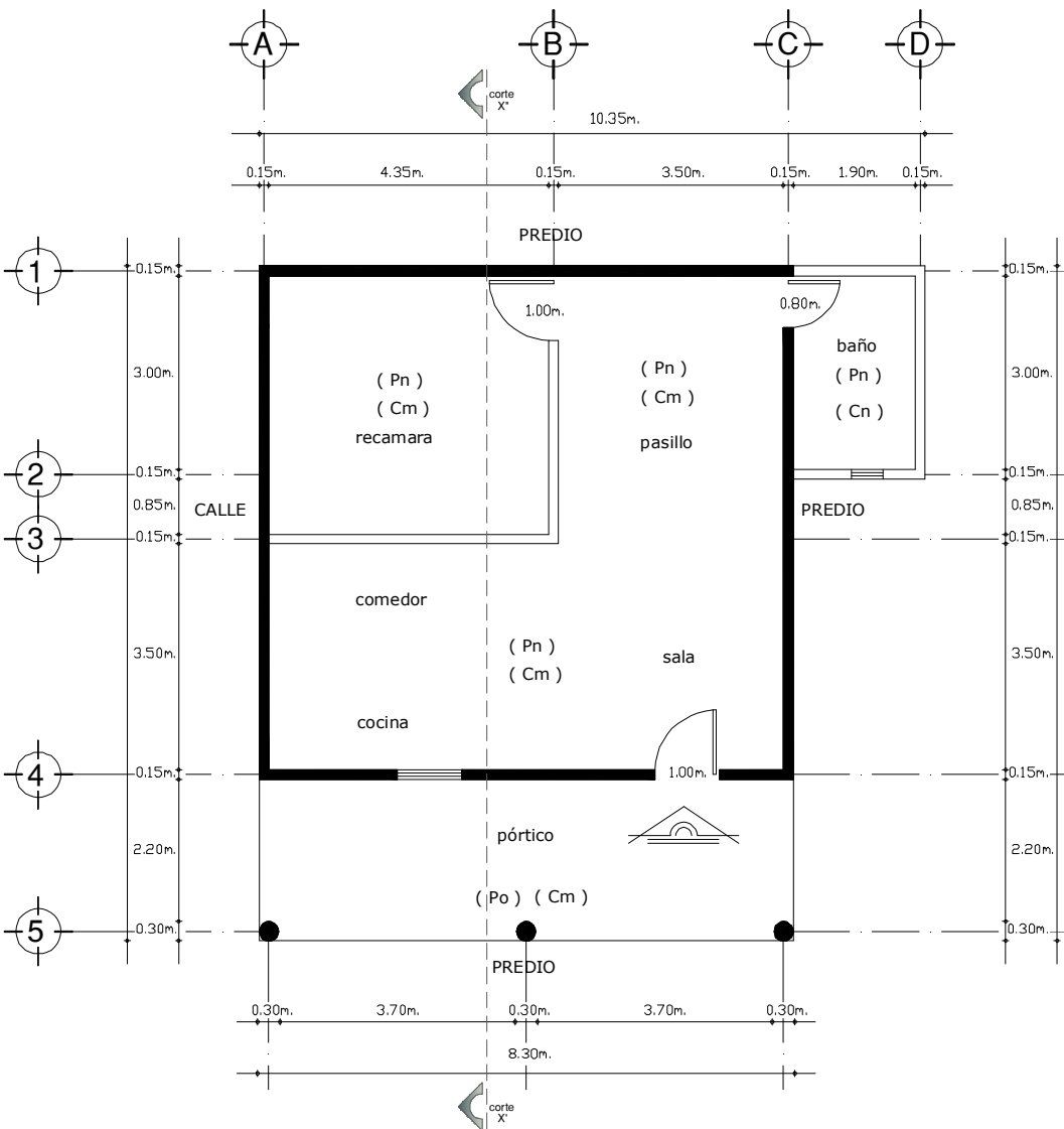
PLANTA ARQUITECTONICA
