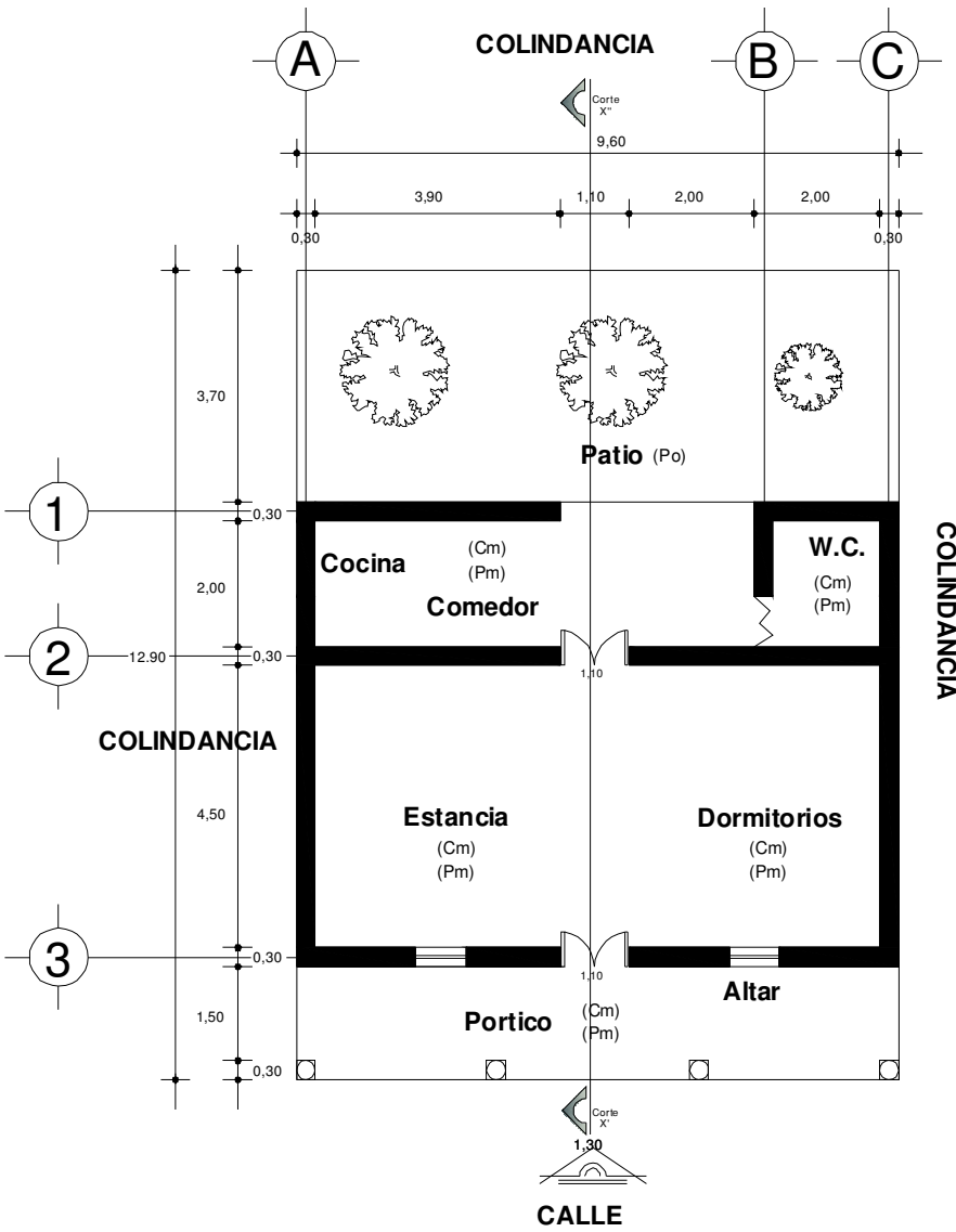
PLANTA ARQUITECTONICA
