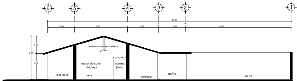
CORTE LONGITUDINAL X-X'
