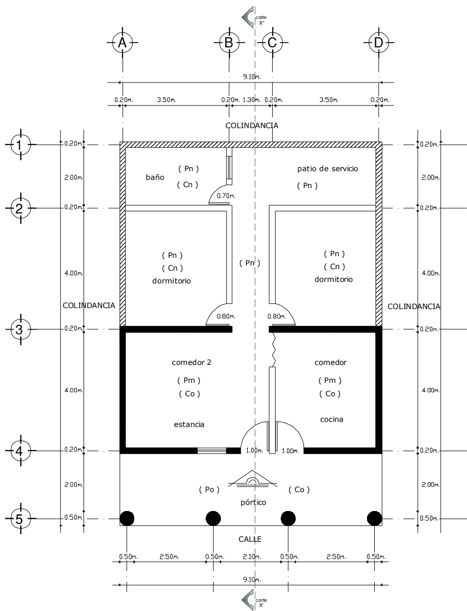
PLANTA ARQUITECTONICA
