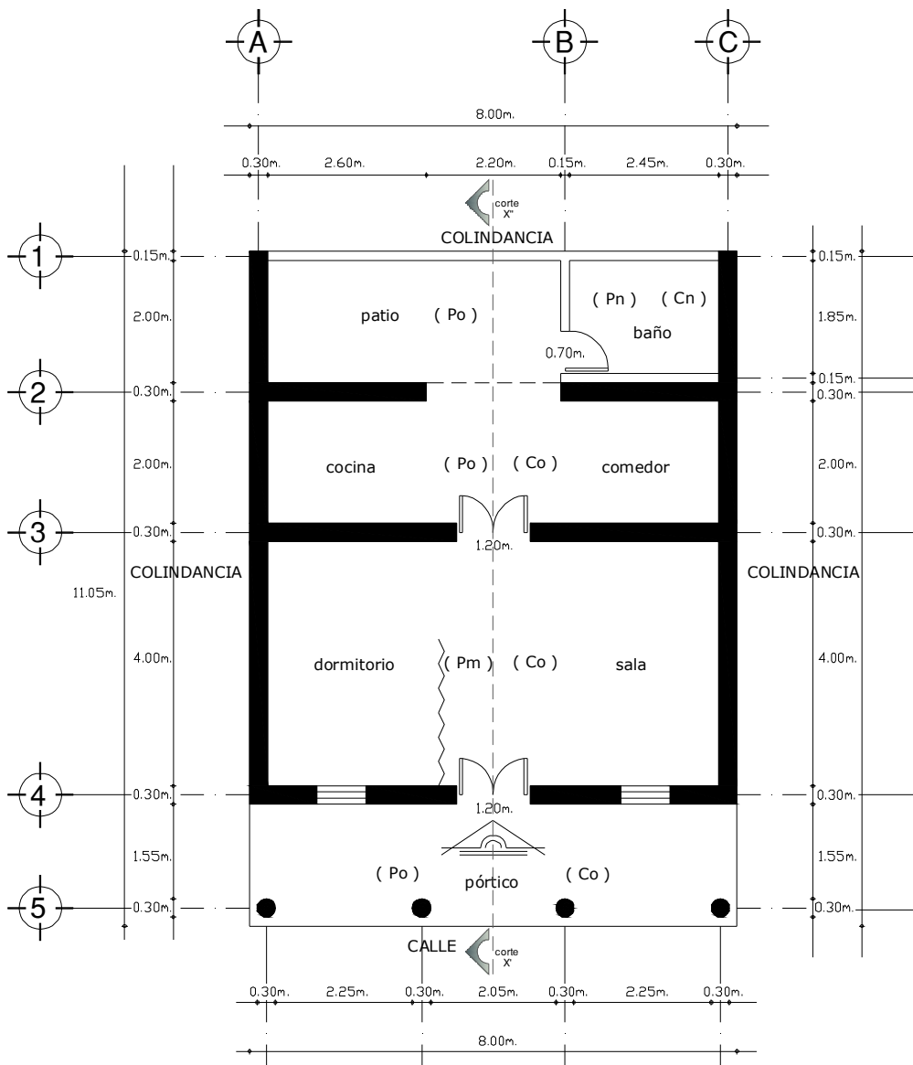
PLANTA ARQUITECTONICA
