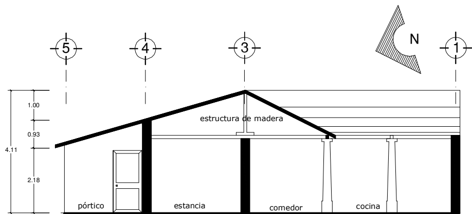
CORTE LONGITUDINAL X-X'
