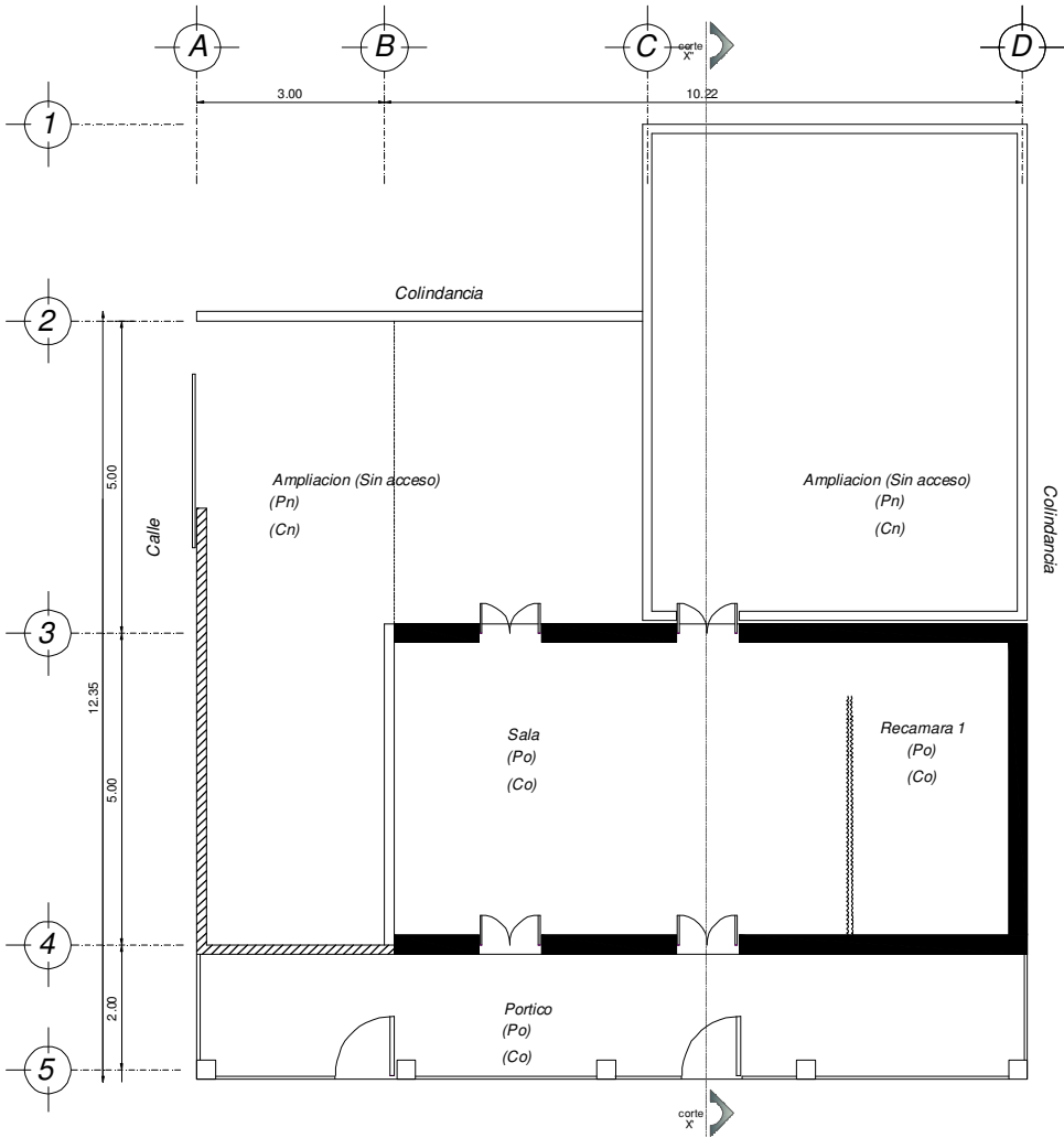
PLANTA ARQUITECTONICA
