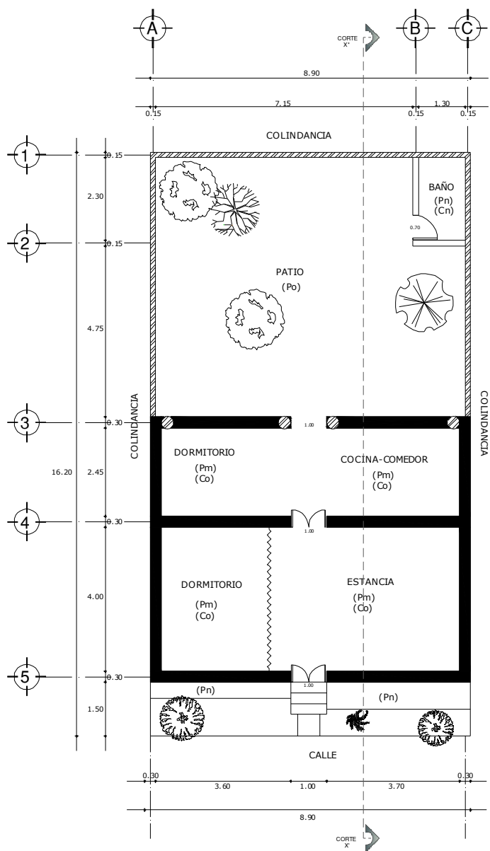
PLANTA ARQUITECTONICA
