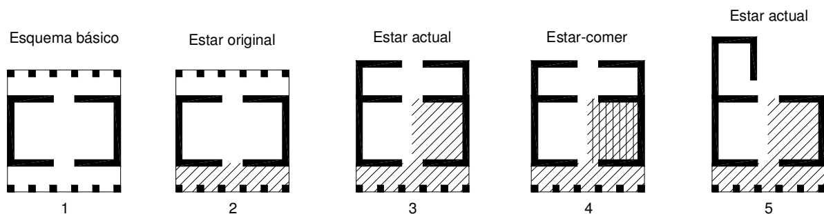
Figura V.1 Esquemas generales de la evolución de la zona de estar en la vivienda tradicional
