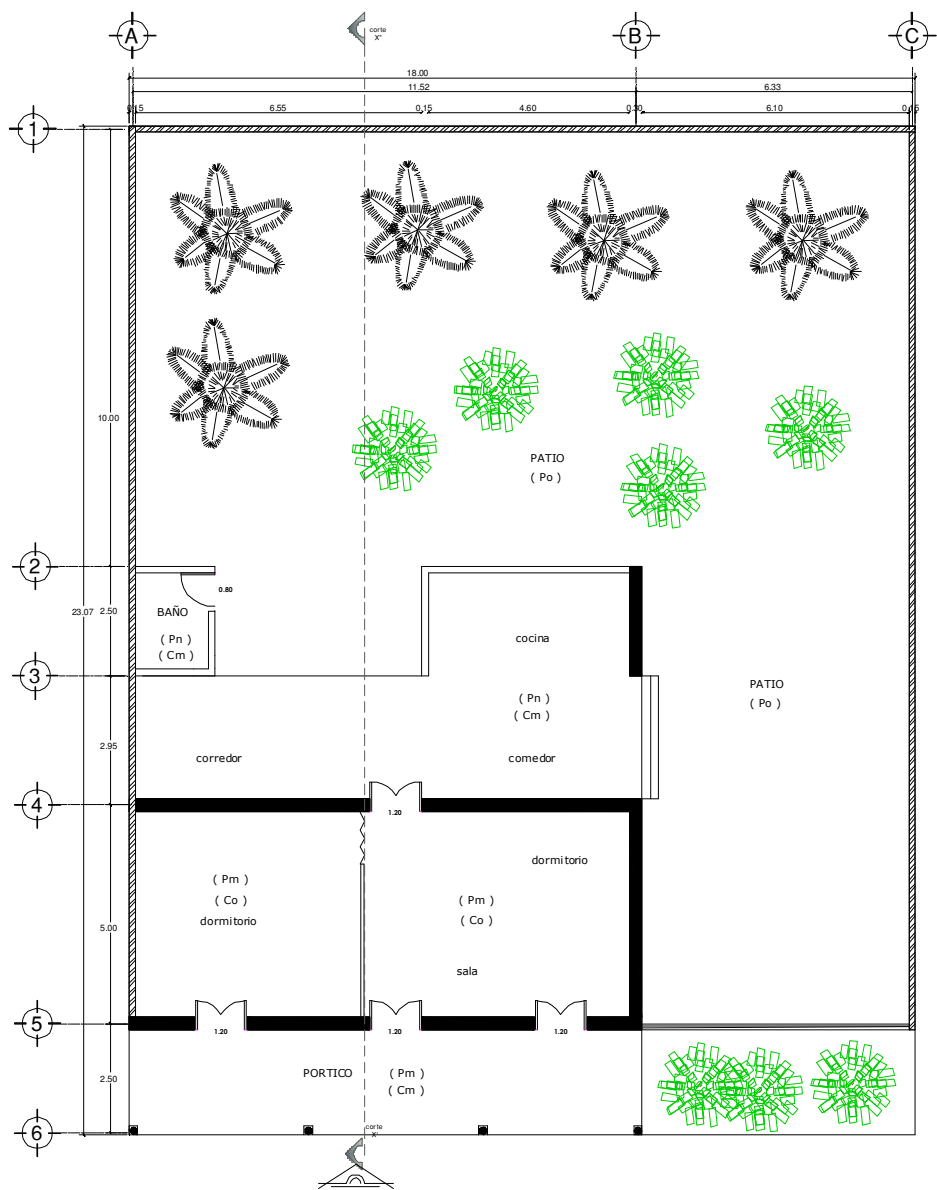
PLANTA ARQUITECTONICA
