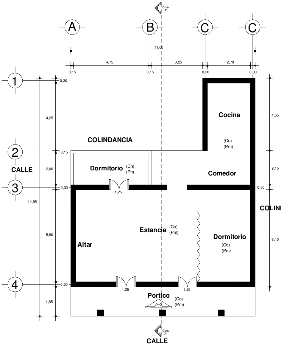
PLANTA ARQUITECTONICA
