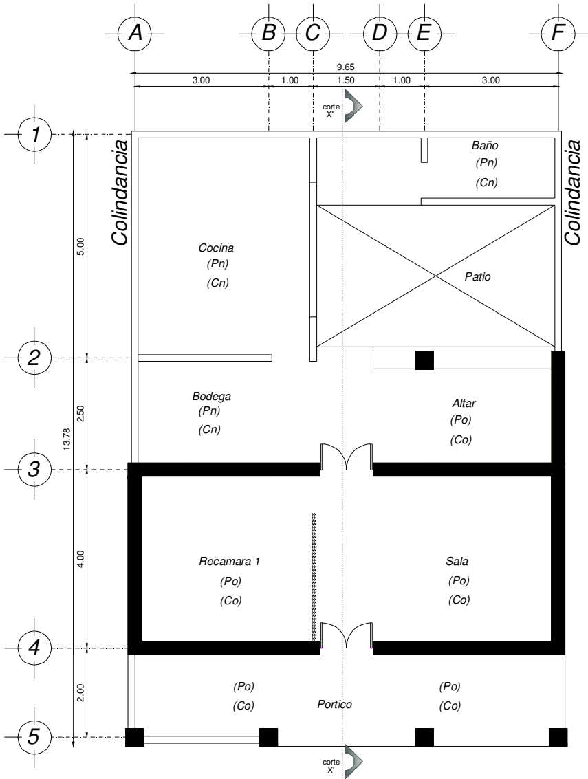
PLANTA ARQUITECTONICA
