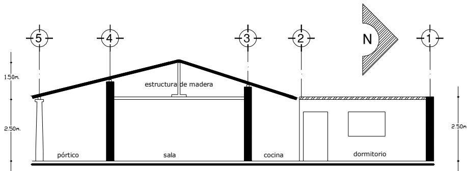
CORTE LONGITUDINAL X-X'
