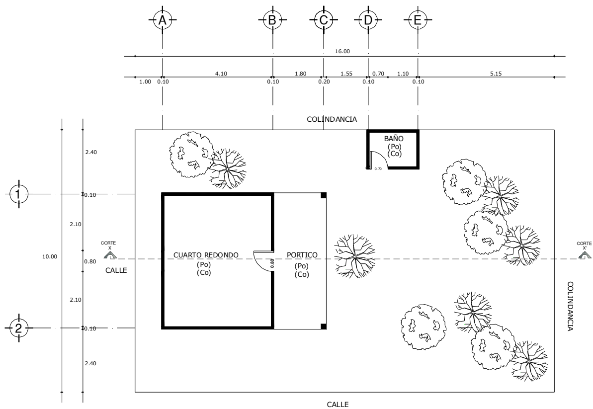
PLANTA ARQUITECTONICA
