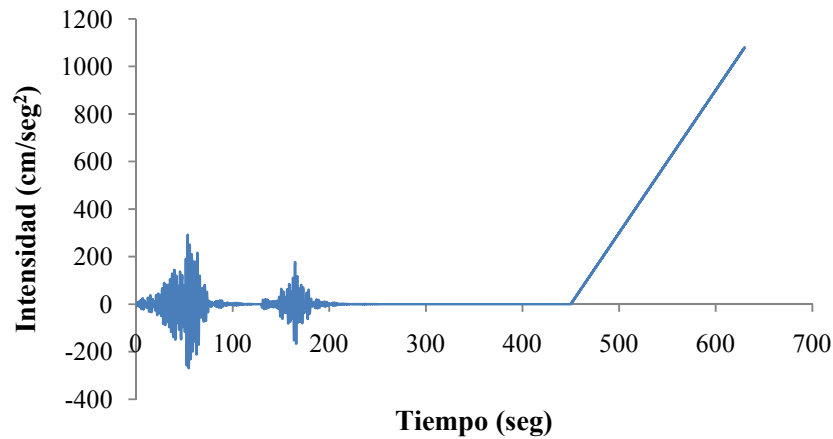
Figura 5.1. Ejemplo de dos movimientos sísmicos y una aceleración monotonía creciente.
