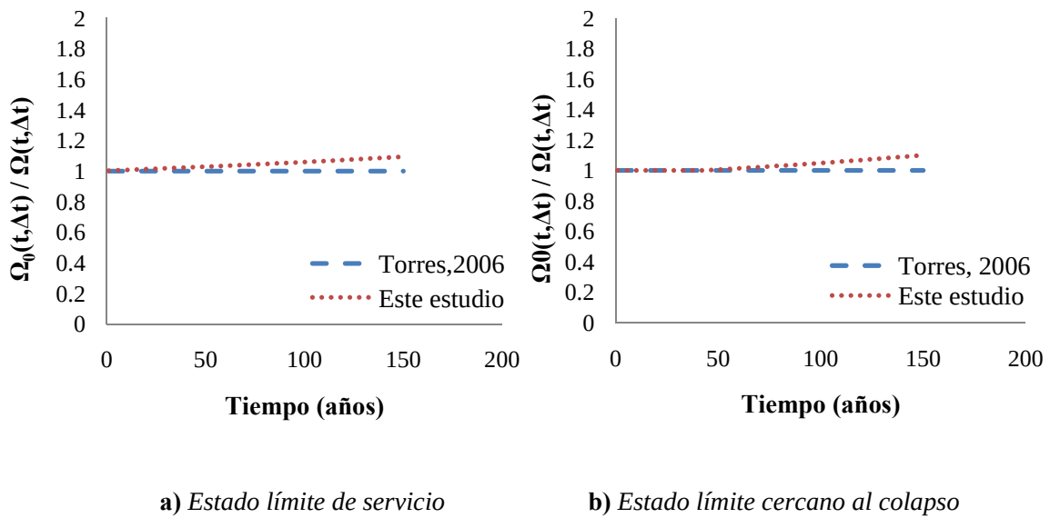
Figura 7.2. Relación de factores de corrección \frac{\Omega_0(t,\Delta t)}{\Omega(t,\Delta t)} para distorsiones máximas de azotea.
