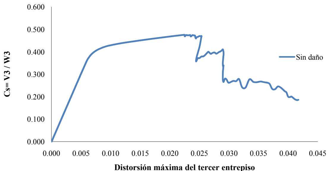
(a) Estructura sin daño acumulado (0 años)
