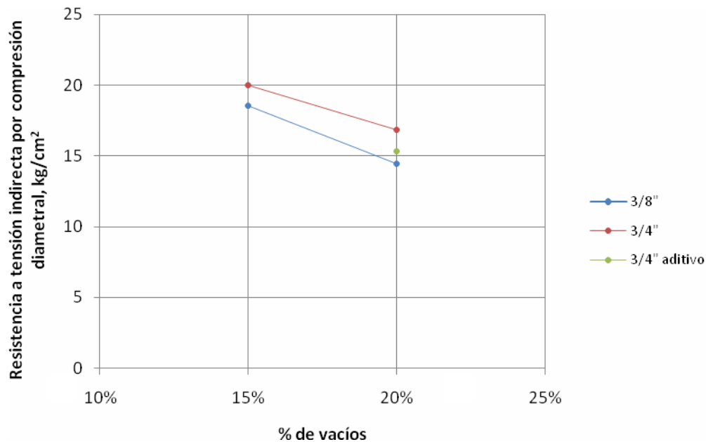
Figura 6.15 Relación entre resistencia a tensión indirecta por compresión diametral a 28 días y el porcentaje de vacíos.
