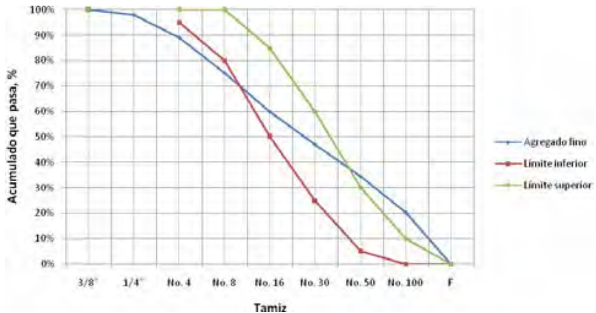
Figura 6.3 Distribución de la curva granulométrica del agregado fino de acuerdo a los límites superior e inferior de la norma ASTM C33.
