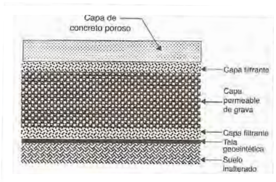
Figura 4.1 Estructura de un pavimento de concreto permeable (ACI 522, 2006).
