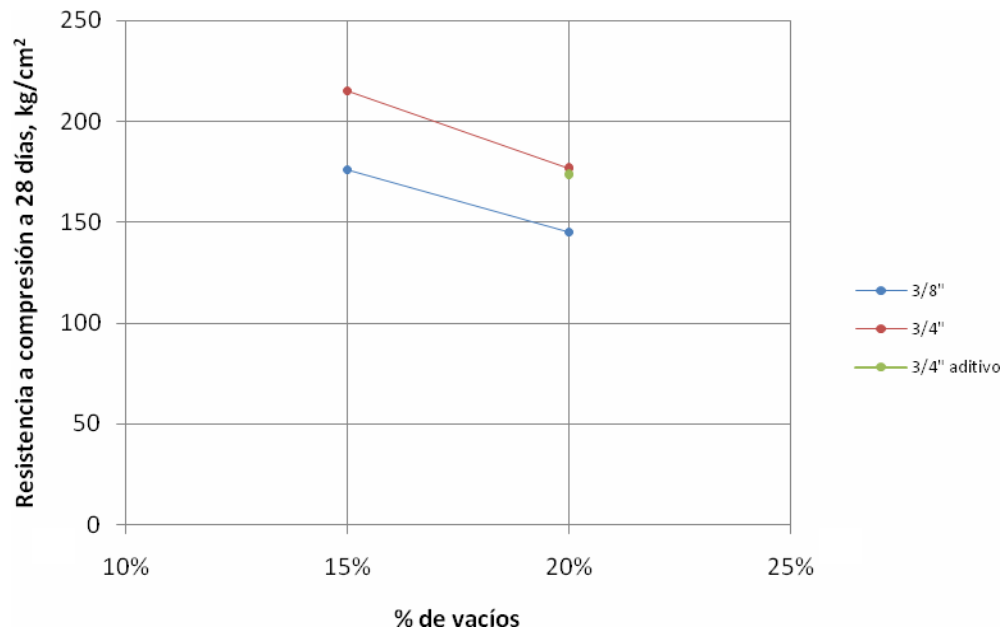
Figura 6.12 Relación entre la resistencia a compresión a 28 días y el porcentaje de vacíos.
