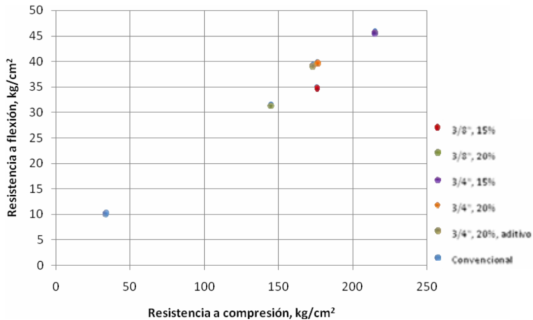
Figura 6.18 Relación entre la resistencia a flexión y la resistencia a compresión.
