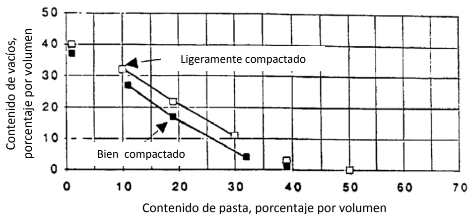
Figura 2.3 Relación entre el contenido de vacíos y el contenido de pasta para agregado No. 8 (3/8") (ACI 211.3R, 1998).
