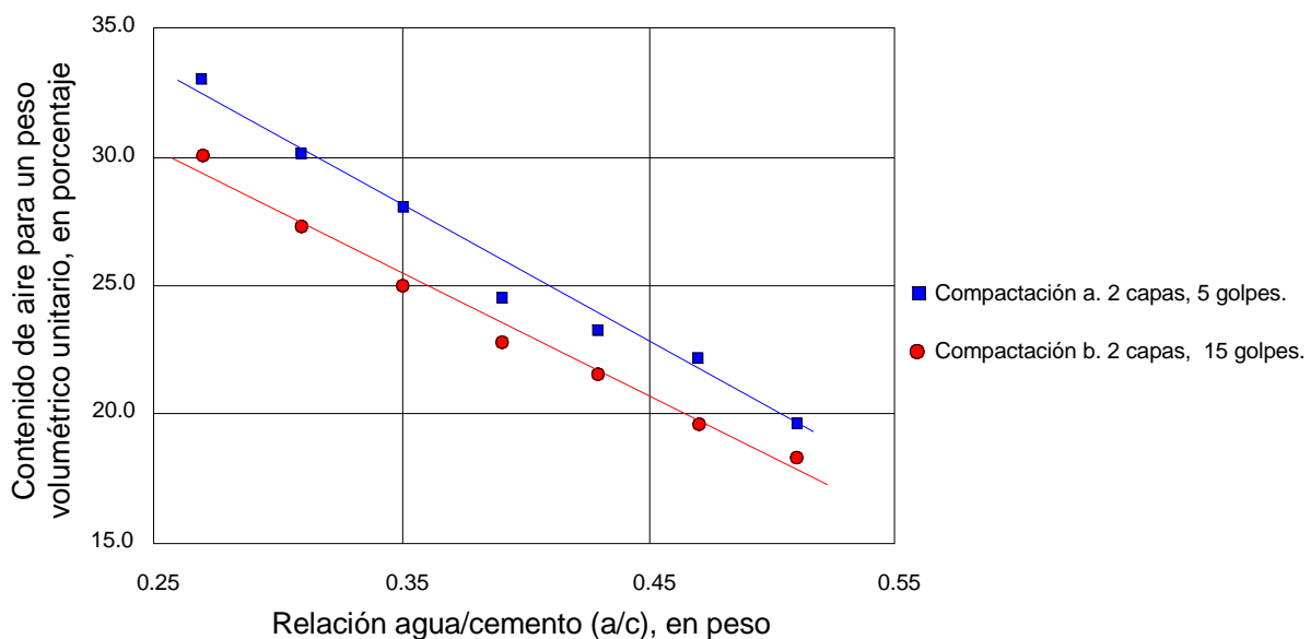
Figura 3.1 Relación entre el contenido de aire y la relación agua/cemento para el concreto permeable (Meininger, 1988).
