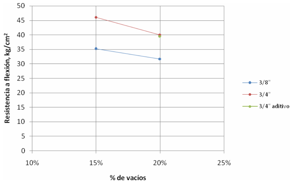
Figura 6.17 Relación entre la resistencia a flexión a 28 días y el porcentaje de vacíos.
