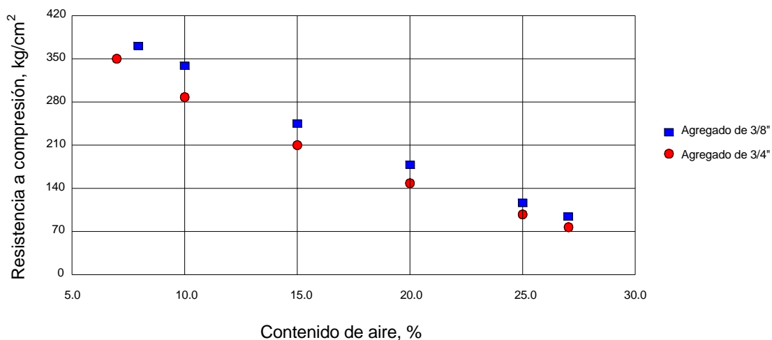
Figura 3.3 Relación entre la resistencia a compresión a 28 días y el contenido de aire para agregado de 3/8" y 3/4" (ACI 211.3R, 1998).
