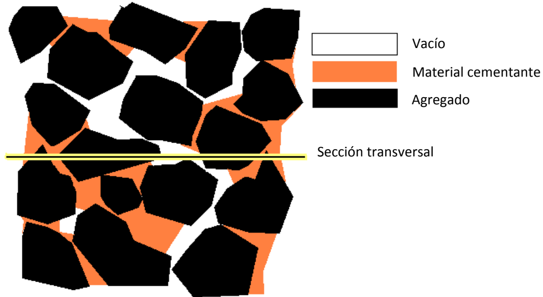
Figura 3.2 Estructura interna de un concreto permeable (Schaefer et al., 2006).
