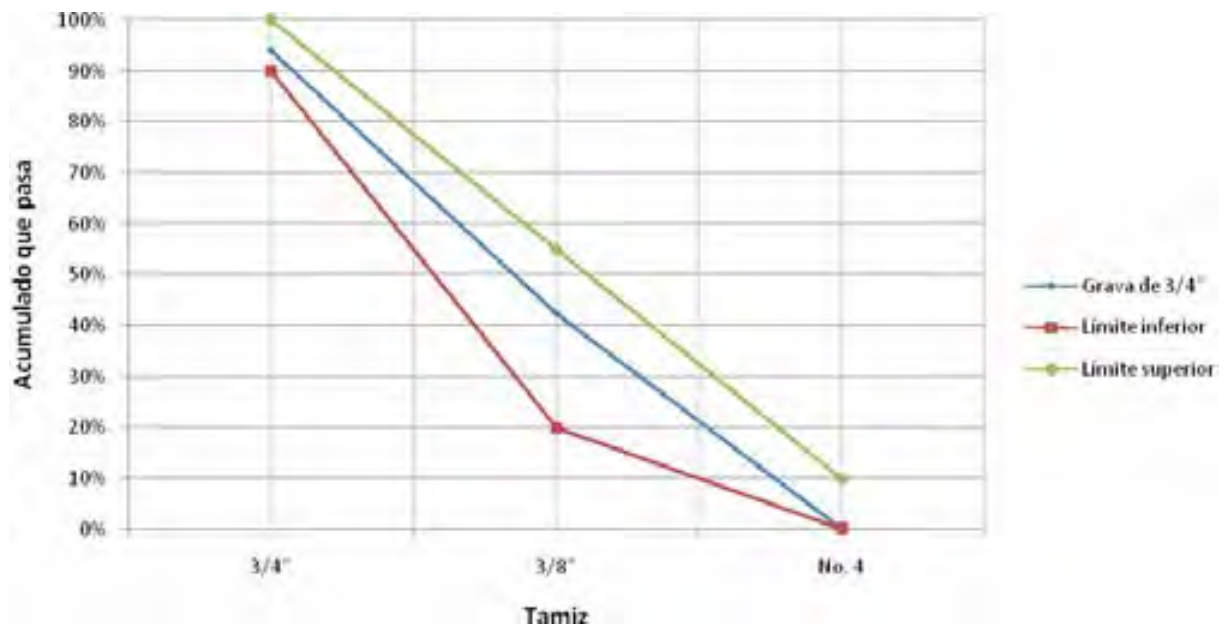
Figura 6.2 Distribución de la curva granulométrica del agregado de 3/4" de acuerdo a los límites superior e inferior de la norma ASTM C33.
