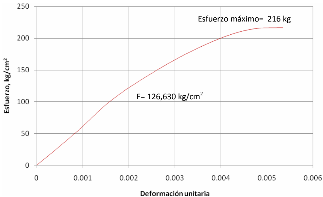
Figura 6.20 Curva de esfuerzo-deformación unitaria de la prueba de módulo de elasticidad de una probeta de concreto permeable de 3/8" y 15% de vacíos.
