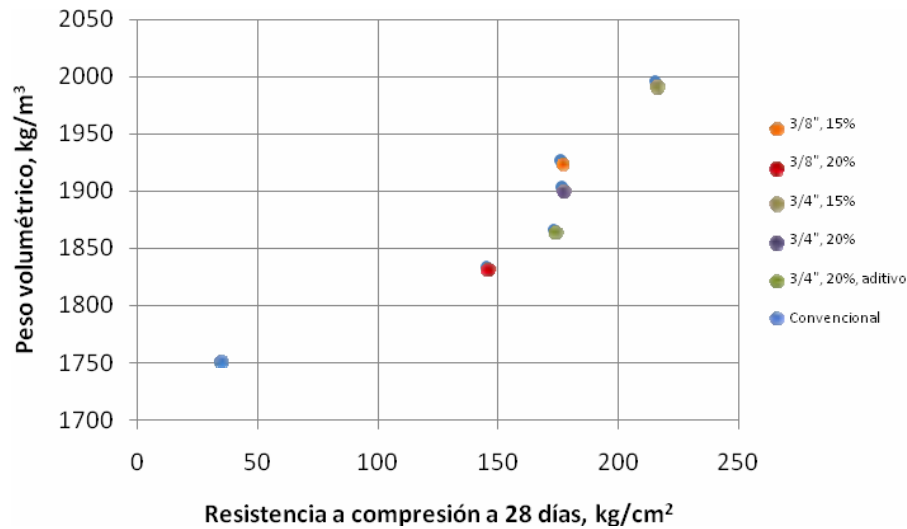
Figura 6.13 Relación entre el peso volumétrico y la resistencia a compresión a 28 días.
