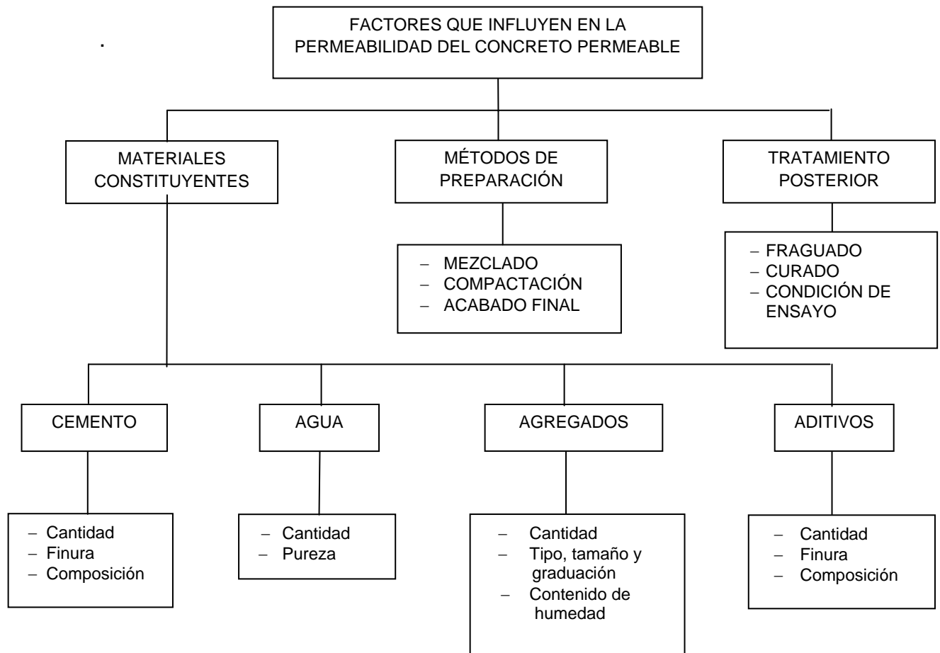
Figura 3.7 Factores que influyen en la permeabilidad del concreto
