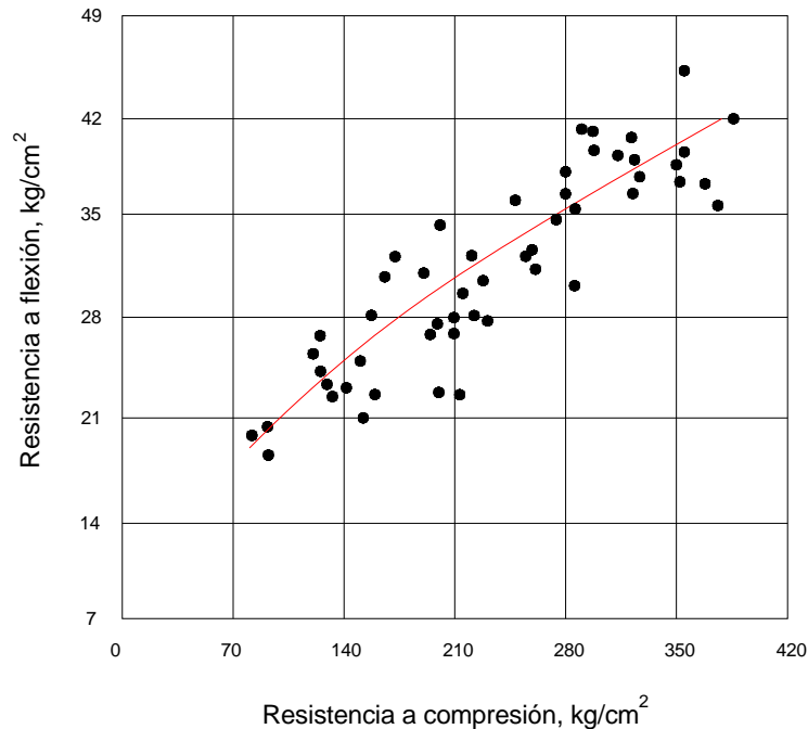
Figura 3.5 Relación entre la resistencia a flexión y la resistencia a compresión para el concreto permeable (Meininger, 1988).
