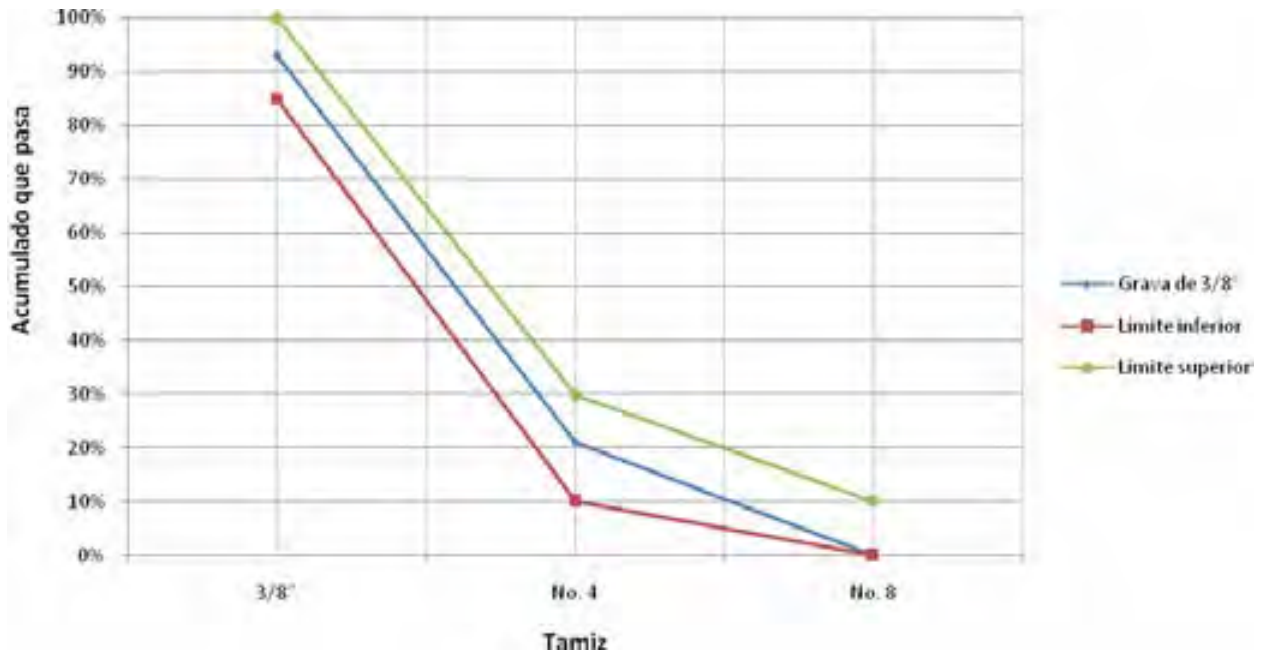
Figura 6.1 Distribución de la curva granulométrica del agregado de 3/8" de acuerdo a los límites superior e inferior de la norma ASTM C33.
