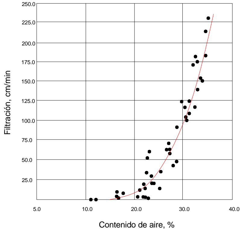
Figura 3.8 Relación entre la filtración y el contenido de aire para el concreto permeable. (Meininger, 1988).
