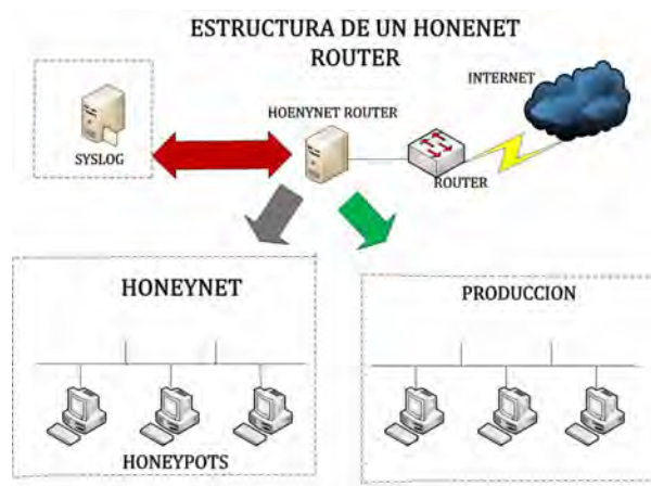
Figura 2.3: Arquitectura de Honeynet Router
