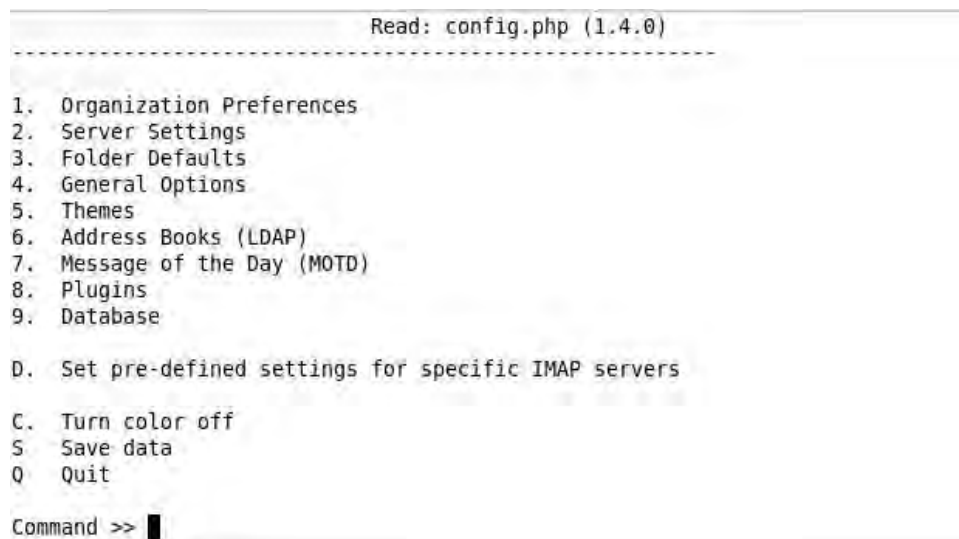
Figura 3.10: Interfaz de configuración de Squirrelmail
