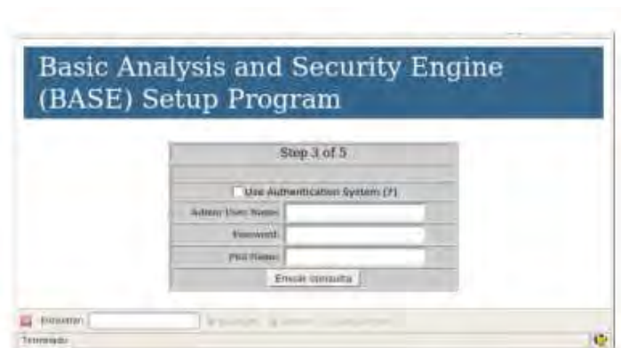
Figura 3.32: Instalación de BASE
