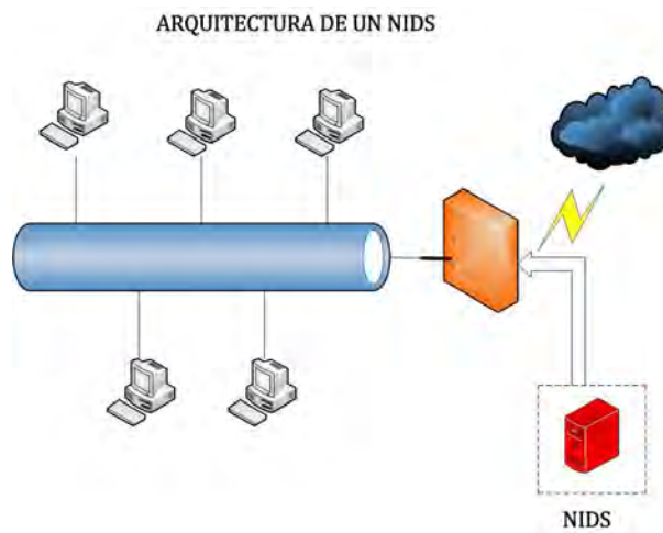
Figura 1.10: Arquitectura de un NIDS
