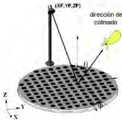
Figura 1. Antena de Arreglos de Fase Reflectivos.
