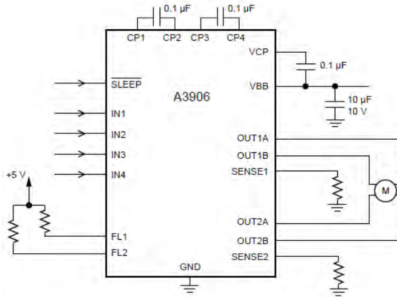
Figura 3.13 Etapa de potencia para cada minimotor.
