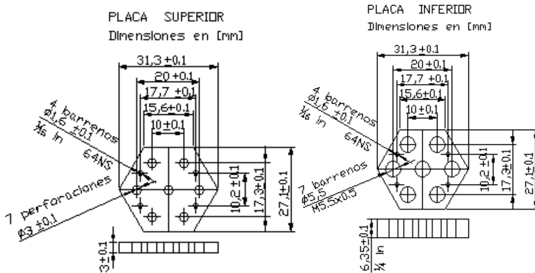
Fig. 1.4 Pantallas metálicas hexagonales.
