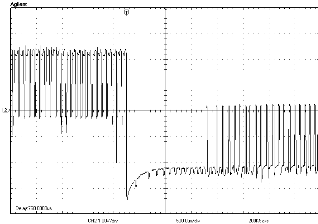
Figura 5.7. Acercamiento para visualizar la PWM.
