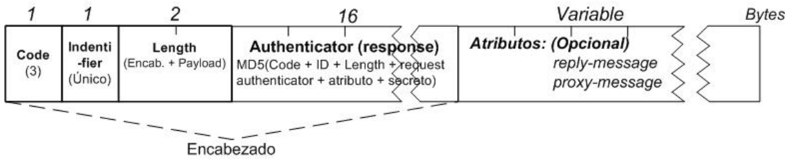
Figura 4.11. Un paquete típico Access-Reject
