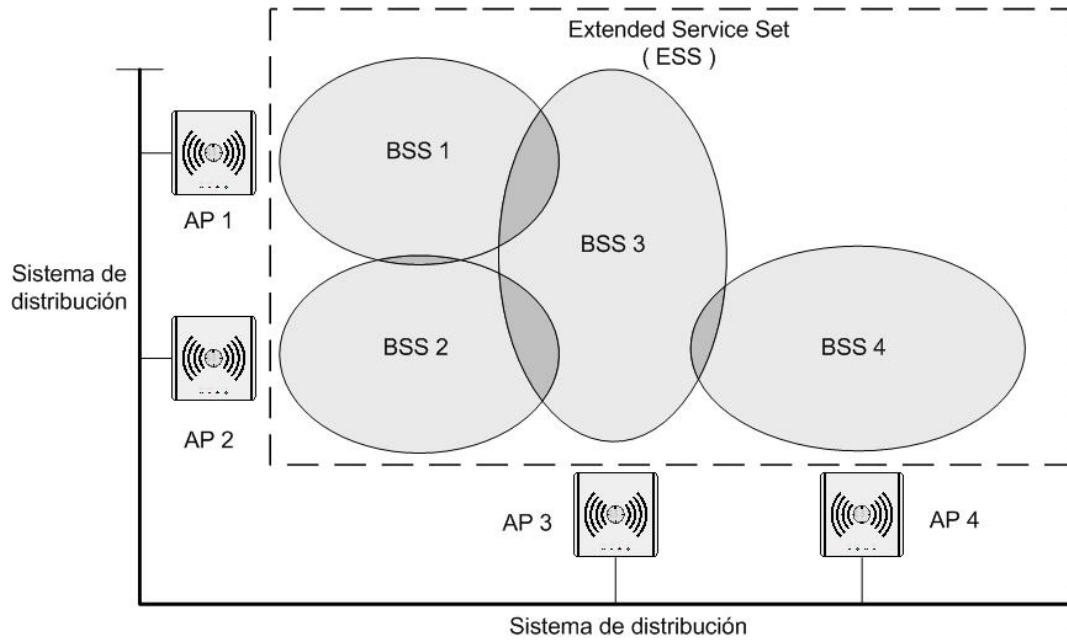
Figura 1.5. Modo infraestructura: ESS
