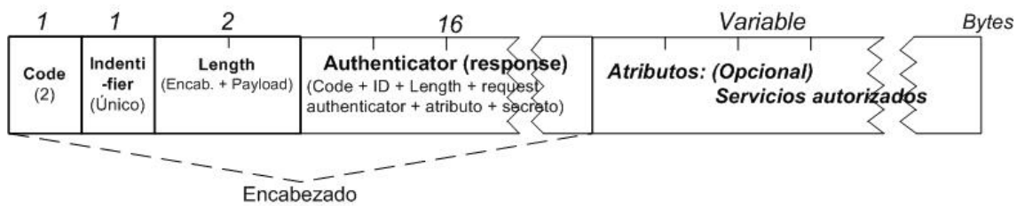
Figura 4.10. Un paquete típico Access-Accept
