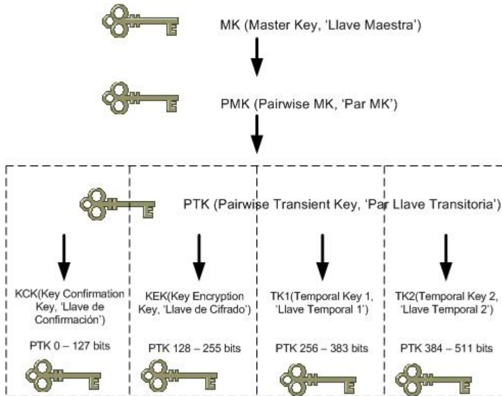
Figura 3.6. Jerarquía de llaves
