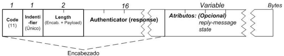
Figura 4.12. Un paquete típico Access- Challenge
