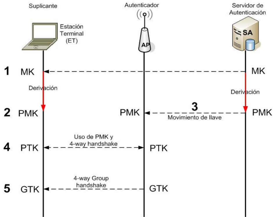
Figura 3.5. 802.11i: Administración y distribución de llaves
