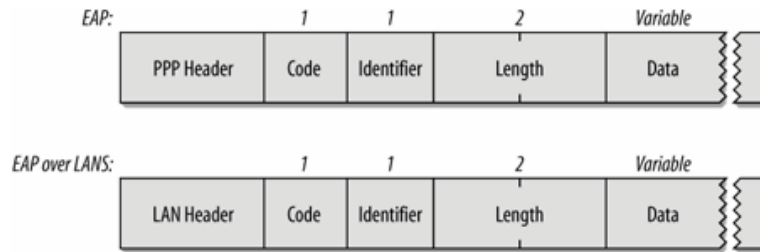
Figura 4.5. Formato de paquete EAP
