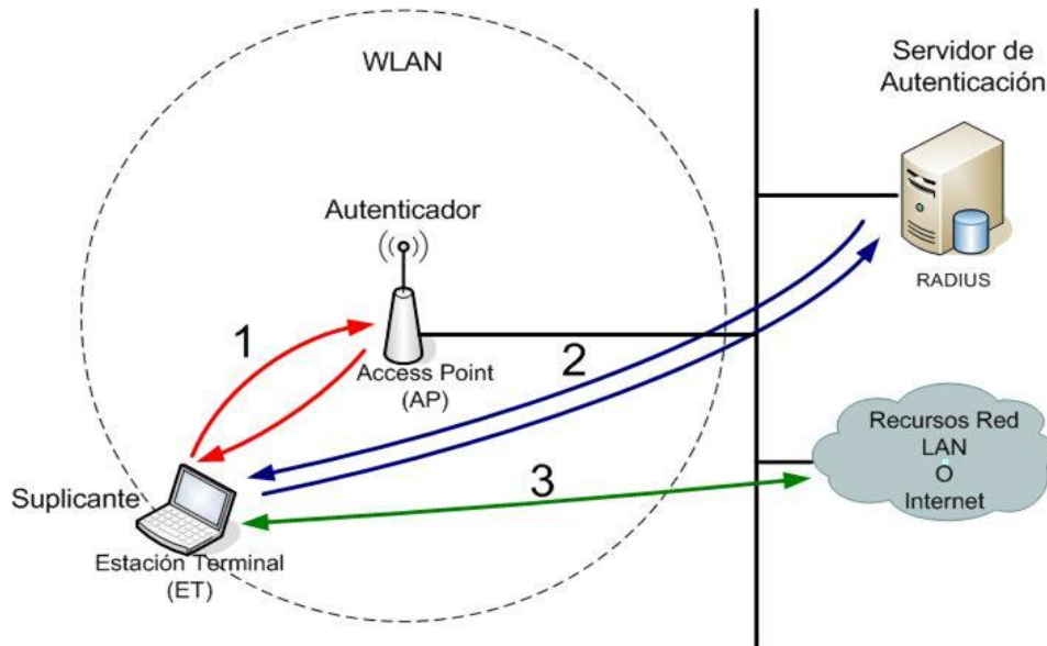
Figura 4.1. Control de acceso IEEE 802.1X
