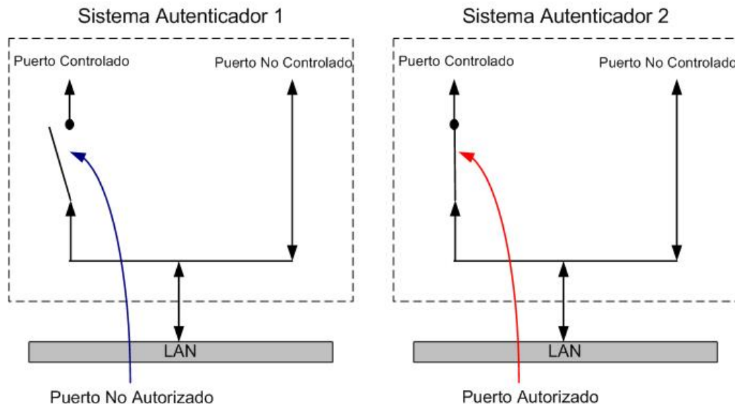
Figura 4.2. Estados de autorización del puerto controlado
