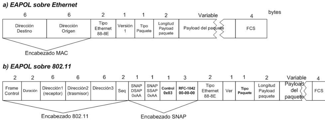
Figura 4.16. Formato de trama EAPOL
