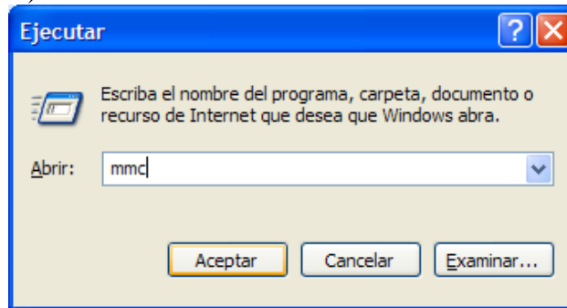
Figura C.11. Iniciando mmc
