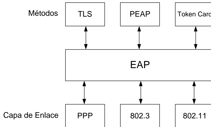
Figura 4.4. Arquitectura EAP
