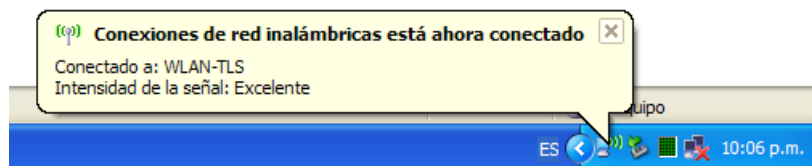
Figura 5.7. Conexión exitosa.
