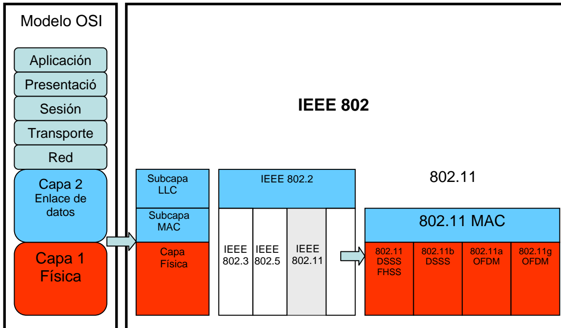
Figura 1.1. Comparación del estándar 802.11 con respecto al modelo OSI
