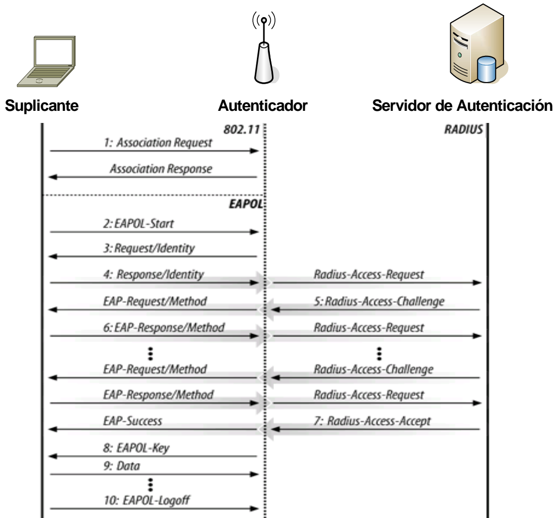
Figura 4.17. Intercambio 802.1X sobre 802.11
