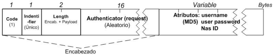
Figura 4.9. Un paquete típico Access-Request
