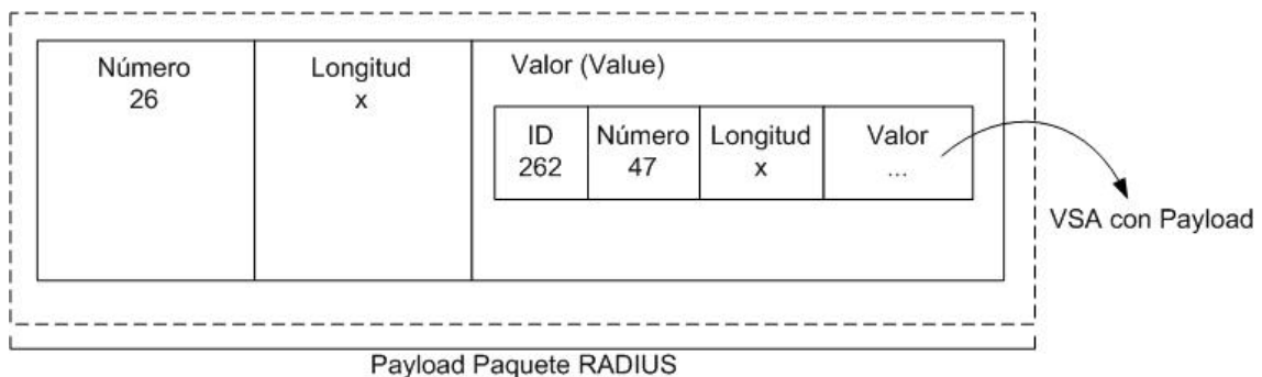
Figura 4.14. Encapsulado de un VSA dentro del atributo estándar 26
