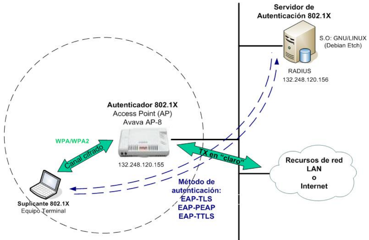
Figura 5.1. Escenario: implementación WPA/802.11i
