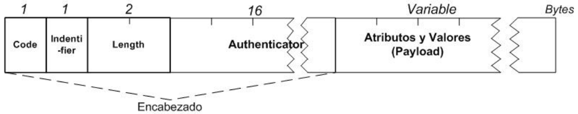
Figura 4.8. Estructura de un paquete de datos RADIUS
