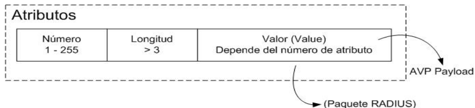
Figura 4.13. Formato estándar de los AVPs
