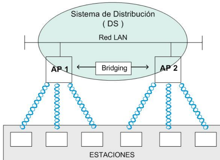
Figura 1.6. Sistema de distribución
