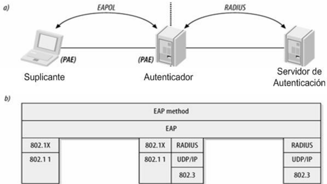
Figura 4.3. Arquitectura 802.1X
