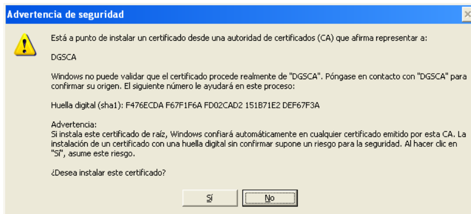
Figura C.6. Advertencia
