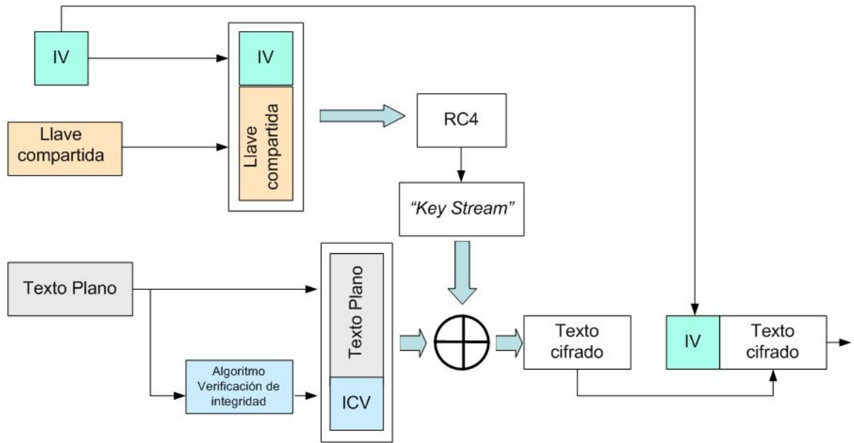
Figura 3.3. Cifrado WEP
