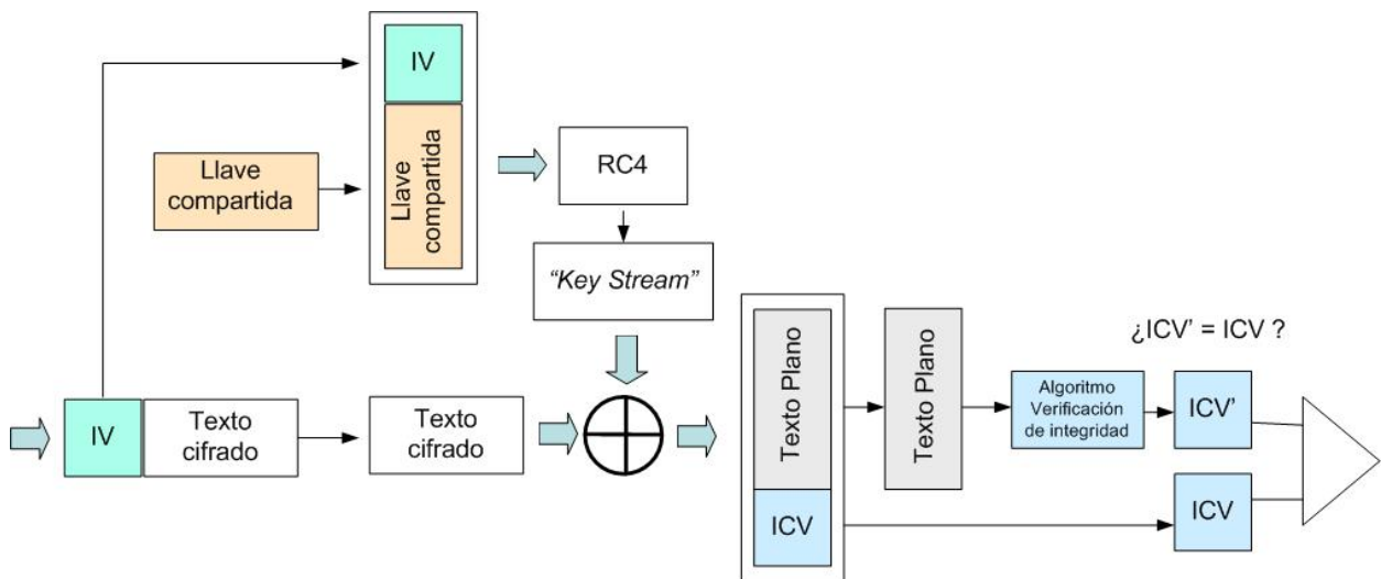
Figura 3.4. Descifrado WEP
