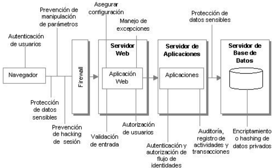
Figura 3-8. Protección a la Base de Datos
