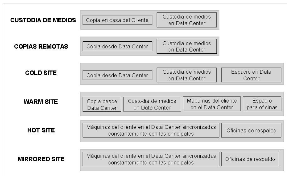
Figura 3-3. Opciones de Respaldo
