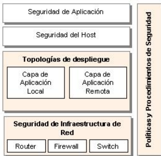
Figura 3-9. Consideraciones en la Capa de Aplicación
