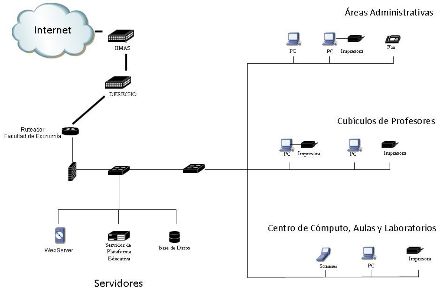
Figura 4-3. Propuesta de Segmentación de la red de la DEP-FE
