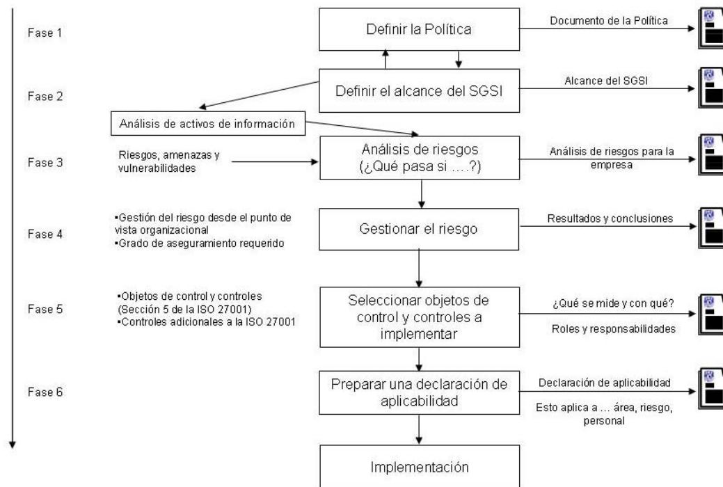
Figura 4-2. Metodología de Seguridad de la Información
