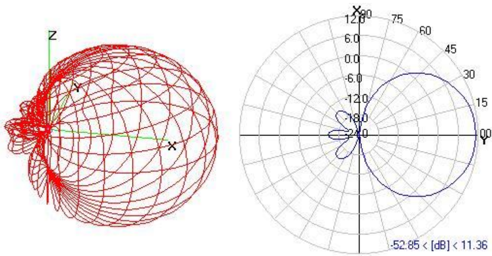
Figura 5-7 Radiación de una antena Direccional
