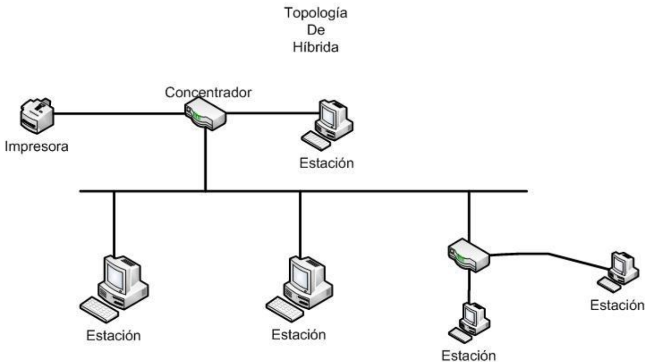
Figura 3-6: Topología Híbrida
