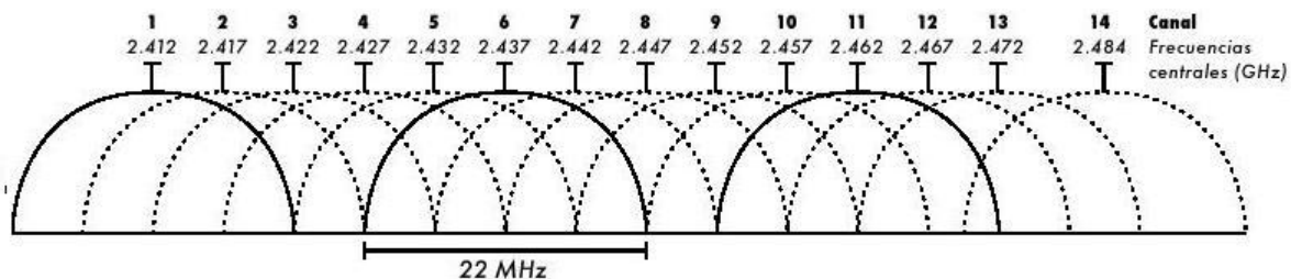
Figura 4-5 Solapamiento de canales
