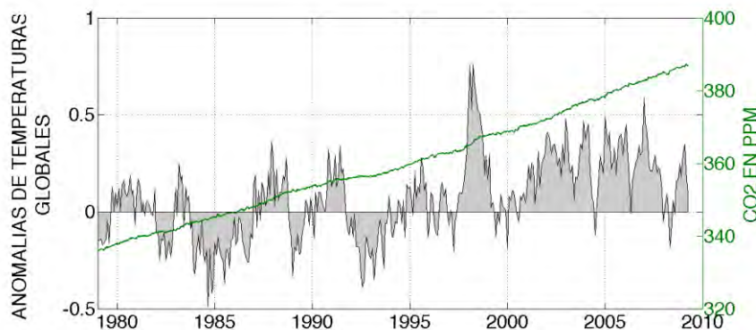
Figura 6.2. Anomalías en la temperatura global y concentración de \text{CO}_2 en partes por millón [63].
