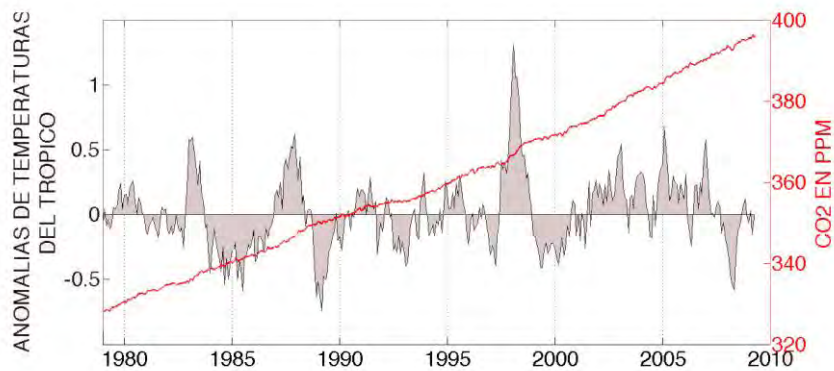
Figura 6.1. Anomalías en la temperatura del Trópico y concentración de \text{CO}_2 en partes por millón [63].
