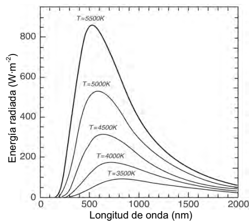
Figura 3.1. Espectros de radiación de cuerpo negro a diferentes temperaturas [31].
