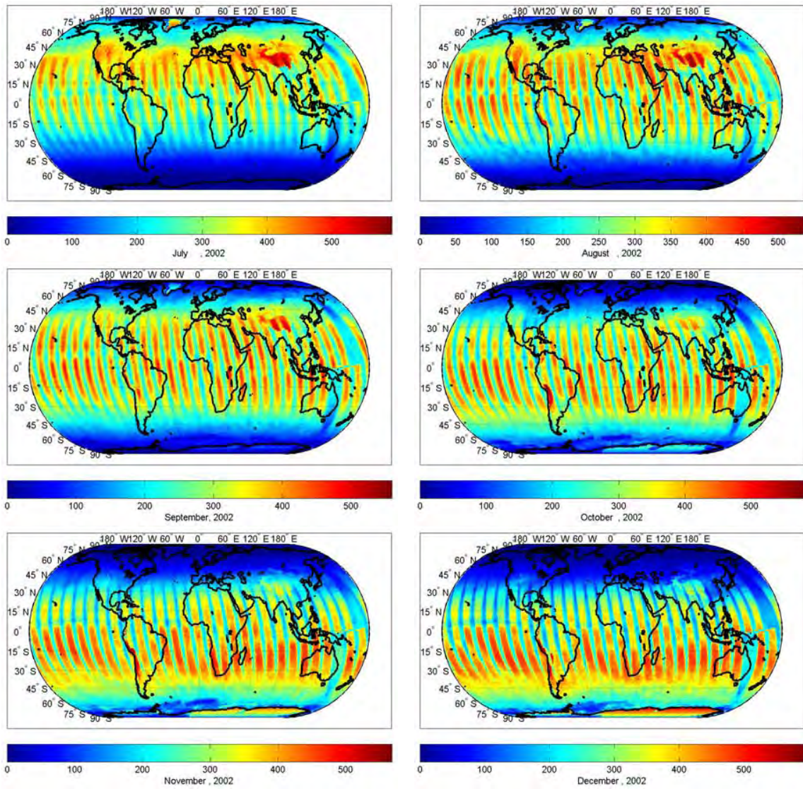
Figura 7.6. Mapas de distribución de la irradiancia espectral en superficie para \lambda=324 \text{ nm} . Periodo de julio a diciembre de 2000 (unidades: \text{mWm}^{-2}\text{nm}^{-1} ).
