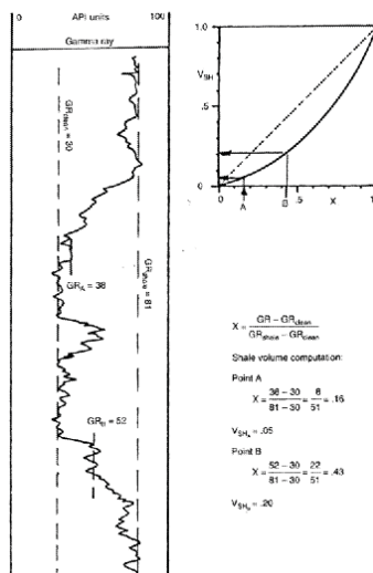
Figura 61. Técnica para determinar el volumen de arcilla a partir del rayos gamma
