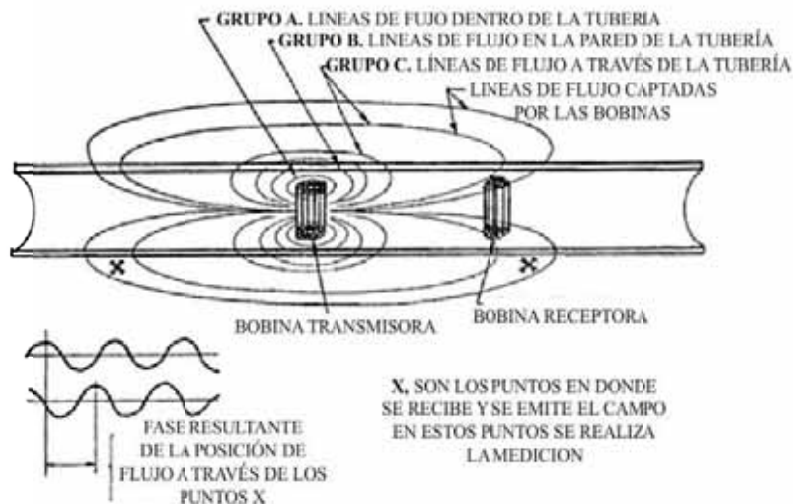
Figura 34. Esquema de la herramienta de inspección de la tubería de revestimiento de dispositivo de cambio de fase electromagnético. Modificado de "Cased Hole and Production Log Evaluation", J. Smolen, 1998
