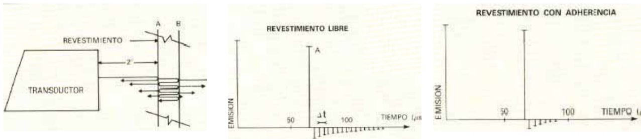
Figura 53. Modelo de reflexiones de la señal ultrasónica. Tomado de "Evaluación de Formaciones México", Schlumberger, 1994.
