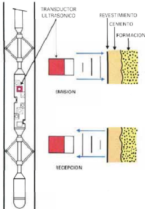
Figura 52. Esquema de a herramienta CET. Tomado de "Evaluación de Formaciones México", Schlumberger, 1994.
