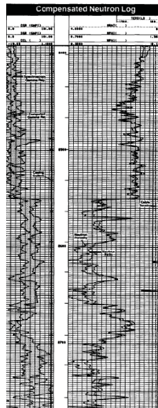
Figura 76. Registro de neutrón compensado
