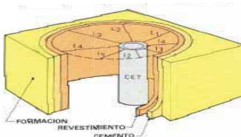
Figura 57. Configuración de calibres acústicos. Tomado de "Evaluación de Formaciones México", Schlumberger, 1994.
