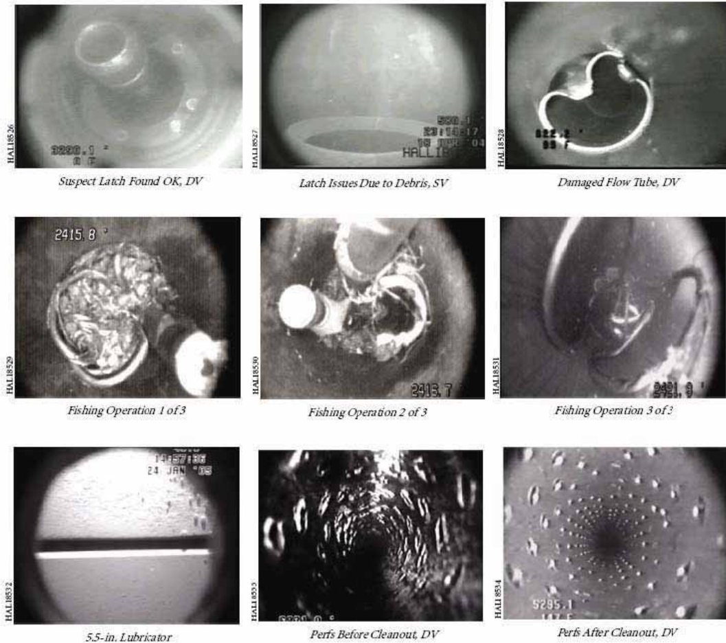
Figura 39. Ejemplos de las distintas aplicaciones de la cámara en pozo, se muestran las distintas operaciones y algunos daños detectados en la tubería de revestimiento. Tomado de EyeDeal™, Halliburton brochure, 2004
