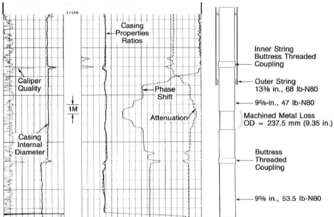
Figura 35. Registro de la herramienta de espesor electromagnético de multifrecuencia. La configuración mecánica del pozo es mostrado de lado derecho de la figura. (Tomado de "Cased Hole Log Interpretation", Schlumberger, 1999)
