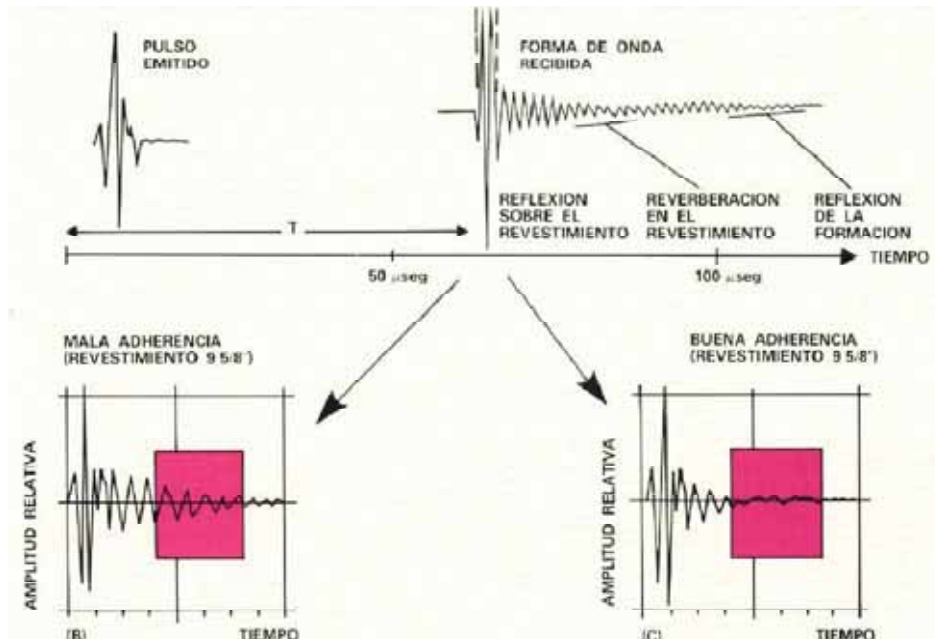
Figura 51. Principio de medición de la herramienta CET. Tomado de "Evaluación de Formaciones México", Schlumberger, 1994.
