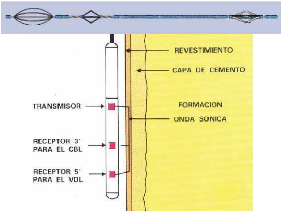
Figura 43. a) Control de la cementación con la herramienta sónica compensada b) Esquema de la herramienta memory slim CBL tool. Tomado de CBL Tool, Brochure of Schlumberger, 2004
