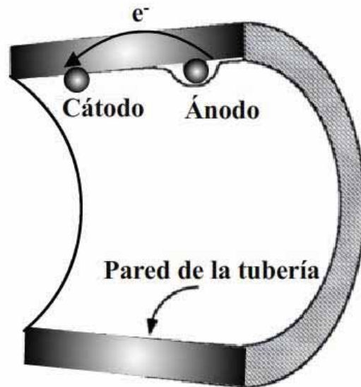
Figura 26. Corrosión electroquímica en la tubería de revestimiento. Modificada de "Degradation during offshore drilling operations, NDE Technology, Inc. 2000"
