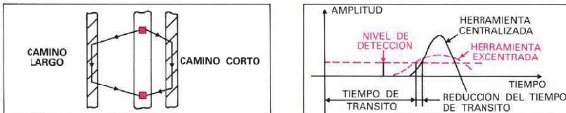
Figura 45. Efecto de excentricación de la herramienta sobre la medición de la amplitud. Tomado de "Evaluación de Formaciones México", Schlumberger, 1994.
