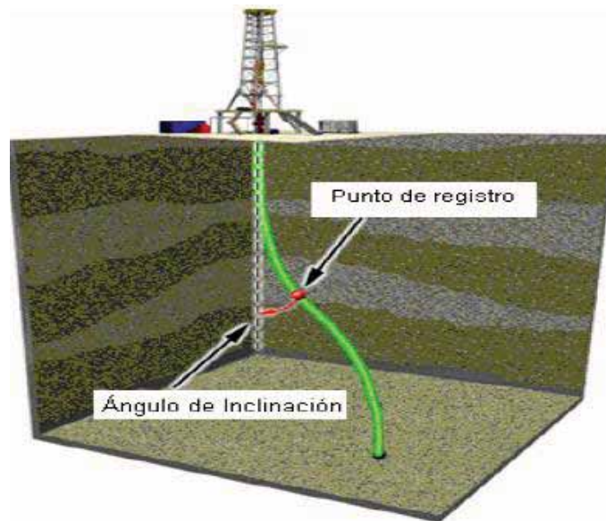
Figura III.2. Ángulo de inclinación. (Chagoya, 2007)
