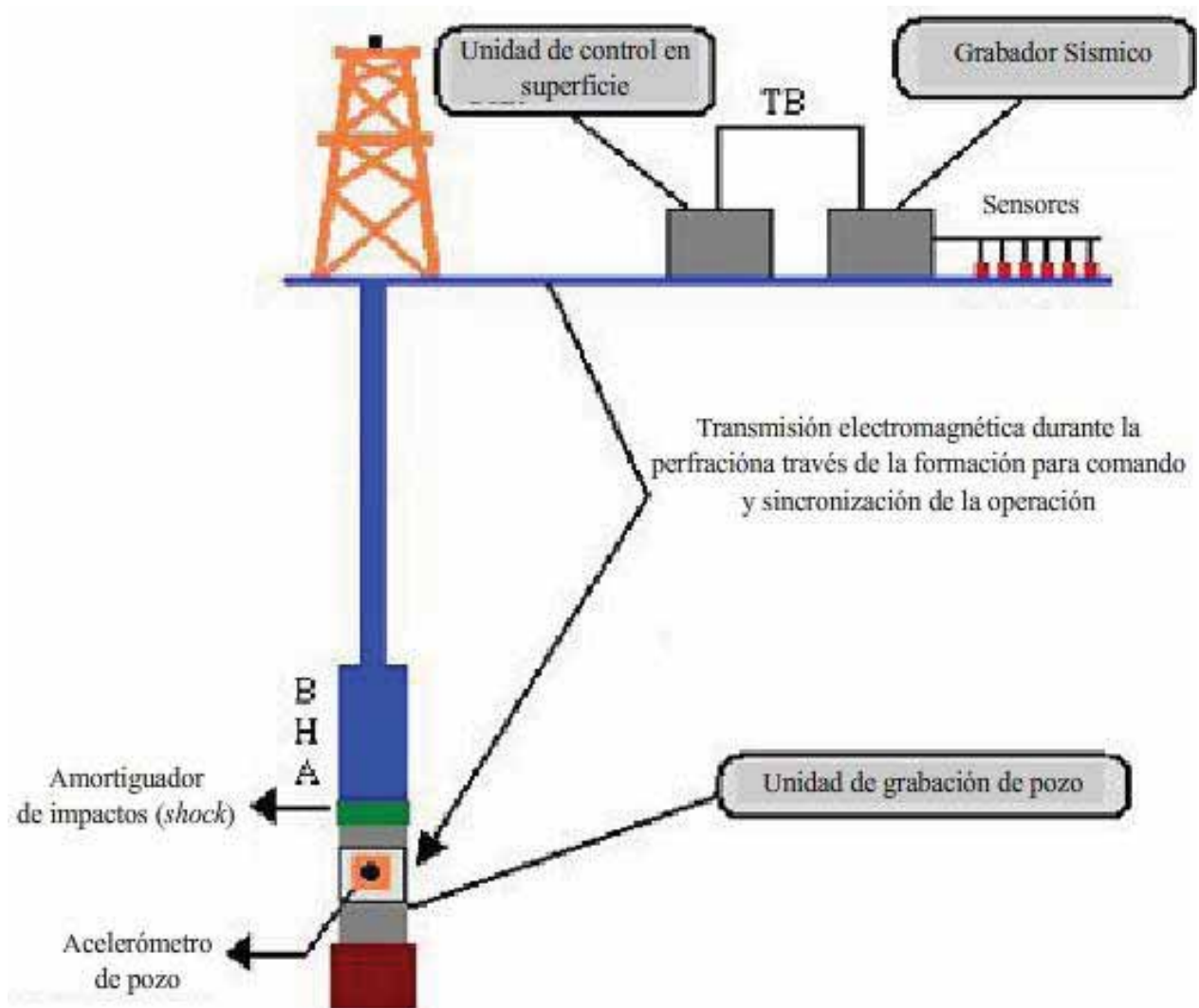
Figura II.6. Muestra de un registro EM-SWD con la barrena. (Anchlya, A., 2006)
