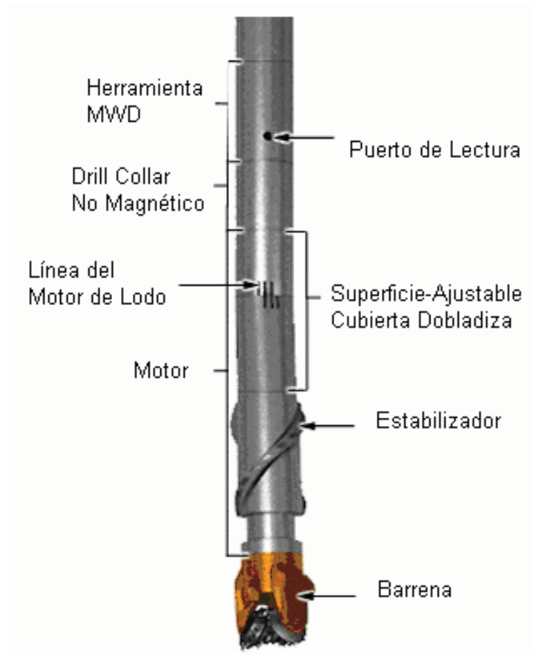
Figura III.3. Cara de la Herramienta. (Chagoya, 2007)
