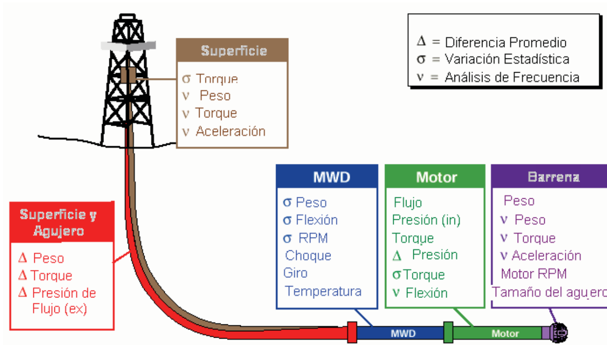
Figura III.20. Puntos de Medición. (Chagoya, 2007)
