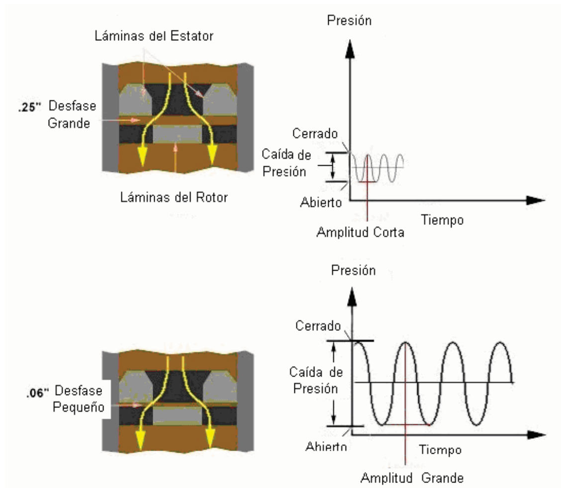
Figura III.14. Generación de caídas de presión en el lodo. (Chagoya, 2007)
