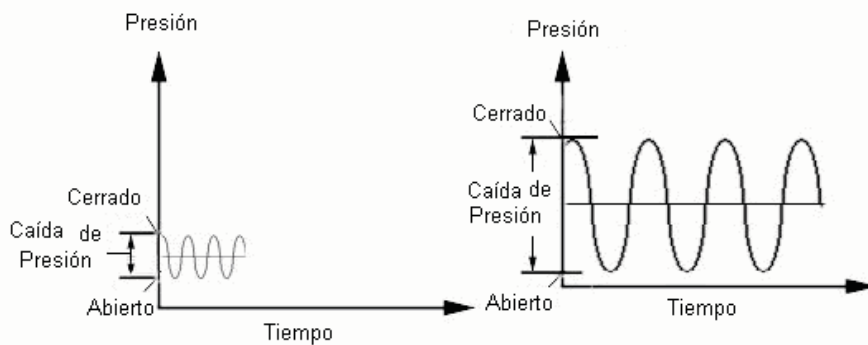
Figura III.13. Fuerza (amplitud) de la señal de pulsos de presión en el lodo. (Chagoya, 2007)
