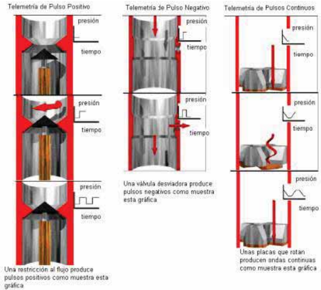
Figura III.12. Tipos de telemetría. (Chagoya, 2007)
