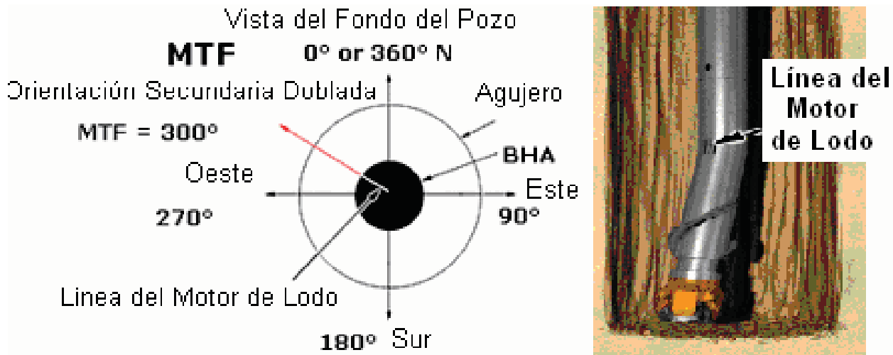
Figura III.4. a) Cara Magnética de la Herramienta. b) Inclinación. (Chagoya, 2007)
