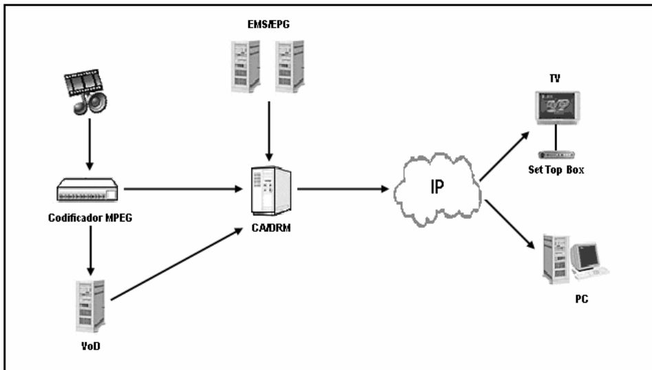
Fig. 3.3.1-1 Arquitectura de IPTV
