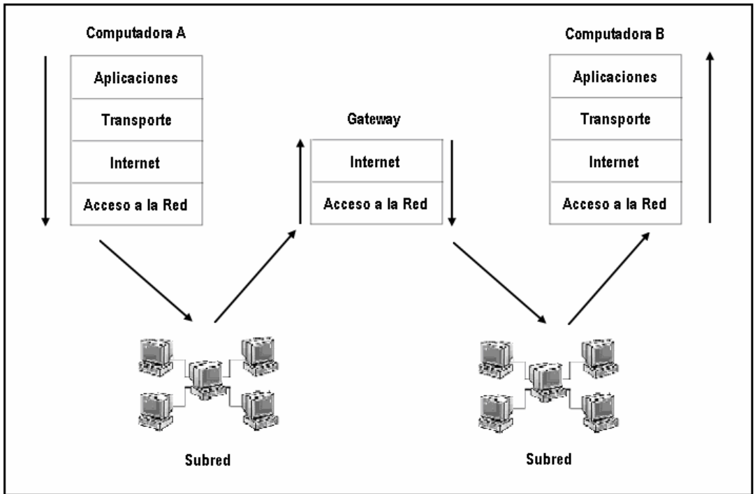
Fig. 1.4.1-2 Topología de la familia TCP/IP
