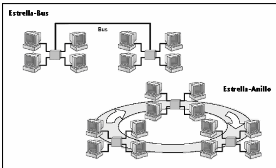
Fig. A.2.2-4 Redes Híbridas
