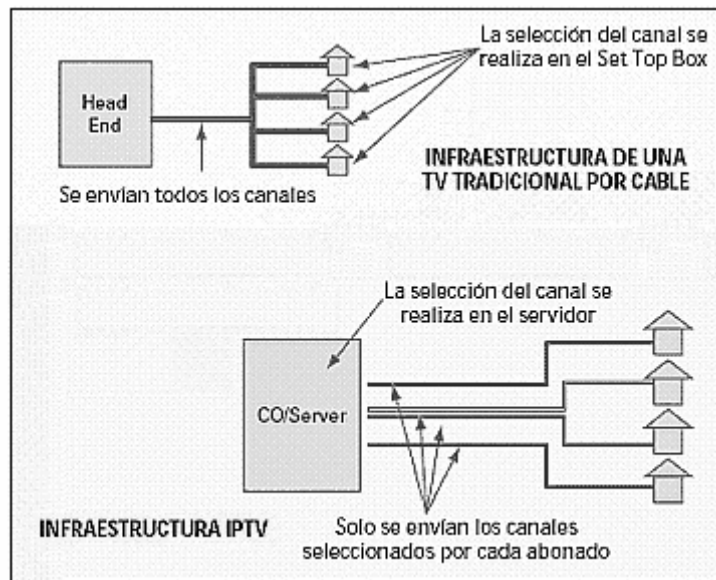
Fig. 2.2.2-1 Infraestructura de IPTV vs Infraestructura de TV tradicional
