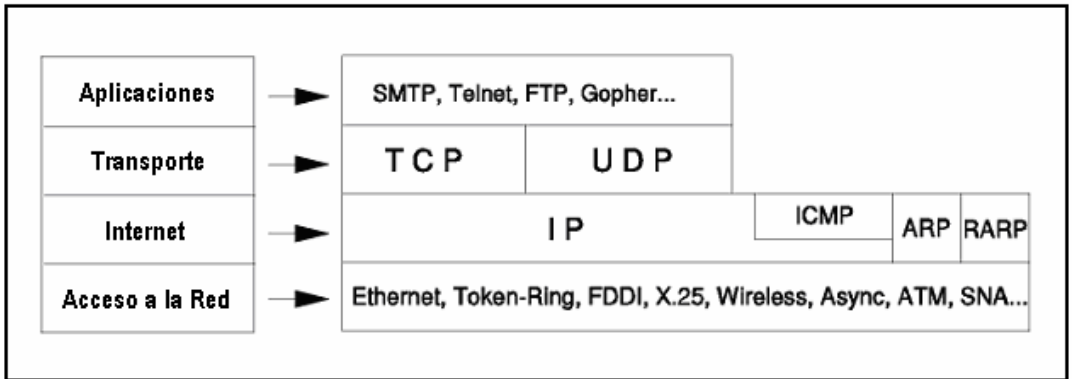
Fig. 1.4.1-1 Arquitectura TCP/IP
