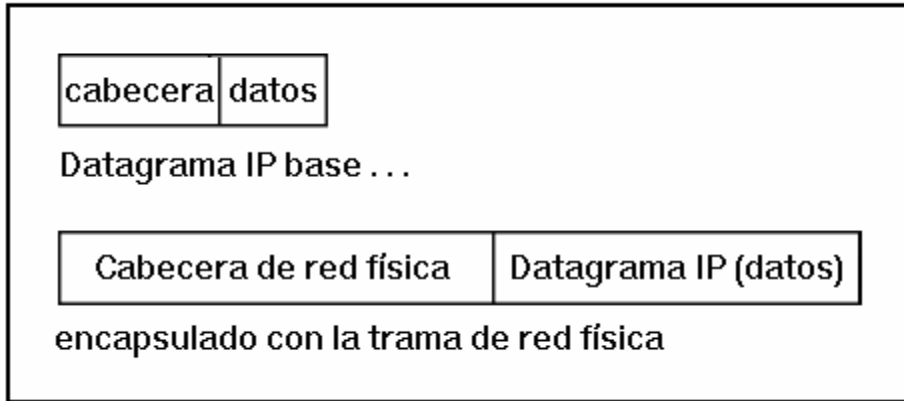
Fig. 1.4.1-3 Datagrama IP
