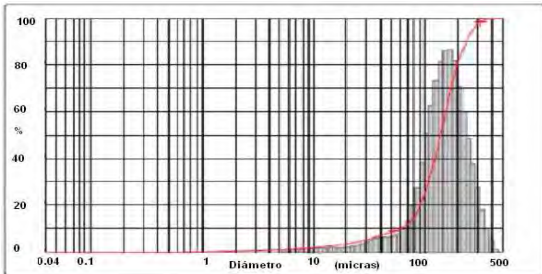
Figura 3.4 Los datos están representados en un gráfico de frecuencia vs diámetro en forma de histograma y curva acumulativa (en rojo).
