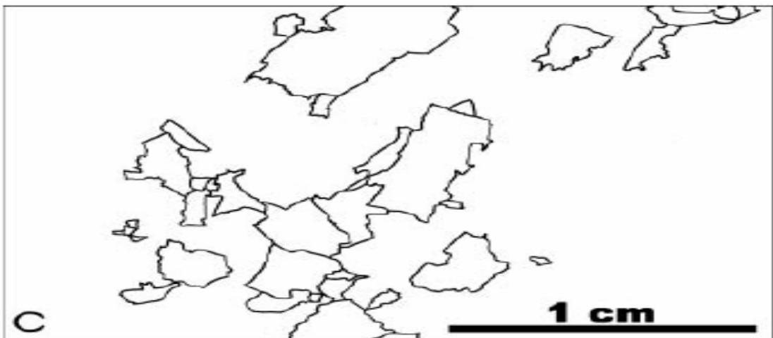
Figura 3.13 Imagen de una tonalita observada mediante microscopía de polarización; nicoles cruzados (a) y nicoles paralelos (b); esquema en el que aparecen solamente los cristales de biotita cuyo tamaño medio de grano se va a estimar(c).
