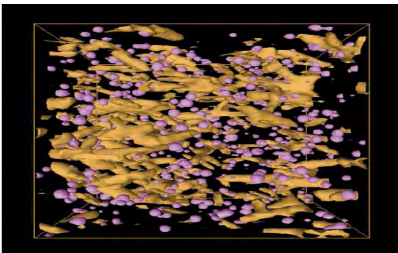
Figura 4.4 Se muestra una iso-superficie de granate y estuarolita en un esquistos de las Montañas Picuris, Nuevo México.
