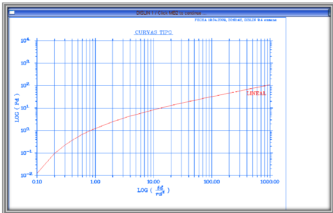
Figura 4.5. Curva tipo para Flujo lineal
