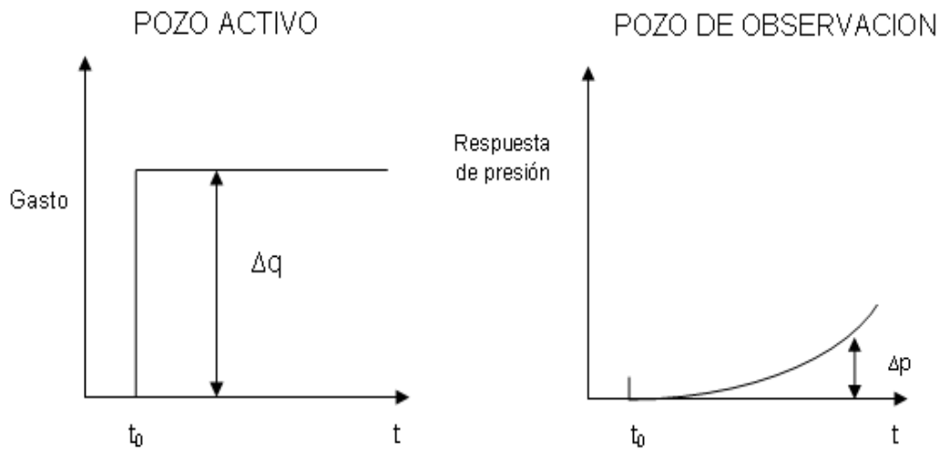
Figura 1.2. Prueba de Interferencia de Presión.
