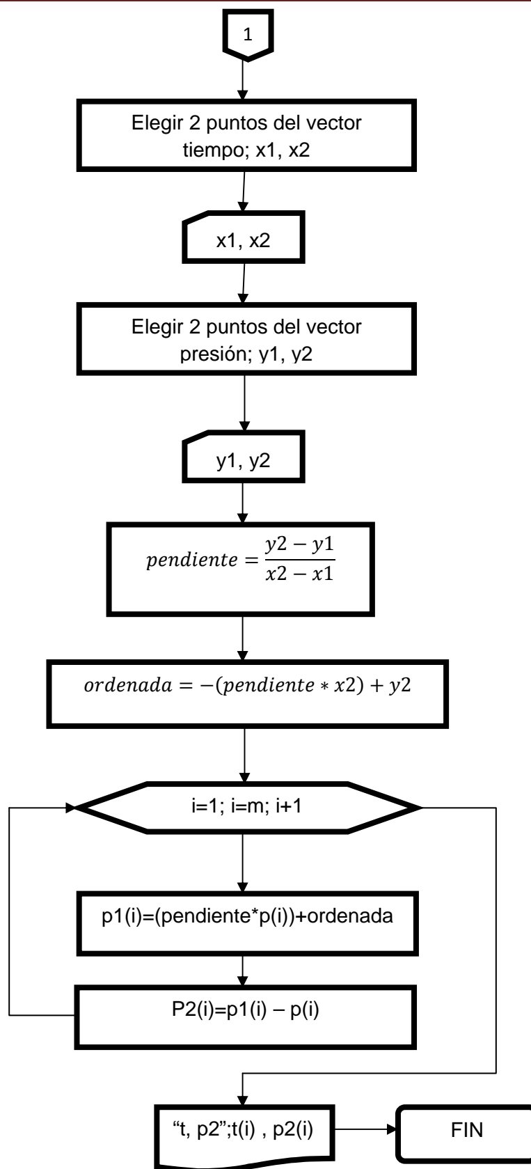
Figura 4.3. Diagrama de flujo para corrección de datos por Tendencia Lineal
