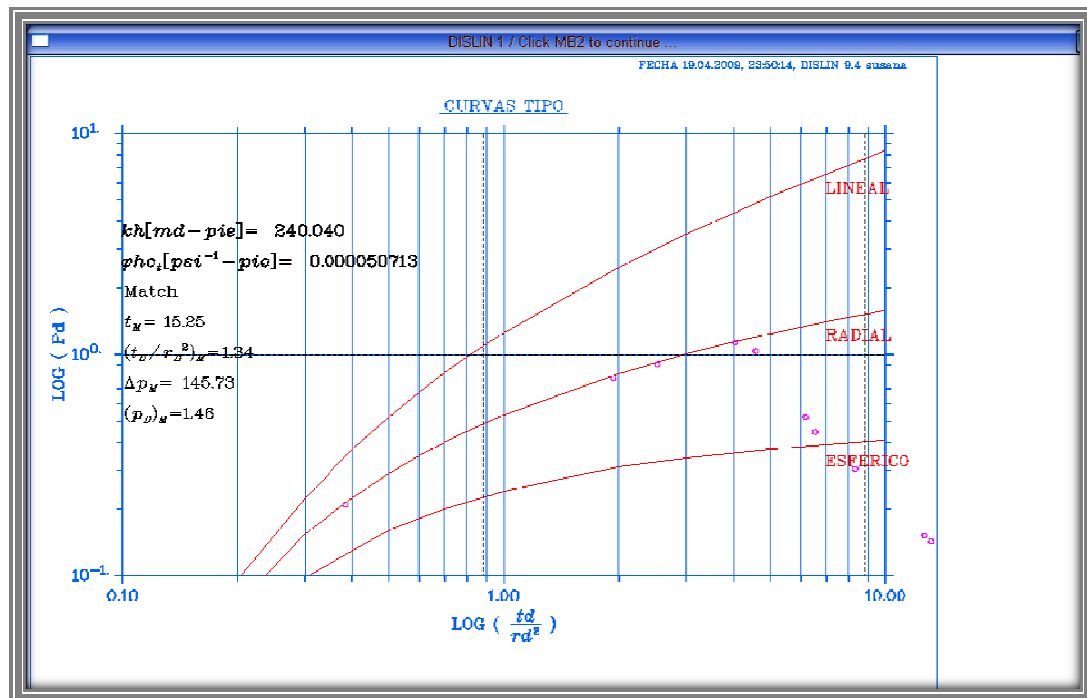
Figura 5.1. Solución al ejercicio 1 mediante el análisis de curvas tipo
