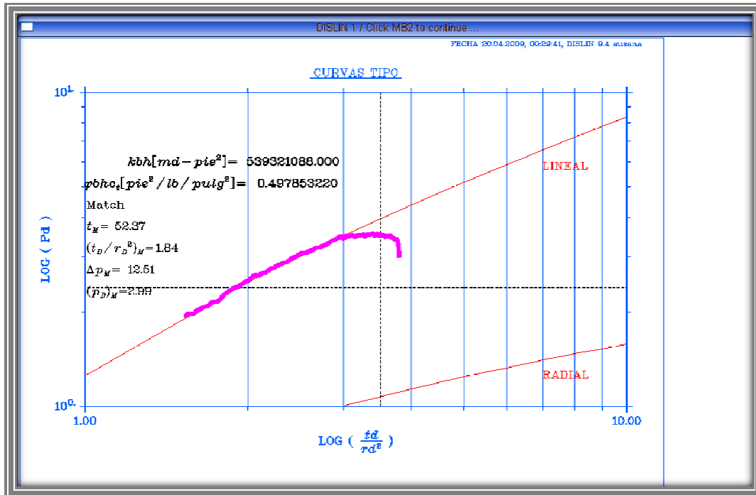
Figura 5.5. Datos corregidos por tendencia, aplicando T_0 y ajustados a la curva tipo de flujo lineal
