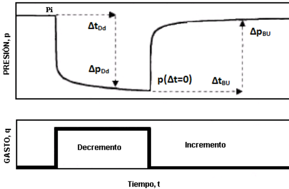
Figura 1.1. Secuencia de pruebas de Decremento e Incremento [1]
