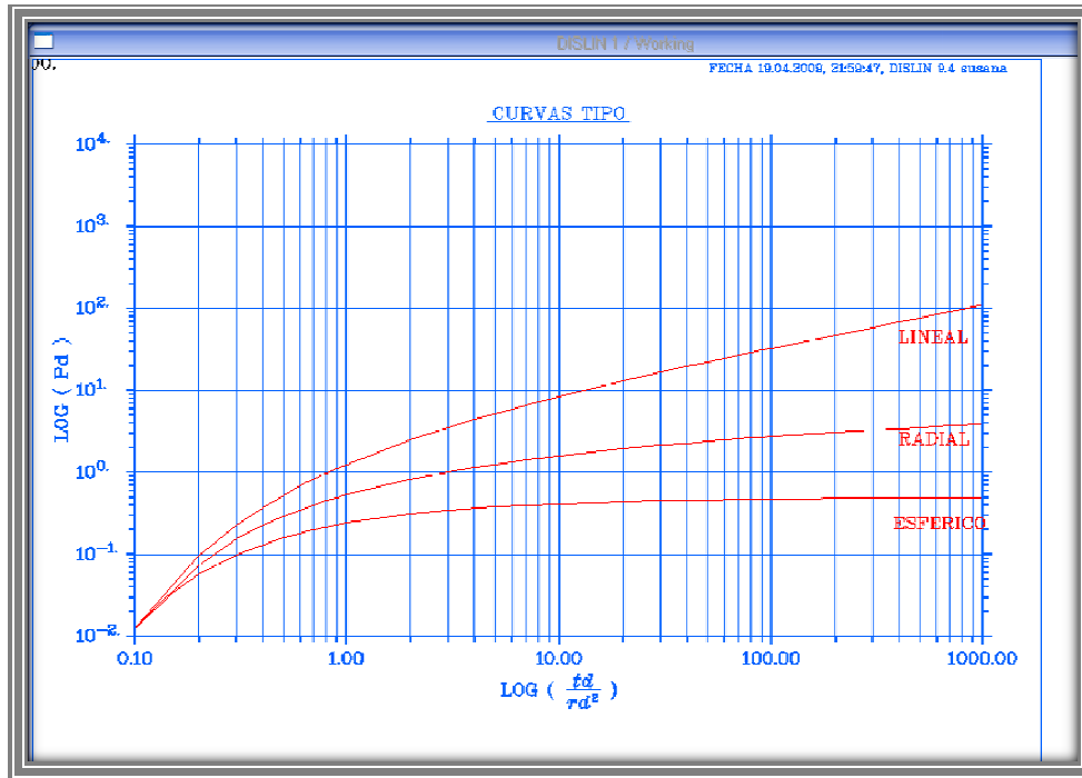
Figura 4.17. Vista de curvas tipo (flujo radial, lineal y esférico).
