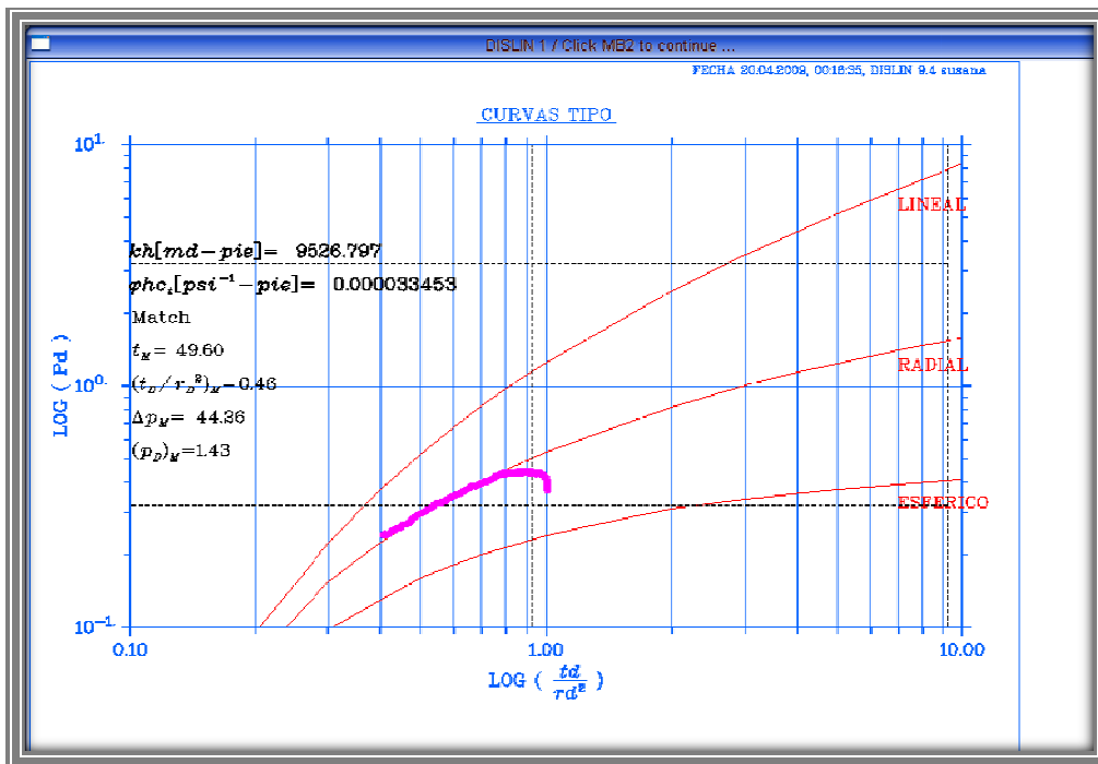
Figura 5.4. Datos corregidos por tendencia, aplicando T_0 y ajustados a una curva tipo
