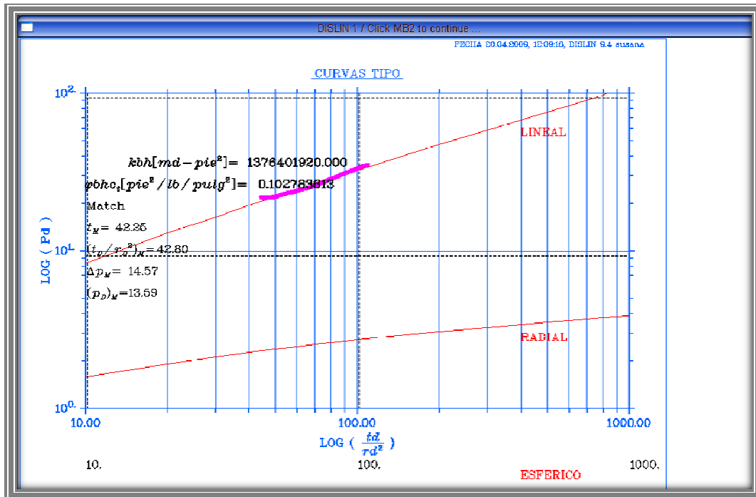
Figura 5.9. Datos corregidos por tendencia, aplicando T_0 y ajustados a la curva tipo de flujo lineal
