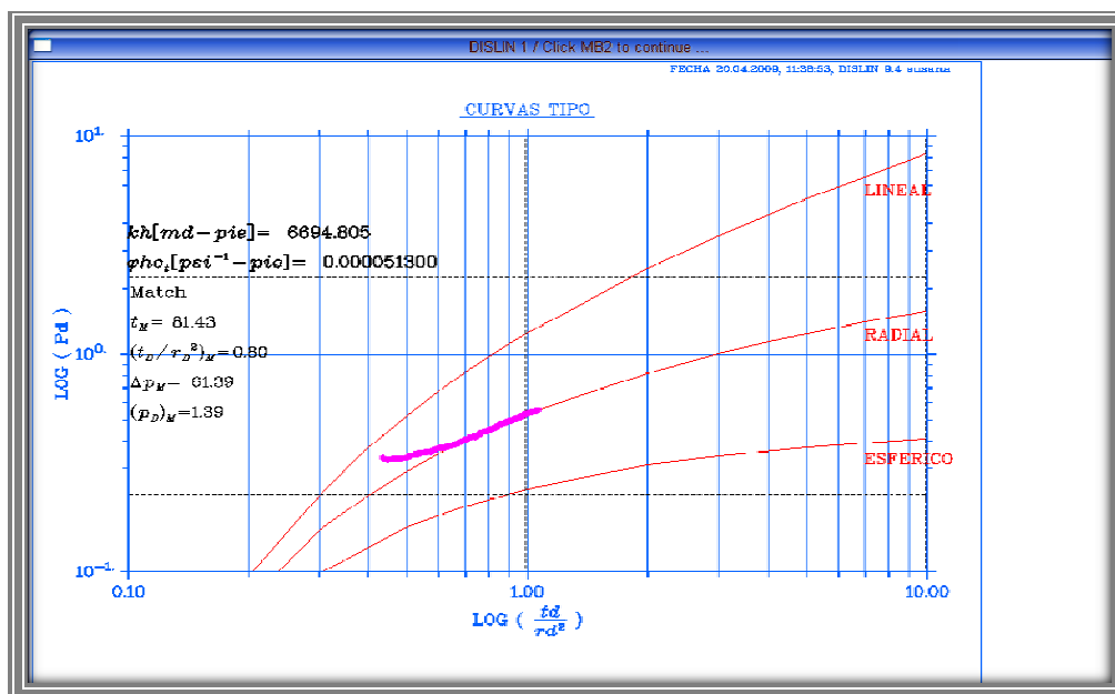
Figura 5.9. Datos corregidos y ajustados a una curva tipo
