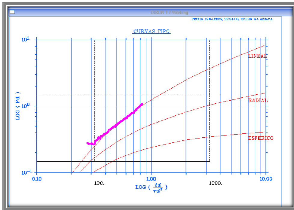
Figura 4.20. Acercamiento de los datos ya ajustados
