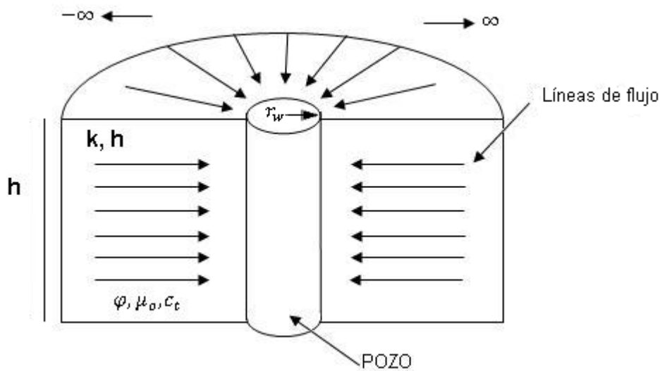
Figura 3.4. Flujo radial hacia un pozo en un yacimiento infinito.
