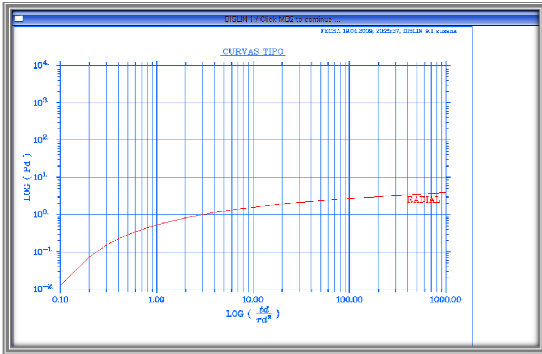
Figura 4.6. Curva Tipo de Flujo Radial
