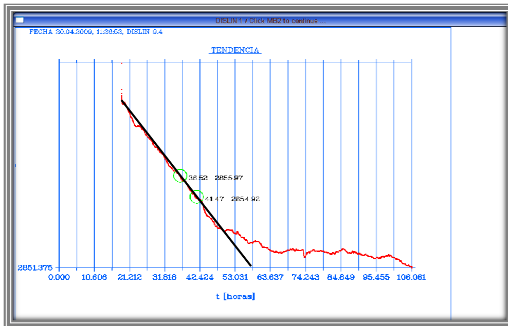
Figura 5.8. Datos corregidos con el método de “Tendencia Lineal”
