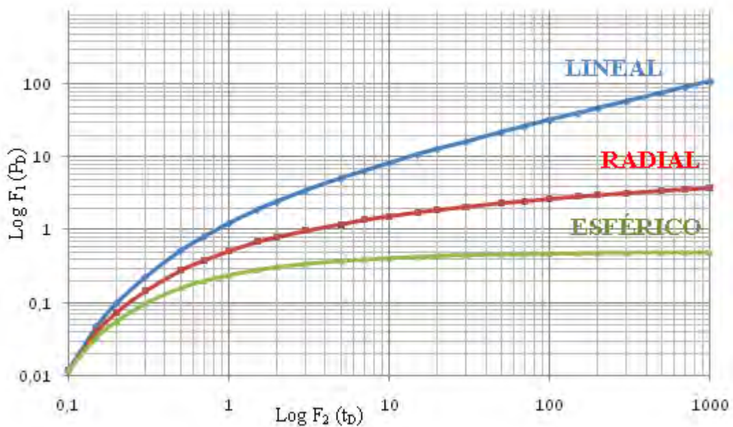
Fig. 3.6. Curvas Tipo: Flujo lineal, radial y esférico
