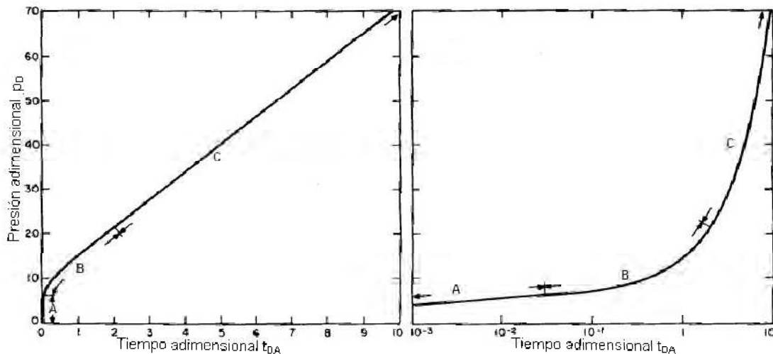
Figura 3.1. Régimen de flujo transitorio: A- Transitorio; B- Transición; C- Pseudo estacionario. Datos de Earlougher y Ramey para un rectángulo 4:1 con un pozo en x/L=0.75 , y/W=0.5 .
