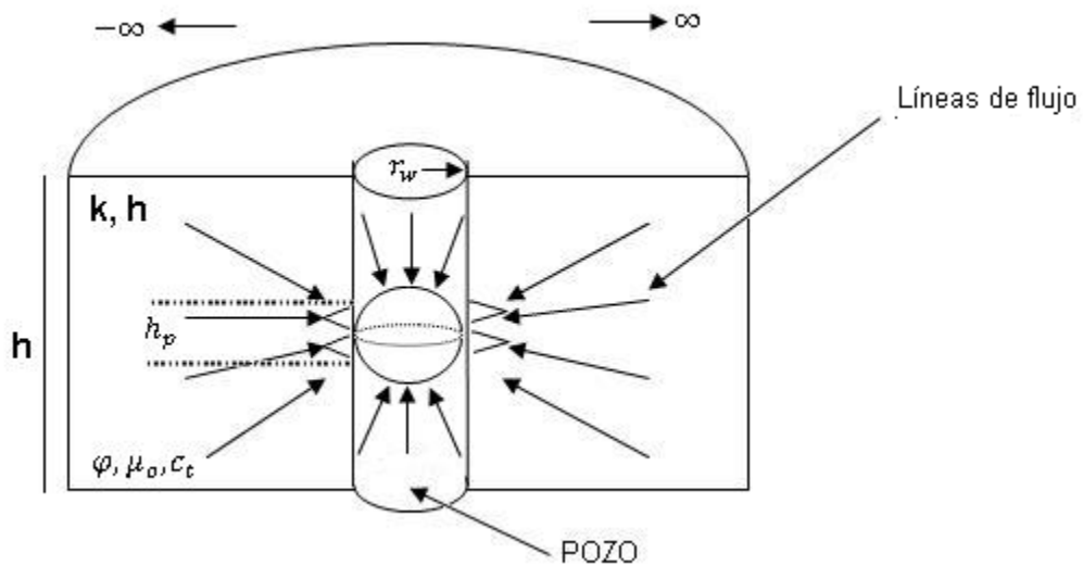
Figura 3.5. Flujo esférico hacia un pozo
