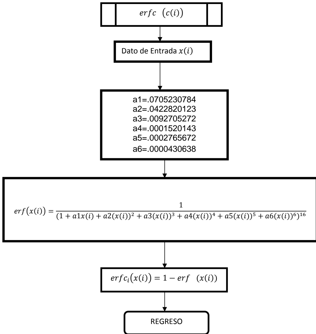
Figura 4.7. Diagrama de flujo para curva tipo de Flujo esférico
