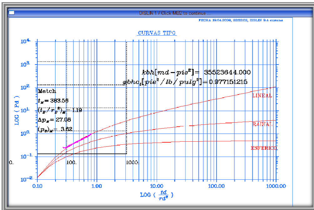
Figura 4.21. Obtención de parámetros en grafica sin acercamiento.
