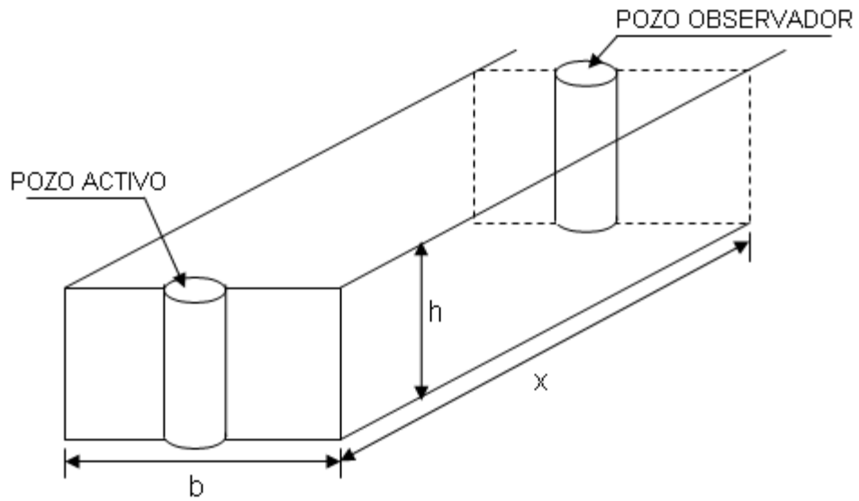
Figura 3.2. Yacimiento Lineal Semiinfinito
