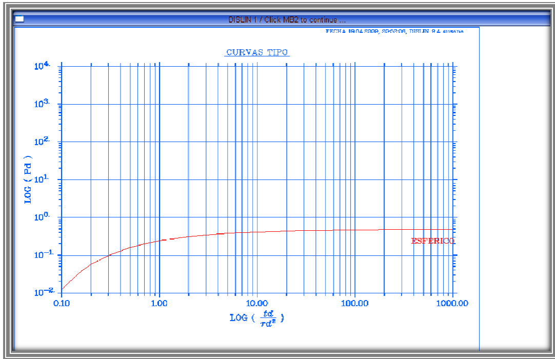
Figura 4.8. Curva tipo de Flujo esférico
