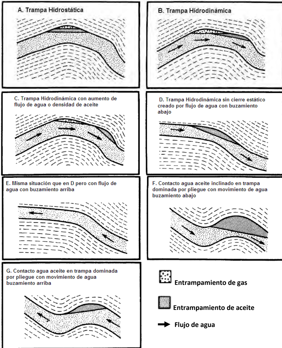
Figura 2.9. Ilustración del efecto cualitativo de la cantidad y dirección del flujo de agua y densidad del aceite en la configuración de una trampa de hidrocarburos. (A) Trampa hidrostática generalizada. (B) Trampa hidrodinámica generalizada. (C) Trampa Hidrodinámica con incremento del flujo de agua o la densidad del aceite. (D) trampa hidrodinámica sin cierre estático creado por el flujo de agua con buzamiento abajo. (E) Misma situación que en D pero con buzamiento arriba. (F) Contacto agua aceite inclinada en trampa dominada por pliegue con movimiento de agua buzamiento abajo. (G) Contacto agua aceite en una trampa dominada por pliegue con movimiento de agua buzamiento arriba [7] .
