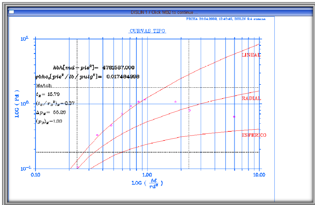
Figura 5.10. Datos ajustados a una geometría de flujo lineal
