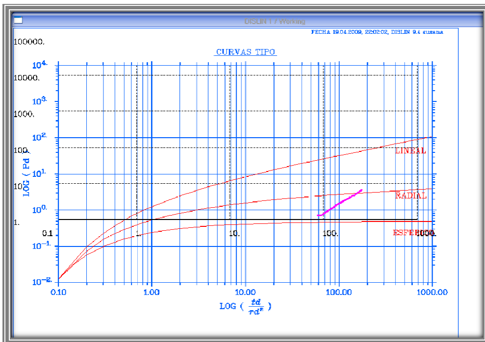
Figura 4.18. Datos de la prueba (color magenta)
