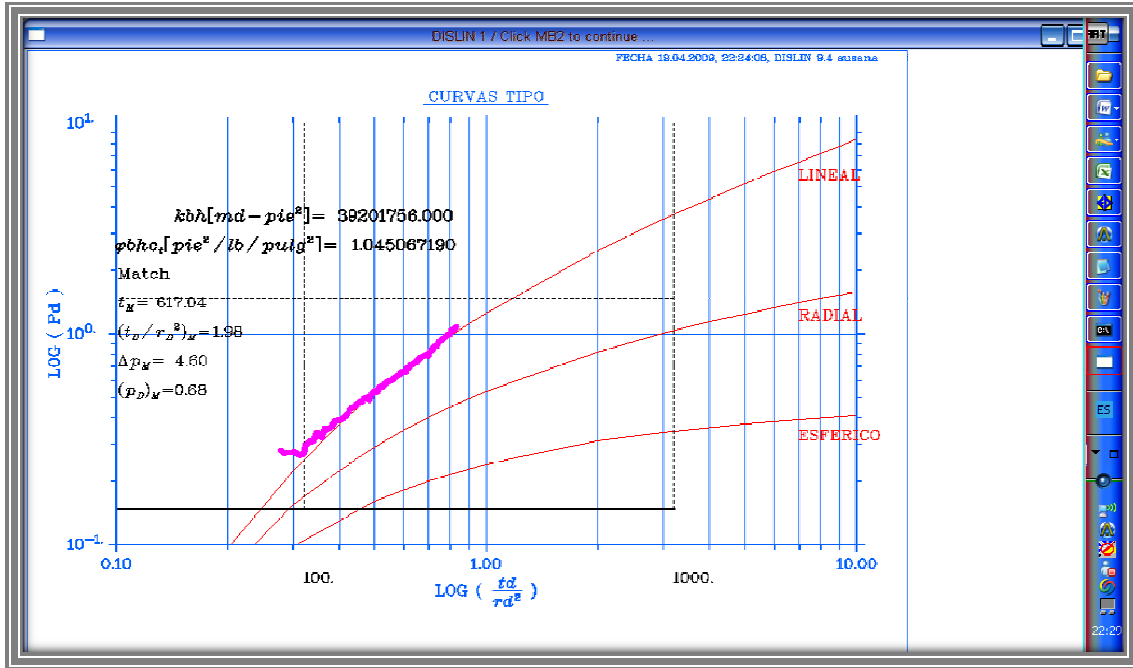
Figura 4.20. Match y parámetros de Flujo lineal
