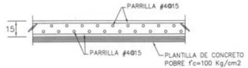
DETALLE - 2 LOSA INFERIOR DE ZAPATA
