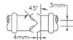
d) BISEL EN V, DOBLE.
