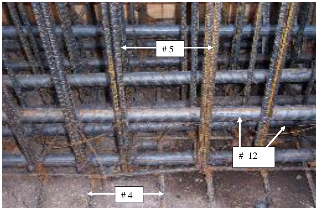
Diferentes espesores de varillas empleadas para el armado.
