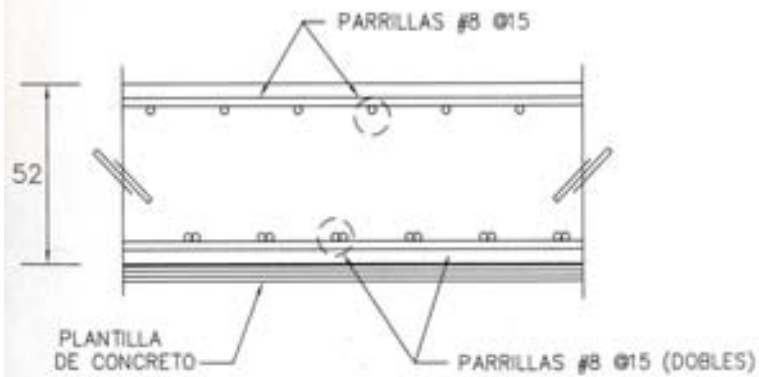
DETALLE - 3 LOSA INFERIOR DE CANDELERO
