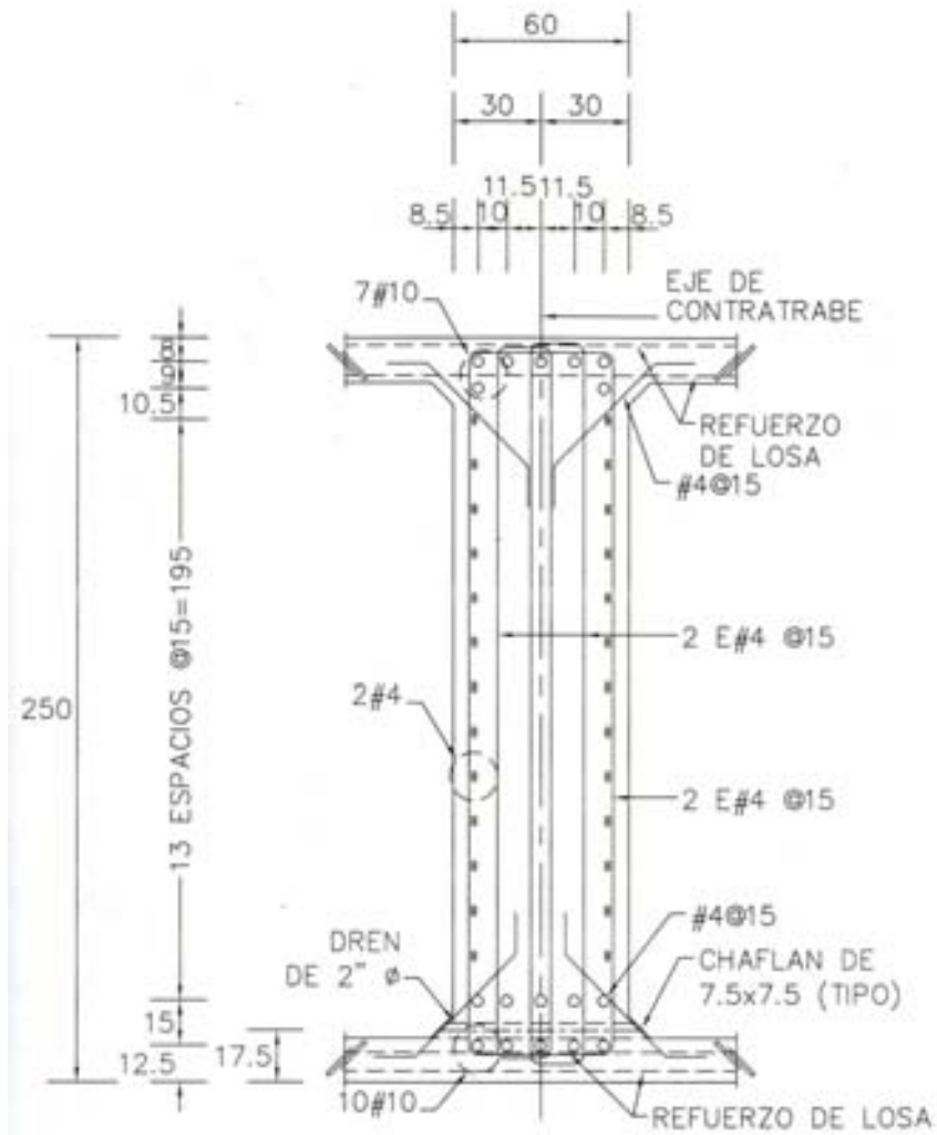
CT-3 CONTRATRABE
