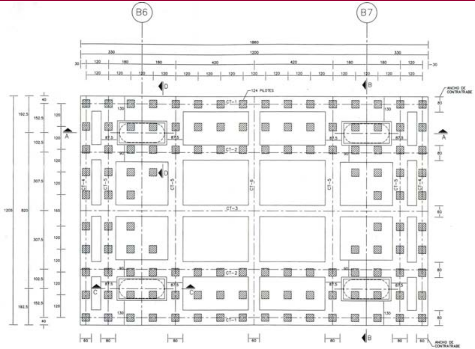
PLANTA ZAPATA
