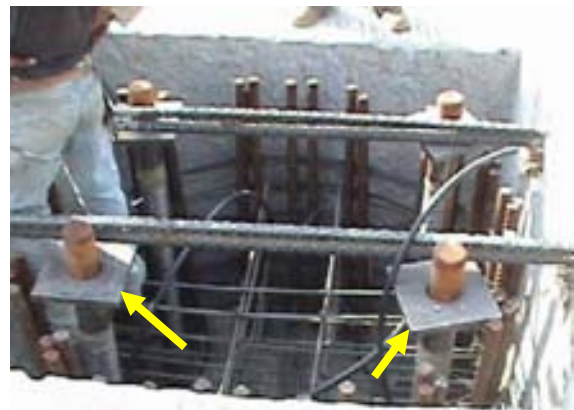
Colocación de las 4 placas para el anclaje directo de los torones
