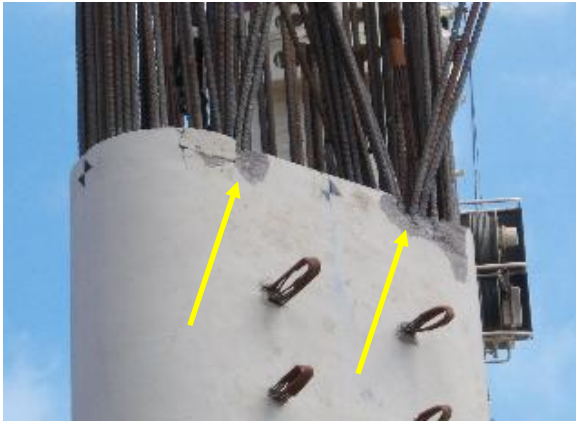
Al descargar la pieza en obra, esta sufrió despostillamientos
