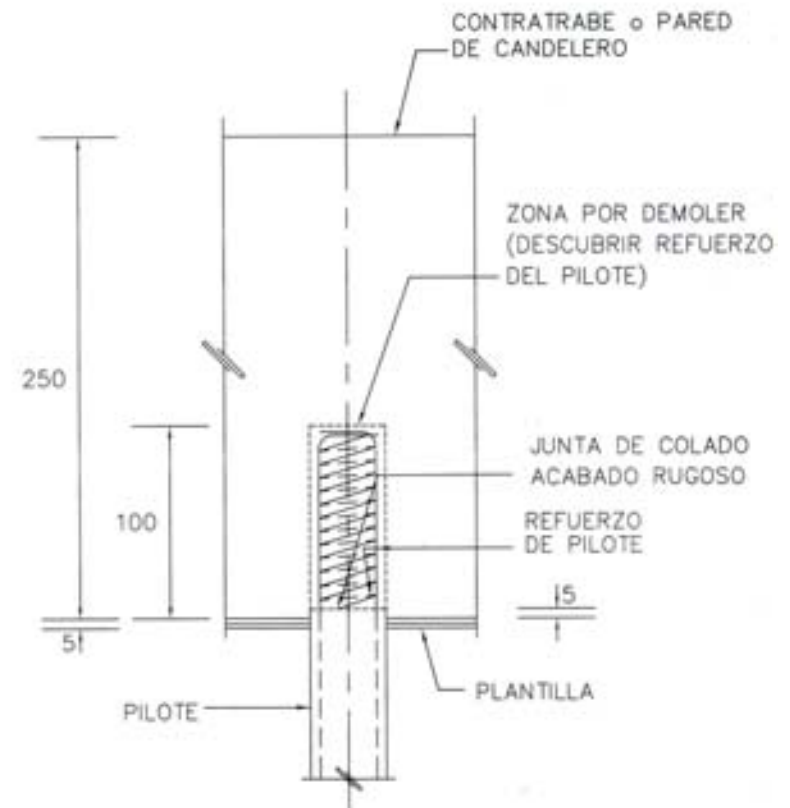
DETALLE EN CONTRATRABE
