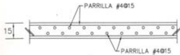
DETALLE - 1 LOSA SUPERIOR DE ZAPATA
