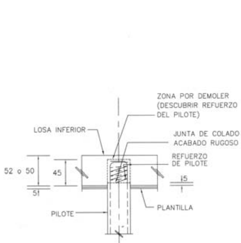
DETALLE EN LOSA
