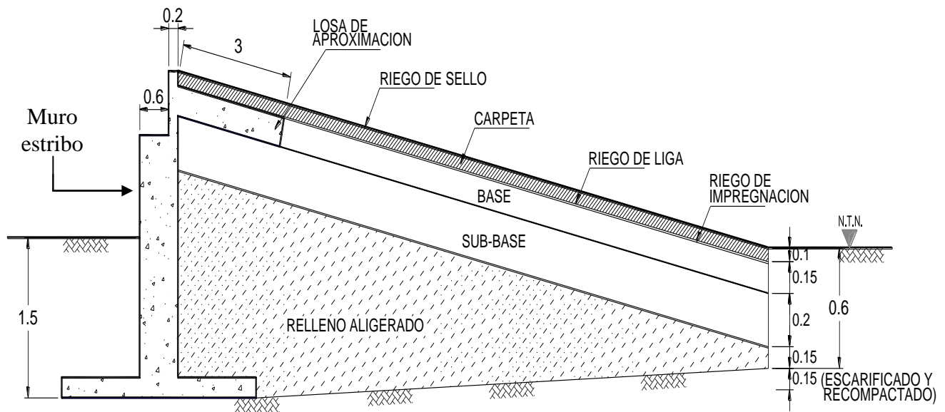
SECCION DE TERRAPLEN DE ACCESO
