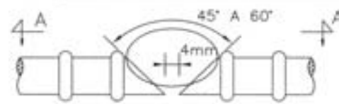
a) BISEL EN V, SENCILLA.
