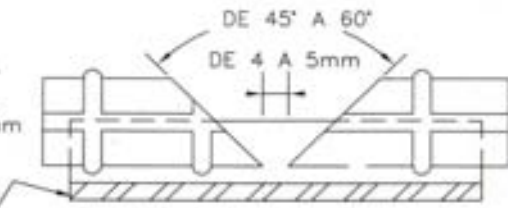
ANGULO O PLACA CURVA DE RESPALDO REQUERIDA PARA VARRILLAS #8, #10, #12.
