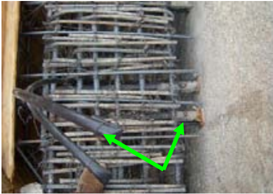
Colocación de las mangueras en los ductos de conexión de la columna-zapata
