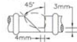
c) BISEL EN V, SENCILLA.
