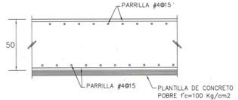
DETALLE - 4 LOSA INFERIOR DE ZAPATA
