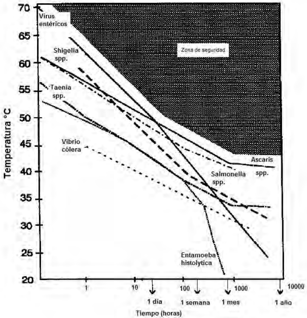
Figura 3.2 Requerimientos de tiempo y temperatura para producir lodo virtualmente libre de patógenos (Carrington et al. , 2001).
