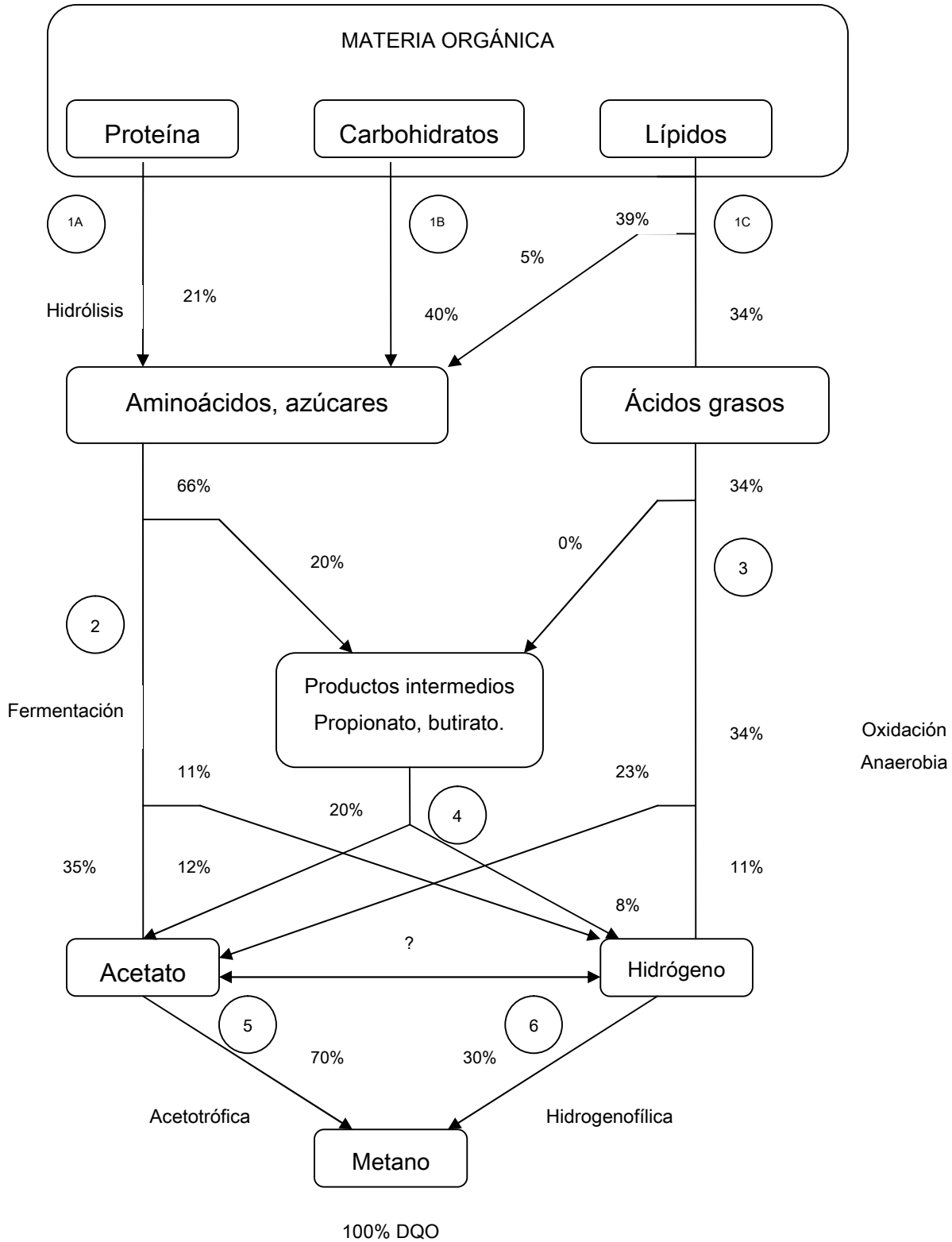
Figura 3.1 Diagrama del flujo de energía (DQO) en la digestión anaerobia de la materia orgánica particulada a metano (Gujer y Zehnder ,1983).
