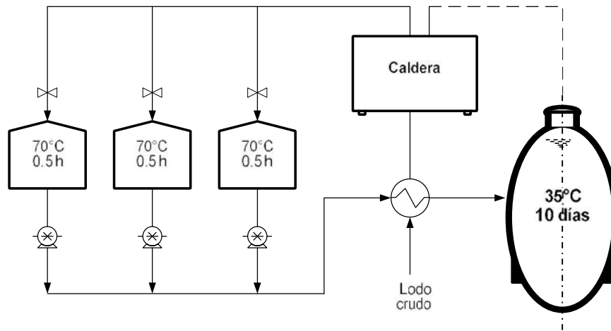
Figura 1 Esquema propuesto para el tratamiento de lodos
