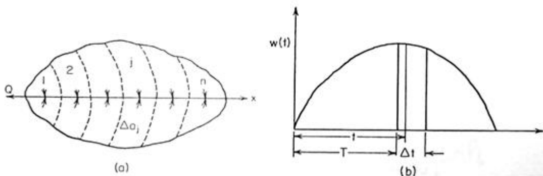
Figura 5- 6. Diagramas que describen el concepto de curvas tiempo-área (Chow, 1988).
