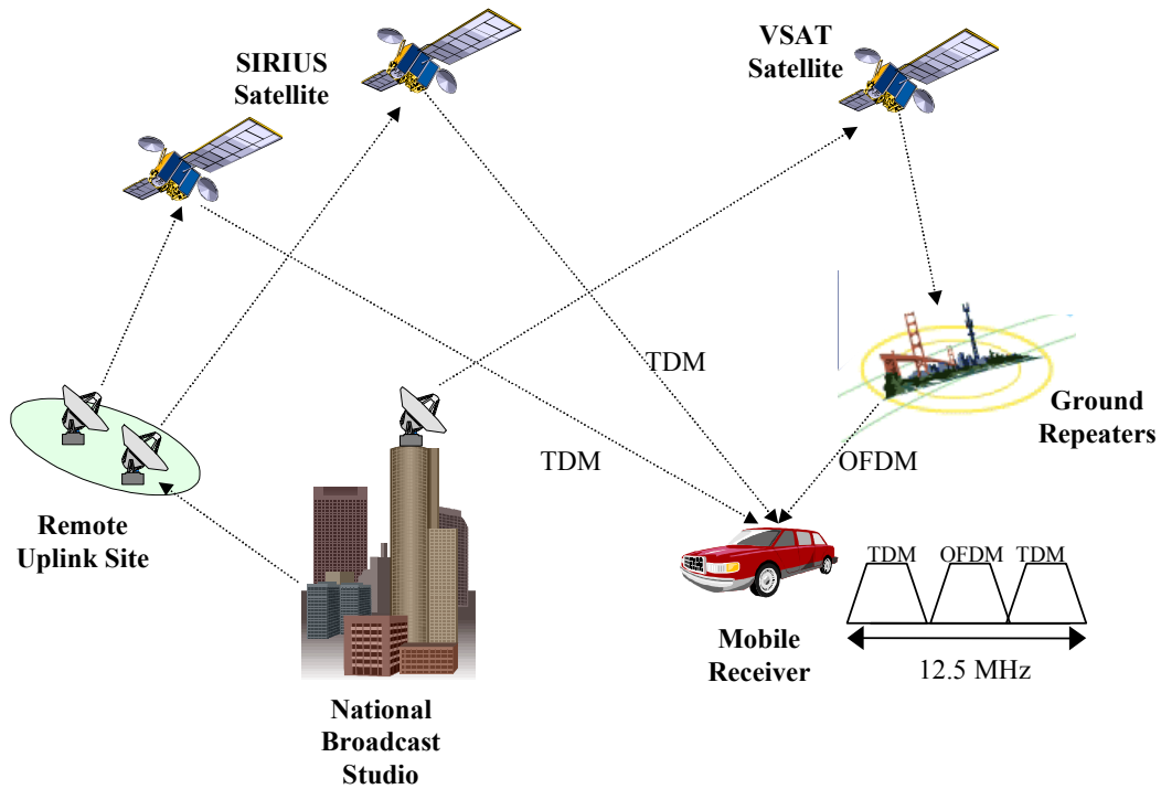
Figura 2.8 Esquema del sistema Sirius [8]
