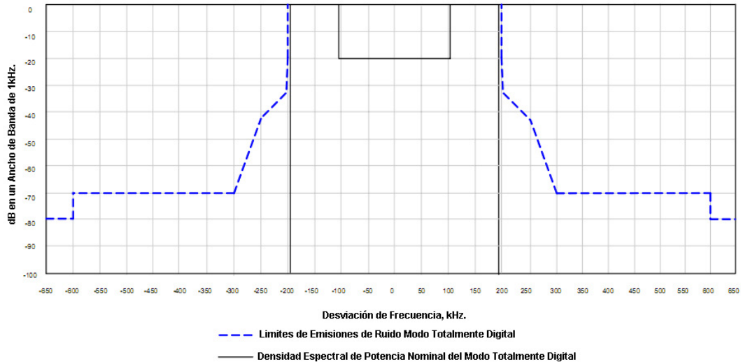
Figura 5.16 Mascara para el espectro de la forma IBOC FM Totalmente Digital
