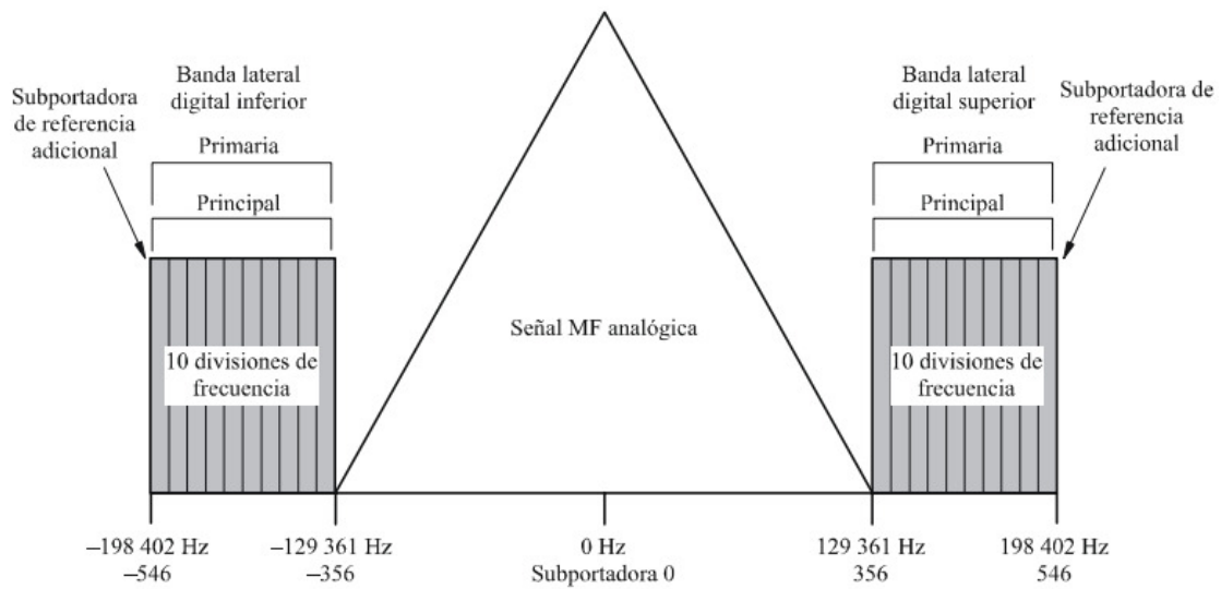
Figura 4.16 Espectro de la forma de onda de la señal IBOC FM híbrida
