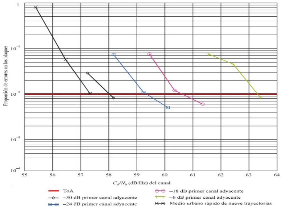
Figura 1.18 Resultados de la BER en los bloques de un sistema IBOC FM Híbrido con desvanecimiento Rayleigh (UF)
