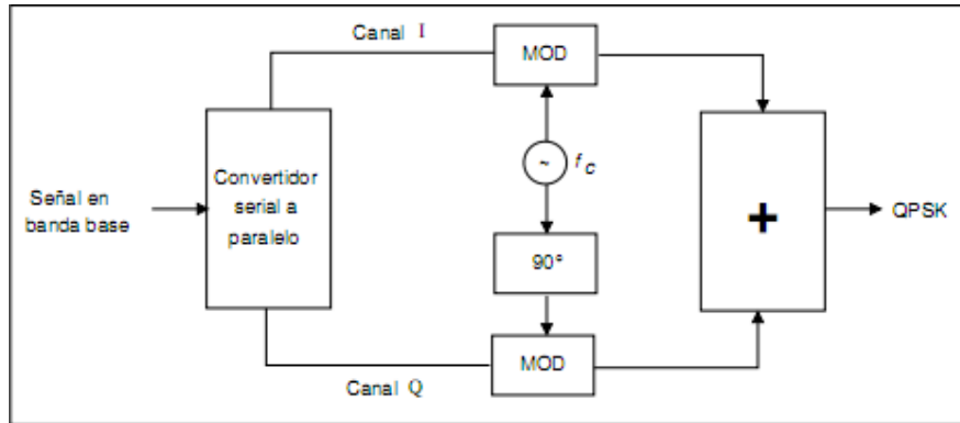
Figura 3.6 Modulador QPSK
