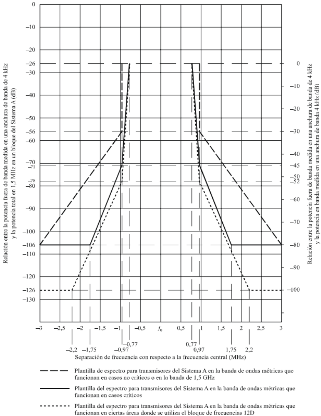
Figura 5.6 Plantillas del espectro fuera de banda para una señal de transmisión del sistema DAB
