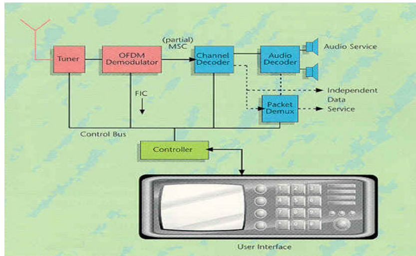
Figura 2.2 Recepción de una señal DAB [3]
