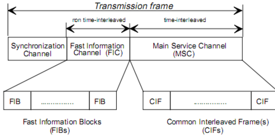
Figura 3.6 Trama DAB
