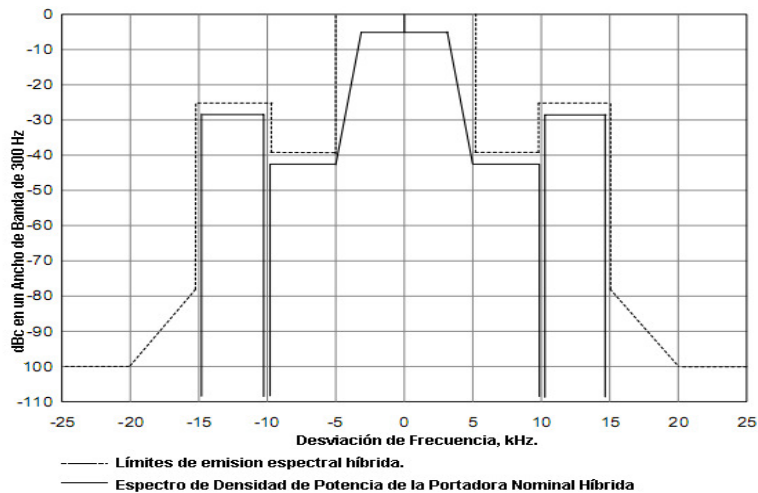
Figura 5.12 Mascara para el espectro IBOC AM híbrido
