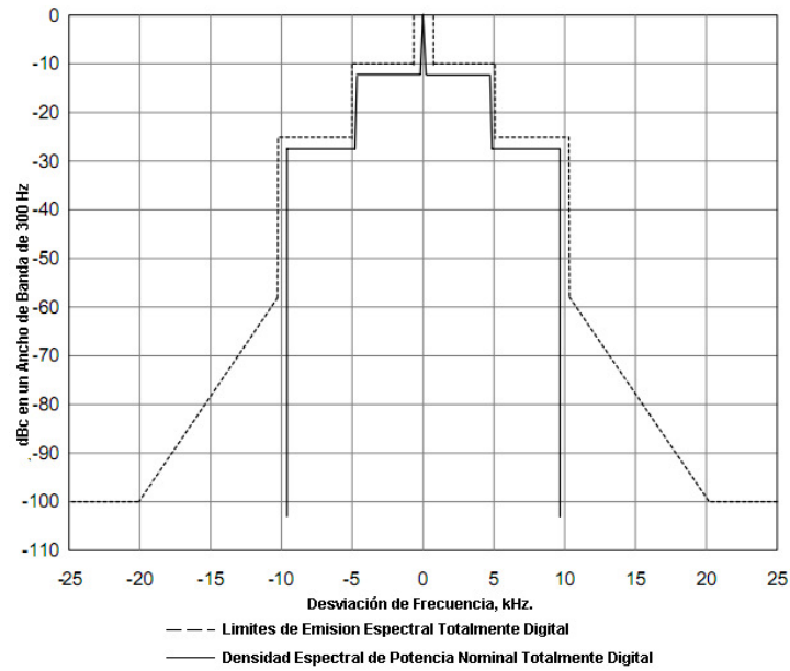
Figura 5.13 Mascara para el espectro IBOC AM totalmente digital
