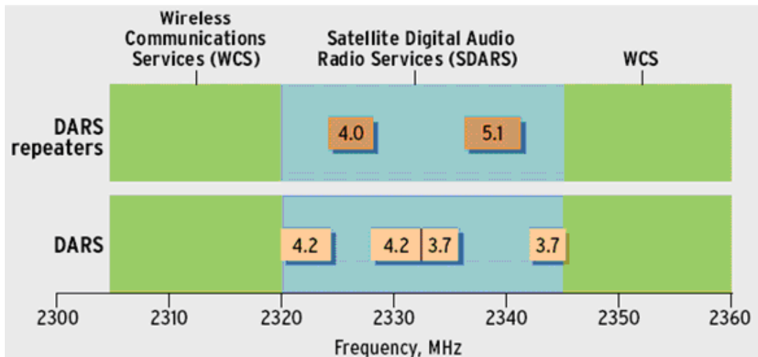
Figura 2.7 Utilización del espectro de frecuencias para DARS [8]
