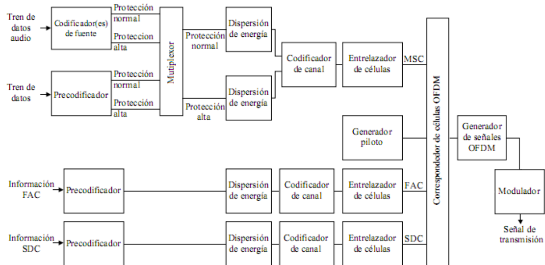
Figura 2.5 - Diagrama de bloques de entrada a un transmisor DRM.
