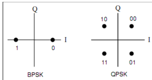
Figura 3.5 Diagramas de constelación para BPSK y QPSK
