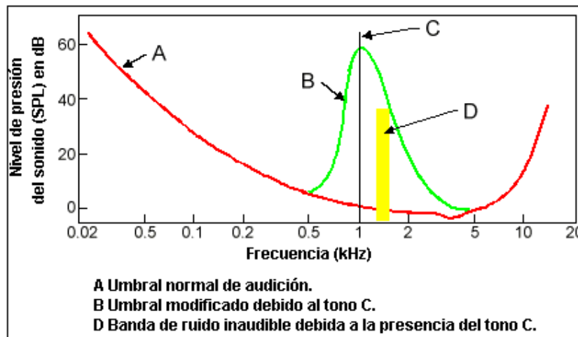
Figura 3.1 Efecto de enmascaramiento del oído humano
