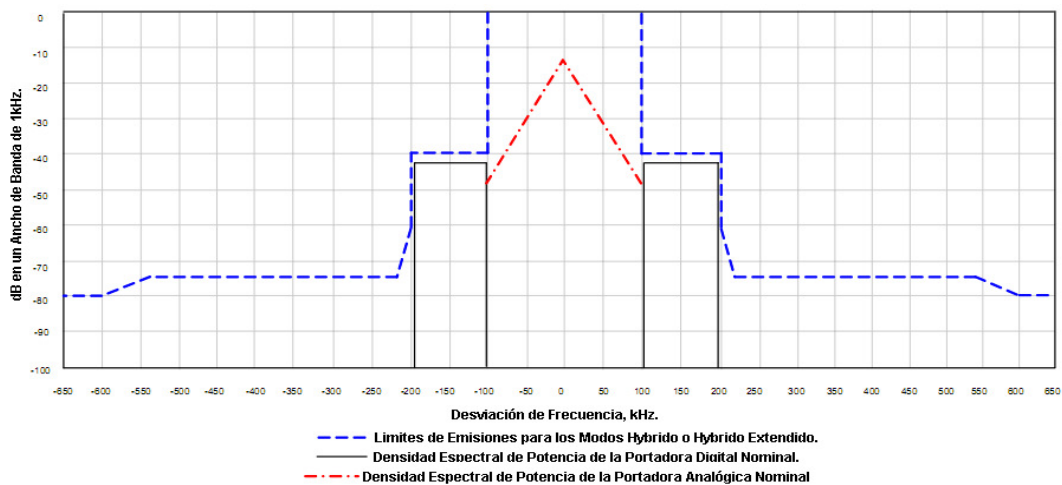
Figura 5.15 Máscara para el espectro de la forma IBOC FM Híbrida
