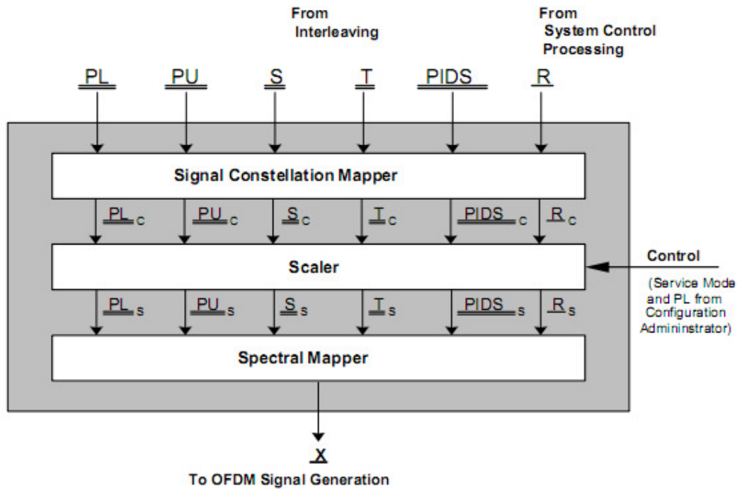
Figura 4.8 Diagrama de bloques conceptual del mapeo de sub-portadoras
