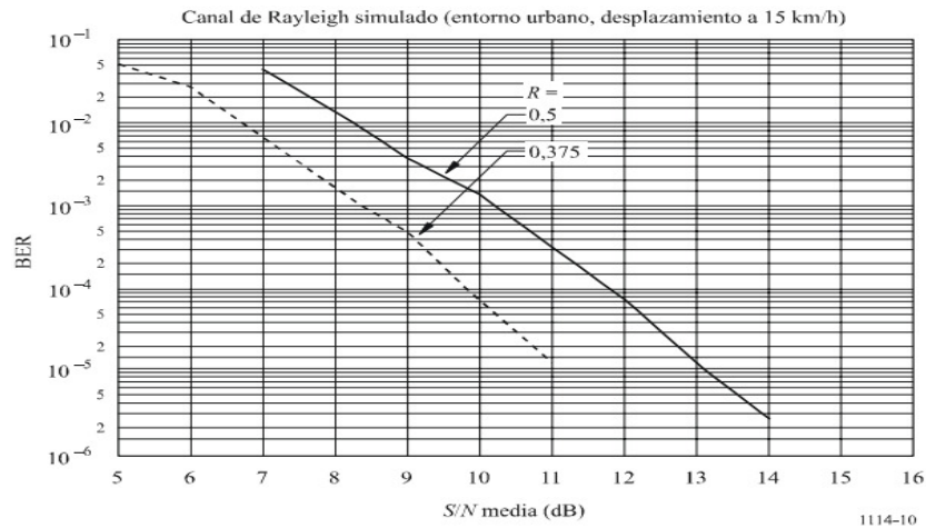
Figura 5.9 BER en función de la relación S/N para el sistema DAB (Modo de transmisión I @ 226 MHz)
