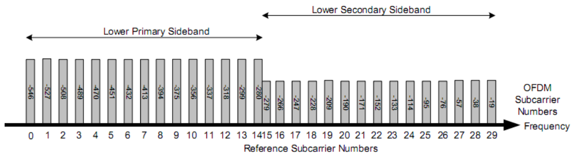
Figura 4.14 Mapeo espectral de la sub-portadora de referencia en la banda lateral inferior
