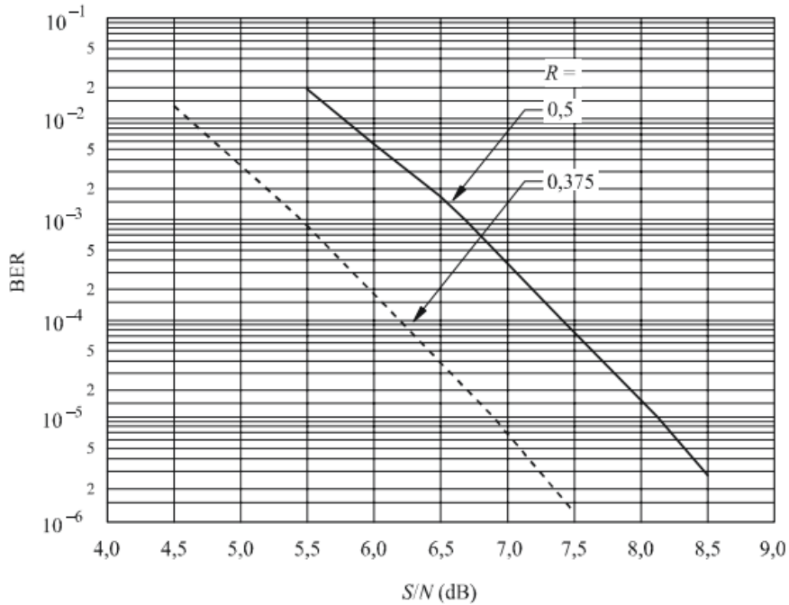
Figura 5.8 BER en función de la relación S/N para el sistema DAB (Modo de transmisión II ó III): Canal gaussiano
