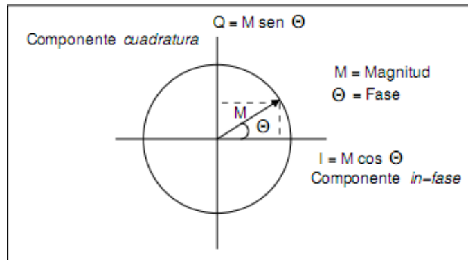
Figura 3.5 Plano I-Q
