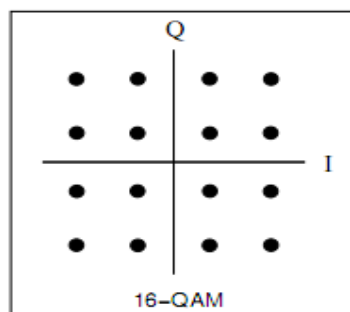
Figura 3.7 Diagrama de la constelación 16 QAM
