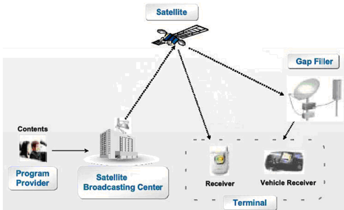
Figura 2.6 Diagrama de transmisión - recepción Radio Satelital [8]
