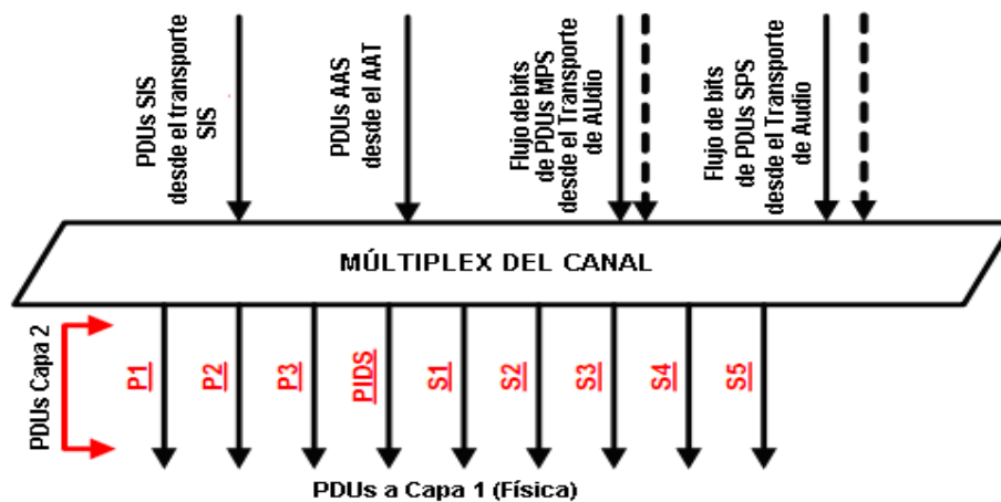
Figura5.3 Múltiplex IBOC
