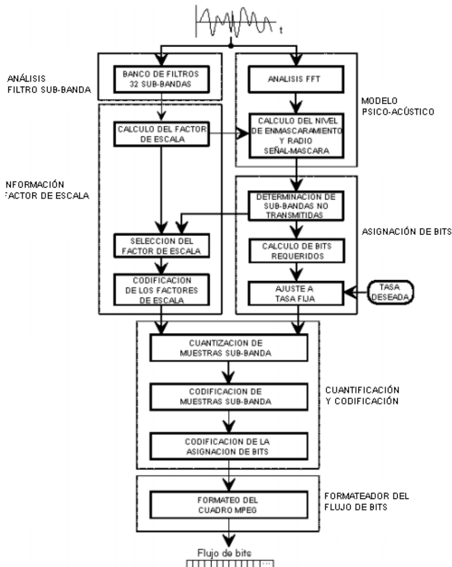
Figura 3.2 Diagrama de la codificación de audio MPEG Capa II
