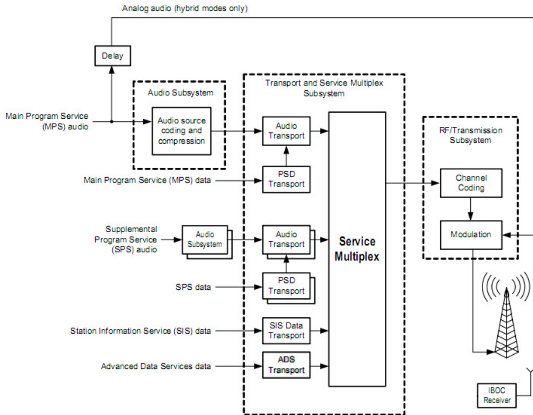
Figura 2.3 Funcionamiento del sistema IBOC
