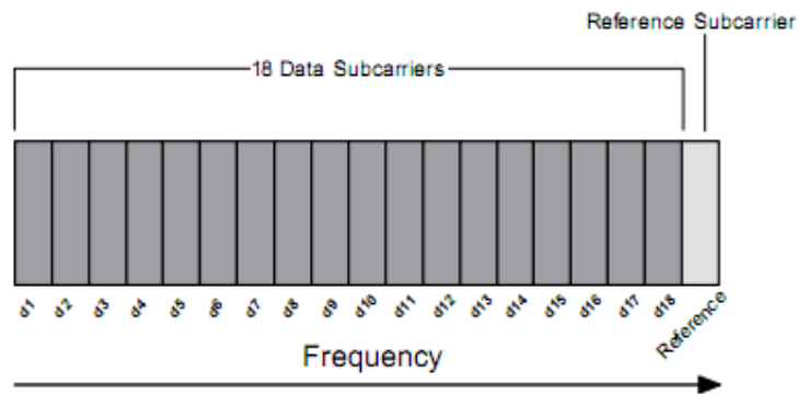
Figura 4.13 Partición de frecuencia. Distribución B
