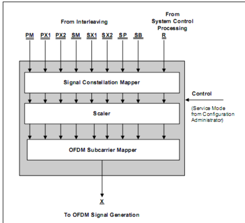
Figura 4.11 Diagrama de bloques del mapeo de sub-portadoras OFDM para IBOC-FM
