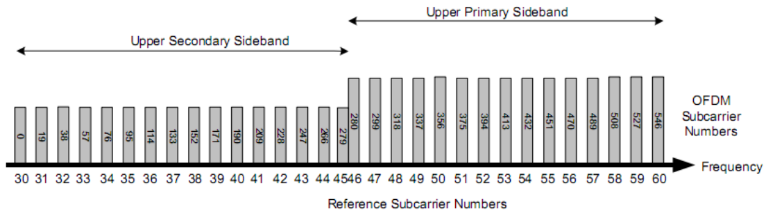
Figura 4.15 Mapeo espectral de la sub-portadora de referencia en la banda lateral superior
