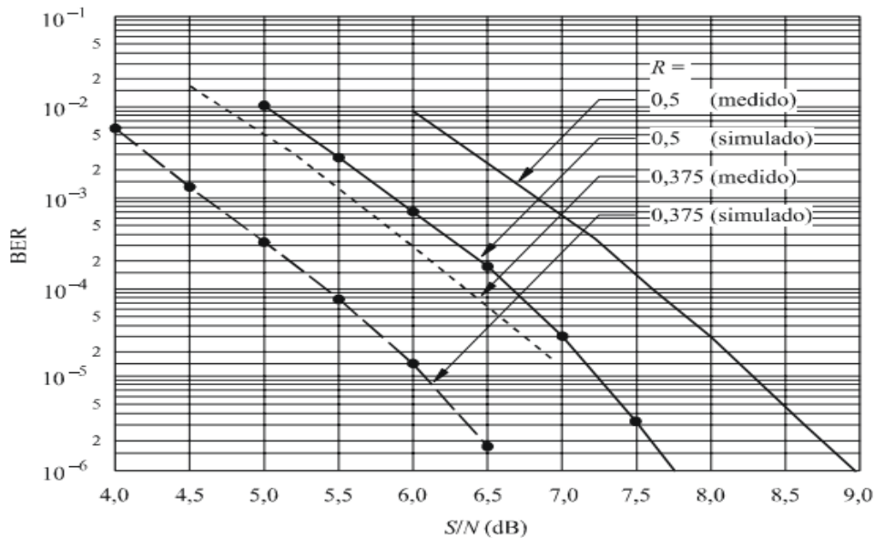
Figura 5.7 BER en función de la relación S/N para el sistema DAB (Modo de transmisión I): Canal Gaussiano
