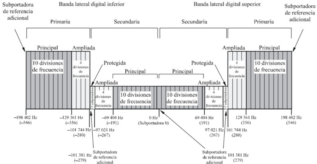
Figura 4.17 Espectro de la señal IBOC FM totalmente digital
