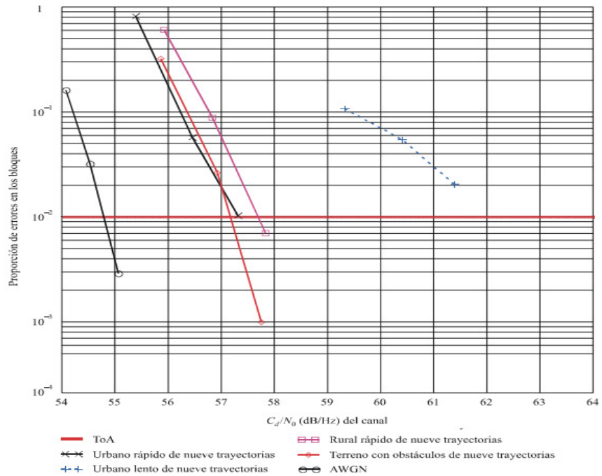
Figura 5.17 Resultados de la BER del sistema IBOC Híbrido en FM ante diferentes tipos de desvanecimiento de nueve trayectorias y ruido gaussiano blanco aditivo (AWGN)
