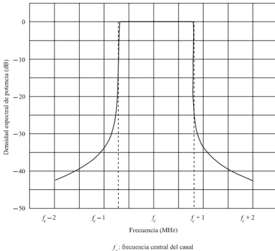
Figura 5.5 Espectro teórico de la señal de transmisión del sistema DAB en el Modo II
