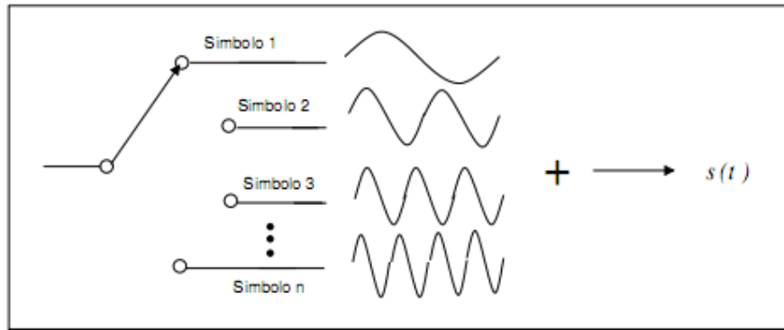
Figura 3.8 Idea básica de la técnica OFDM
