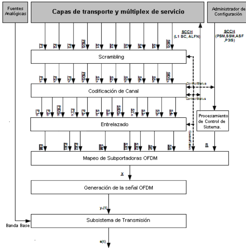
Figura 5.14 Diagrama de Bloques de la Capa Física IBOC FM
