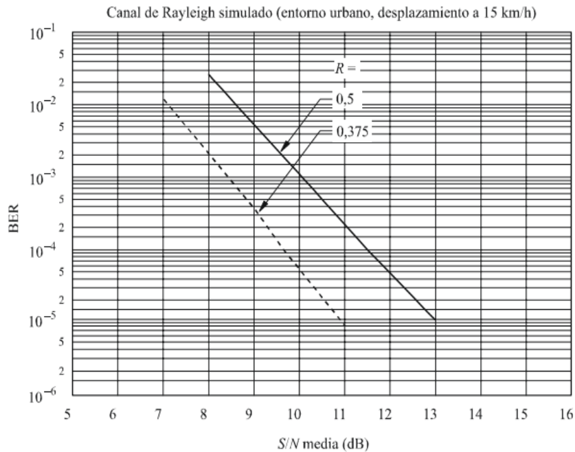
Figura 5.10 BER en función de la relación S/N para el sistema DAB (Modo de transmisión II @ 1480 MHz)
