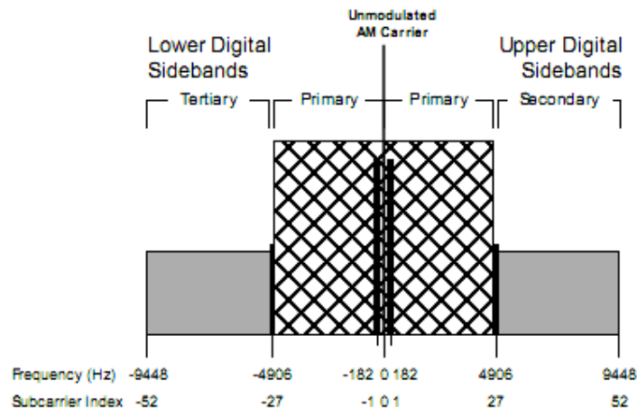
Figura 4.10 Espectro de la señal IBOC AM totalmente digital
