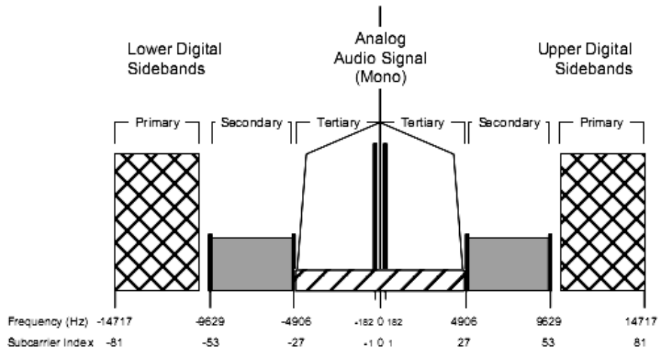
Figura 4.9 Forma de onda del espectro de AM IBOC híbrido
