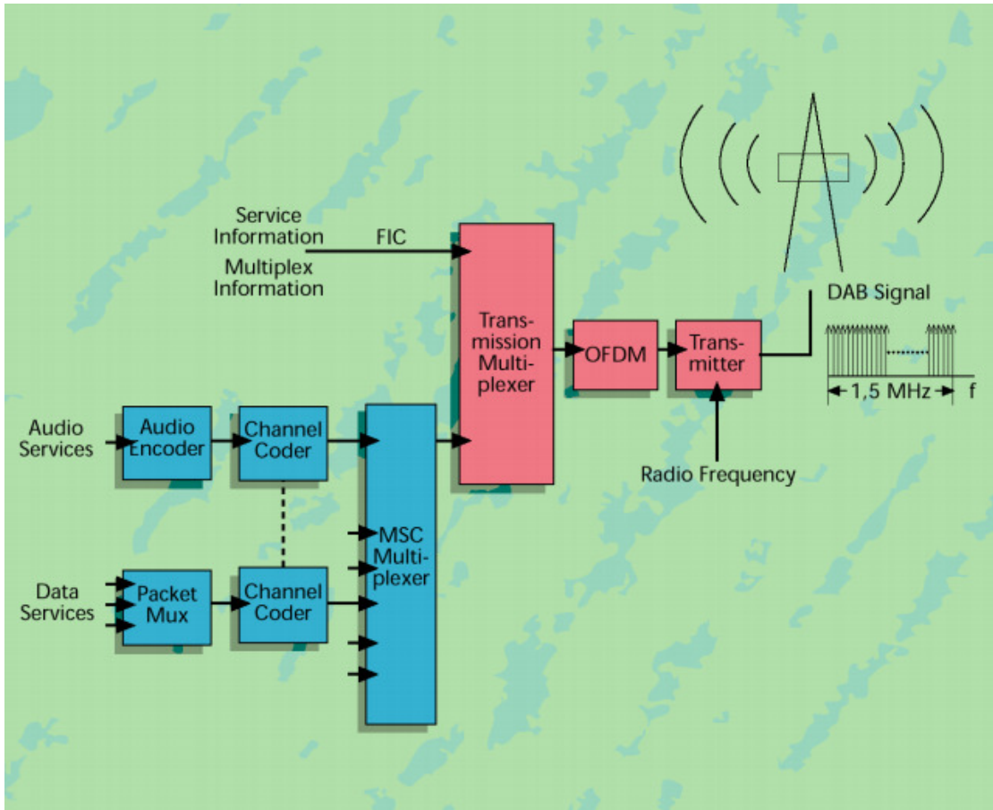
Figura 2.1 Generación de una señal DAB [3]
