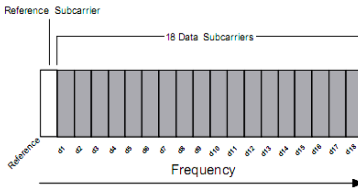
Figura 4.12 Partición de frecuencia. Distribución A
