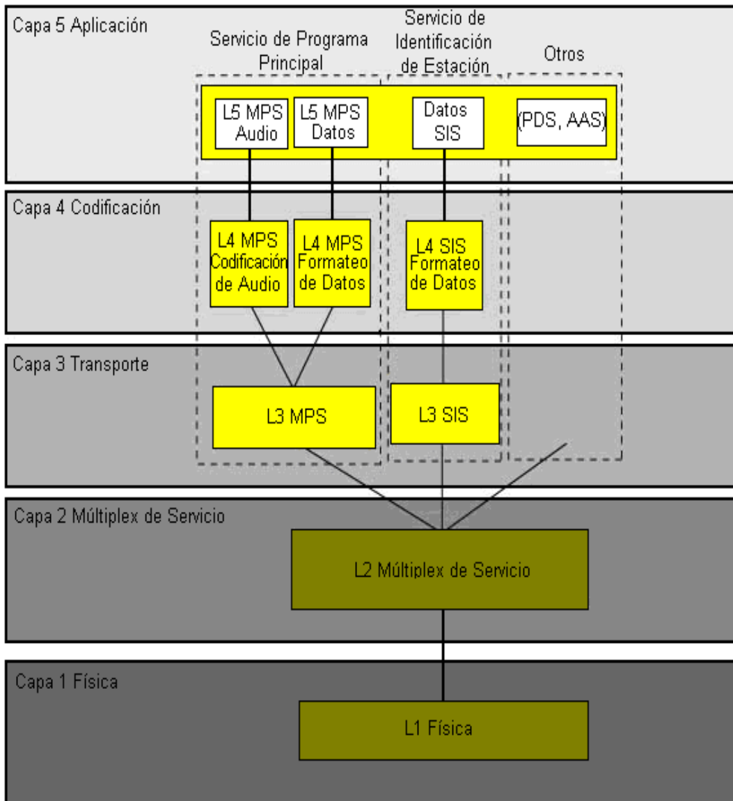
Figura5.1 Modelo por capas IBOC [2]
