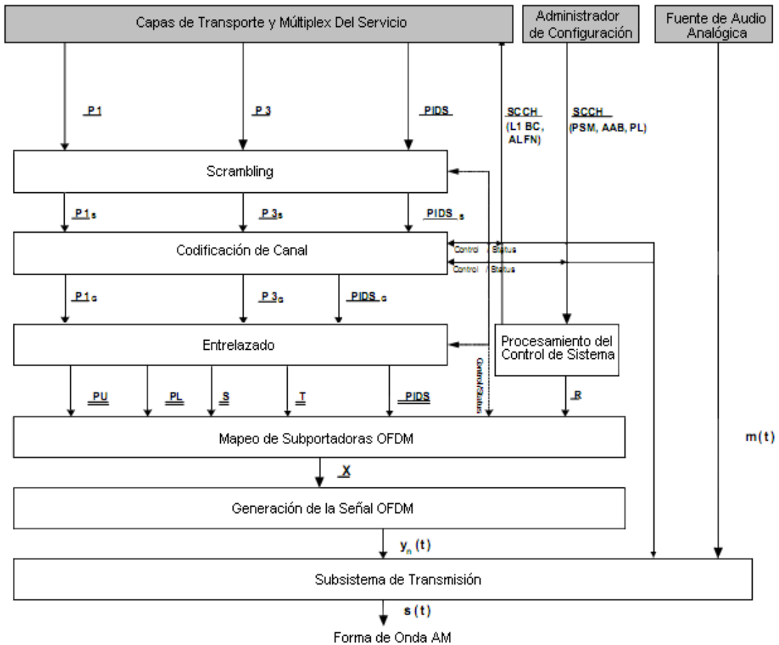
Figura 5.11 Diagrama de Bloques de la Capa Física IBOC AM
