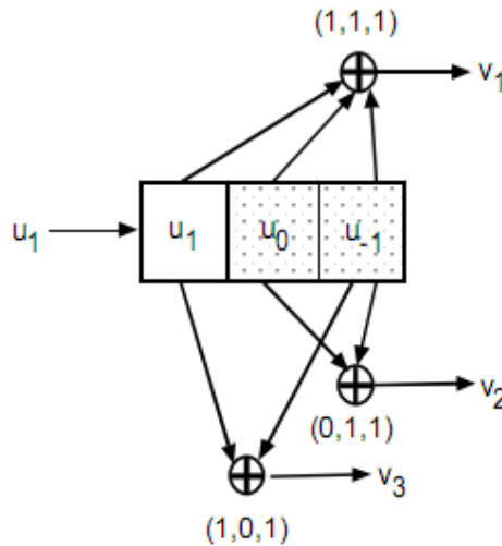
Figura 3.4 - Ejemplo de un código convolucional de tres registros de memoria.
