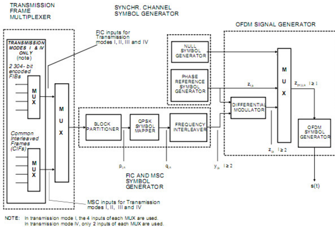
Figura 4.1 Diagrama de bloques del proceso de modulación OFDM en DAB
