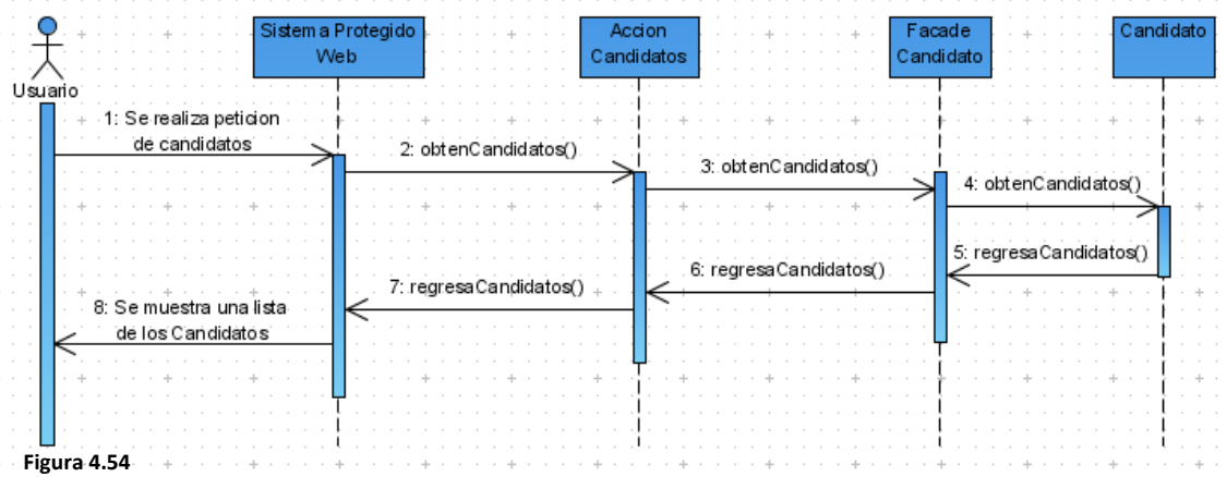
Diagrama de secuencia del caso de uso Consultar Candidatos
