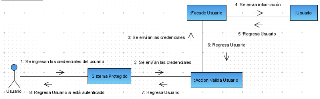
Figura 4.31 Diagrama de colaboración del caso de uso Ingresar al Sistema Protegido
