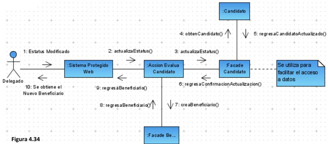
Diagrama de colaboración del caso de uso Evaluar Candidato
