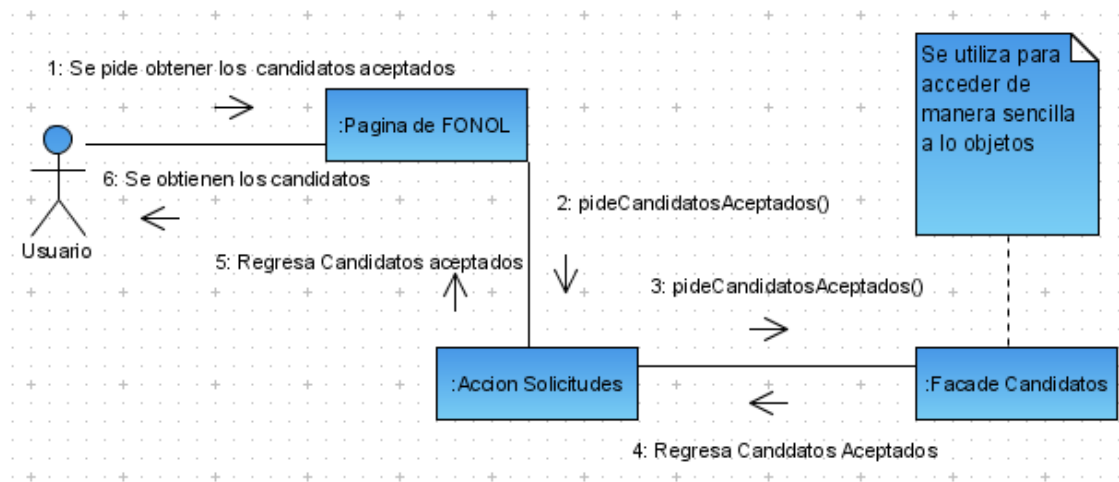
Figura 4.30 4.2.5.8. Ingresar al Sistema Protegido Diagrama de colaboración del caso de uso Revisar Candidatos Aceptados
