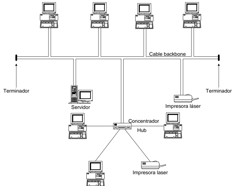
Figura 1.8. Topología de árbol.
