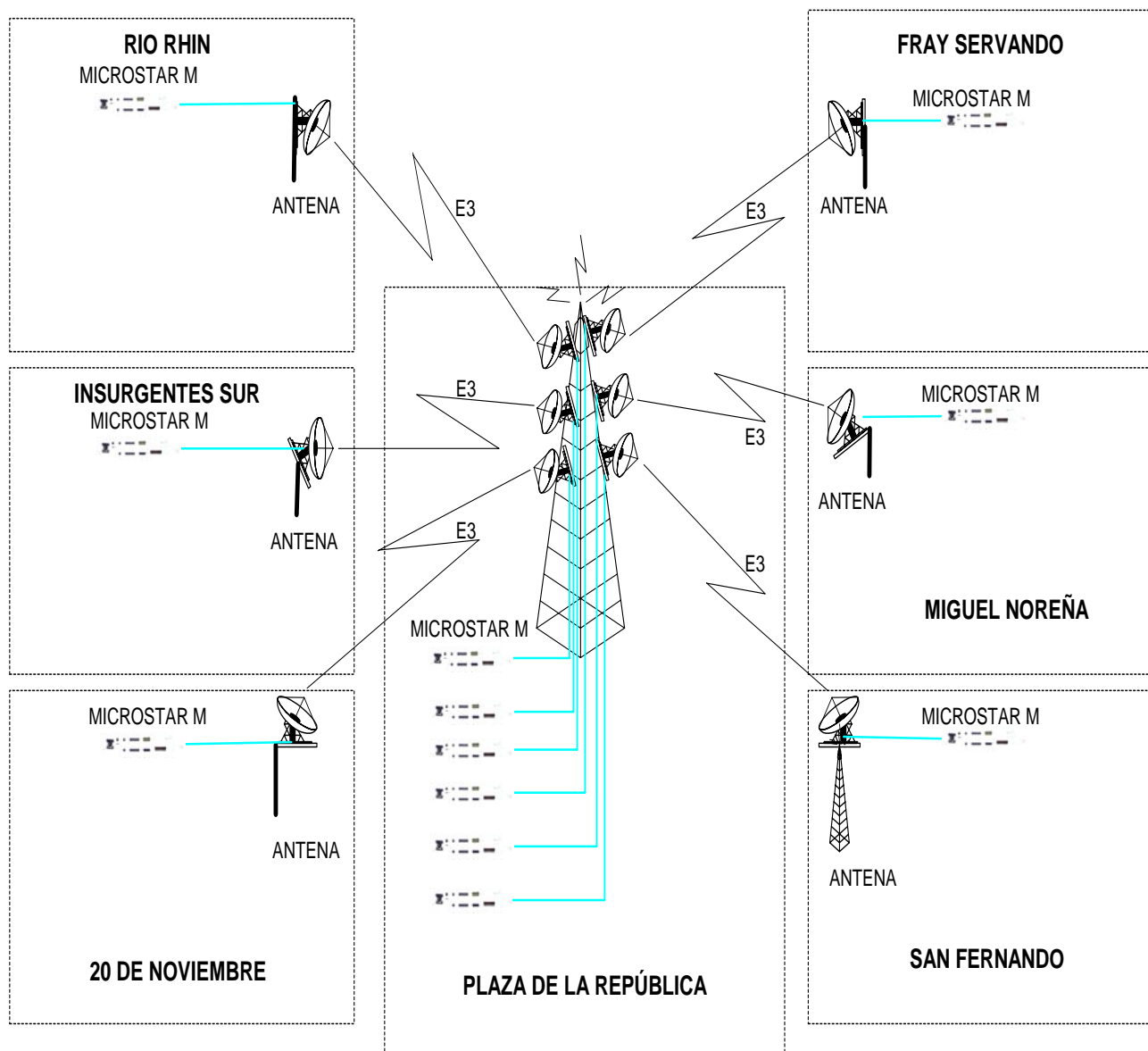
Figura 4.1. Esquema general de enlaces de microondas.
