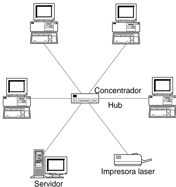
Figura 1.6. Topología de estrella.
