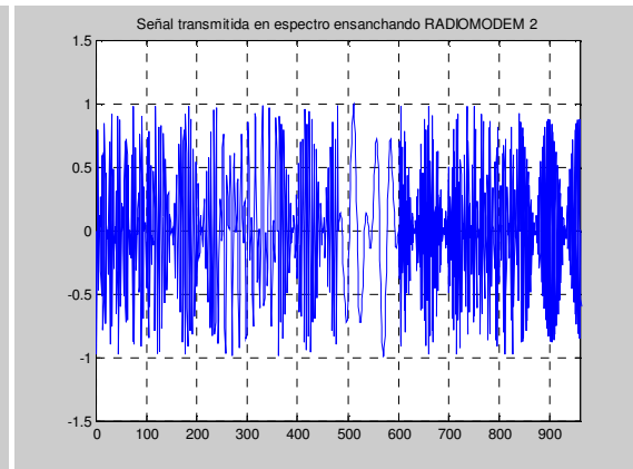
Fig 46. Señal transmitida del radio 2
