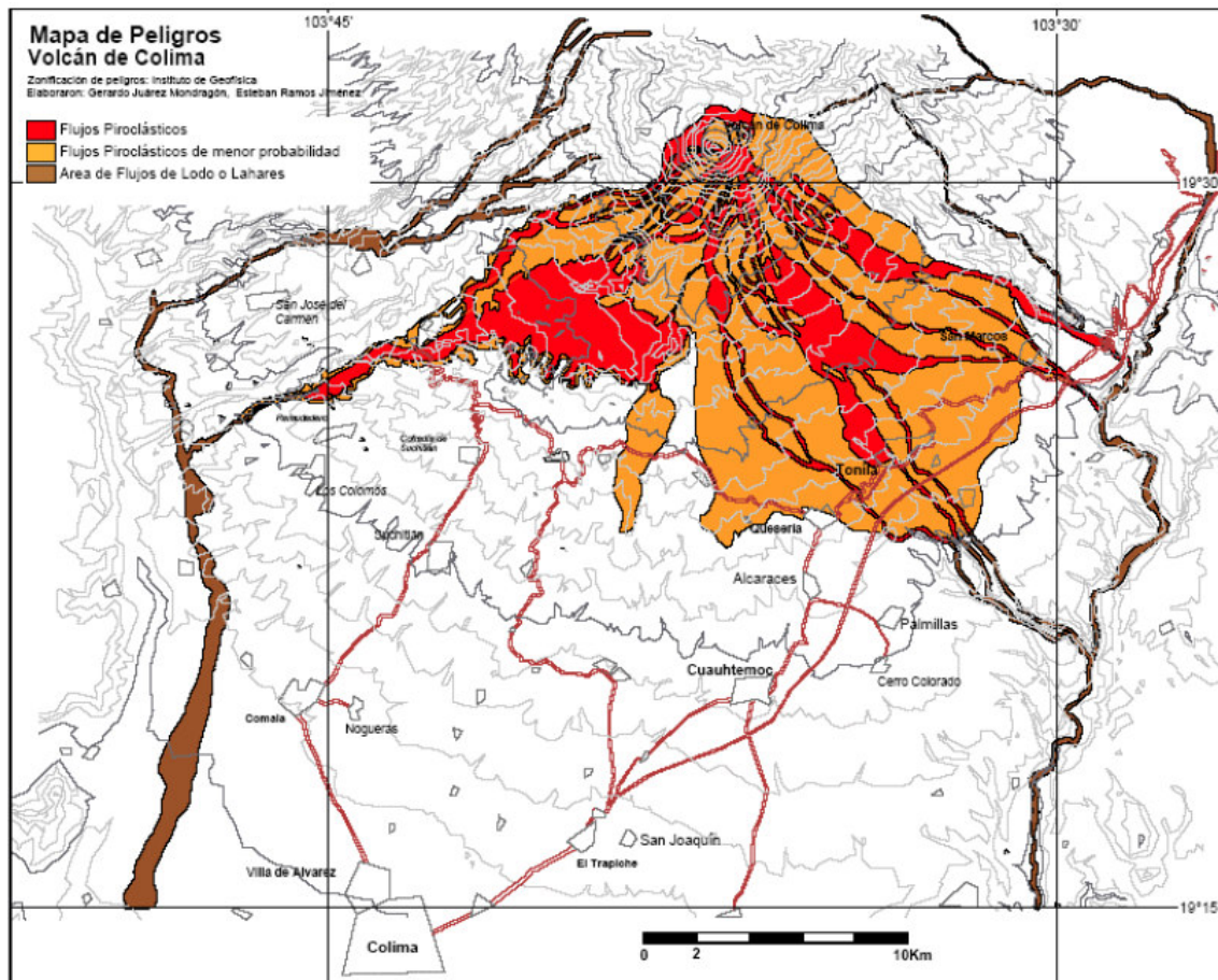
Fig 9. Mapa de peligros del volcán de Fuego de Colima
