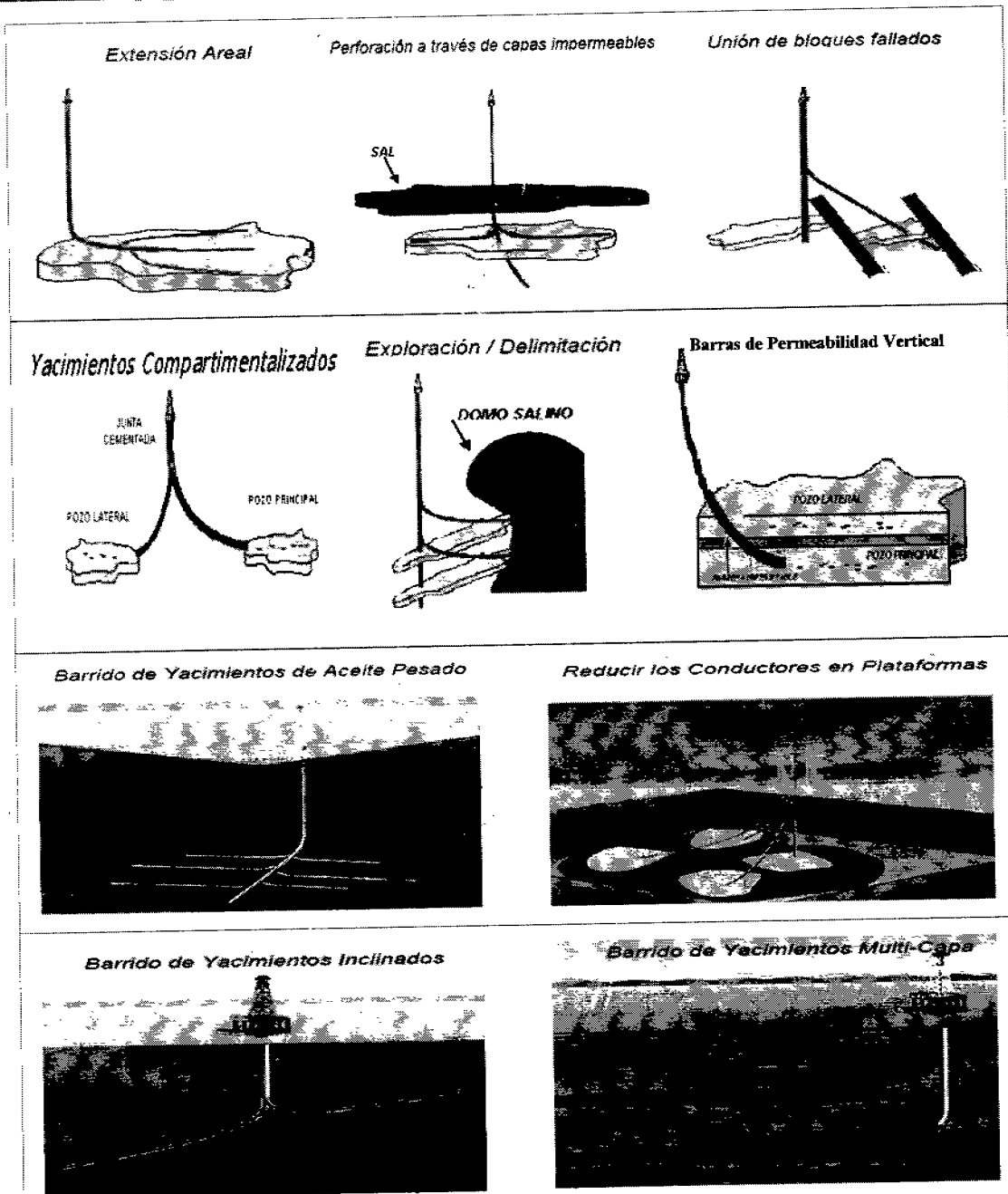
Figura 4.15. Principales aplicaciones de pozos multilaterales (Rocío León, 2007).
