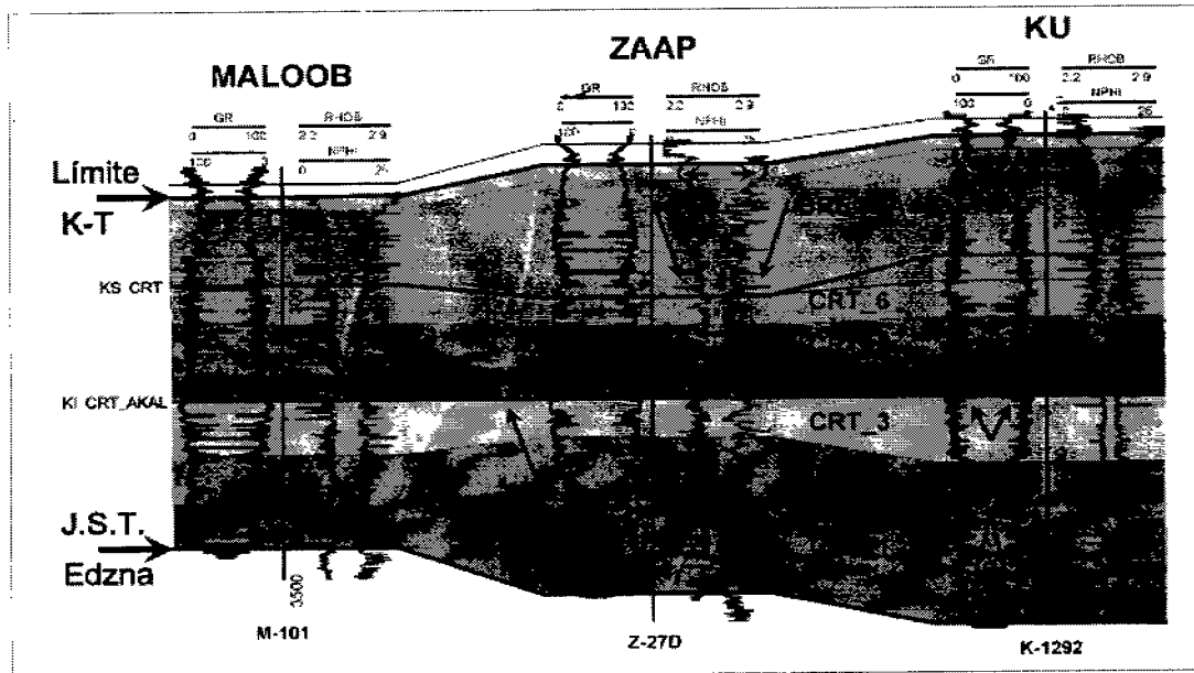
Figura 2.8. Correlación estratigráfica para los campos de KMZ utilizando registros convencionales (RG, RHOB y NPHI); el nivel de referencia es el contacto entre Cretácico Inferior y Superior; KI-CRT_AKAL (PEMEX, 2006).
