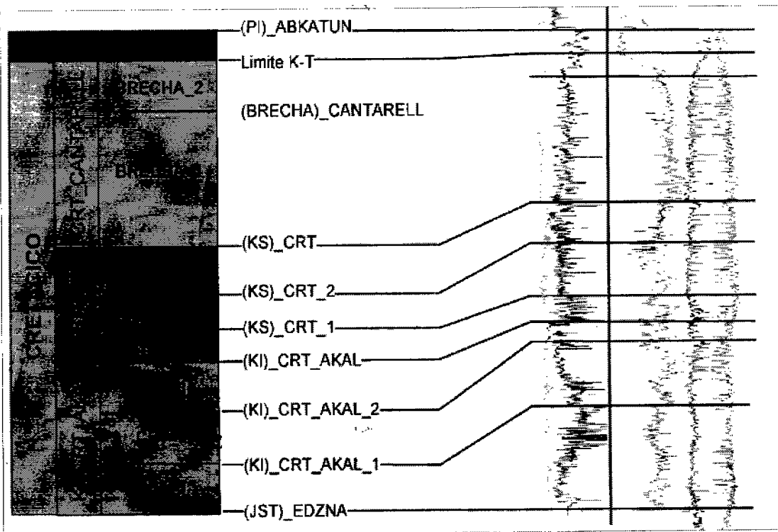
Figura 2.7. Columna estratigráfica con las 8 unidades definidas y registros convencionales en un pozos Tipo de KMZ (Pemex Exploración y Producción, 2006).
