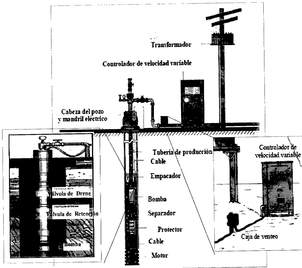
Figura 5.23. Componentes del aparato de BEC (Prado, 2003).
