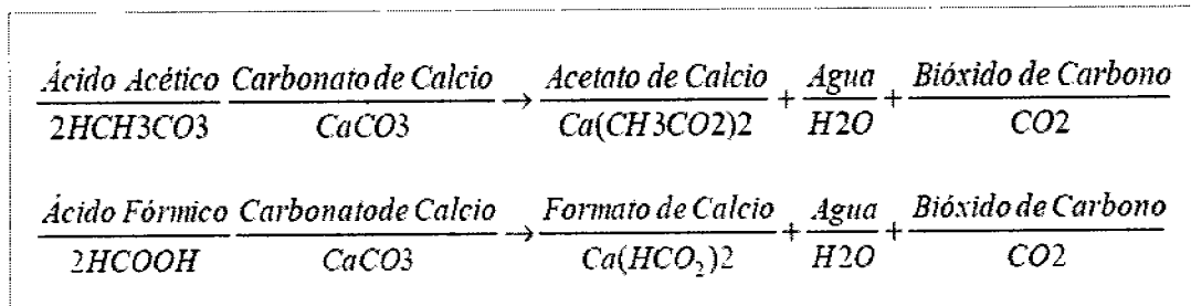
Figura 4.24. Reacción de los ácidos orgánicos con la caliza (Guía para el diseño de estimulación de pozos, PEMEX, 2004).
