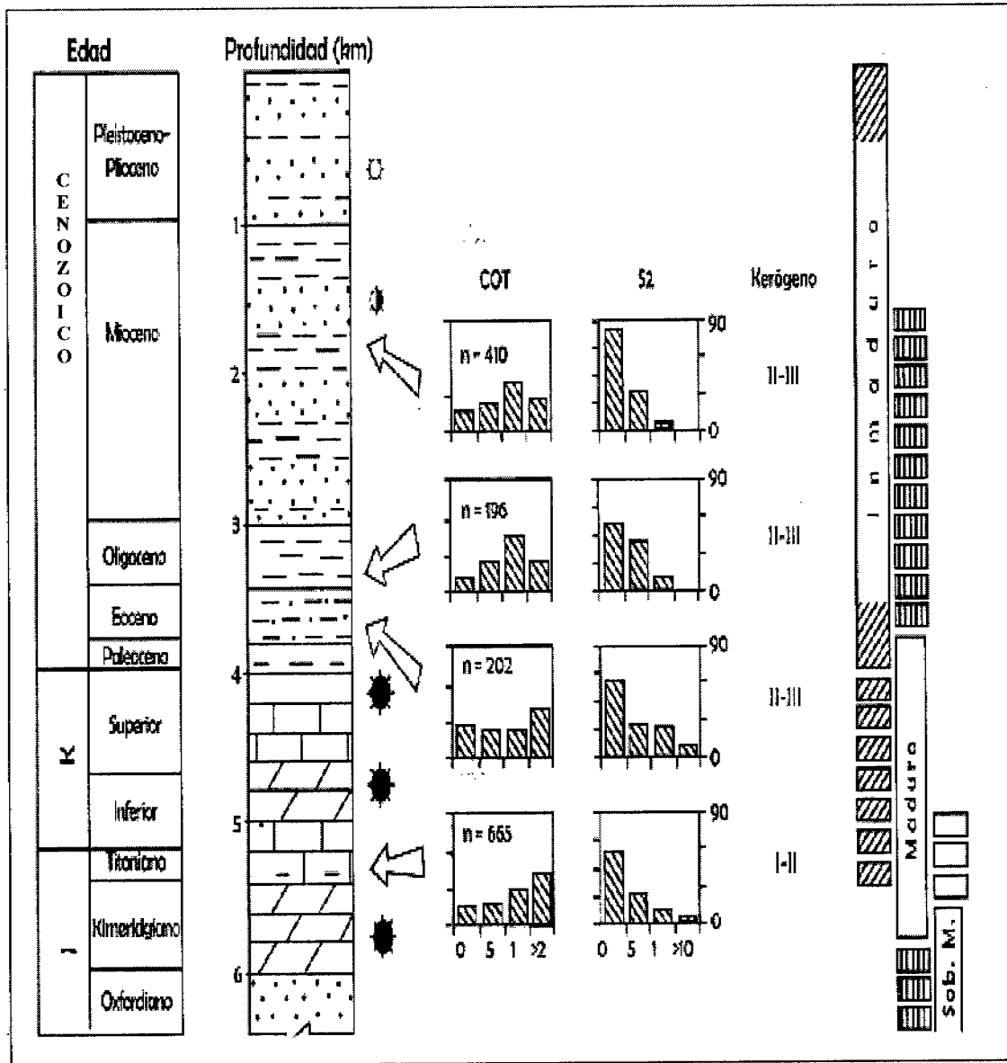
Figura 3.2. Secuencias generadoras de la Sonda de Campeche. El Titoniano y Kimeridgiano son las secuencias estratigráficas de mayor madurez y mayor cantidad de COT, con kerógeno de tipo I-II (Modificado de González y Holguín, 1991).
