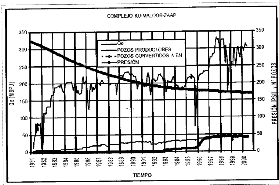
Figura 5.13. Caída de presión en los yacimientos del K-T en el complejo KMZ desde su explotación hasta el 2001 (Publicación del CIPM, 2003).
