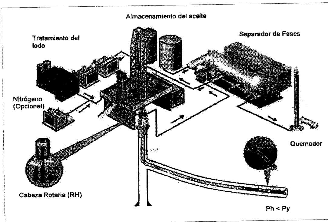
Figura 4.4. Arreglo típico de la perforación bajo balance (Cuahtémoc García, 2007).
