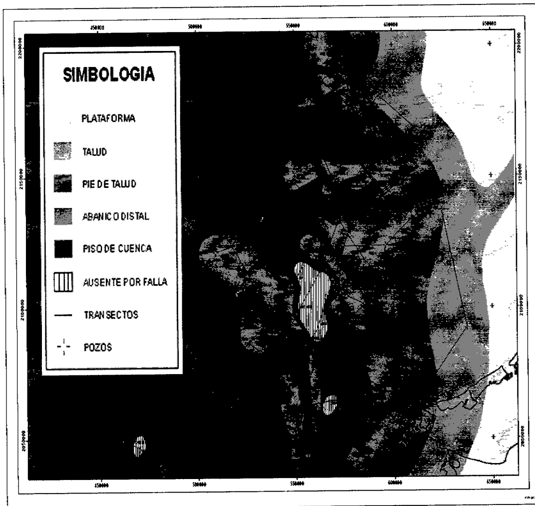
Figura 3.43. Mapa de Litofacies del KM, Albiano (PEMEX 2006).
