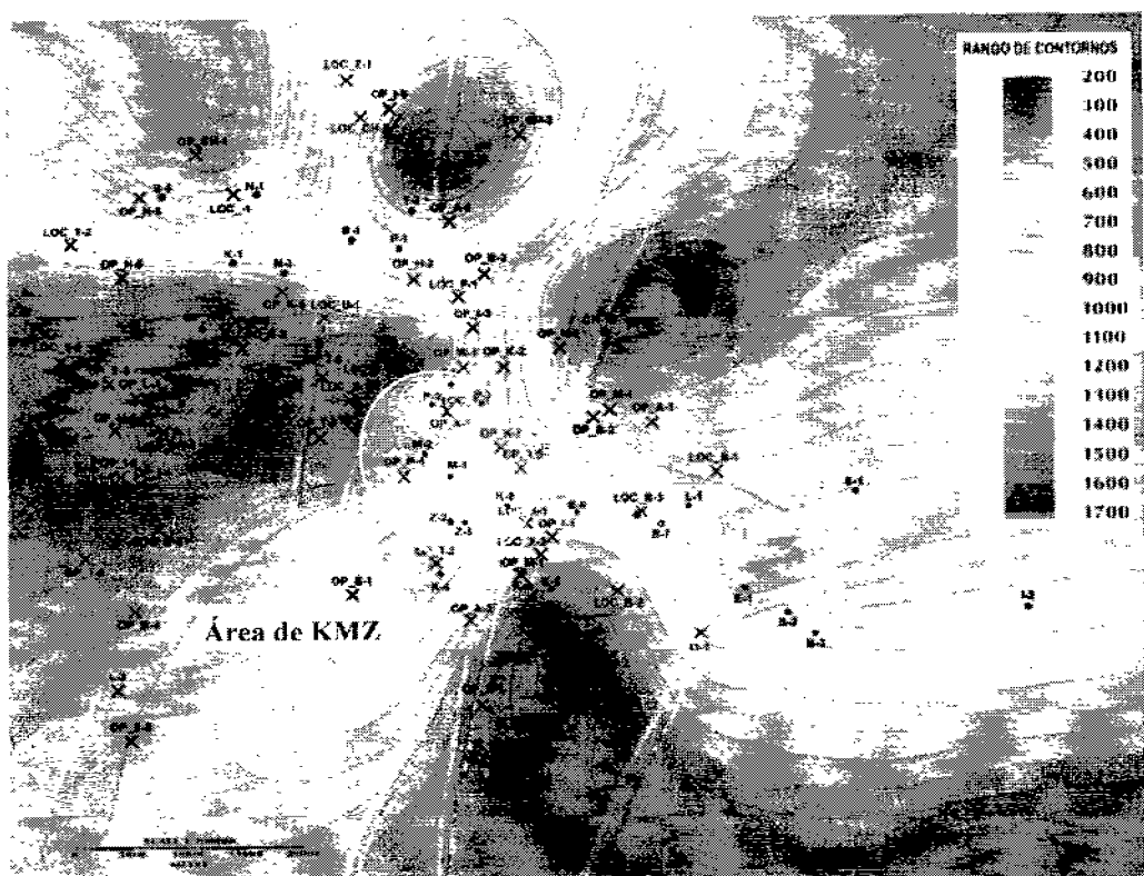
Figura 3.60. Espesor bruto de la Unidad V en la Sonda de Campeche correspondiente al Mioceno-Plioceno. (Nancy Rodrigues, 2007)
