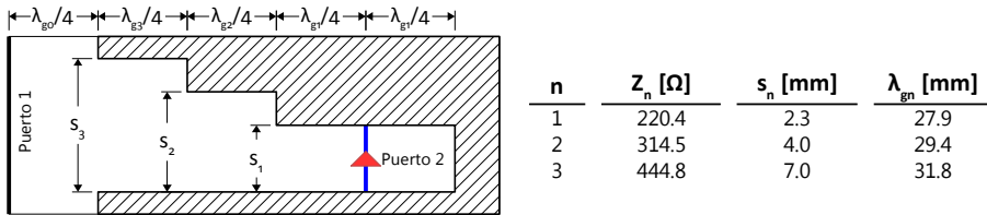
Figura 4.12: Diseño de la red de entrada utilizando un transformador binomial.
