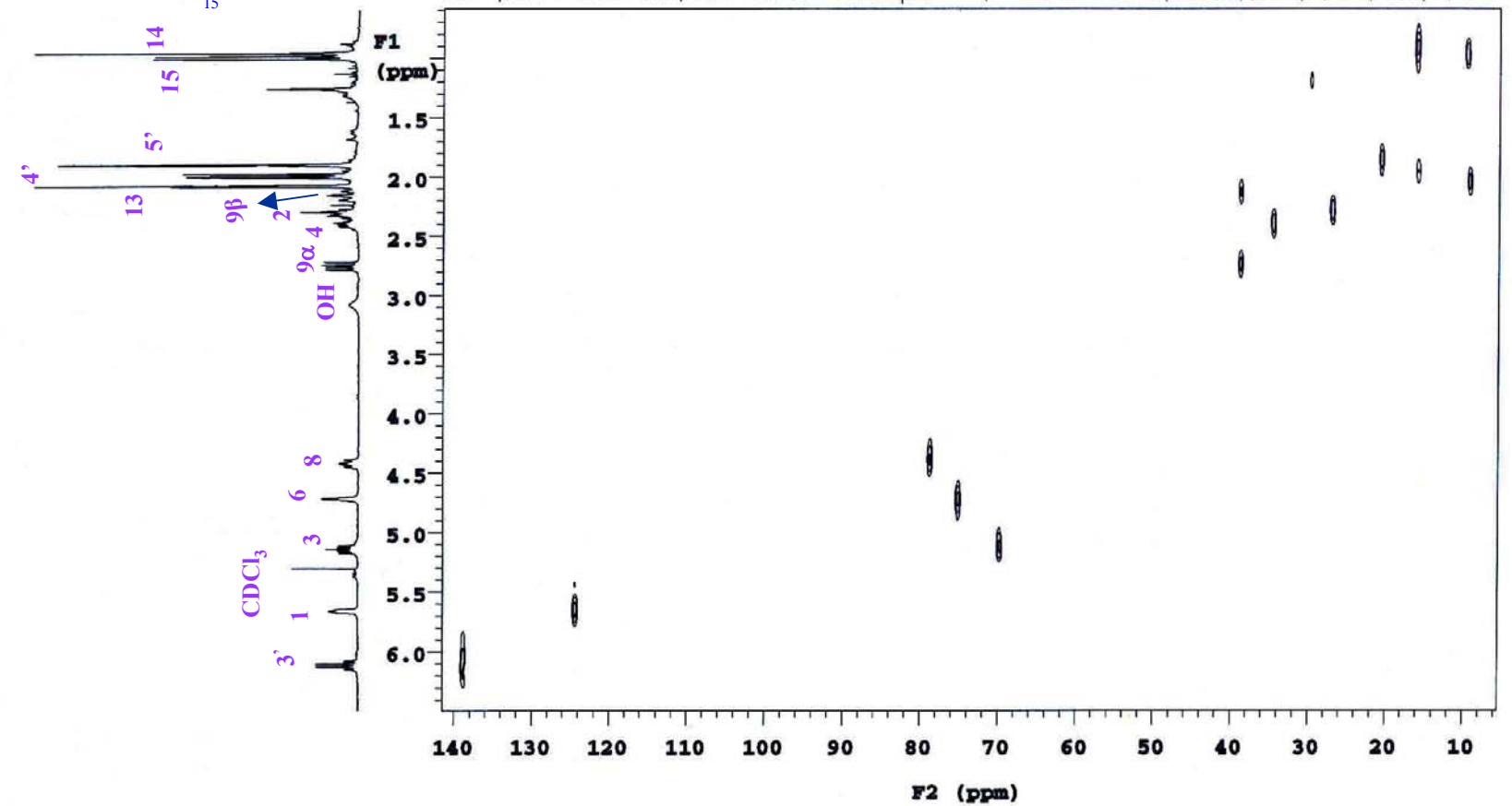
ESPECTRO 2d: Experimento HETCOR del compuesto II
