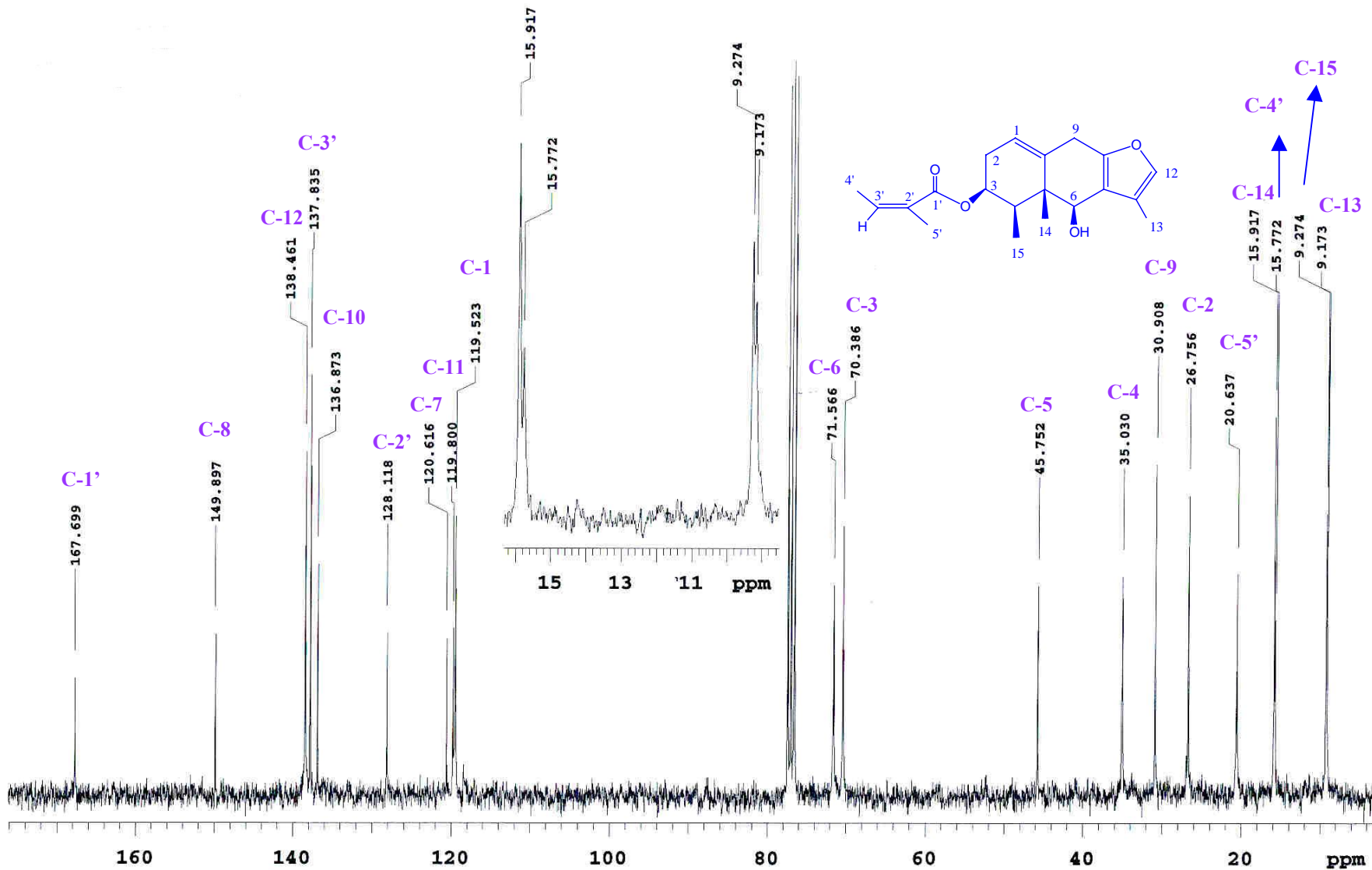
ESPECTRO 1b: RMN- 13 C del compuesto I
