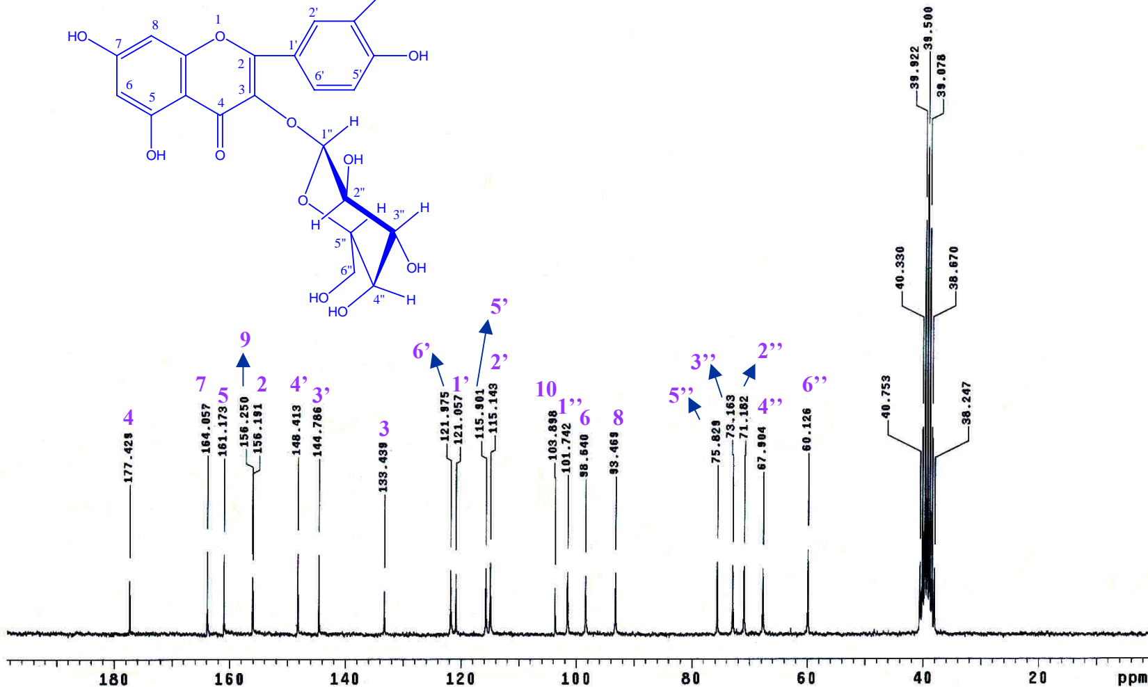
ESPECTRO 5b:RMN- 13 C del Galactósido de Quercetina
