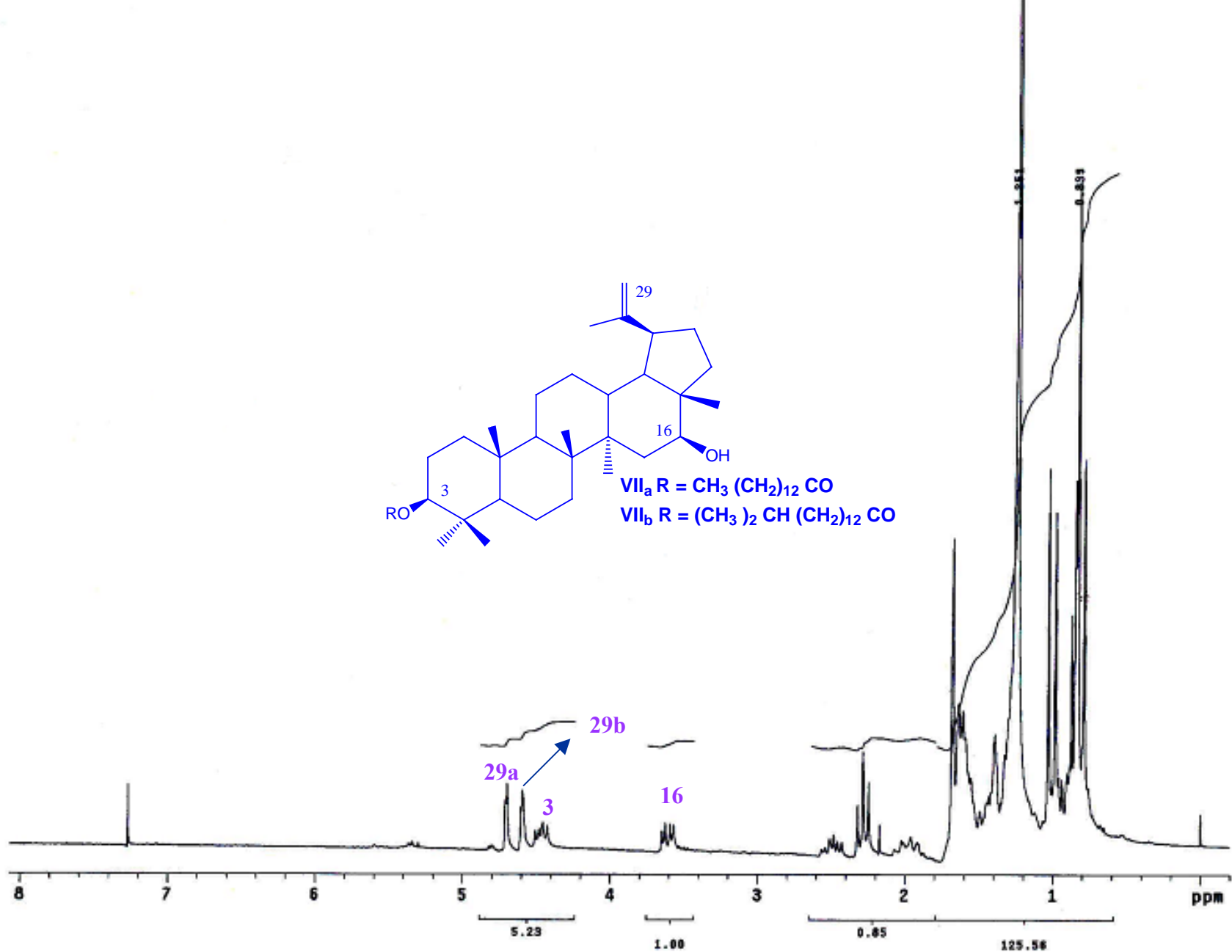
ESPECTRO 4a: RMN- 1 H del compuesto VII
