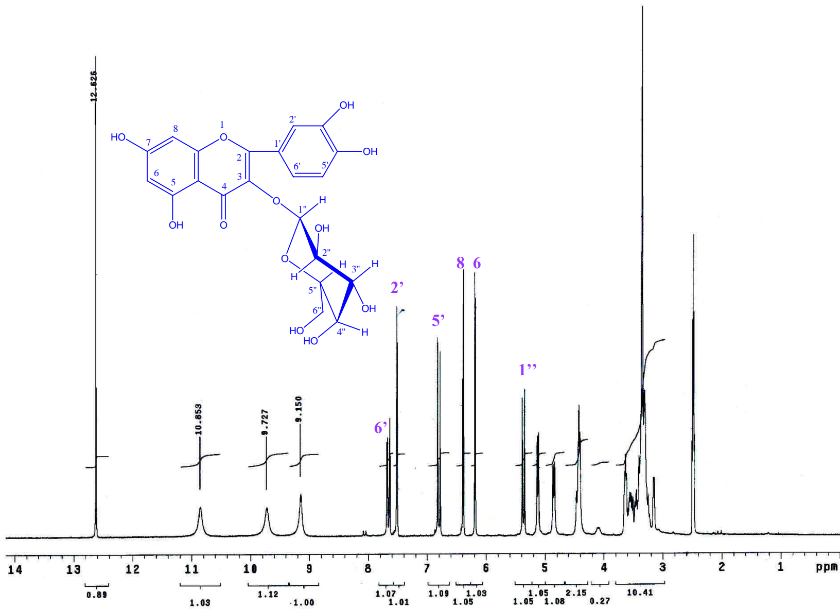
ESPECTRO 5a: RMN- 1 H del compuesto VIII
