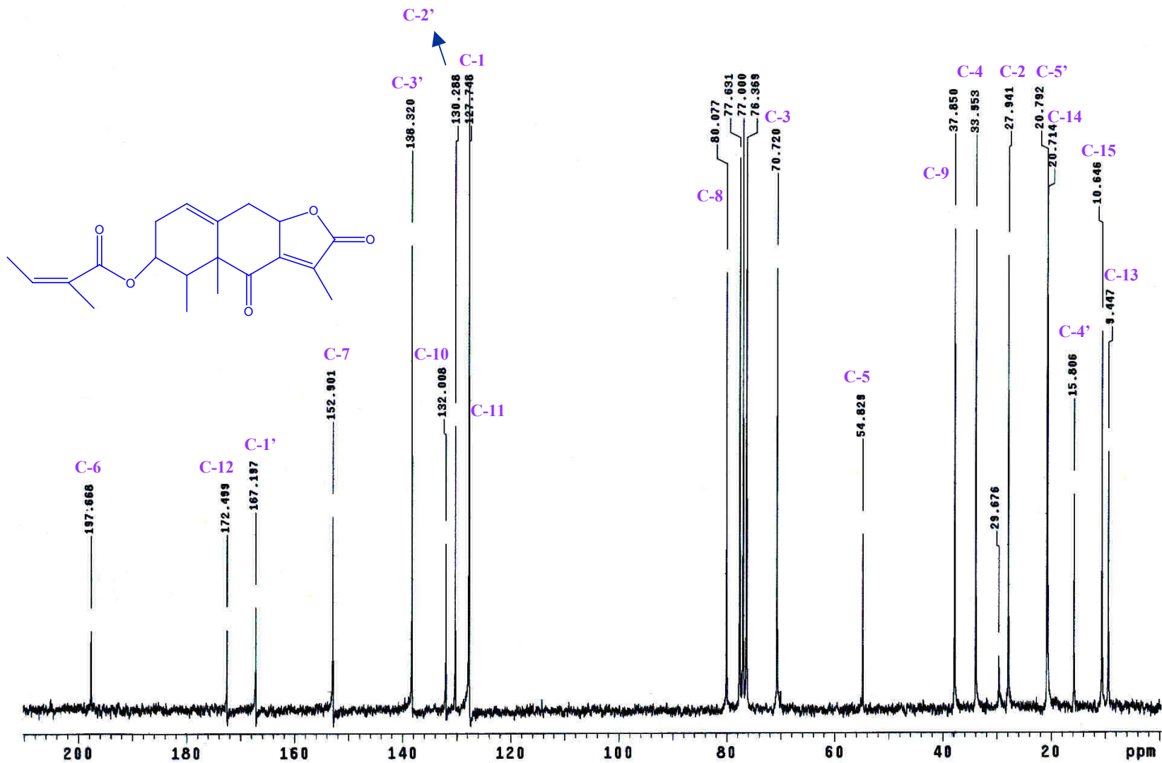
ESPECTRO 10b: RMN- 13 C del compuesto XIII
