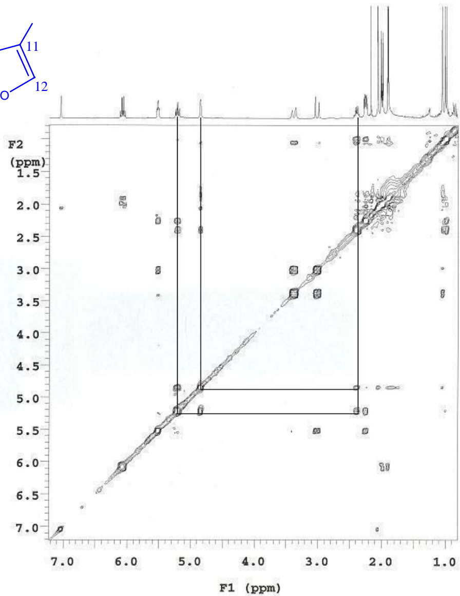
ESPECTRO 1d: Experimento NOESY del compuesto I
