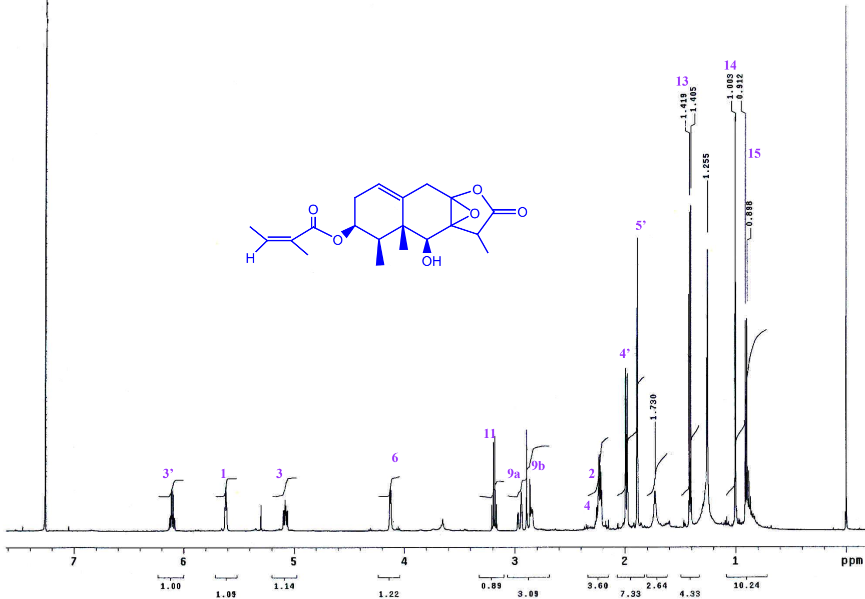
ESPECTRO 9a: RMN- 1 H del compuesto XII
