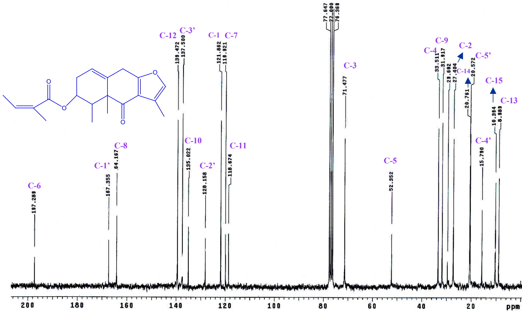
ESPECTRO 7b: RMN- 13 C del compuesto X
