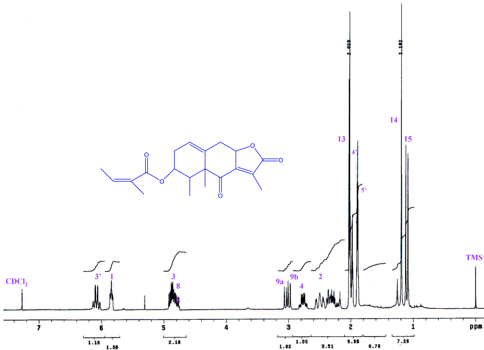
ESPECTRO 10a: RMN- 1 H del compuesto XIII
