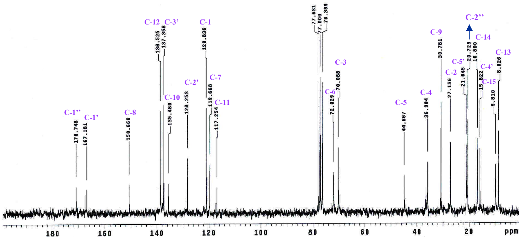
ESPECTRO 8b: RMN- 13 C del compuesto XI
