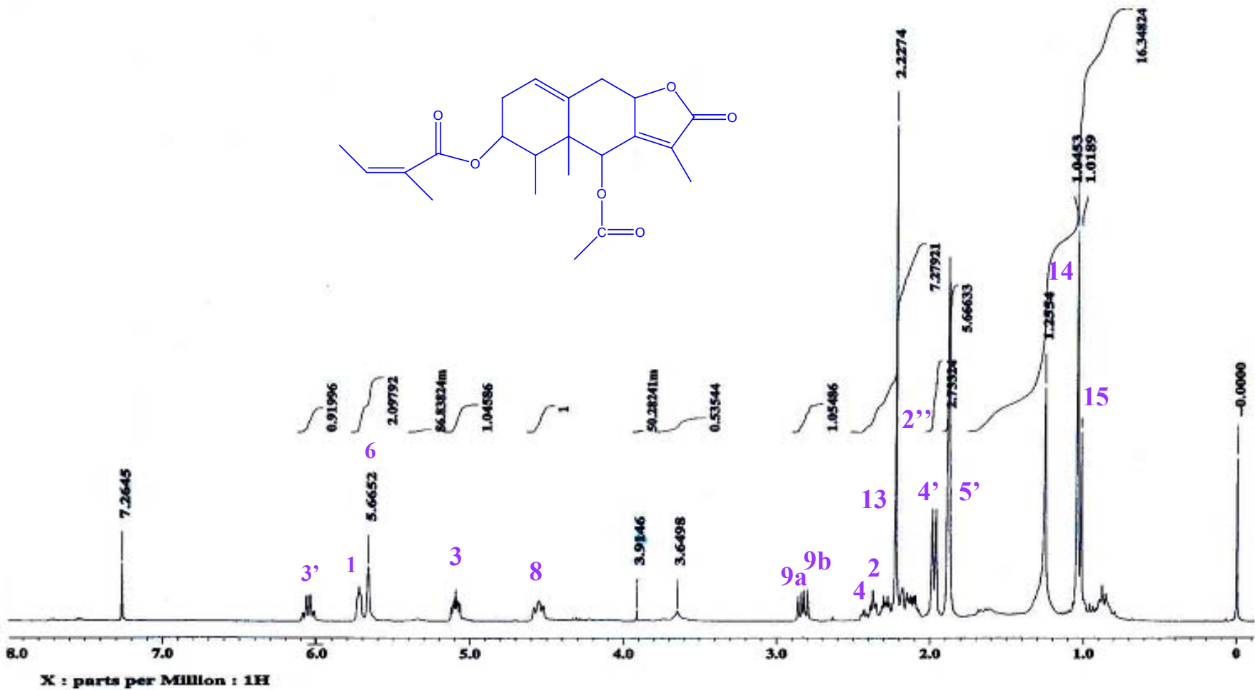
ESPECTRO 11a: RMN- 1 H del compuesto XIV
