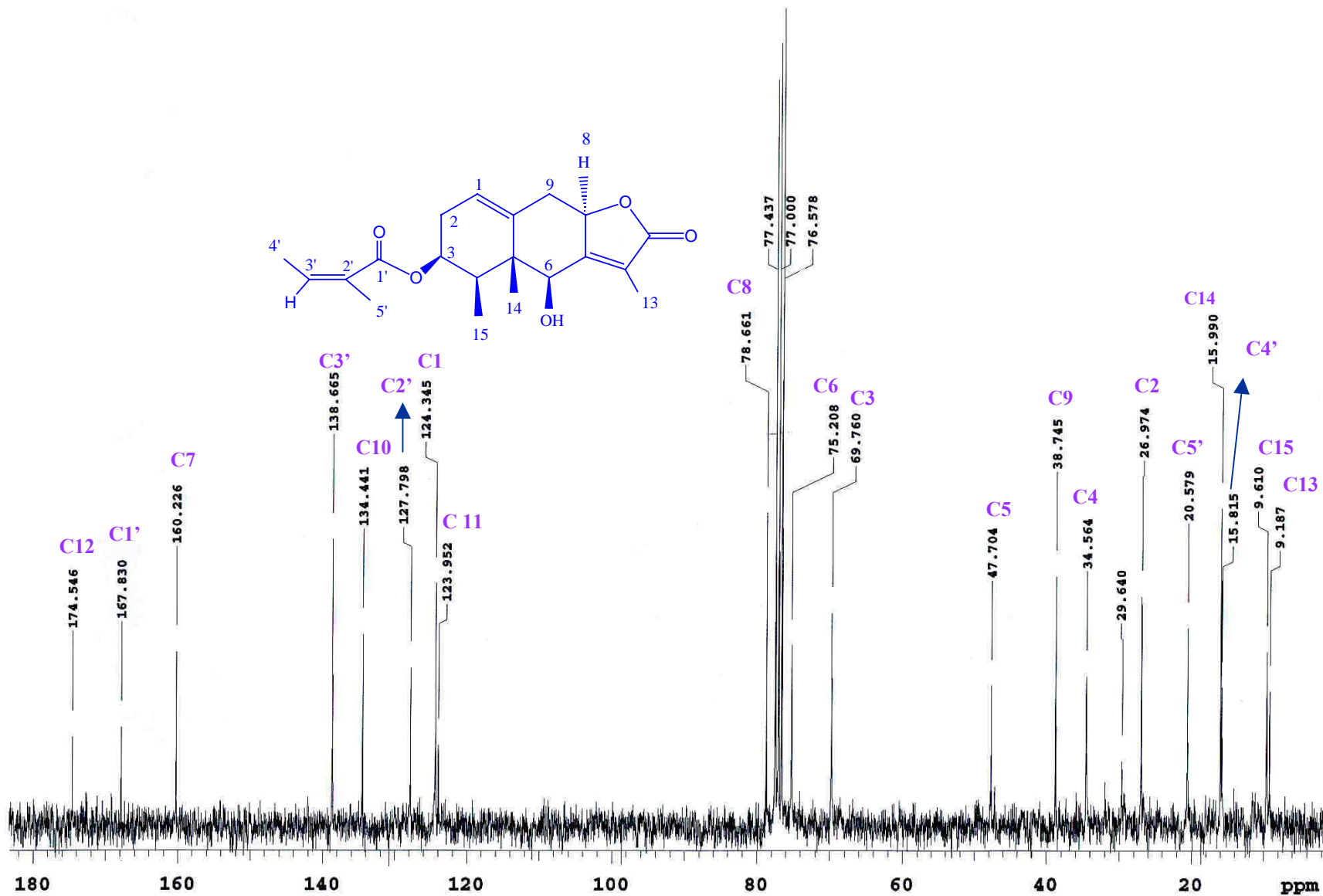
ESPECTRO 2b: RMN- 13 C del compuesto II
