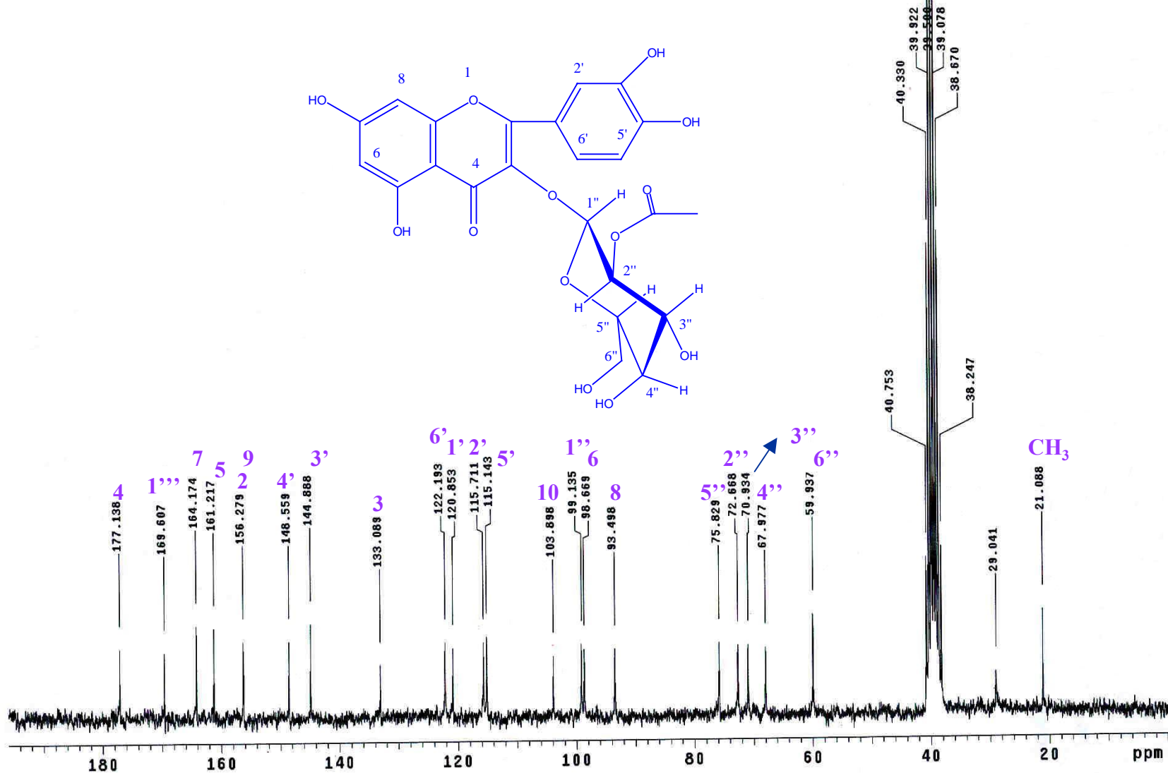
ESPECTRO 6b: RMN- 13 C del compuesto IX
