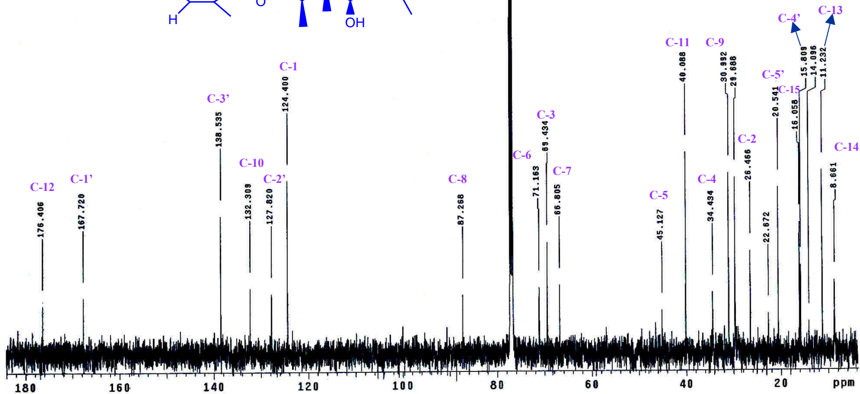
ESPECTRO 9b: RMN- 13 C del compuesto XII
