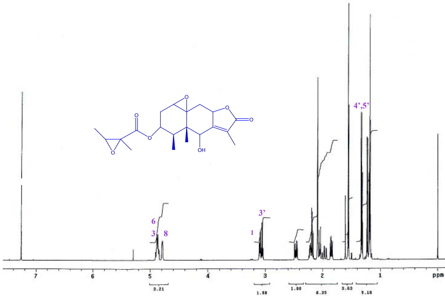
ESPECTRO 14a: RMN- 1 H de la mezcla de estereoisómeros XVI
