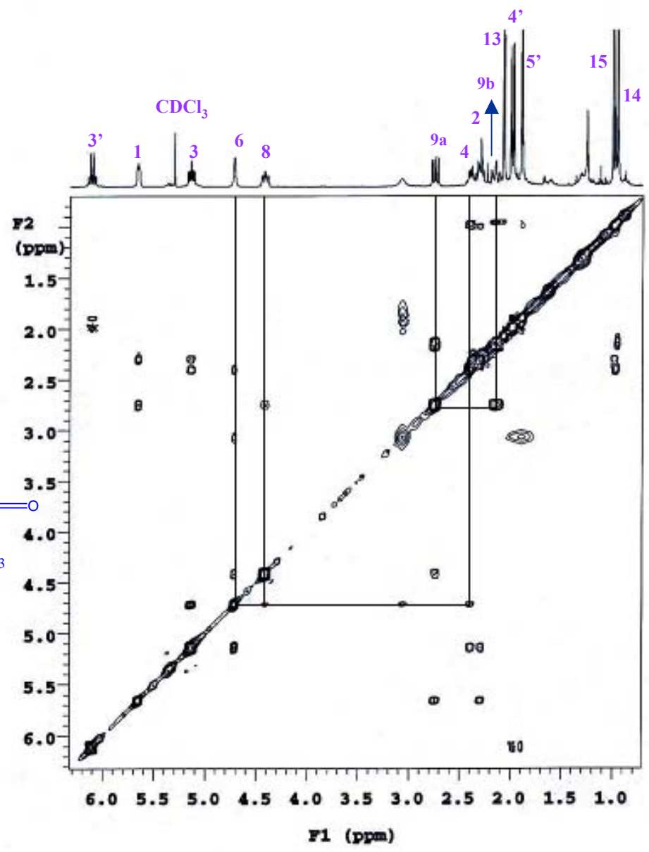
ESPECTRO 2e: Experimento NOESY del compuesto II
