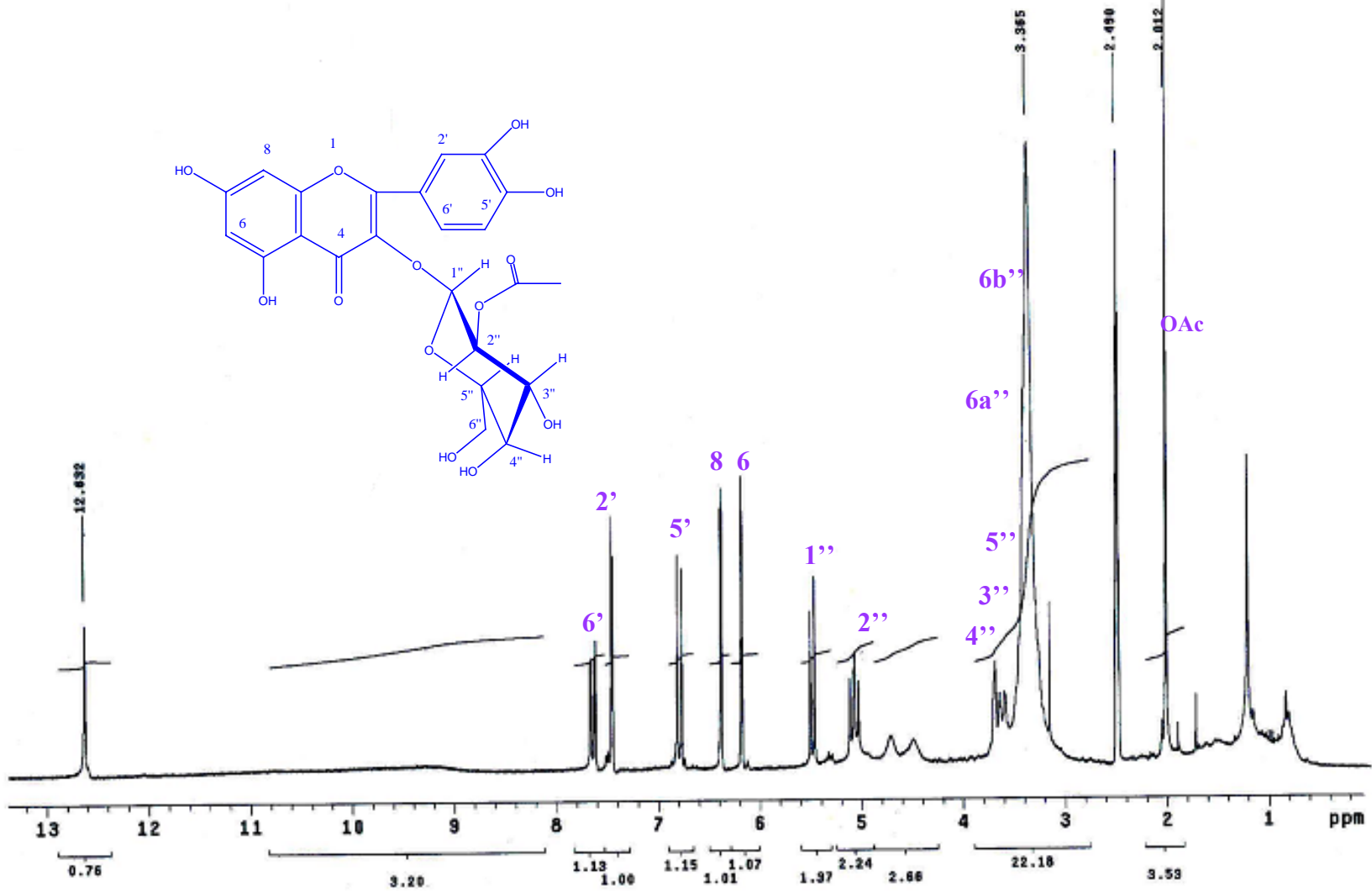
ESPECTRO 6a: RMN- 1 H del compuesto IX
