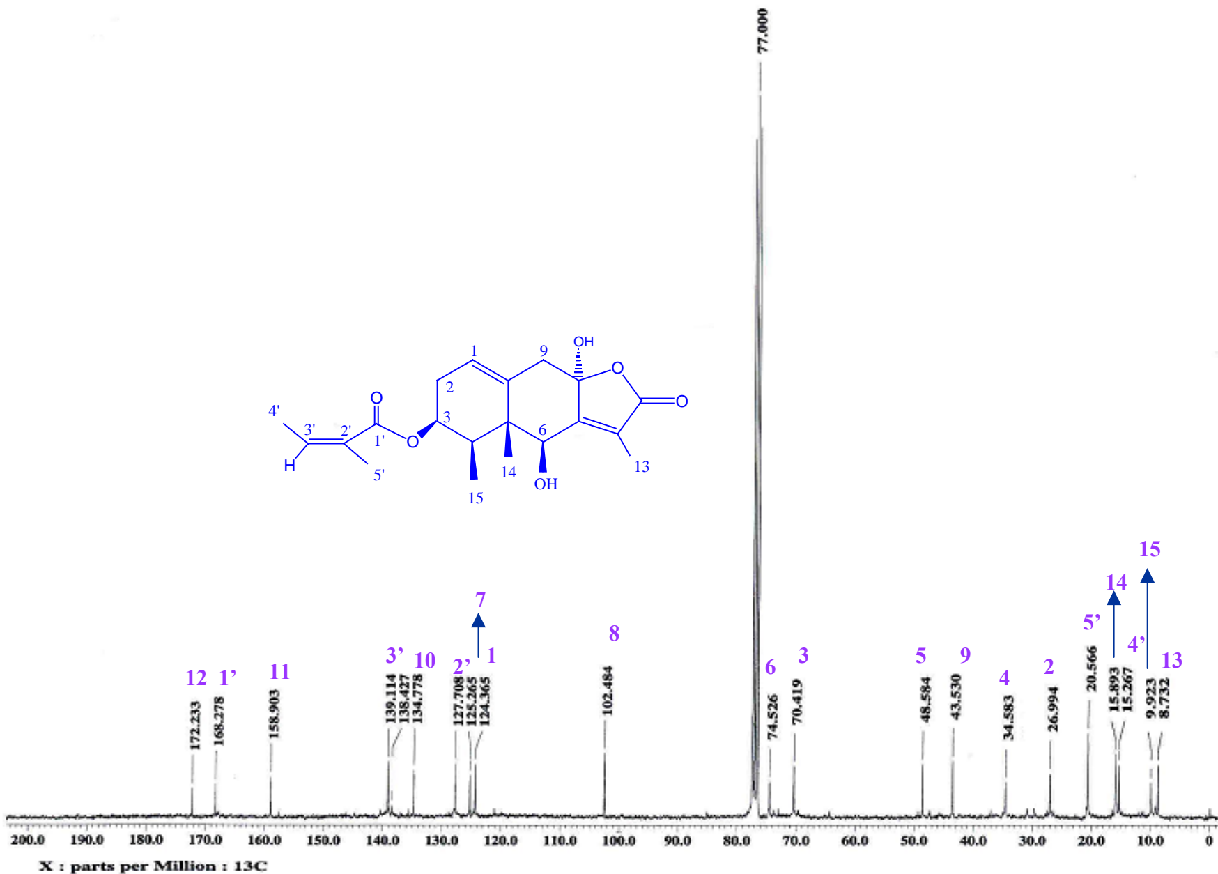
ESPECTRO 3b: RMN- 13 C del compuesto III
