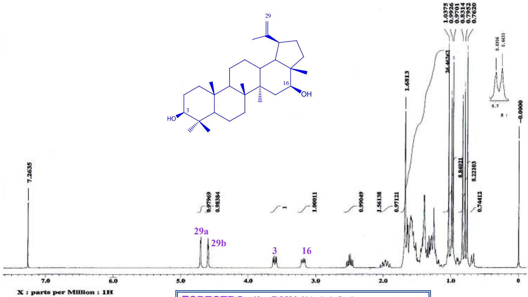
ESPECTRO 4b: RMN- 1 H del Calenduladiol
