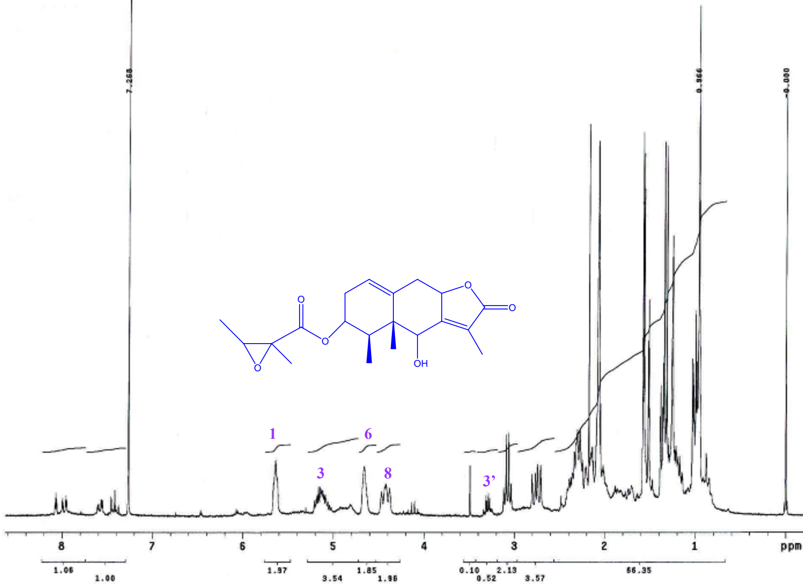
ESPECTRO 12a: RMN- ^1\text{H} de la mezcla de estereoisómeros XV
