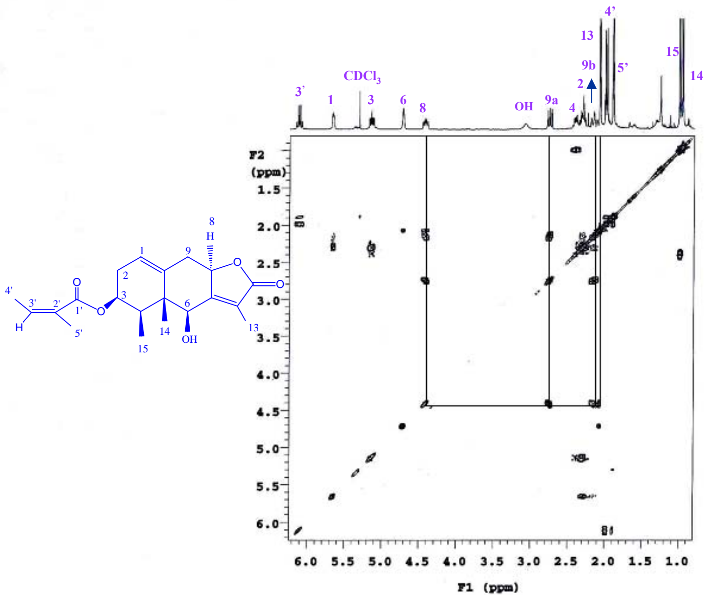
ESPECTRO 2c: Experimento COSY del compuesto II
