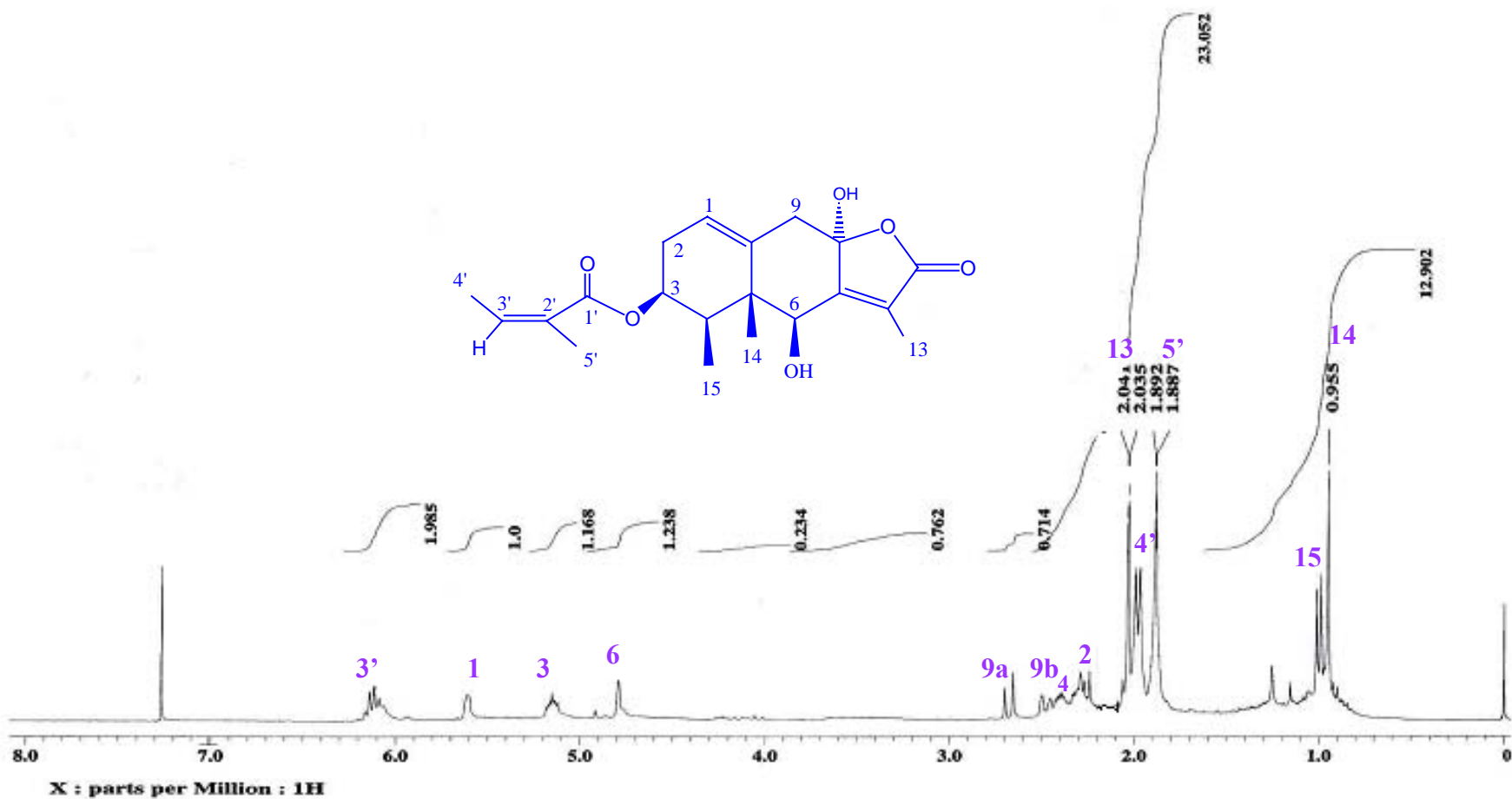
ESPECTRO 3a: RMN- 1 H del compuesto III
