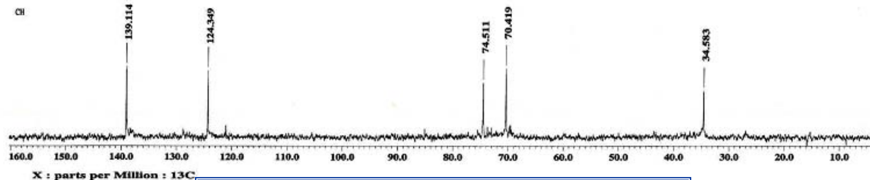
ESPECTRO 3d: Experimento DEPT del compuesto III
