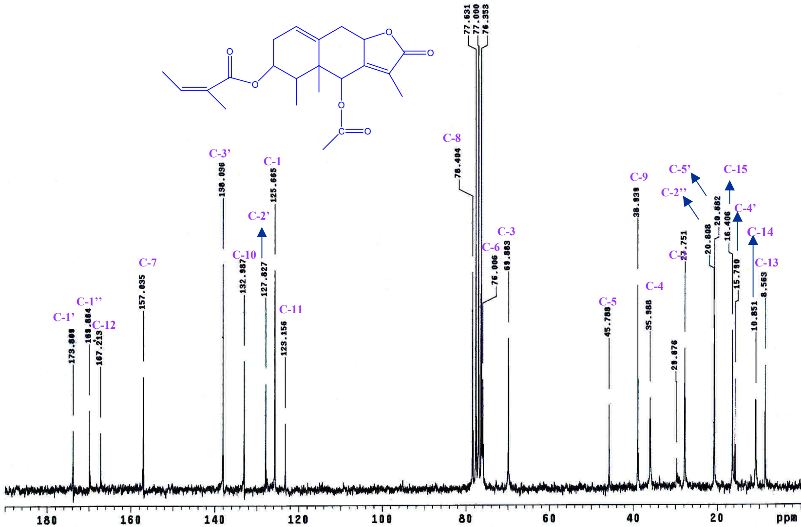
ESPECTRO 11b: RMN- 13 C del compuesto XIV
