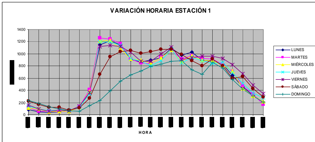
Figura 3.7.8. Gráfica resumen de variación horaria para una estación de aforo
