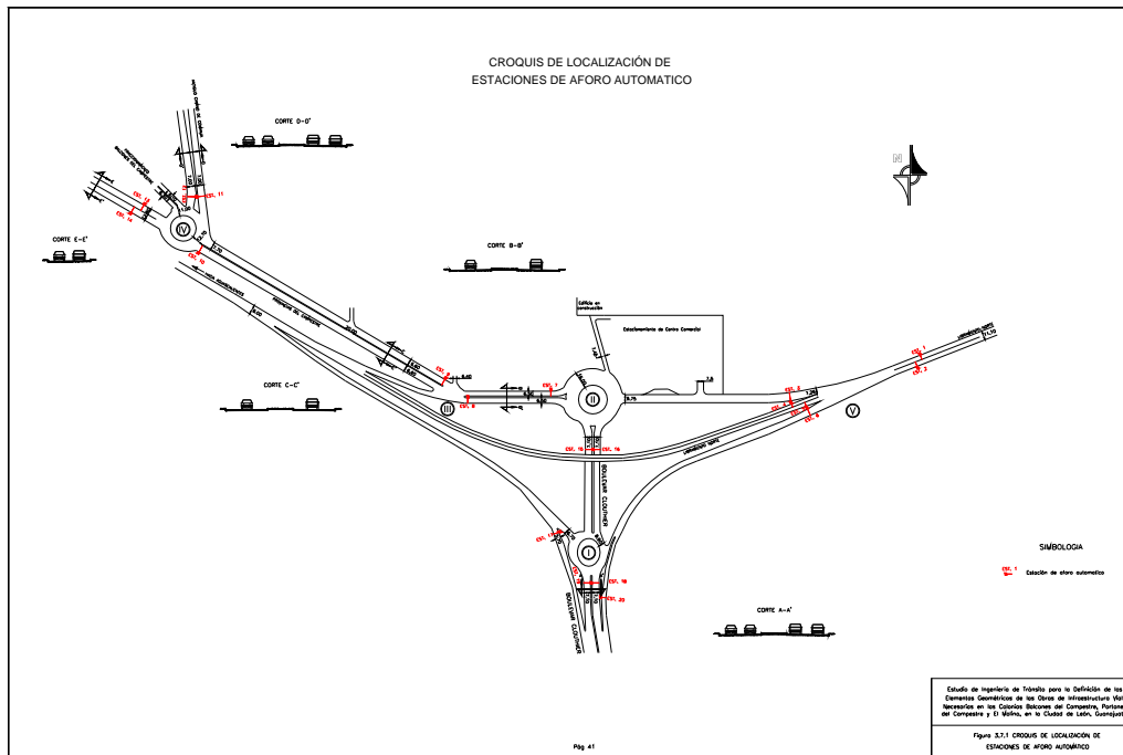
FIG. 3.7.1. Localización de Estaciones de Aforo automático
