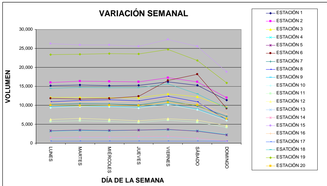
Figura 3.7.9. Variación semanal para las 20 estaciones de aforo
