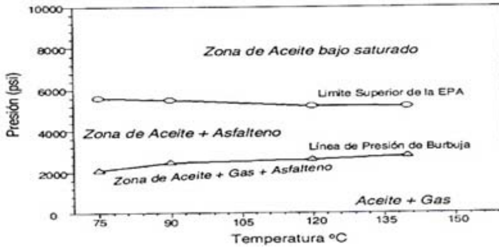
Figura 5.5 Envoltorio de precipitación de asfaltos (Buenrostro, 2002) 5 .
