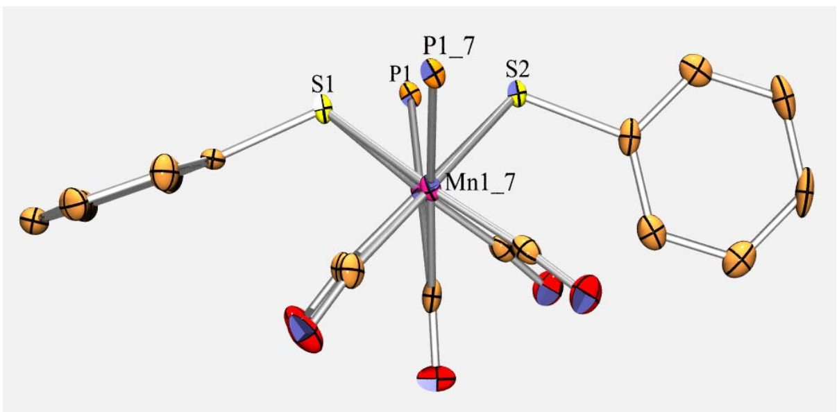
Compuesto 3
