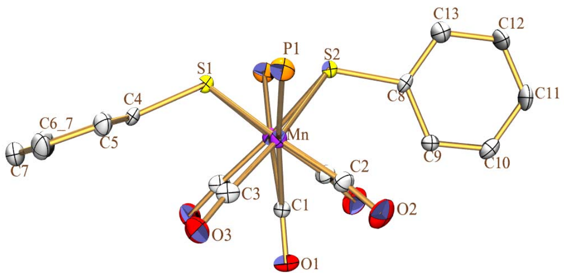
Compuesto 6
