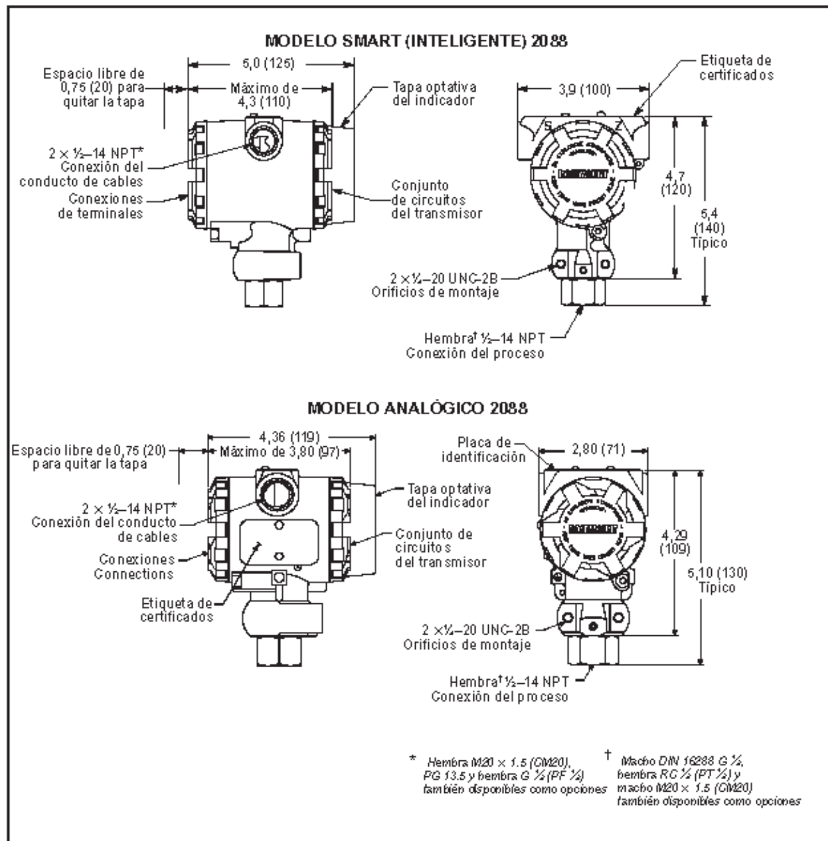
FIGURA 3. Dibujos acotados del transmisor.
