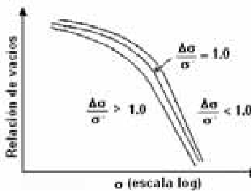
Figura 2.38 Efecto de la relación de esfuerzos en curvas de compresibilidad.
