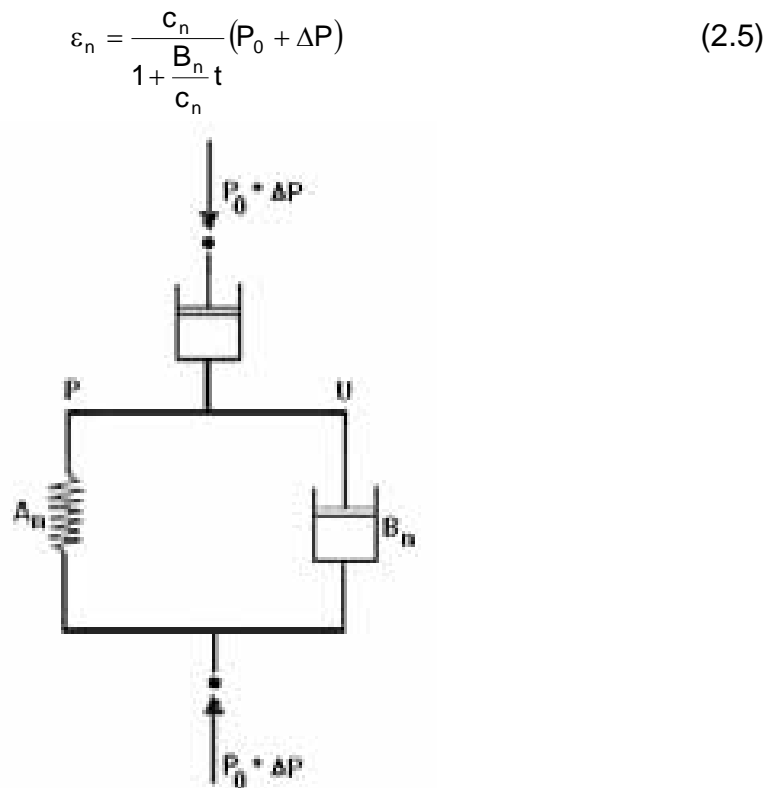
Figura 2.10 Modelo reológico de Wahls 1962
