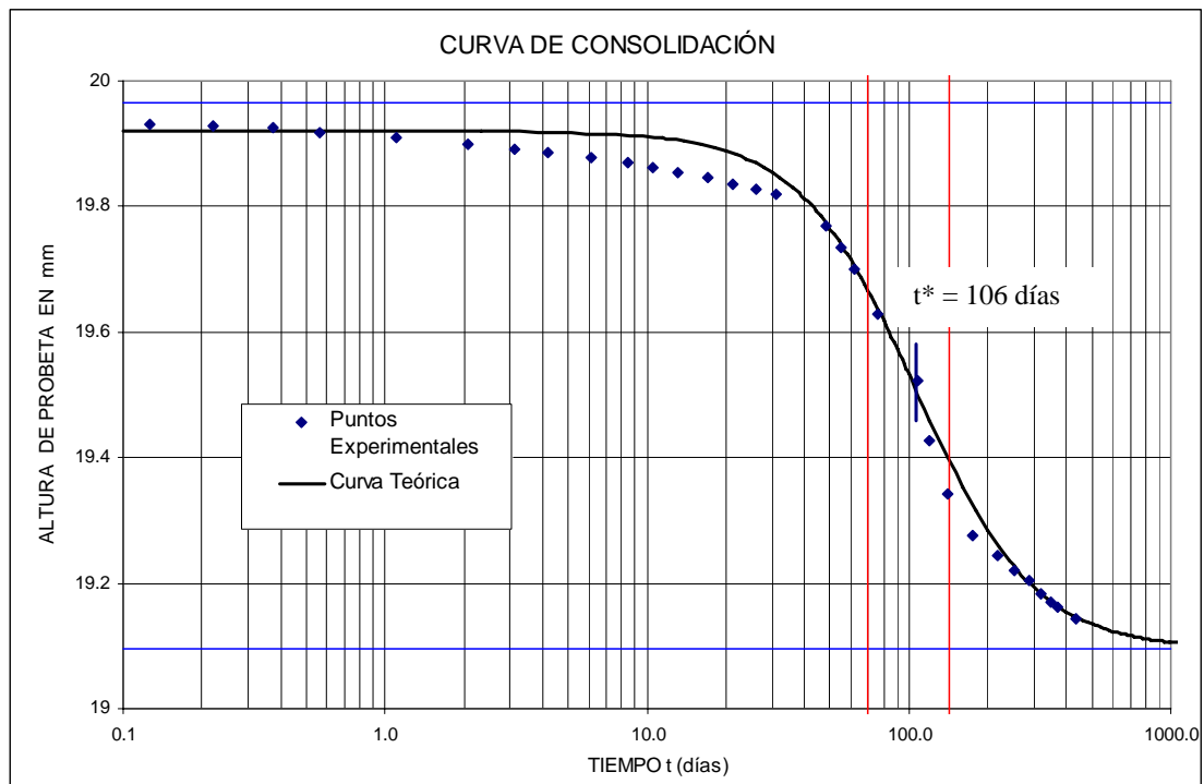
Figura 5.9 Trazo de la curva de consolidación en función de la altura de probeta ensayo E01.
