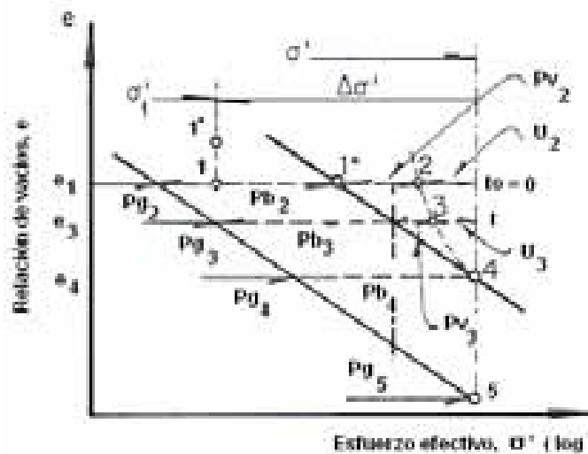
Figura 2.3 Componentes del esfuerzo efectivo según Taylor
