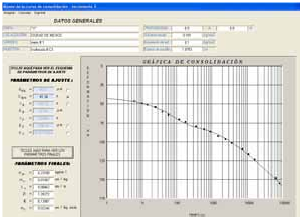
Figura A.3 Ajuste de curva de consolidación, incremento 3
