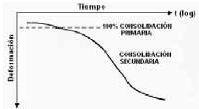
Figura 2.42 Curva de donde predomina el efecto secundario
