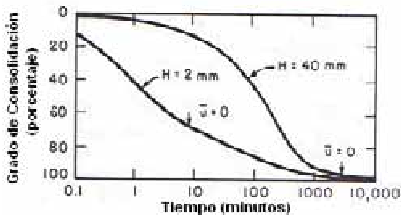
Figura 2.28 Gráficas de consolidación representando la influencia de la distancia de drenaje y la presencia de la consolidación secundaria. Barden (1965).
