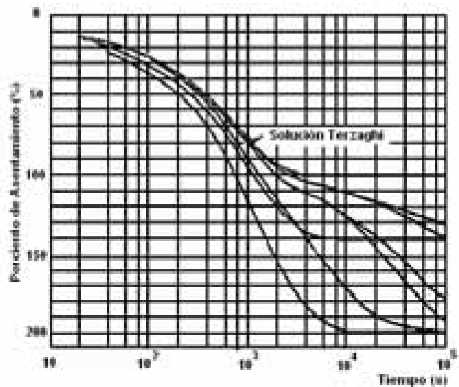
Figura 2.4 Curvas obtenidas por Tan.
