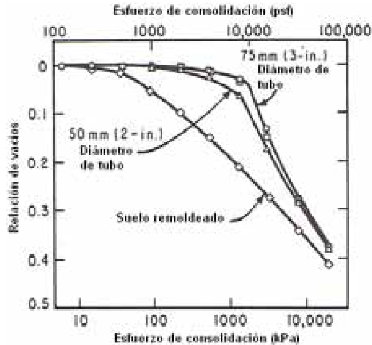
Figura 2.27 Curvas de compresibilidad para diferentes muestreadores
