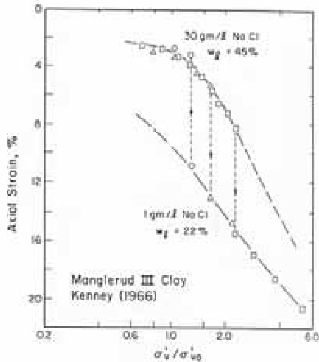
Figura 2.50 Efecto de lixiviado de sal durante la consolidación de la arcilla Manglerud III, Kenney (1966).
