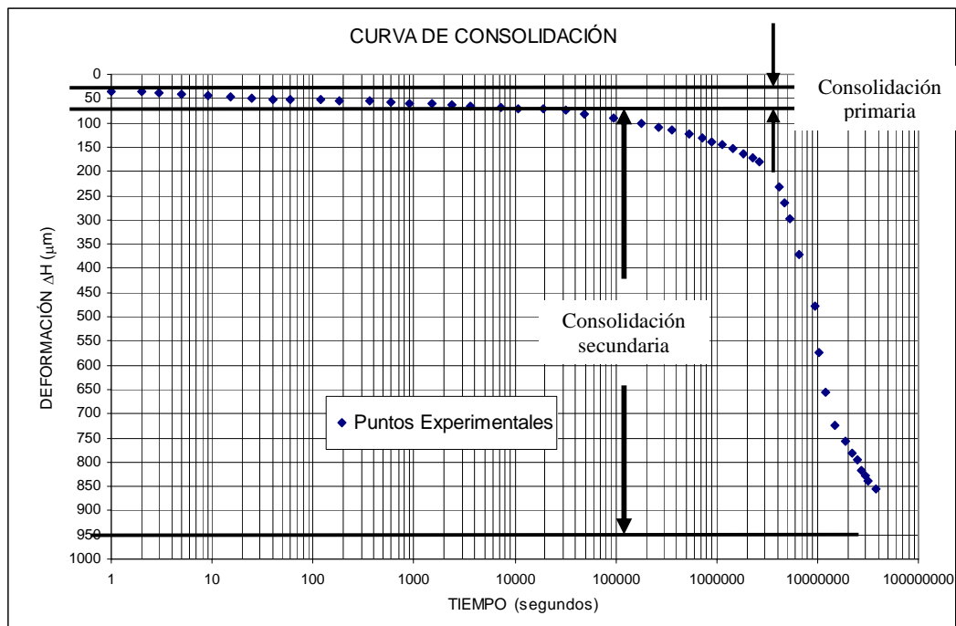
Figura 5.5 Magnitudes de consolidación primaria y secundaria en la prueba a largo plazo para el ensayo E01.
