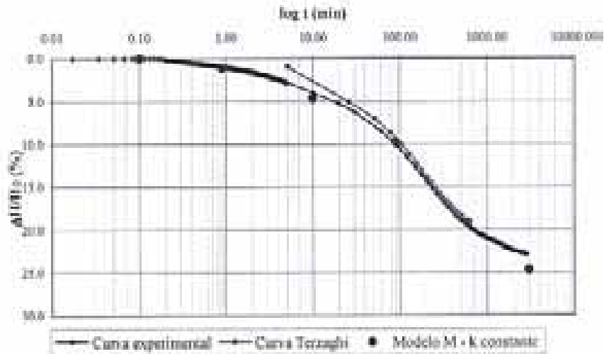
Figura 2.27 Curva de consolidación para una carga aplicada cercana al esfuerzo de preconsolidación, ajustada por los modelos Terzaghi y Alberro.
