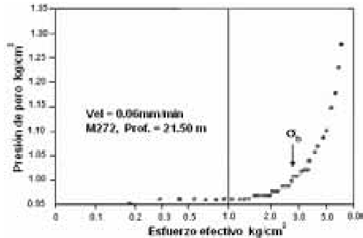
Figura 2.35 Gráfica Presión de poro vs. Esfuerzo efectivo
