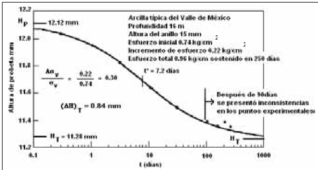
Figura 3.16. Arcilla típica del Valle de México, Cambio de altura del espécimen probado durante 250 días.
