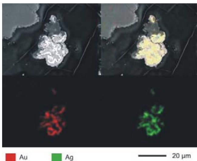
Fig. 21 Imágenes de microscopio electrónico de barrido. La fotografía en el recuadro superior izquierdo muestra el aspecto de una partícula mixta de dos fases auro-argentíferas intercrecidas. El recuadro superior derecho muestra la distribución de Au y Ag en la partícula, los recuadros inferiores muestran la distribución de cada elemento por separado.
