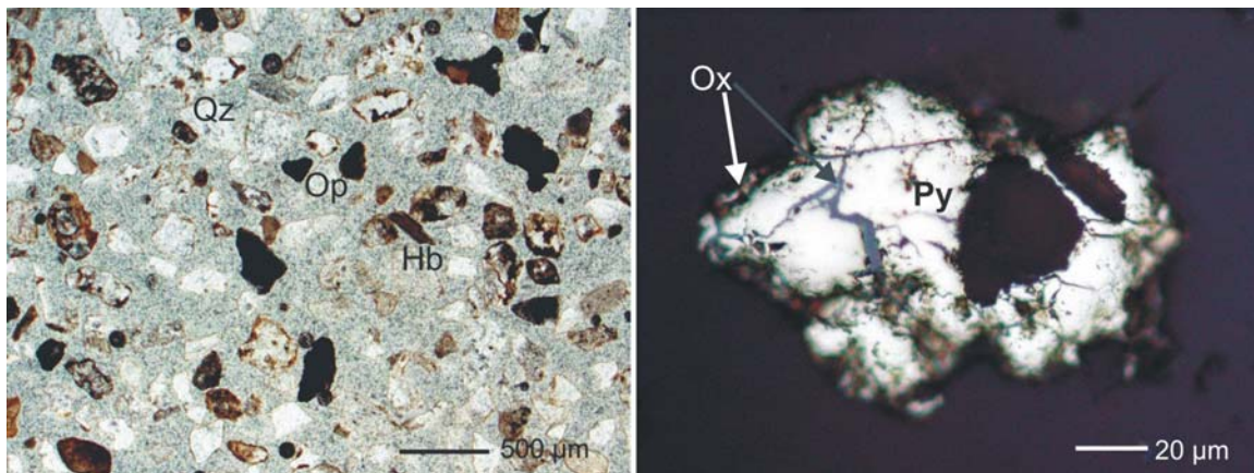
Fig. 17 Fotomicrografías de la muestra del horizonte E4H2. A la izquierda, vista general de la muestra donde se observa la mineralogía dominante y los aspectos texturales generales (microscopio petrográfico con luz paralela y objetivo 2x). A la derecha, partícula de pirita que exhibe bordes de corrosión por remplazamiento de oxihidróxidos de Fe y remplazamiento de las mismas fases a través de fracturas (microscopio minerográfico con luz paralela y objetivo de 50x).
