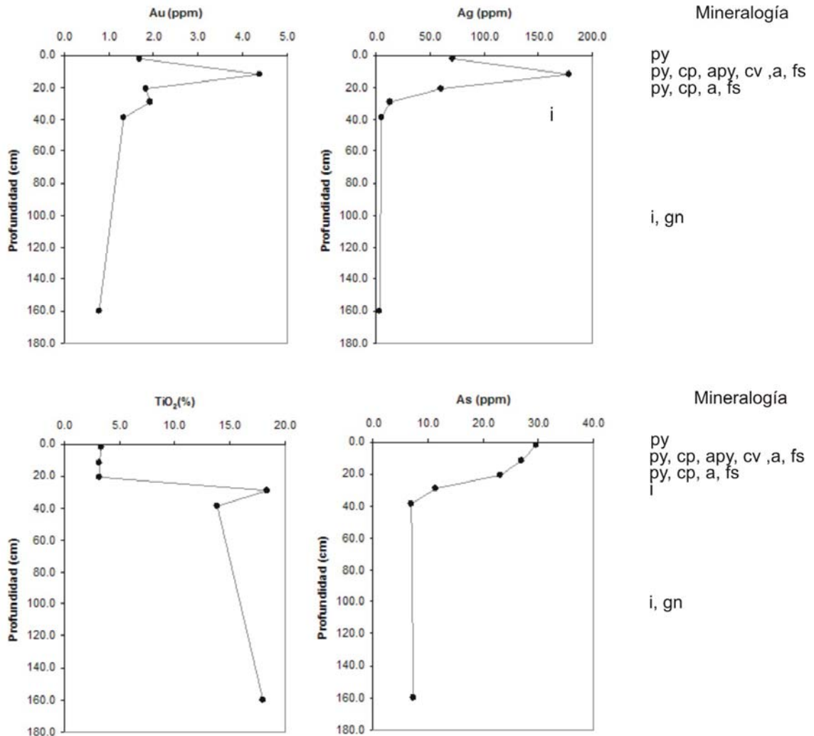
Fig. 30 Gráficas que muestran la concentración de Au, Ag, Ti y As respecto a la profundidad en el perfil E3, así como la mineralogía presente. Se observa la relación directa entre las fases minerales opacas y el la abundancia relativa del elemento químico correspondiente. py= pirita, gn=galena, i=ilmenita, apy=arsenopirita, cp=calcopirita, a=aguilarita, fr=freibergita, cv=covelita.
