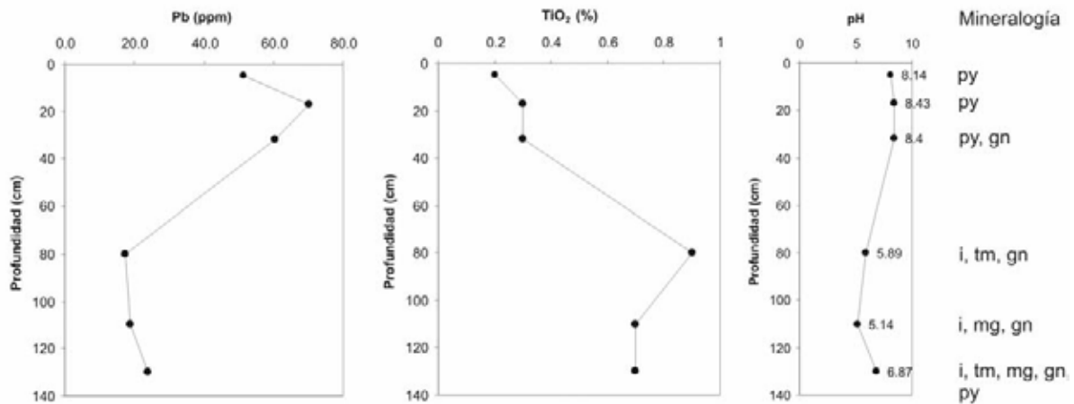
Fig. 33 Gráficos que muestran la concentración de Pb y Ti, el valor de pH y la mineralogía presente respecto a la profundidad en el perfil E3. py= pirita, gn=galena, i=ilmenita, tm=titanomagnetita, mg=magnetita.
