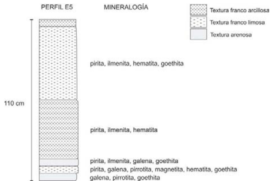
Fig. 18 Representación del perfil E5 que muestra la distribución vertical de los minerales presentes.
