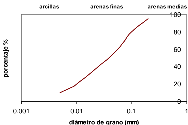
Fig. 2 Curva que muestra la distribución del tamaño de grano en los jales (modificada de Robertson, 1994; Younger et al., 2002)
