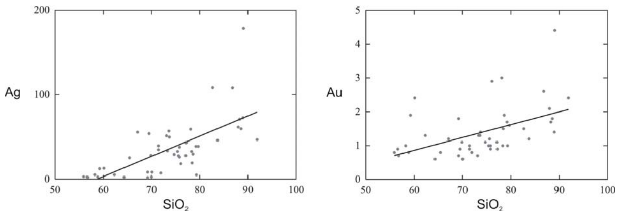
Fig. 32 Relación química del contenido de Au y Ag (ppm) respecto a \text{SiO}_2 (%) en análisis de muestra total por ICP-MS, la tendencia es coherente con la relación textural identificada entre los metales preciosos y el cuarzo.
