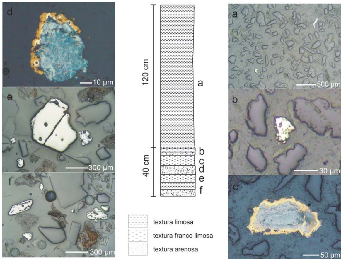
Fig. 26 Esquema sintético que muestra los diferentes horizontes del perfil E7 y las variaciones mineralógicas verticales identificadas. a) aspecto general de la parte superior del perfil donde se aprecia la poca cantidad de partículas minerales opacas las cuales consisten en pirita, hematita y goethita (microscopio mineragráfico con luz paralela). b) partícula de pirita característica de los niveles intermedios del perfil (microscopio mineragráfico con luz paralela). c) partícula mixta perteneciente al horizonte E7H3 constituida por cuarzo, calcopirita, freibergita? y aguilarita que exhibe crecimiento concéntrico en el borde (microscopio mineragráfico con luz paralela). d) partícula mixta similar a la anterior perteneciente al horizonte E7H4, este nivel del perfil se caracteriza por la presencia de distintas fases minerales auro-argentíferas. e) al centro partícula subedral de ilmenita, a la derecha de la ilmenita un fragmento de hematita en tono más claro (microscopio mineragráfico con luz paralela). f) aspecto del nivel inferior del perfil caracterizado por la presencia de ilmenita (fragmento subedral a la izquierda, hematita a la derecha y galena (pequeño fragmento blanco en la parte superior de la fotografía).
