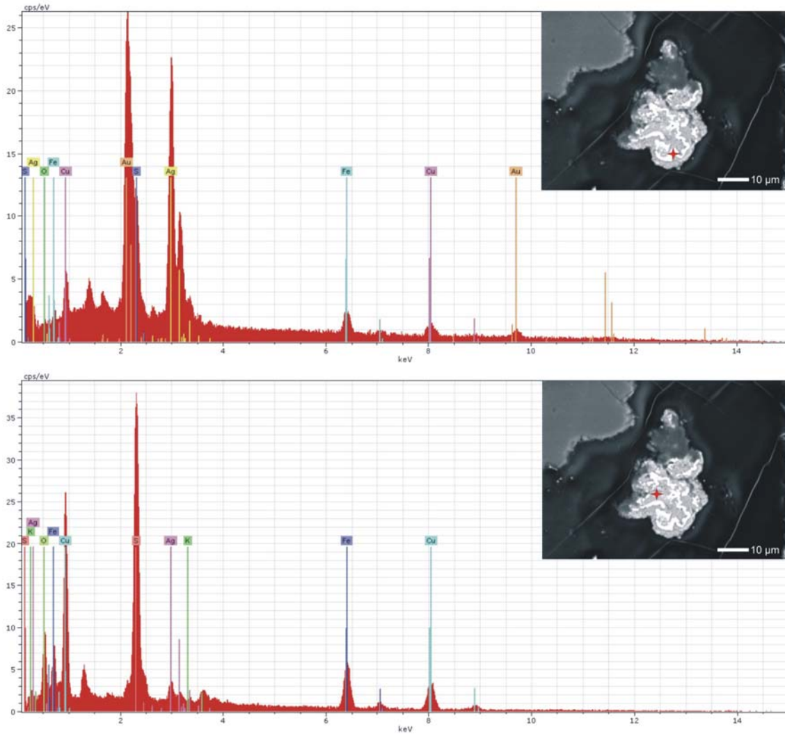
Fig. 22 Espectros de rayos-X de energía dispersiva (EDS) obtenidos para una partícula mixta de dos fases minerales perteneciente a la muestra E7H3. La imagen superior muestra el análisis de una amalgama de oro y plata distribuida en la parte más luminosa de la partícula. La imagen inferior muestra un análisis de freibergita? que presenta enriquecimiento en plata.
