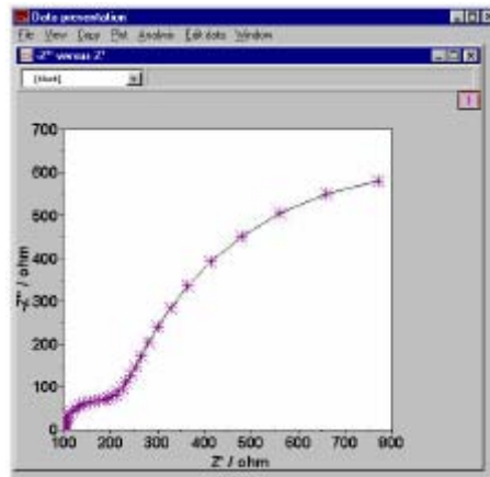
Figura 3.6 Circuito equivalente de un recubrimiento orgánico y su representación en un diagrama de Nyquist.
