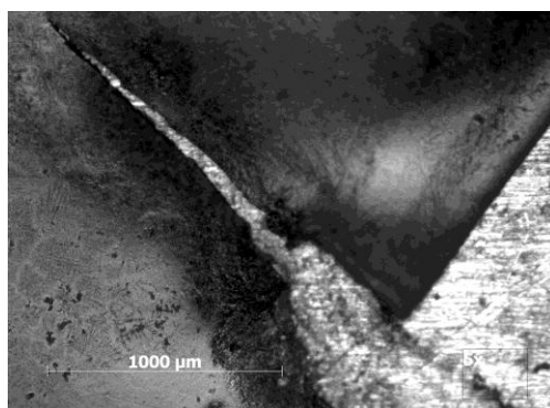
Figura 5.24 Micrografía a 5x. Se observa la ruptura de la pintura, y su corrimiento.
