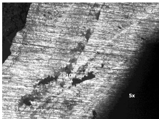
Figura 5.25 Micrografía a 5x. Se observa el sustrato metálico expuesto, debido al desprendimiento de la pintura.
