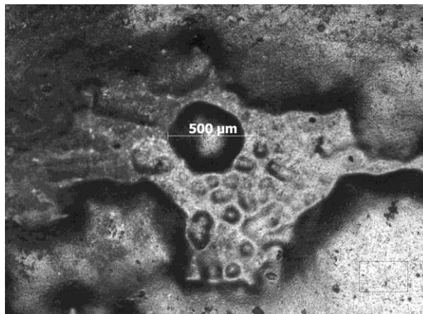
Figura 5.20 Micrografía a 5x. Se observan ampollas de diversos tamaños, que van desde las microscópicas hasta las macroscópicas.
