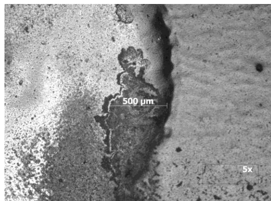
Figura 5.23A Micrografía a 5x. Se pueden observar depósitos de óxido sobre la ampolla, señal de que el sustrato se está oxidando.
