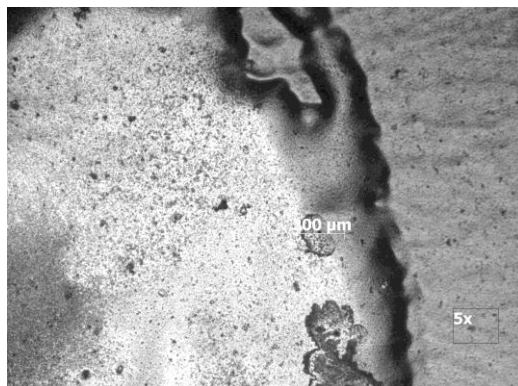
Figura 5.23B Micrografía a 5x. Se pueden observar depósitos de óxido sobre la ampolla.
