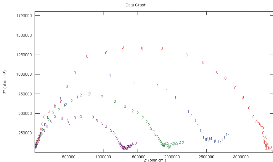
Figura 5.9 Resistencia a la transferencia de carga de los tres primeros ciclos de AC-DC-AC.
