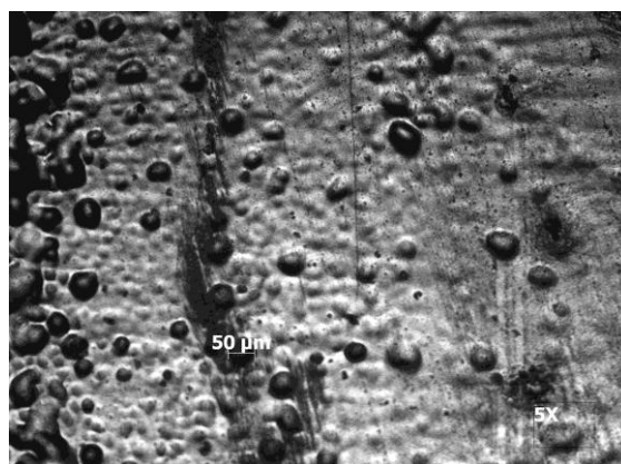
Figura 5.22 Micrografía a 5x. Formación de ampollas.
