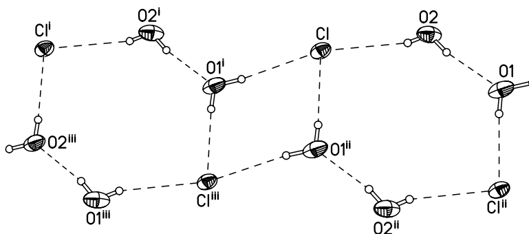
Figura 22. Detalles de la red conformada por moléculas de agua y iones cloruro en el cristal de 24 a través de puentes de hidrógeno. Distancia de enlace H...Cl, 2.793 Å.
