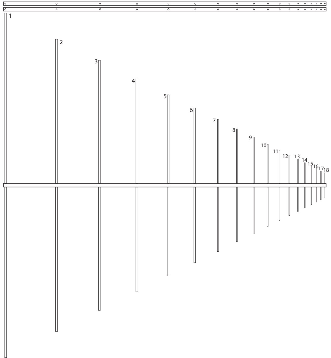
Figura 5.8: Elementos de la antena
