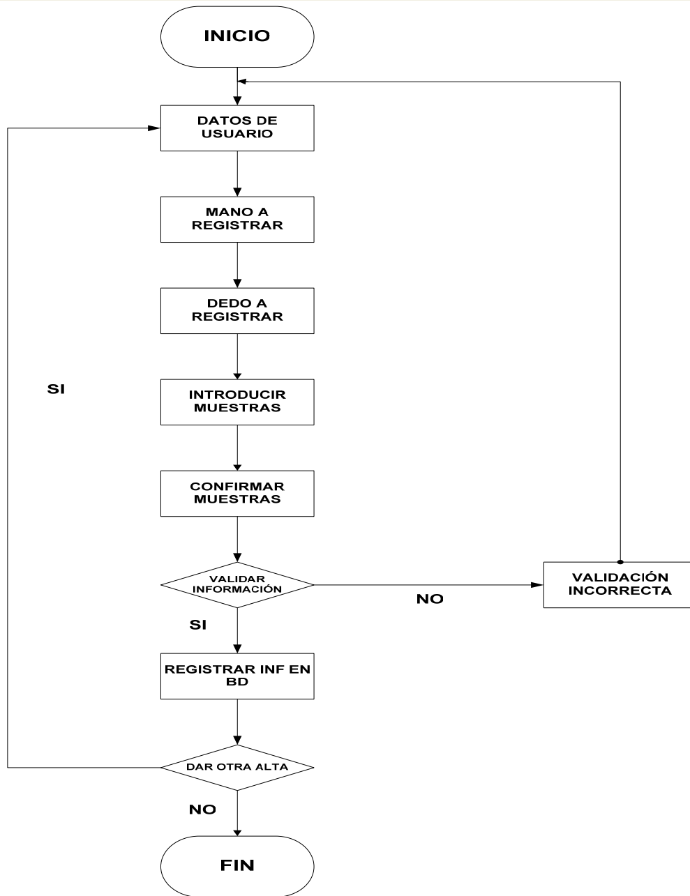
Figura IV.1.2.12 Diagrama de flujo tradicional del reloj checador.
