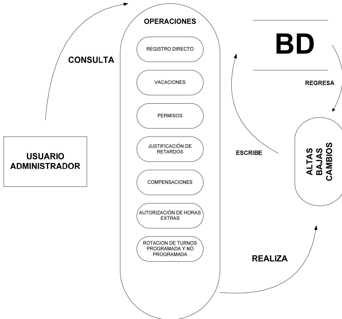
Figura IV.1.2. 8 DFD del ACCYS TIME nivel 3, menú operaciones.
