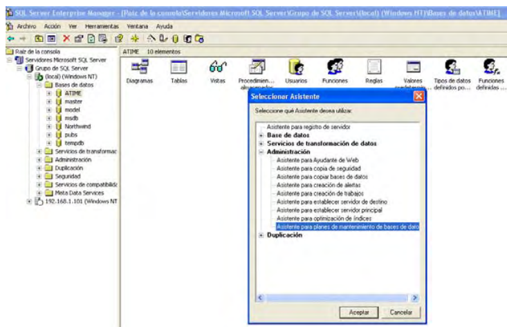
Figura 15. Pantalla de Asistente del Administrador corporativo.
