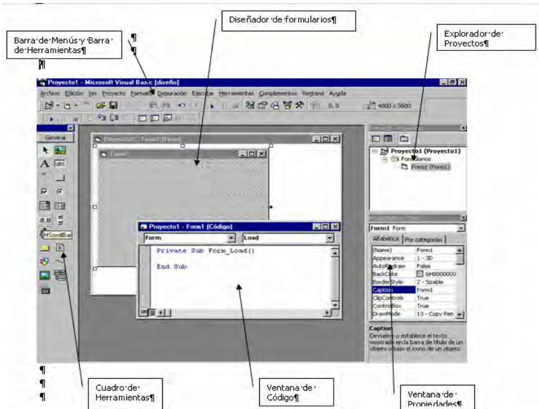
Figura II.5.2 Entorno de trabajo Visual Basic
