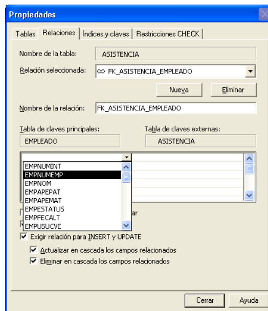
Figura IV.2.1.13 Generando una nueva relación
