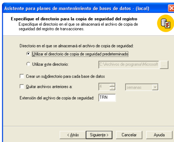
Figura 23. Pantalla de opción para directorio para la copia de seguridad
