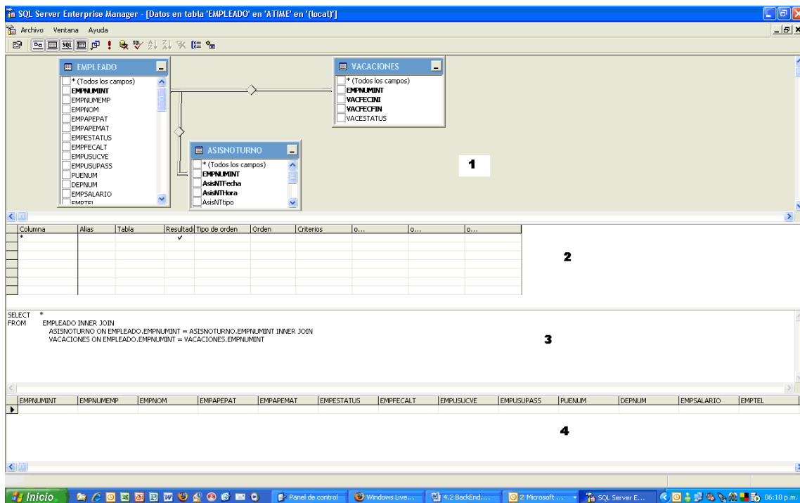
Fig. IV.2.1.9 Creación de los Join. Manipulación de los datos
