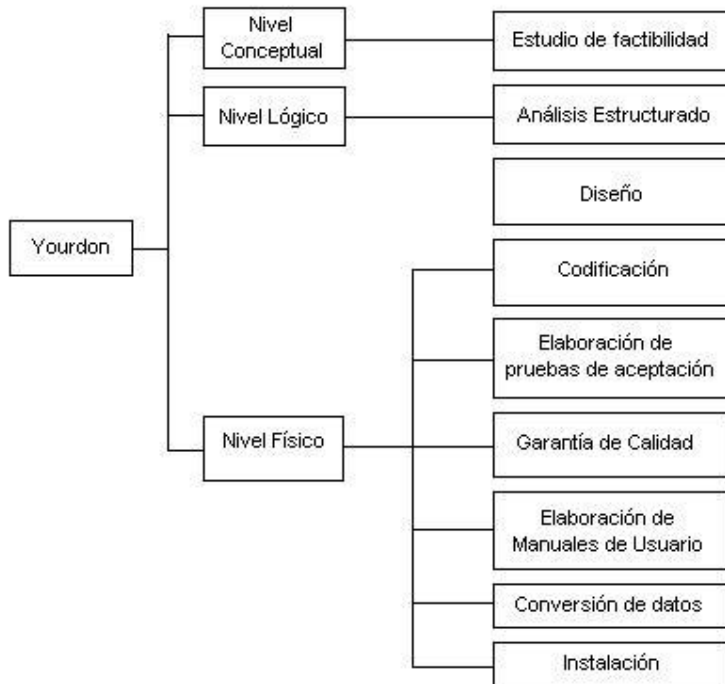
Figura II.1. Diagrama de Yourdon
