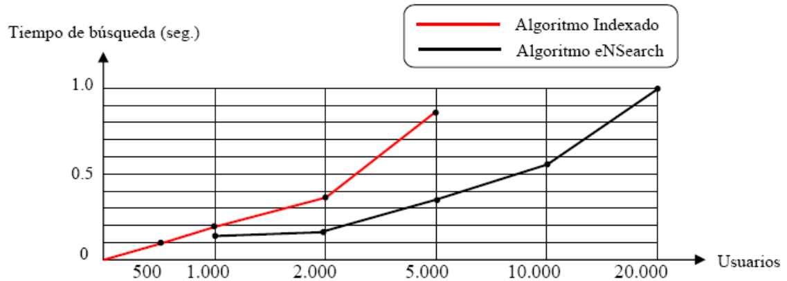
Figura II.2.1 Test sobre Windows 2000, P-III 1GHz y 256MB de RAM.
