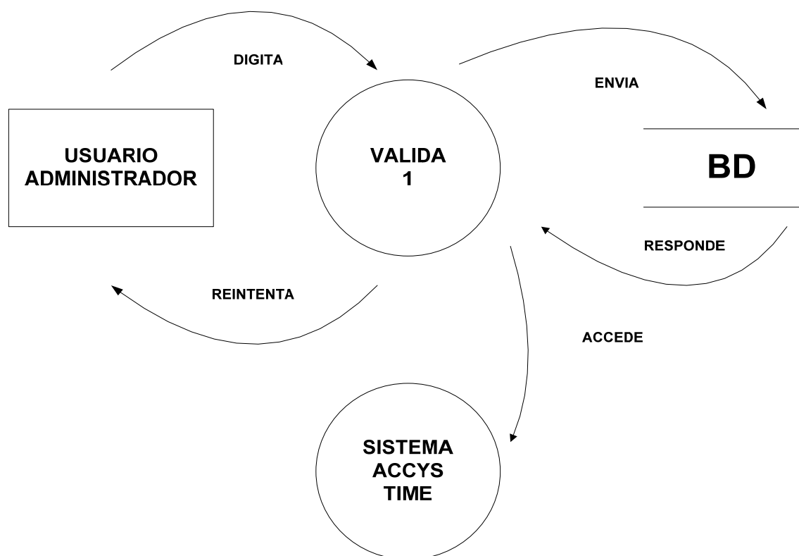
Figura IV.1.2.3 DFD del ACCYS TIME nivel 1.
