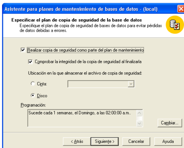
Figura 20. Opciones para le plan de copia de seguridad de la base de datos.
