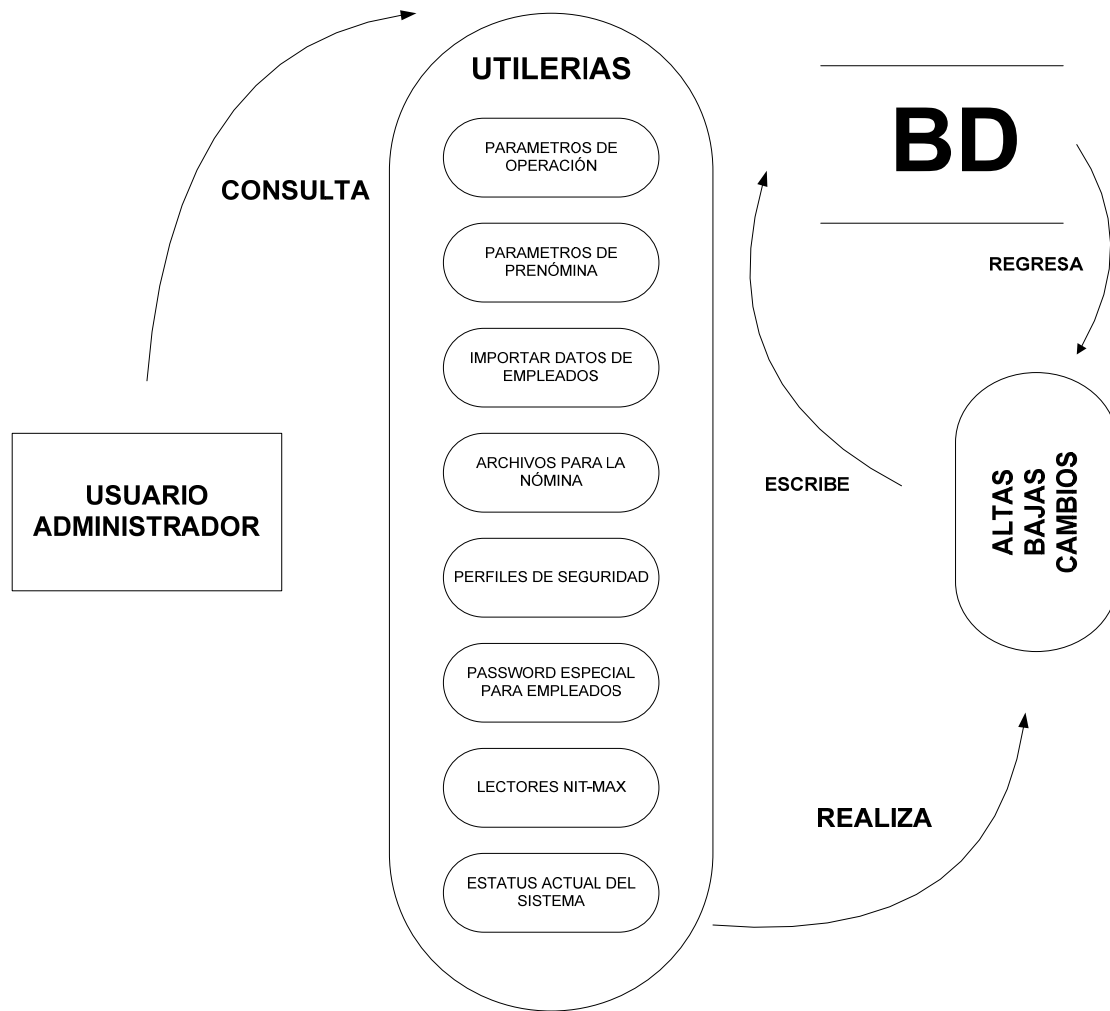
Figura IV.1.2.10 DFD del ACCYS TIME nivel 3, menú utilerías.
