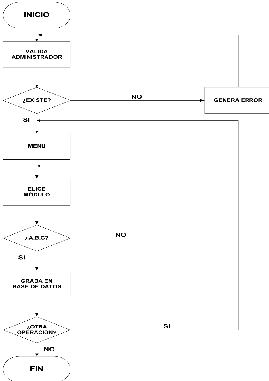
Figura IV.1.2.13 Diagrama de flujo tradicional del ACCYS TIME.
