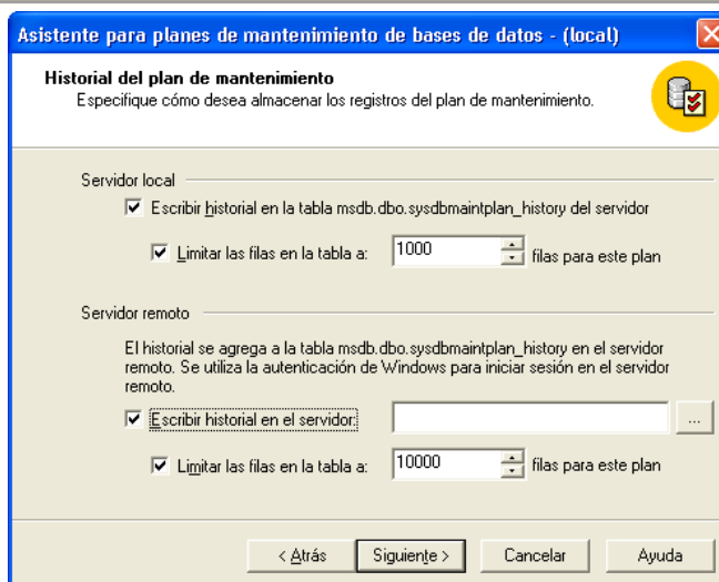
Figura 25. Pantalla de opción para el historial del plan de mantenimiento.
