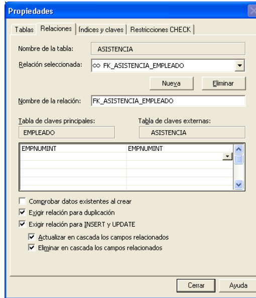
Figura IV.2.1.15 Columnas que relacionan las dos tablas
