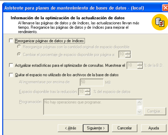
Figura 18. Ventana para la optimización de la actualización de datos
