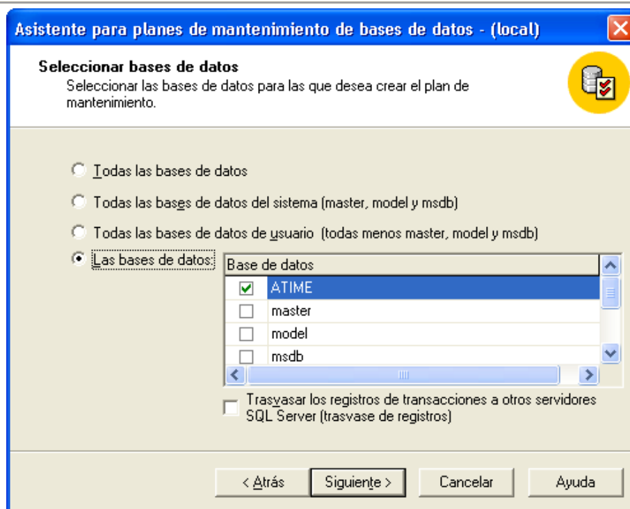
Figura 17. Ventana para la selección de base de datos.
