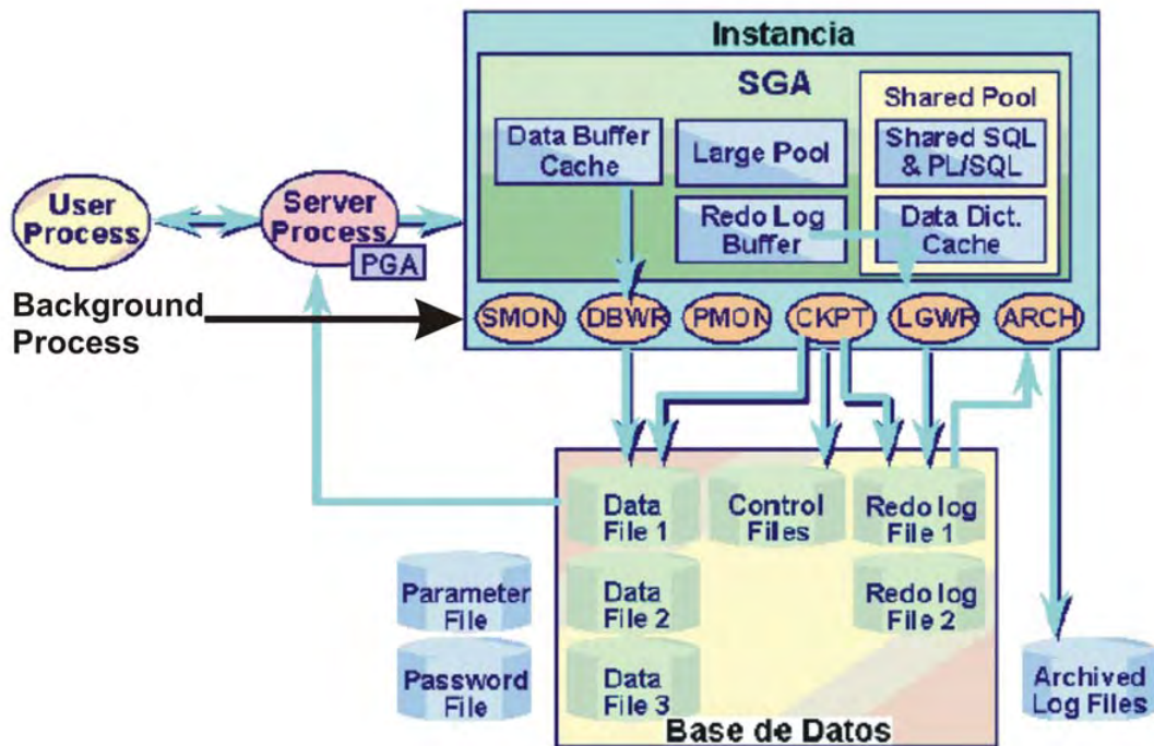
Figura III.4.1.1 Diagrama de la arquitectura de Oracle
