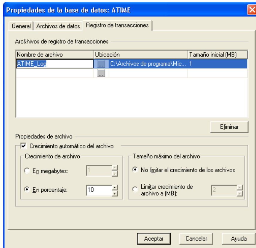
Figura IV.2.1.4. Ficha de registro de transacciones.
