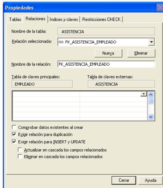
Figura IV.2.1.13 Generando una nueva relación
