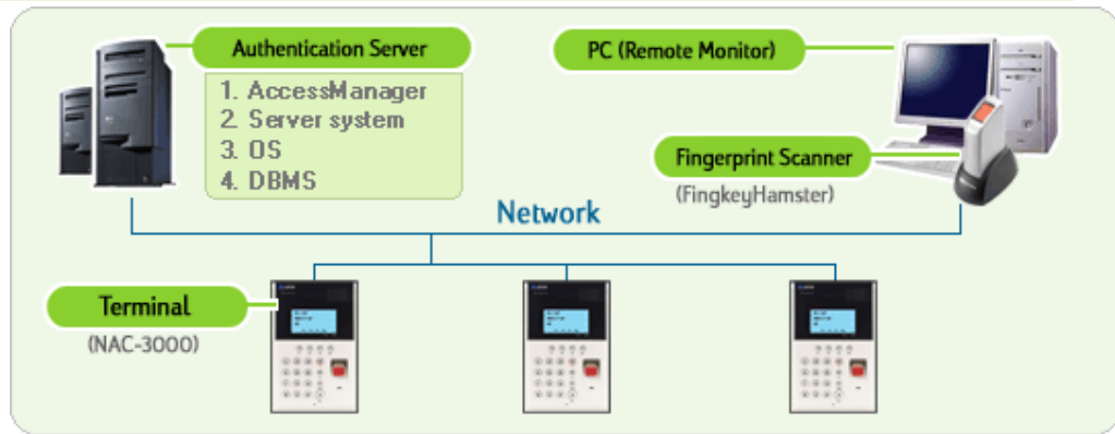
Figura II.2.4.1 Diagrama de solución.
