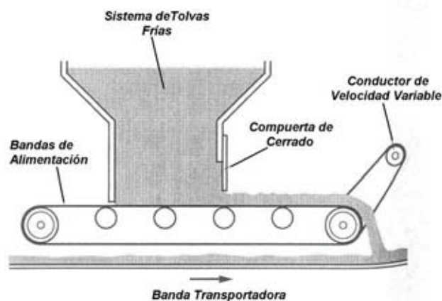
SISTEMA DE ALIMENTACIÓN EN FRÍO
