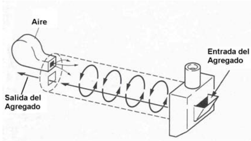
FLUJO Y MEZCLADO DEL AGREGADO
