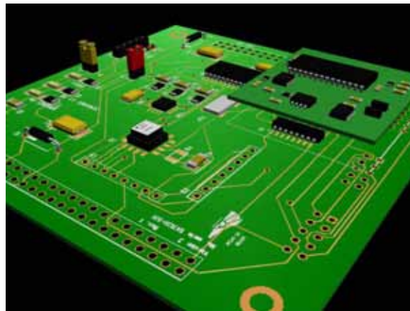
Figura 1.14. Modelo en realidad virtual del Subsistema de sensores.
