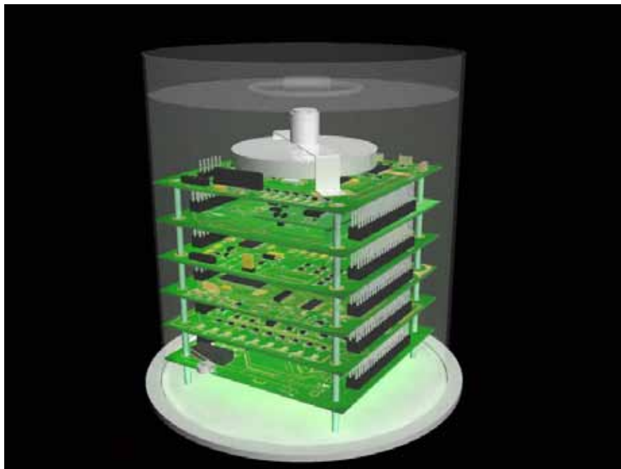
Figura 1.8. Modelo de SATEDU hecho con herramientas de realidad virtual.
