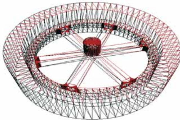
Figura 3.8. Figura compuesta (correspondiente a la rueda inercial de SATEDU).
