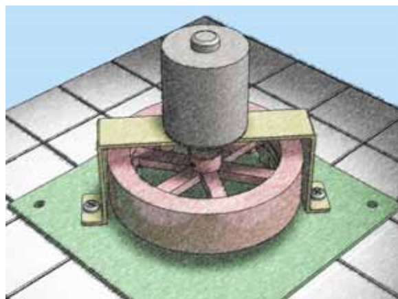
Figura 1.13. Bosquejo artístico del subsistema de estabilización por rueda inercial.
