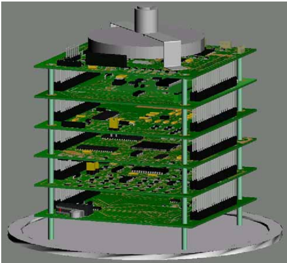
Figura 3.22. Réplica en realidad virtual del Satélite Educativo.
