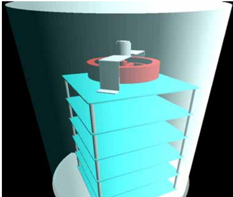
Figura 3.3. Modelo final de SATEDU para el módulo de seguimiento en tiempo real del software del SATERHUM.
