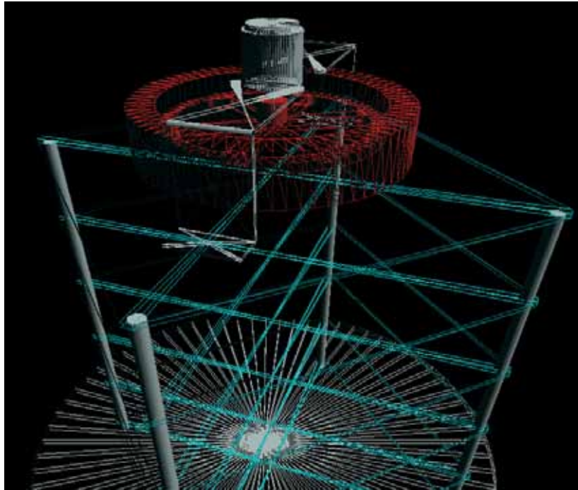
Figura 3.14. Modelo de SATEDU visualizando los triángulos que lo conforman.
