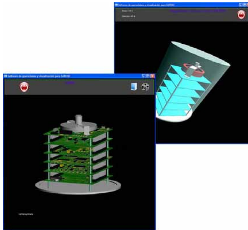
Figura 1.15. Software del SATERHUM.
