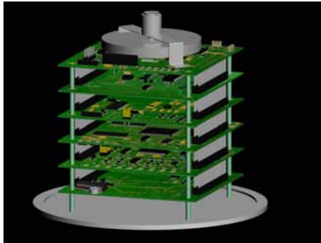
Figura 2.3. Modelo virtual detallado de SATDEDU.
