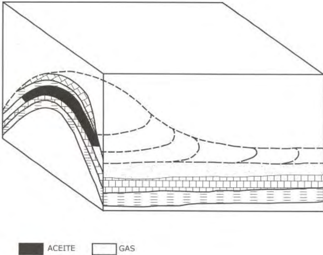
Figura 2.- Corte de una formación y representación en la misma de un yacimiento con acumulación de aceite y gas.
