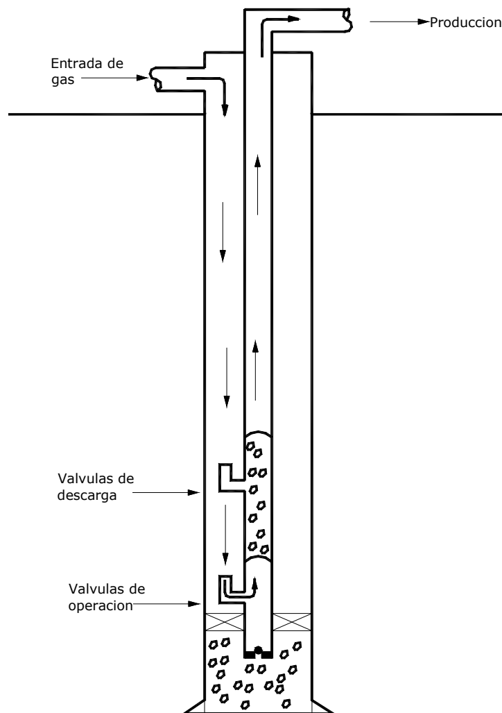
Figura 9.- Instalación cerrada adecuada para bombeo intermitente.
