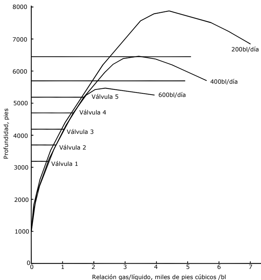
Figura 14.- Los gastos en la tubería de producción a las profundidades de las válvulas instaladas quedan por debajo de 200 y 600 bl/día.
