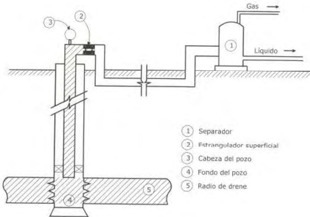
Figura 1.- Sistema Integral de producción.
