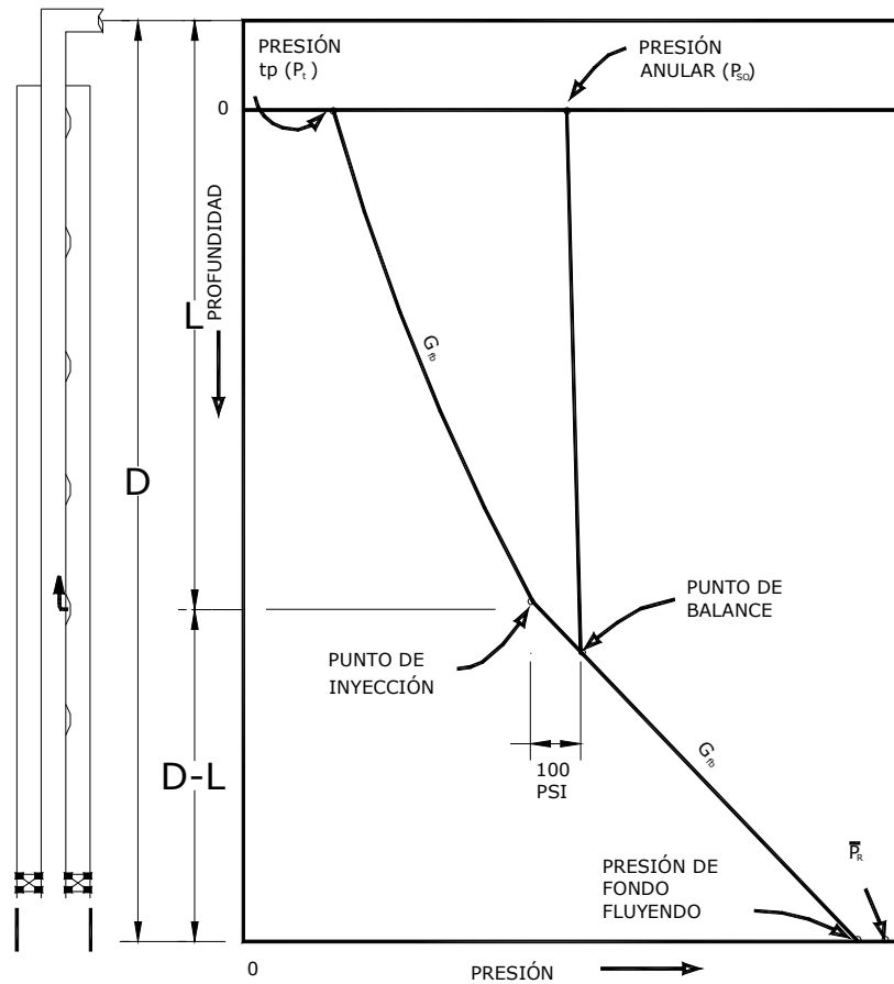
Figura 18.- Gradientes y presiones del recorrido de los fluidos hasta la superficie.
