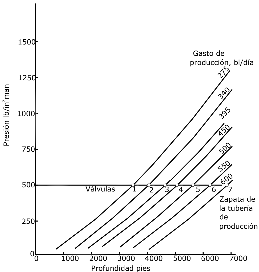
Figura 13.- Gasto de producción de 275 lb/día en la primera válvula.
