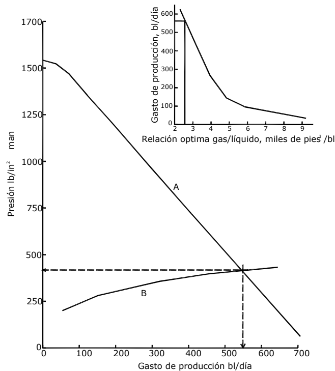
Figura 15.- La intersección de las curvas A y B muestra que el pozo producirá a 545 bl/día, la presión opuesta a la válvula 6 es de 410 lb/in 2 . La gráfica pequeña muestra que con un gasto de 545 bl/día por una tp de 2 7/8 in, la RGL óptima es de 2.6 mil pies cúbicos/bl.
