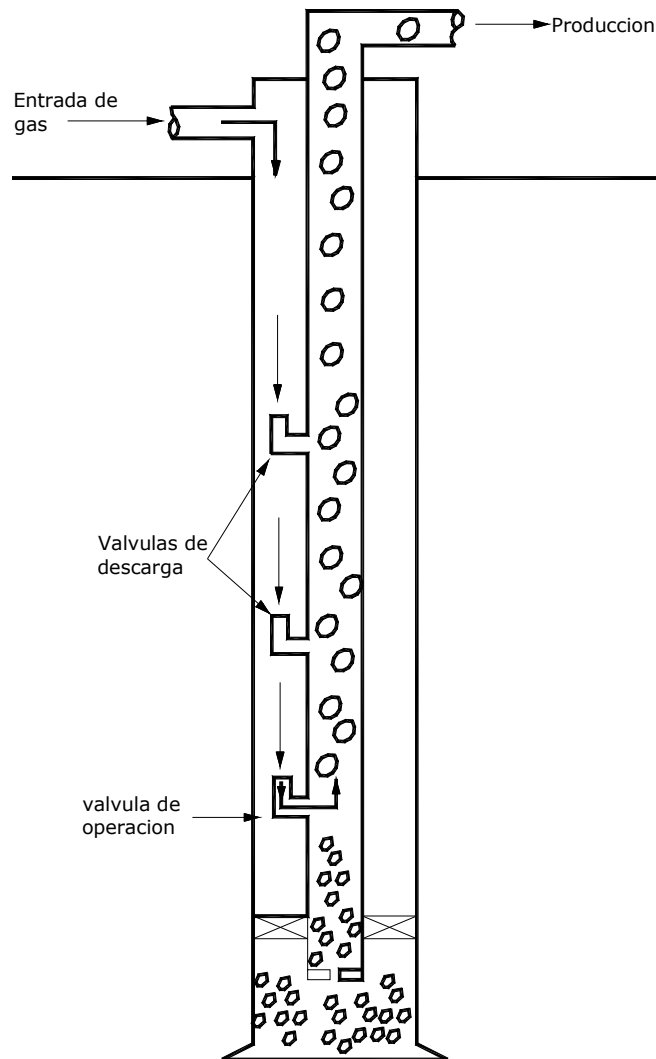
Figura 8.- Instalación semi-cerrada adecuada para flujo constante e intermitente.
