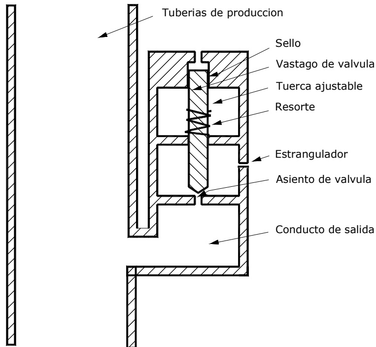
Figura 10.- Válvula diferencial se usa en pozos poco profundos y de baja producción.
