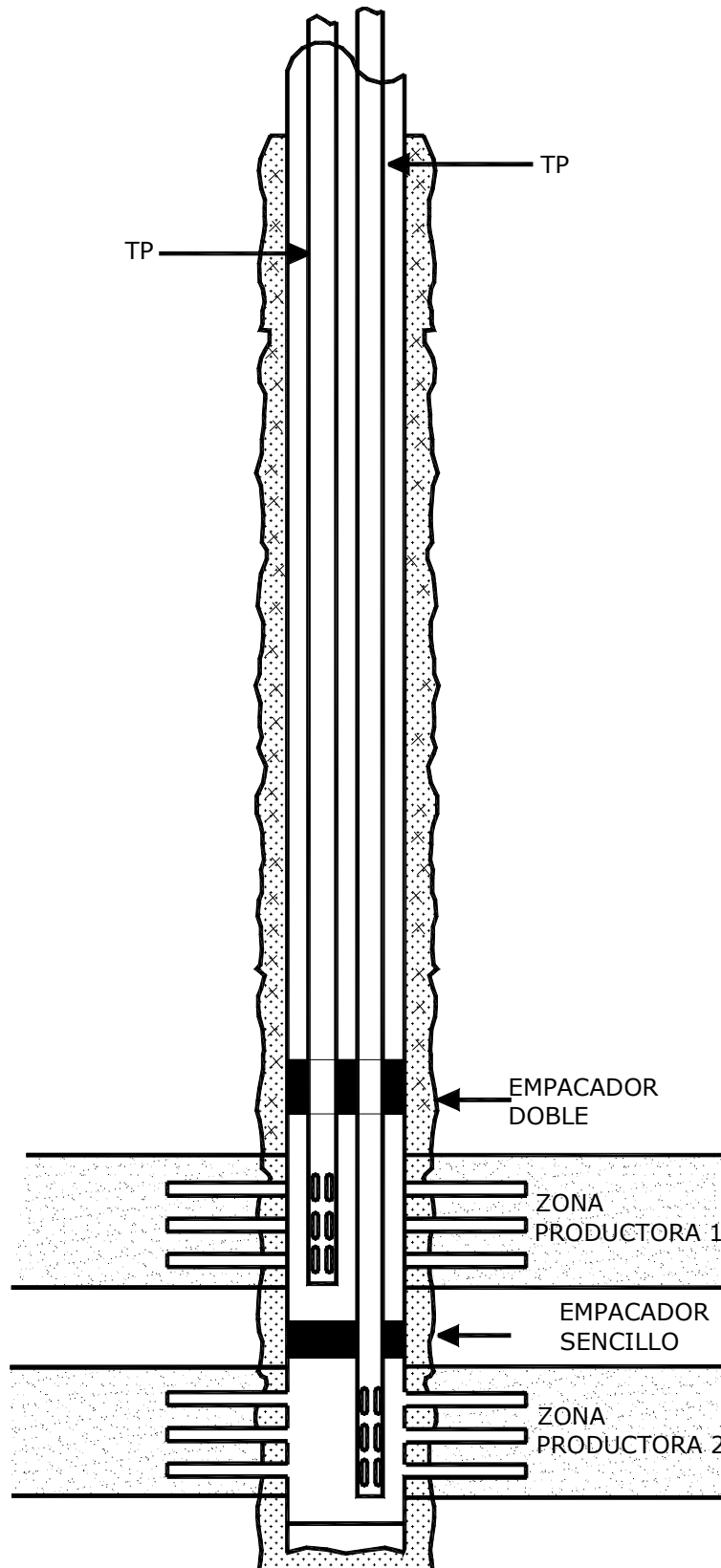
Figura 4.- Nótese las dos zonas productoras con sus respectivos empacadores; uno doble y el otro sencillo.
