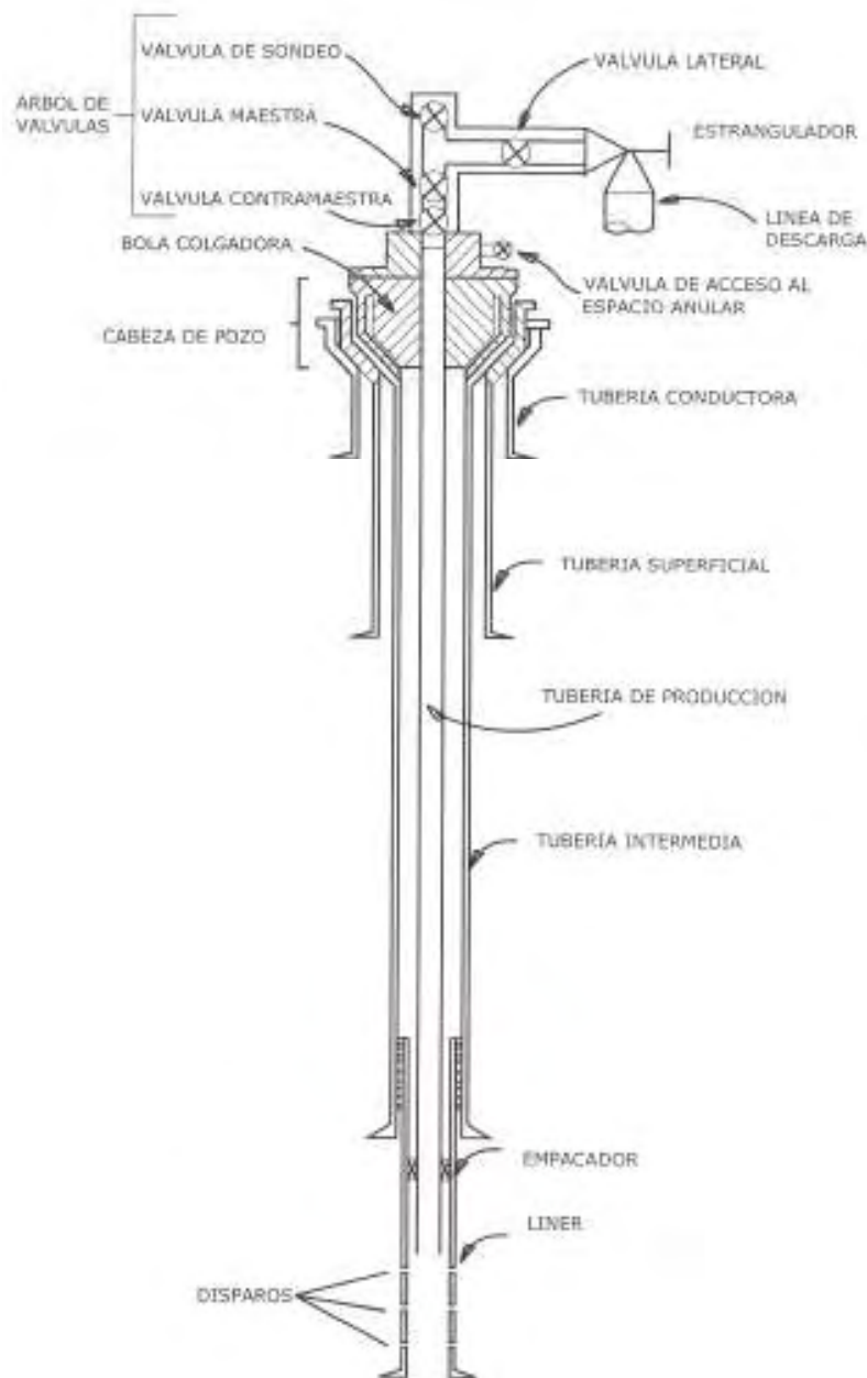
Figura 3.-. Sarta de producción.
