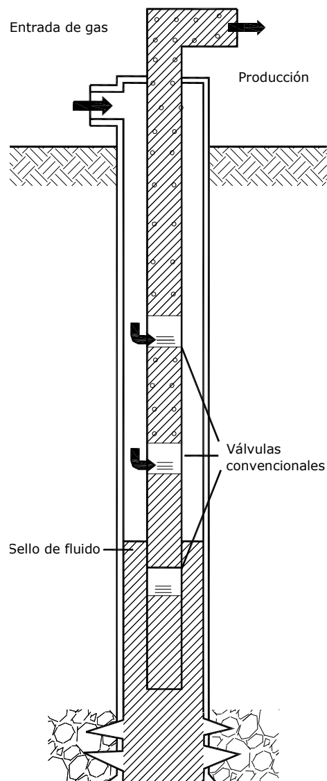
Figura 7.- Instalaciones abiertas se usan para flujo continuo e intermitente.
