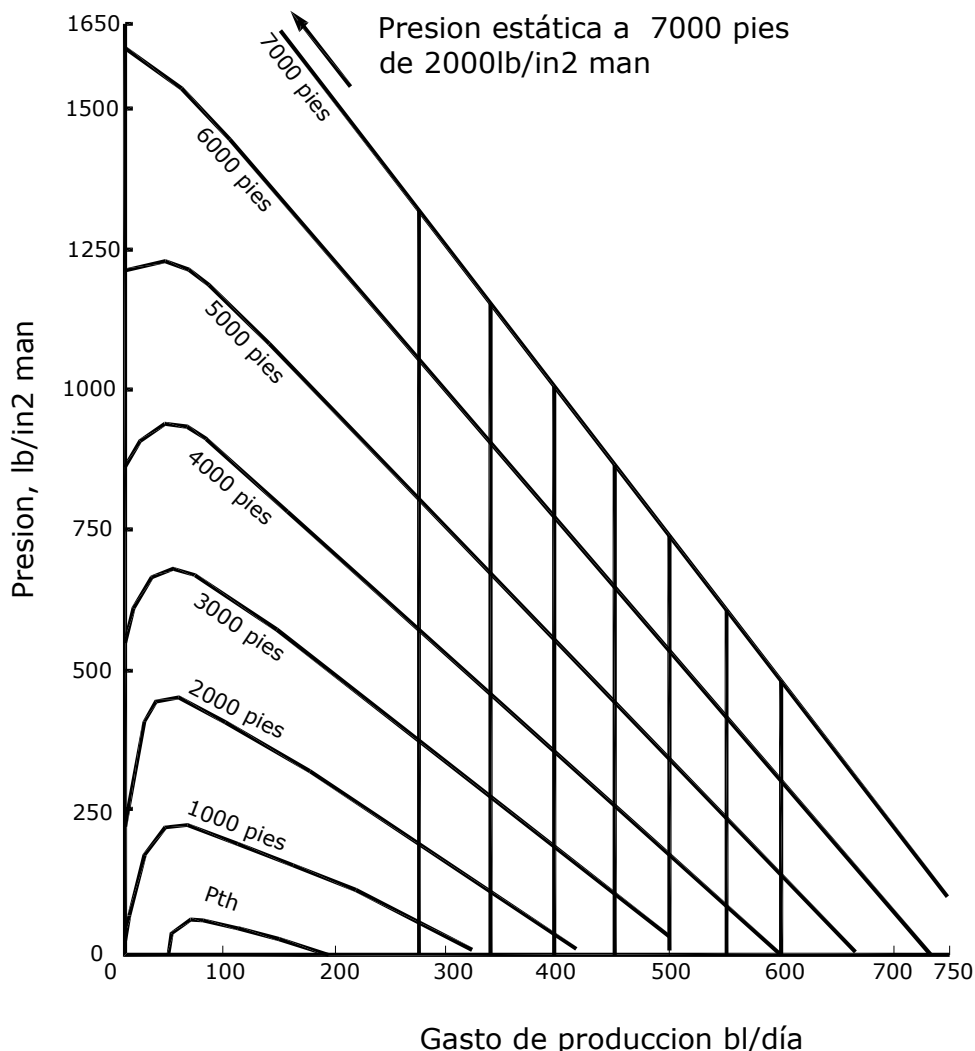
Figura 11.- En la tubería de producción a diversas profundidades (presión estática a 7000 pies de 2000 lb/in 2 man.).
