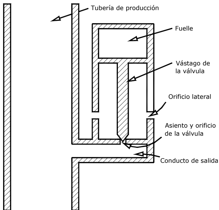
Figura 16.- Válvula con fuelle cargado a presión también llamada de flujo intermitente, se usa para flujo constante e intermitente.
